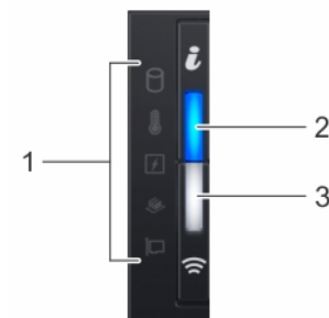
Abbildung 5. Linkes Bedienfeld mit optionaler iDRAC-Quick-Sync-2.0-Anzeige
