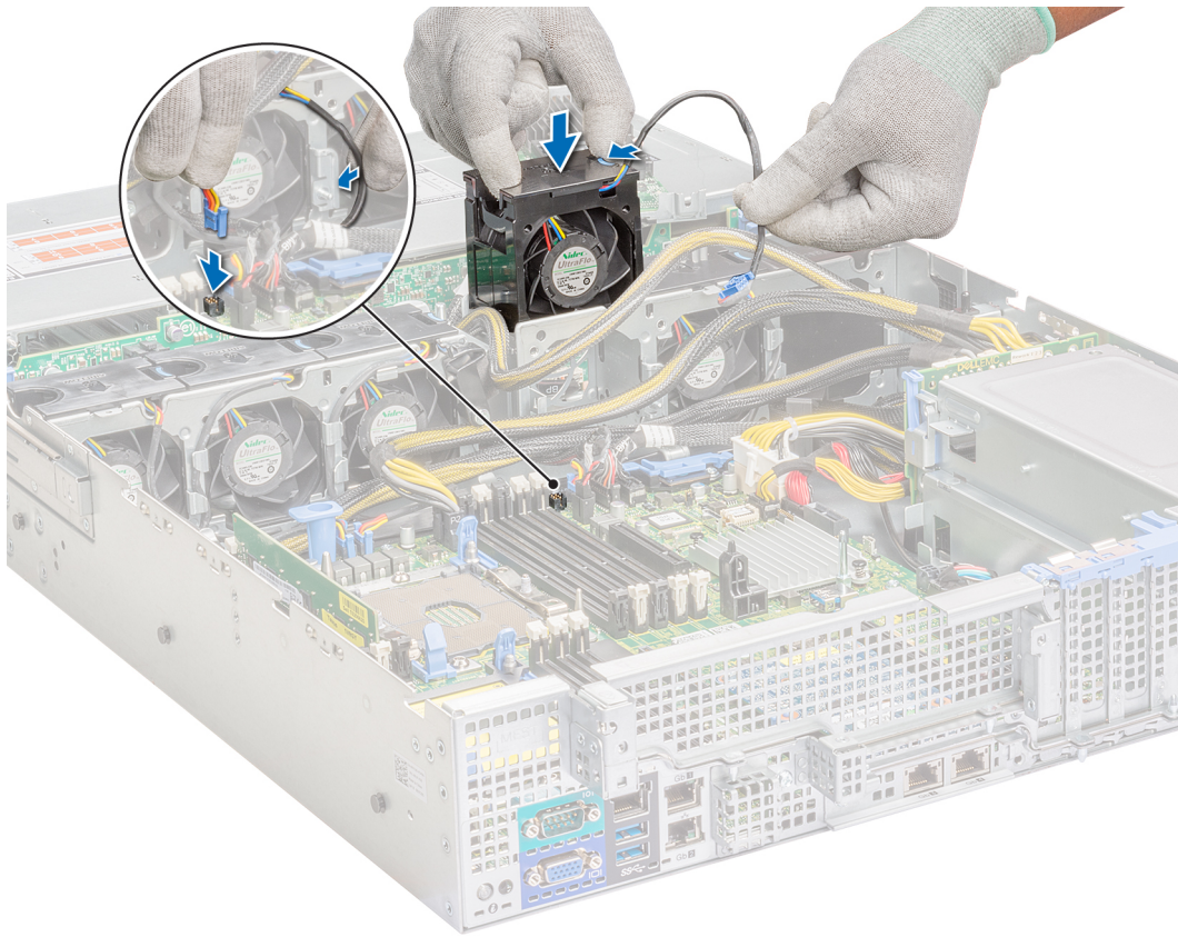
Abbildung 35. Installieren des Lüfters
