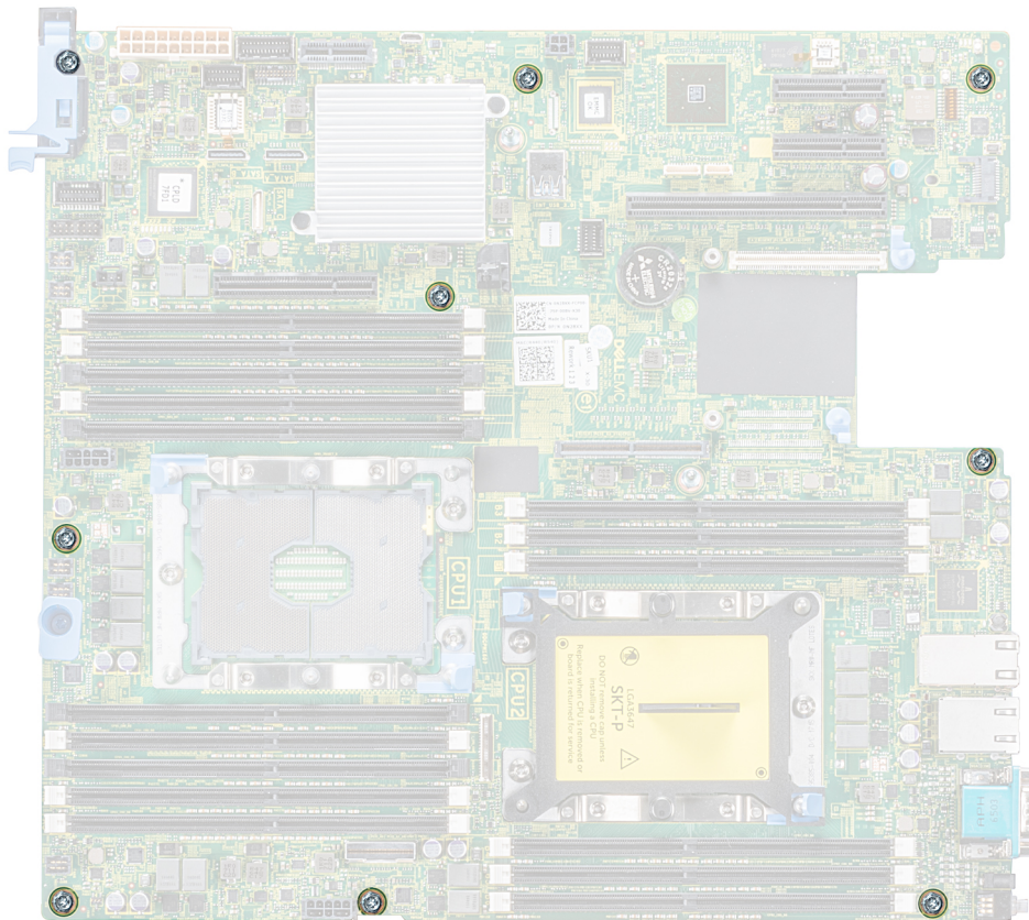
Abbildung 125. Schrauben der Systemplatine
