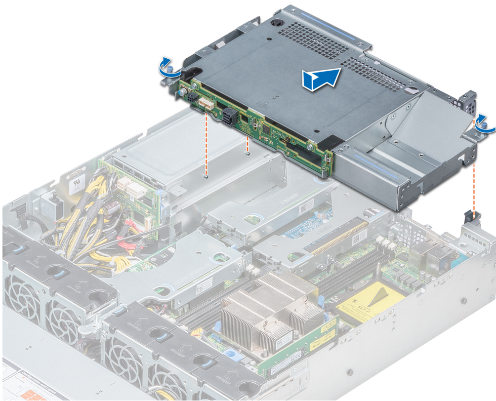
Abbildung 108. Einsetzen des hinteren Laufwerksgehäuses
