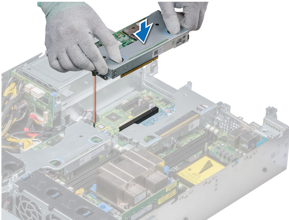
Abbildung 86. Einbauen des linken Risers mit flachem Profil
