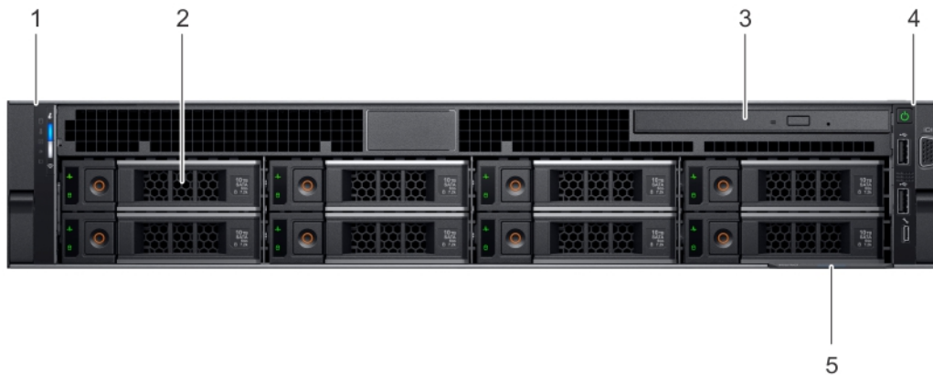
Abbildung 3. Frontansicht eines Systems mit 8 x 3,5-Zoll-Laufwerken
