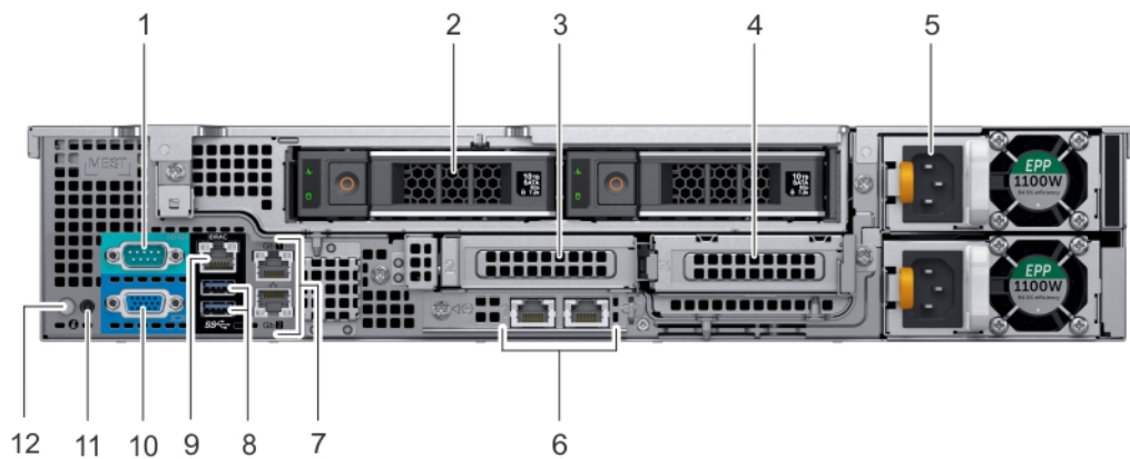
Abbildung 9. Rückseitenmerkmale eines Systems mit 12 x 3,5-Zoll- + 2 x 3,5-Zoll Laufwerken (hinten)
