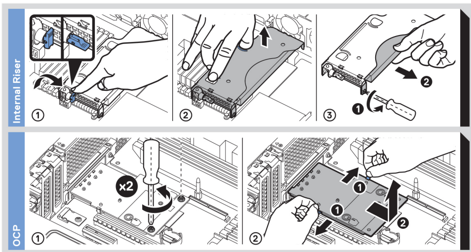
Abbildung 19. Installation von OCP und des internen PERC-Risers
