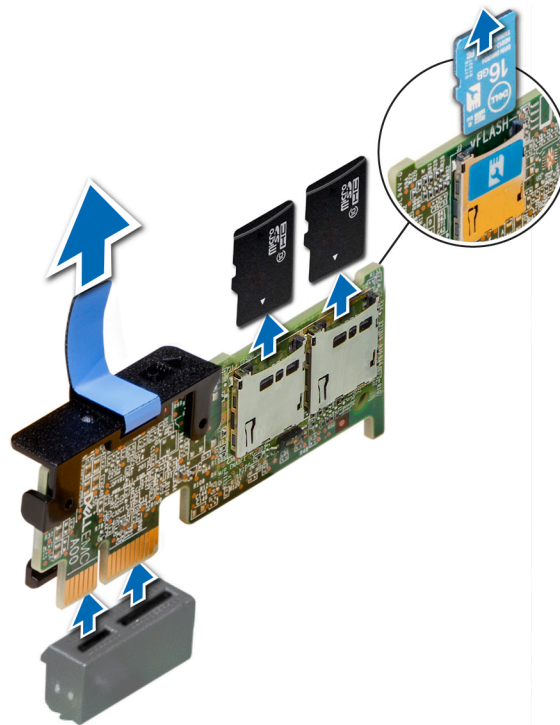
Abbildung 91. Entfernen der optionalen IDSDM-/vFlash-Karte
