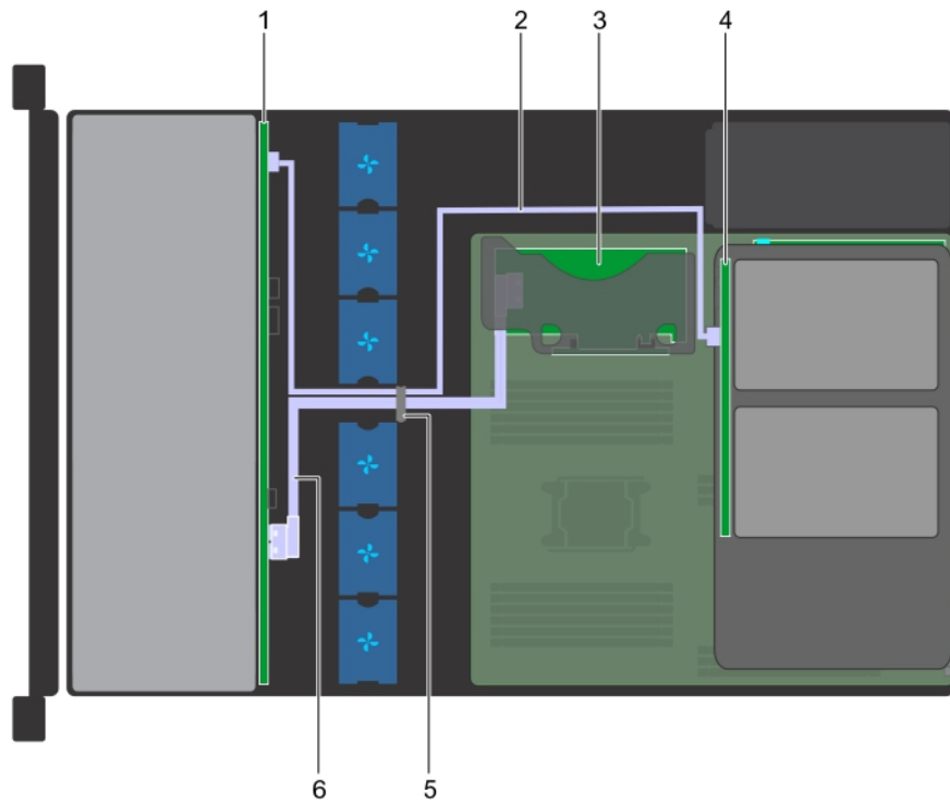
Abbildung 103. Kabelführung – 12 x 3,5-Zoll-Laufwerksrückwandplatte und hintere 2 x 3,5-Zoll-Laufwerksrückwandplatte mit internem PERC-Riser
