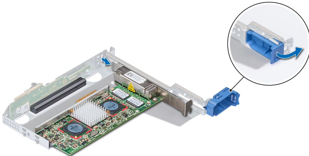
Abbildung 65. Entfernen einer Erweiterungskarte aus einem Riser mit flachem Profil
