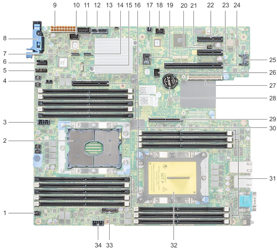
Abbildung 129. Jumper und Anschlüsse auf der Systemplatine
