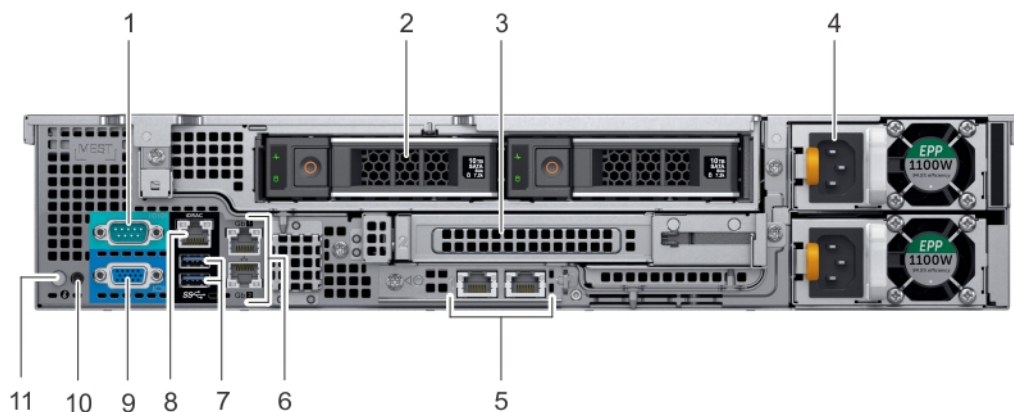
Abbildung 10. Rückseitenmerkmale eines Systems mit 12 x 3,5-Zoll- + 2 x 3,5-Zoll Laufwerken (hinten)
