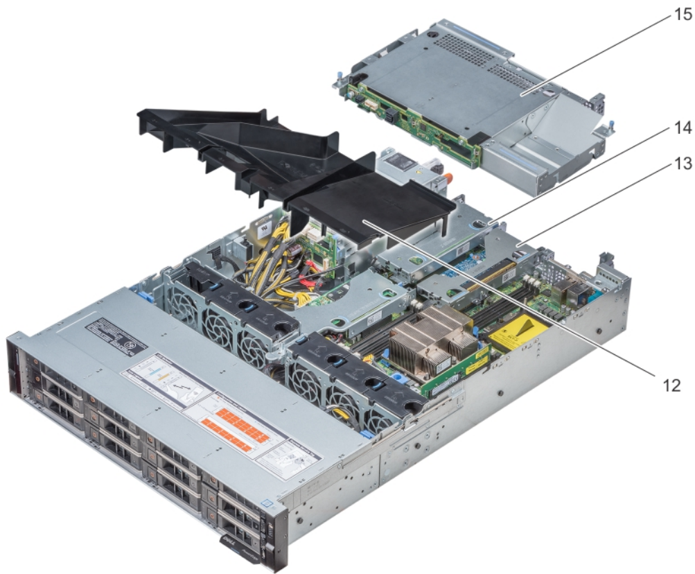
Abbildung 30. Im Inneren des Systems mit hinterem Laufwerksgehäuse
