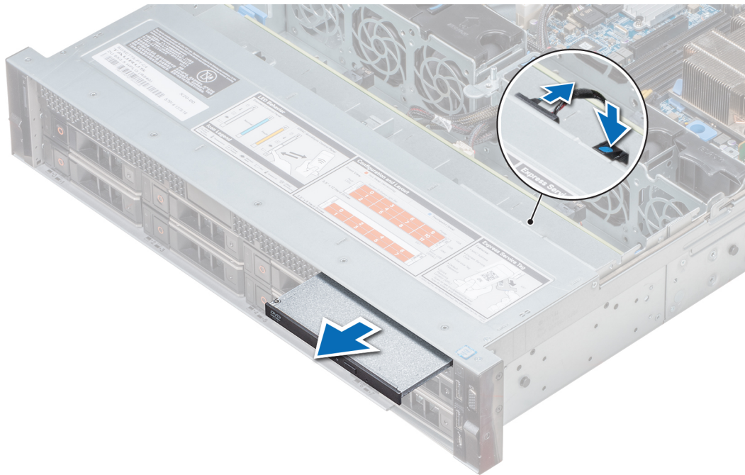
Abbildung 111. Entfernen des optischen Laufwerks
