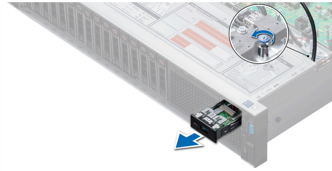
Abbildung 123. Entfernen des USB 3.0-Moduls
