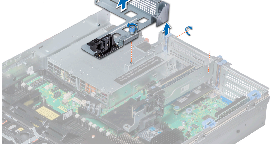
Abbildung 77. Entfernen des Platzhalters für Riser 3
