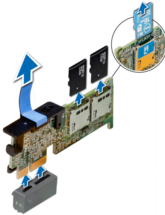
Abbildung 62. Entfernen der optionalen vFlash SD-Karte
