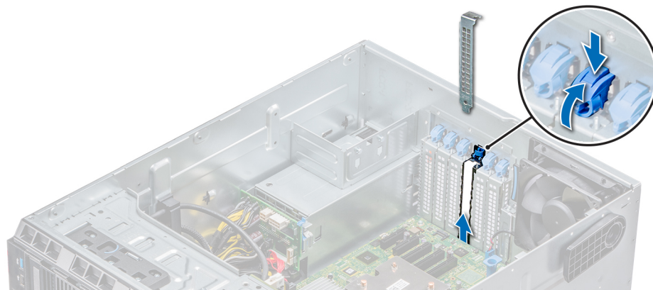
Abbildung 60. Entfernen des Abdeckblechs
