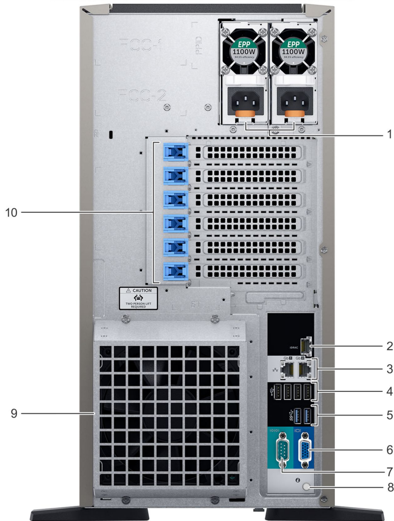
Abbildung 9. Rückseite des Systems mit optionalem redundantem Kühlungsüfler
