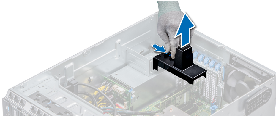
Abbildung 56. Entfernen des Erweiterungskartenhalters
