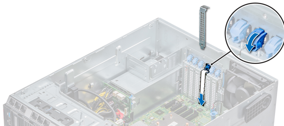
Abbildung 59. Einsetzen des Abdeckblechs
