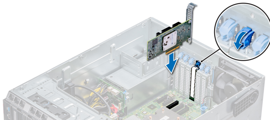
Abbildung 61. Installieren einer Erweiterungskarte
