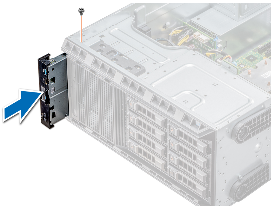
Abbildung 83. Installieren der Bedienfeldbaugruppe
