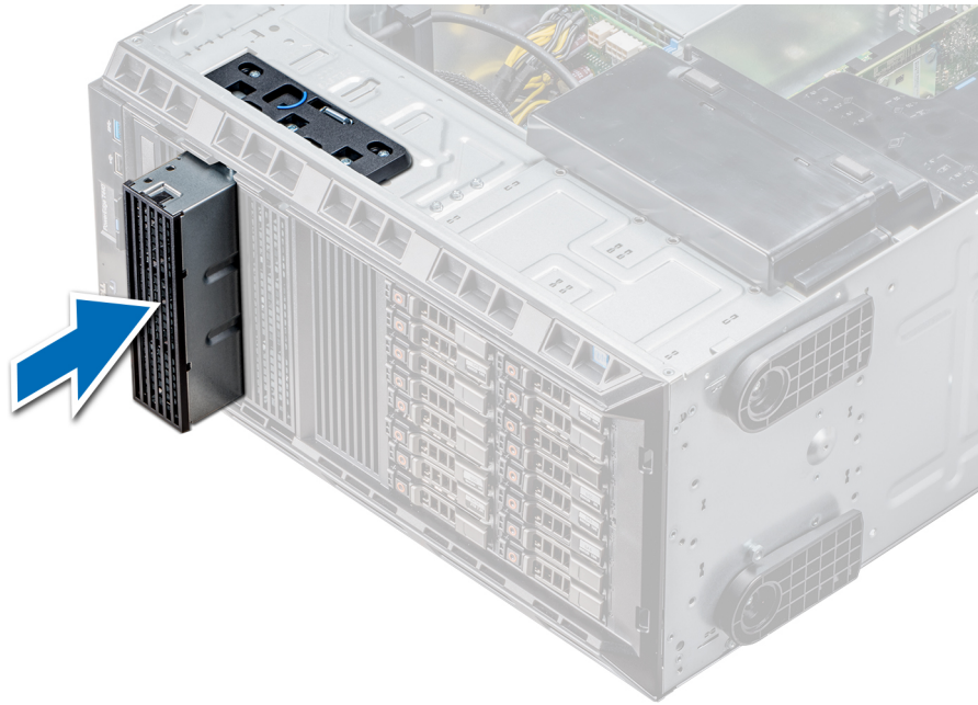
Abbildung 34. Installieren des Platzhalters für optische Laufwerke oder Bandlaufwerke
