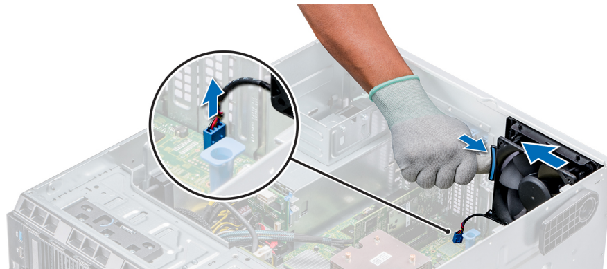
Abbildung 52. Entfernen des internen Lüfters
