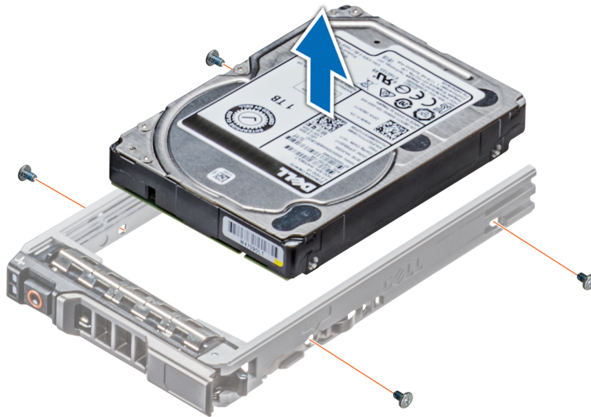
Abbildung 27. Entfernen des Laufwerks aus dem Laufwerksträger
