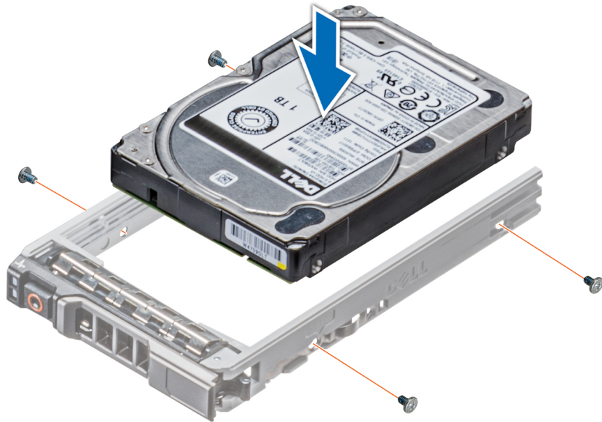
Abbildung 28. Installieren eines Laufwerks im Laufwerksträger
