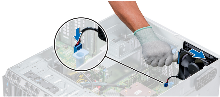
Abbildung 53. Installieren des internen Lüfters
