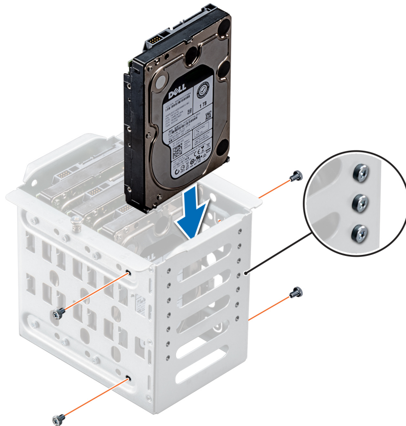
Abbildung 40. Installieren eines verkabelten Laufwerks
