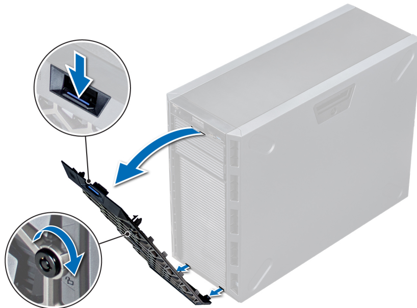
Abbildung 13. Entfernen der Frontverkleidung
