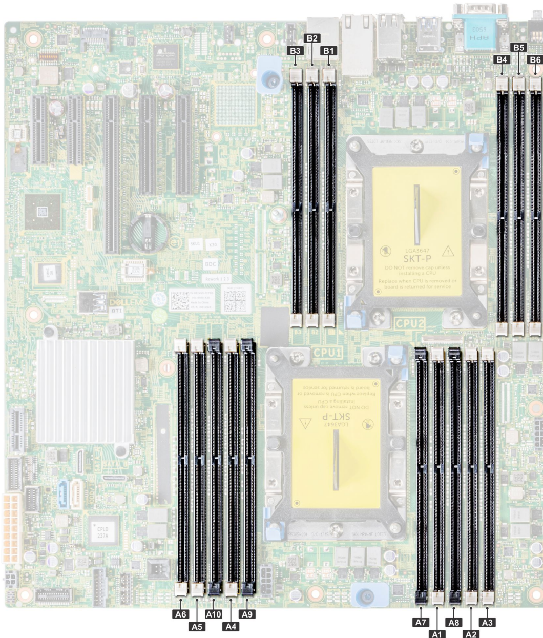
Abbildung 49. Draufsicht Systemspeicher
