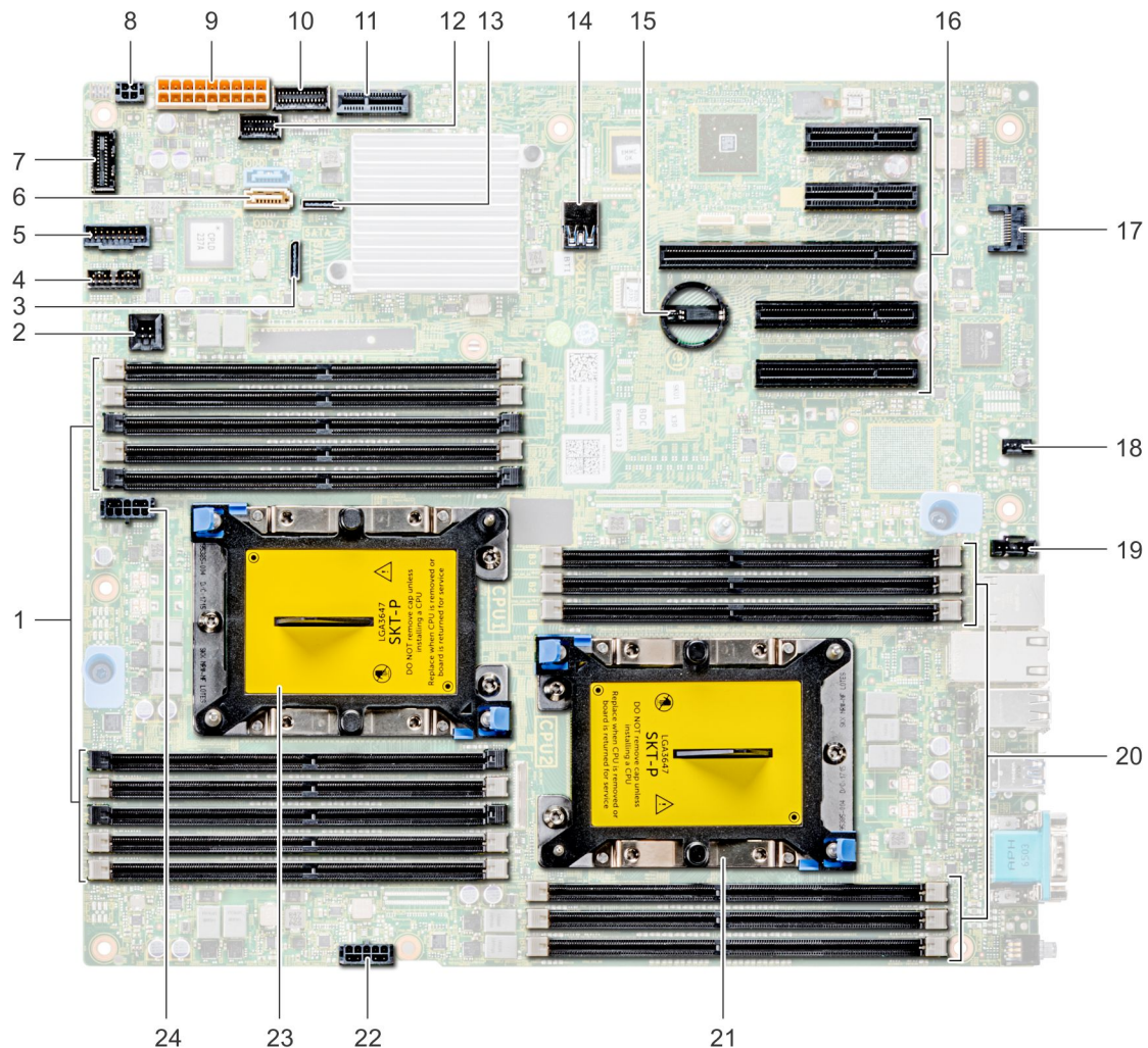
Abbildung 89. Jumper und Anschlüsse auf der Systemplatine des T440
