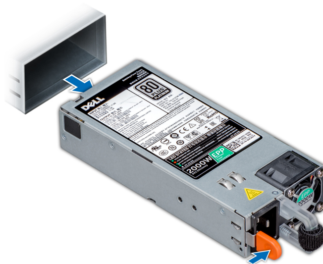
Abbildung 73. Entfernen einer Netzteilinheit
