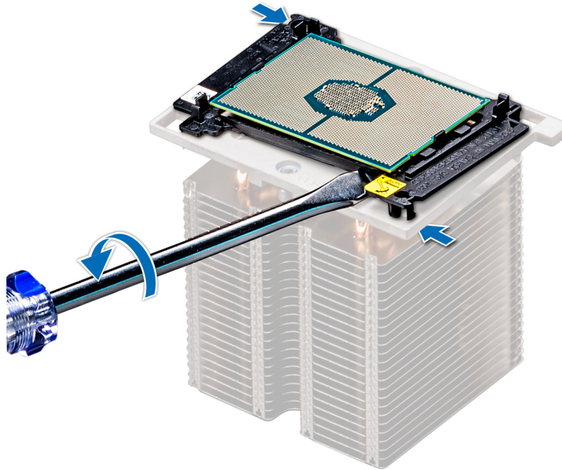
Abbildung 65. Das Lösen der Prozessorhalterung
