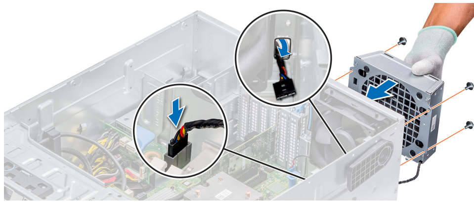
Abbildung 55. Installieren des externen Lüfters
