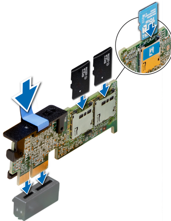
Abbildung 63. Installieren optionaler IDSDM- oder vFlash-Karten
