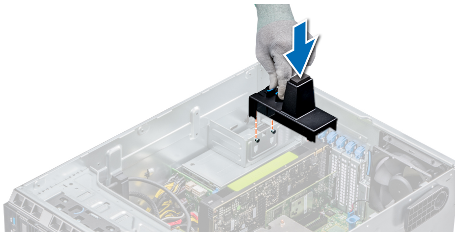
Abbildung 57. Installieren des Erweiterungskartenhalters
