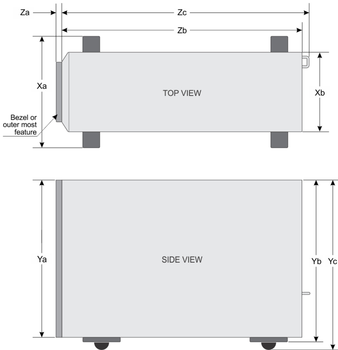
Abbildung 12. Übersicht über die Abmessungen des PowerEdge T440-Systems
