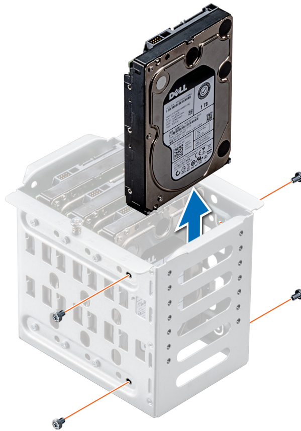
Abbildung 39. Entfernen eines verkabelten Laufwerks
