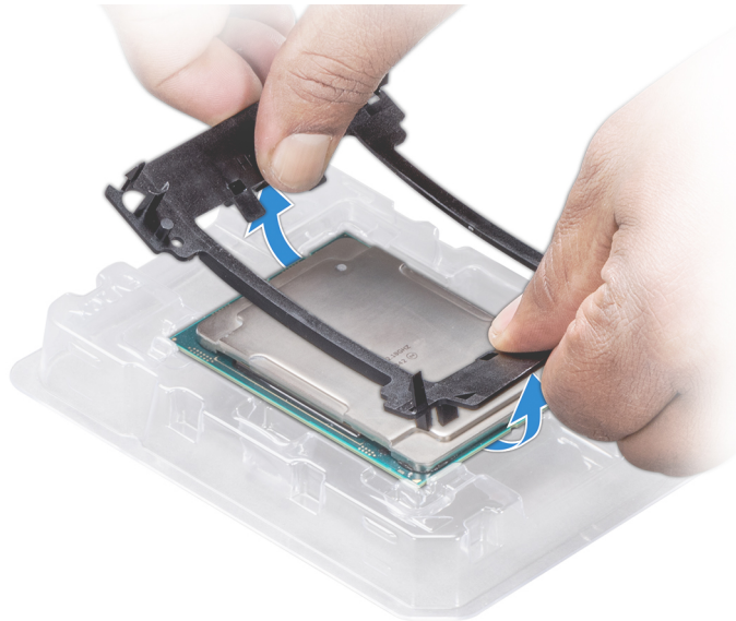
Abbildung 66. Entfernen der Prozessorhalterung
