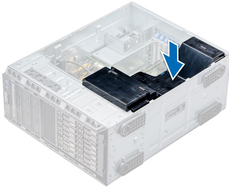
Abbildung 22. Installieren des Kühlgehäuses
