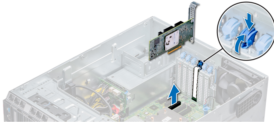
Abbildung 58. Entfernen einer Erweiterungskarte
