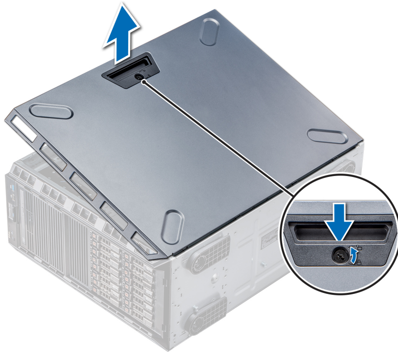
Abbildung 19. Entfernen der Systemabdeckung
