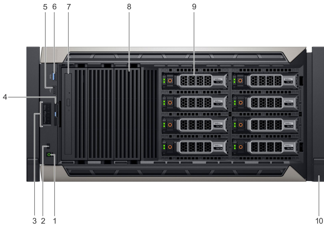
Abbildung 4. Frontblende eines mit acht Hot-Swap-fähigen 3,5-Zoll-Laufwerken ausgestatteten Systems im Rack-Modus
