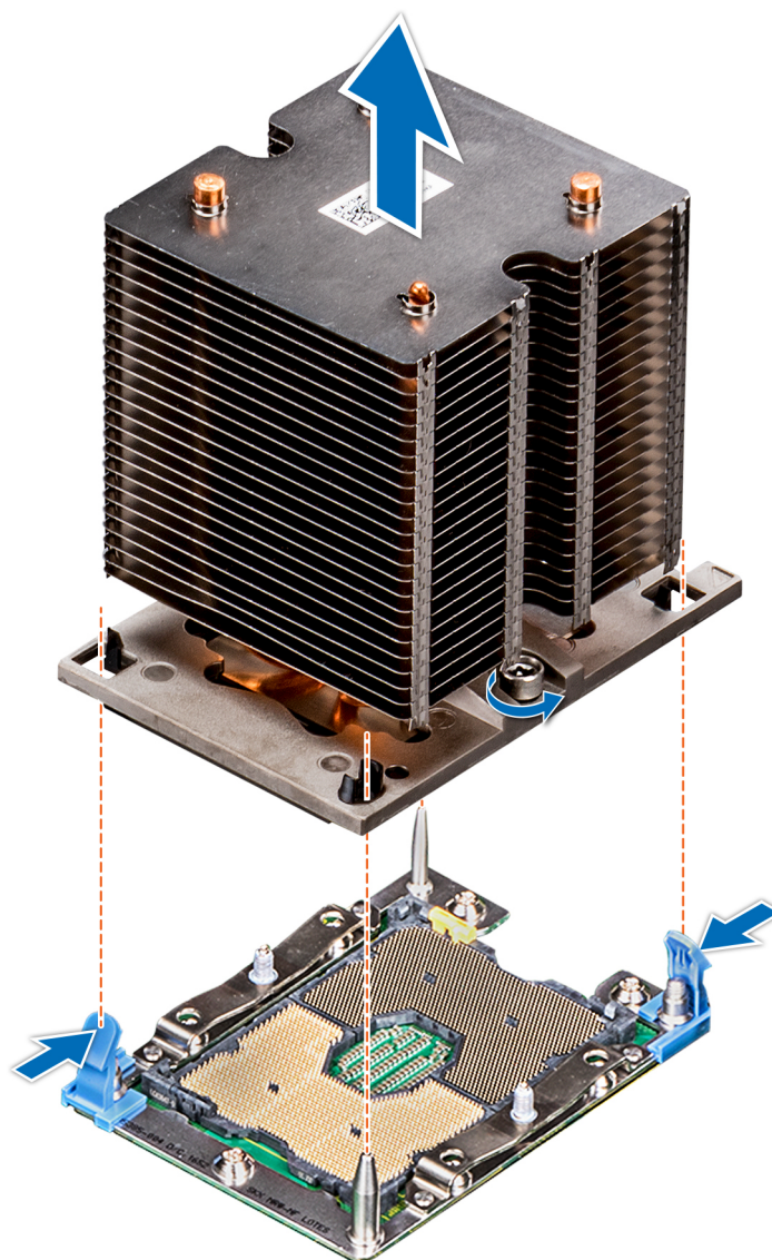
Abbildung 64. Entfernen des Prozessor- und Kühlkörpermoduls
