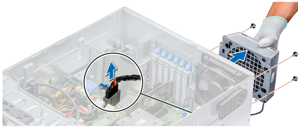
Abbildung 54. Entfernen des externen Lüfters
