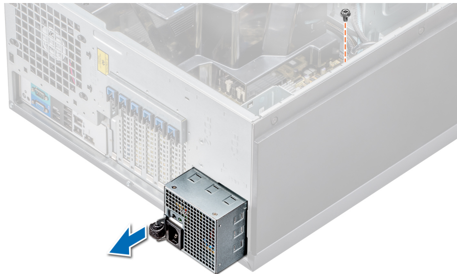
Abbildung 75. Entfernen eines verkabelten Netzteils
