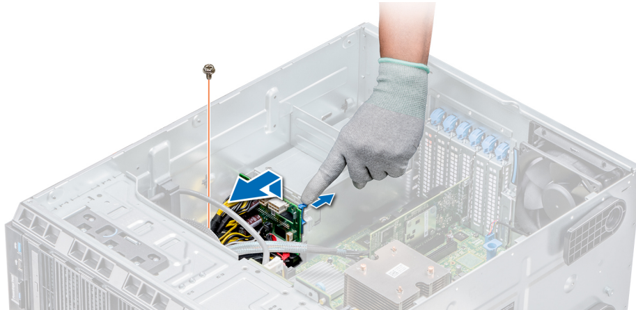
Abbildung 77. Entfernen der Stromzwischenplatine
