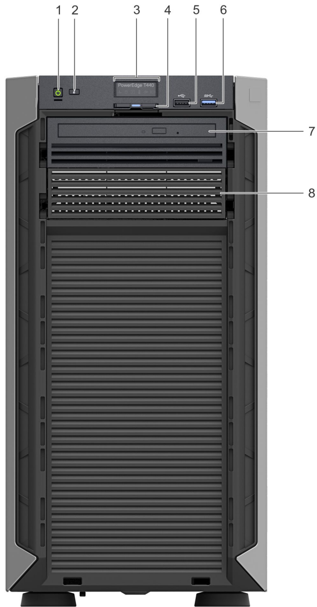
Abbildung 2. Frontblende eines Systems mit vier verkabelten 3,5-Zoll-Laufwerken
