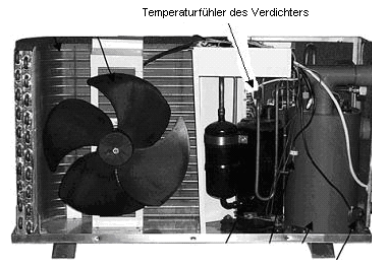
Abbildung 27: Temperaturfühler des Verdichters.
