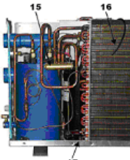
Abbildung 1: Hauptkomponenten der Wärmepumpe.
