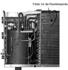
Abbildung 23: Fühler für die Raumtemperatur.
