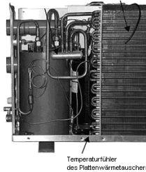
Abbildung 26: Temperaturfühler des Plattenwärmetauschers.
