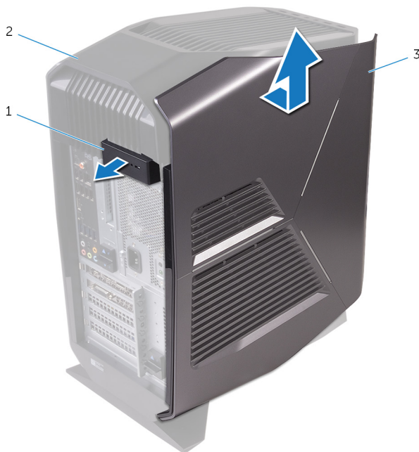
Figure 2. Retrait du panneau latéral gauche
