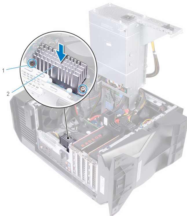
Figure 23. Remise en place du dissipateur de chaleur du régulateur de tension
