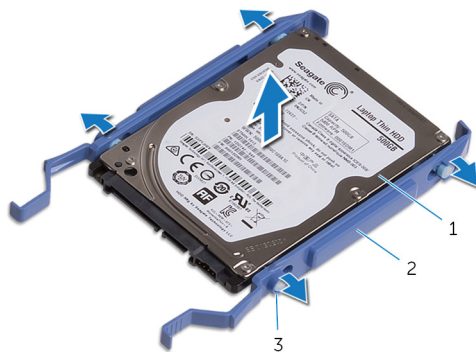
Figure 16. Retrait d'un disque dur de son support
