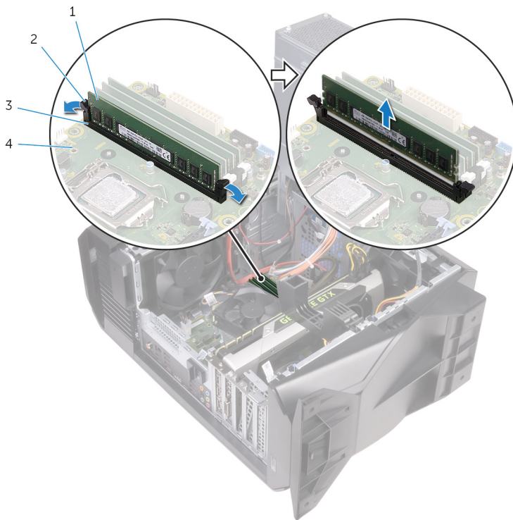
Figure 25. Retrait du module de mémoire
