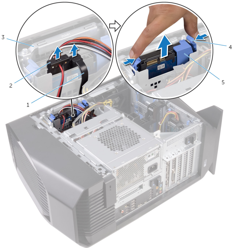
Figure 13. Retrait du disque dur
