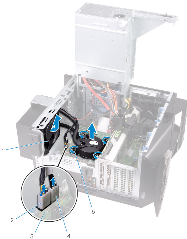
Figure 21. Retrait du bloc de refroidissement du processeur
