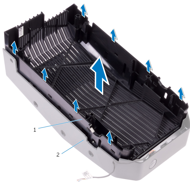
Figure 11. Soulèvement du panneau supérieur du cadre supérieur de l'ordinateur
