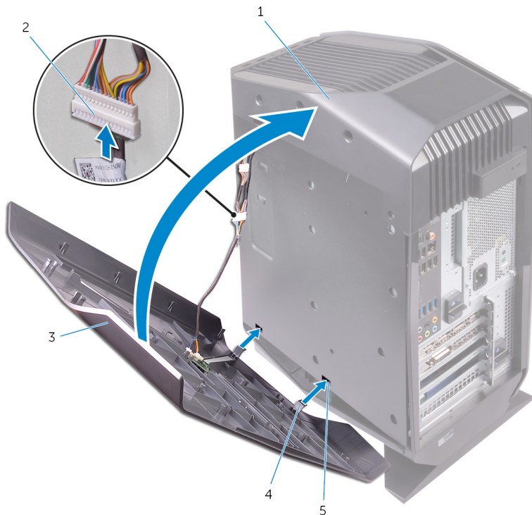
Figure 6. Branchement du câble d'éclairage
