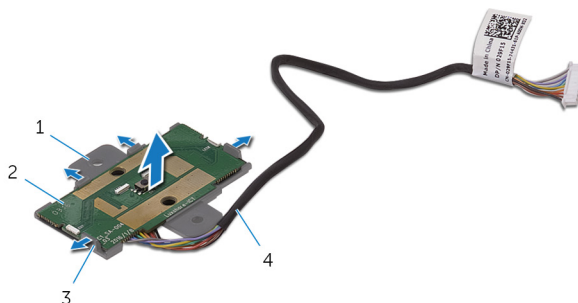
Figure 48. Retrait du module du bouton d'alimentation
