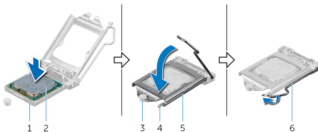
Figure 32. Remplacement du processeur
