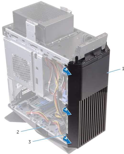
Figure 45. Retrait du cadre avant
