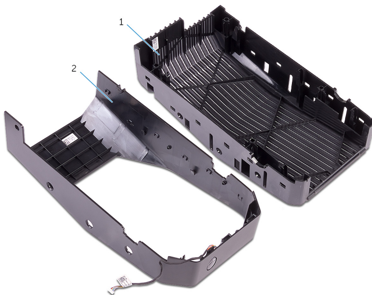
Figure 12. panneau supérieur et cadre supérieur
