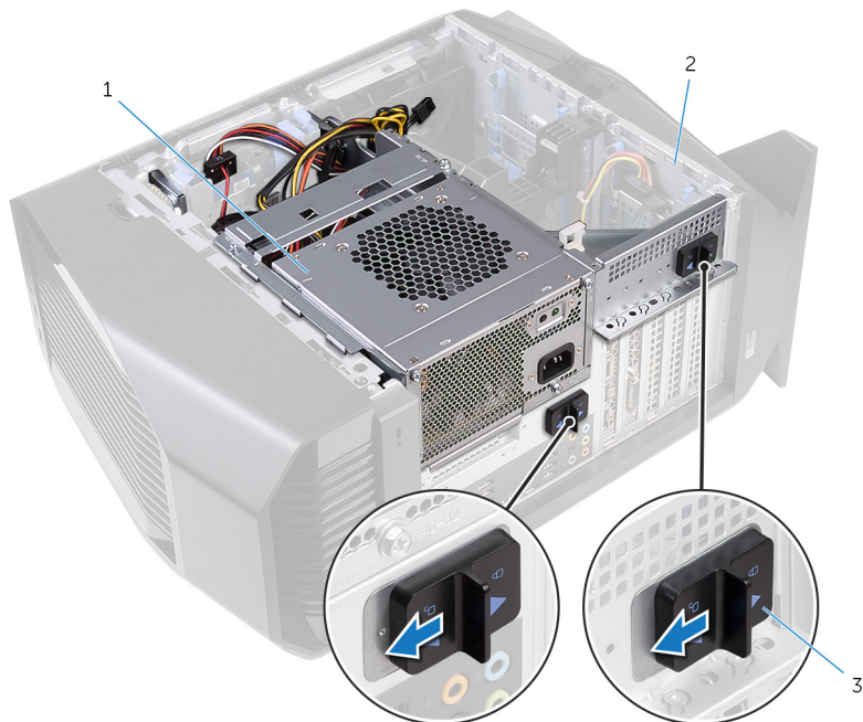
Figure 18. Faire glisser les loquets de verrouillage du bâti du bloc d'alimentation
