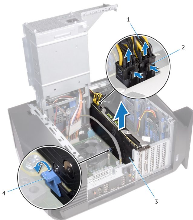
Figure 28. Retrait de la carte graphique
