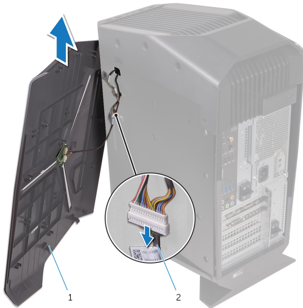
Figure 5. Retrait du panneau latéral droit
