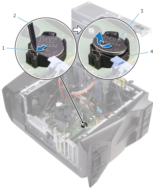
Figure 24. Retrait de la pile bouton
