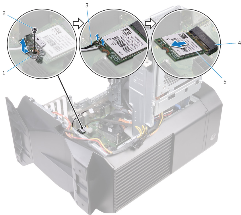
Figure 33. Retrait de la carte sans fil
