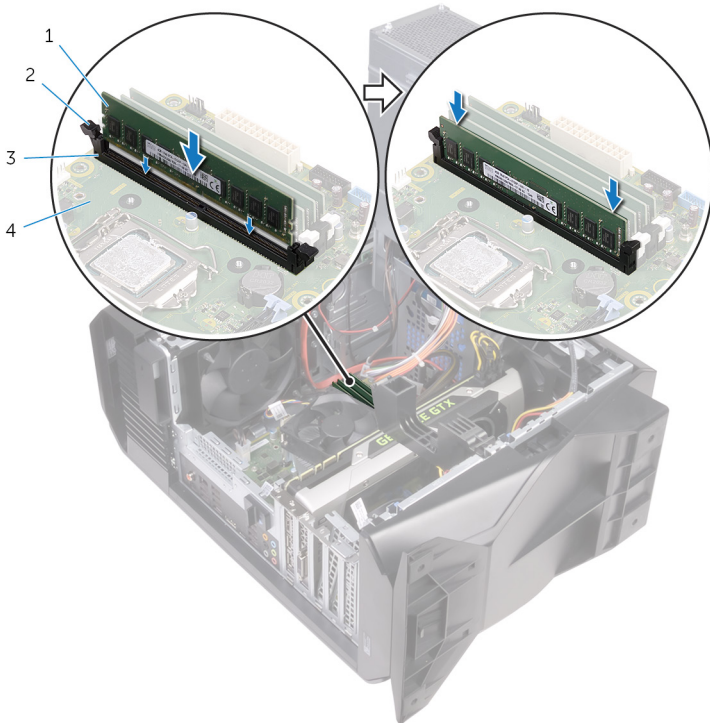
Figure 26. Remise en place du module de mémoire
