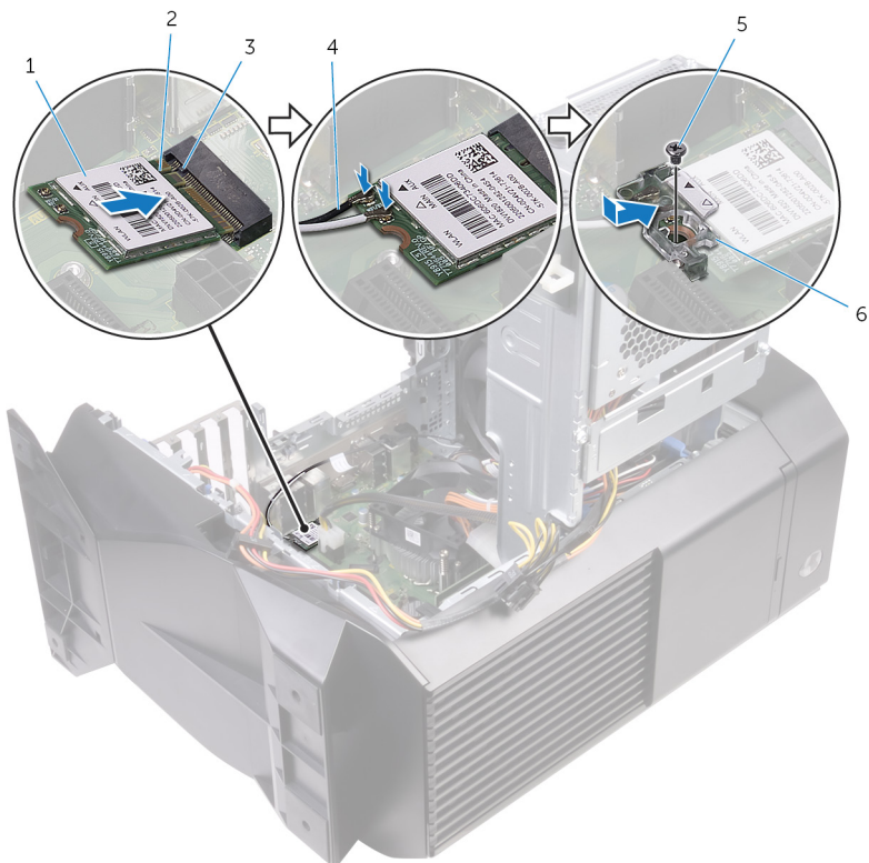
Figure 34. Remise en place de la carte sans fil
