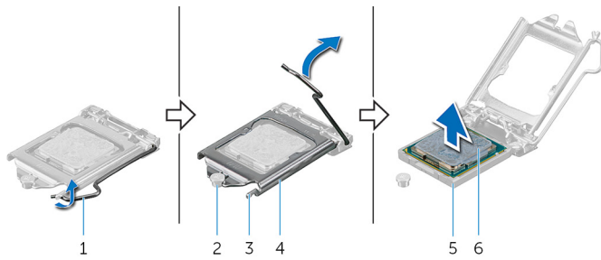
Figure 31. Retrait du processeur
