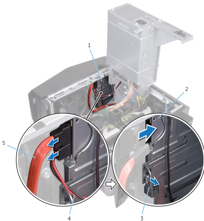
Figure 41. Déconnectez le câble d'alimentation et le câble de données
