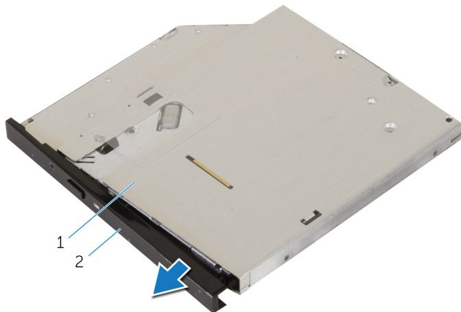
Figure 44. Retrait du lecteur optique
