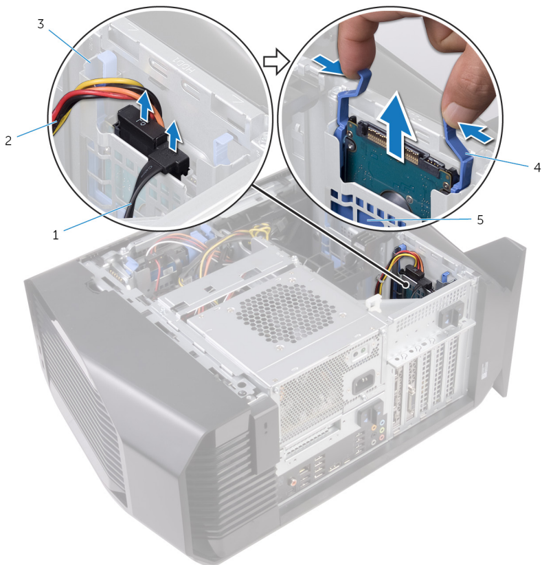
Figure 15. Retrait du disque dur
