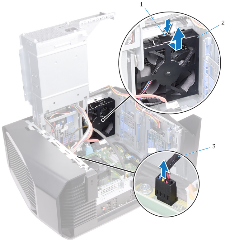
Figure 37. Retrait du ventilateur du châssis
