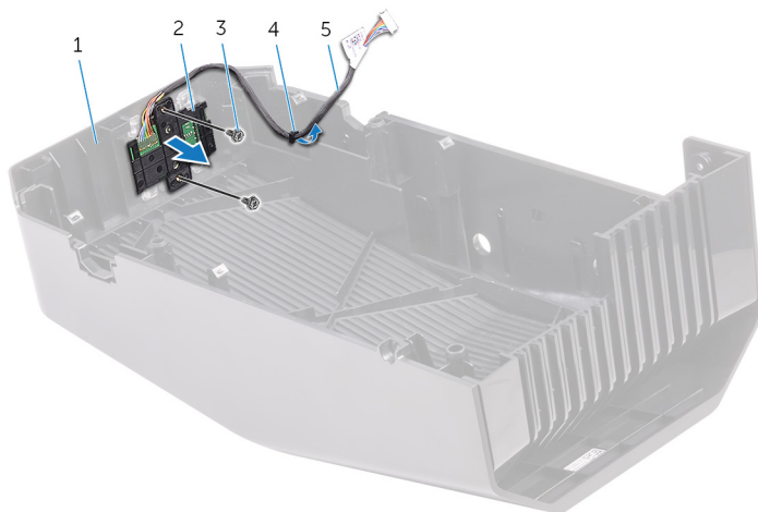
Figure 47. Retrait du module du bouton d'alimentation
