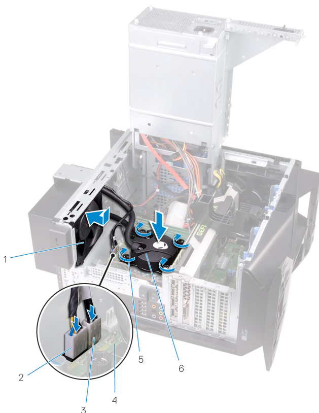
Figure 22. Remise en place du bloc de refroidissement du processeur
