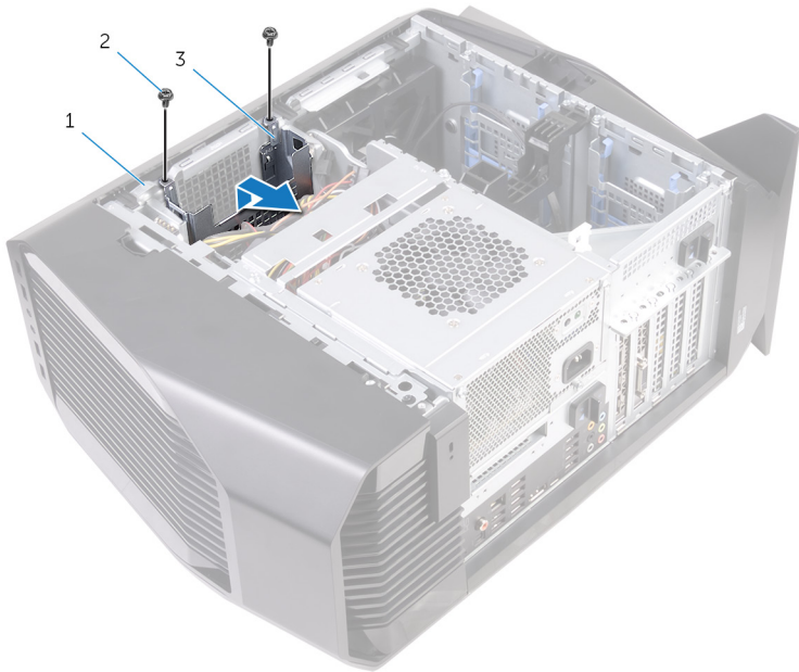
Figure 17. Retrait du bâti du disque dur
