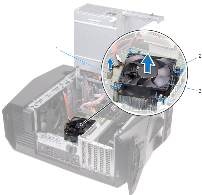
Figure 30. Retrait du bloc ventilateur-dissipateur de chaleur du système
