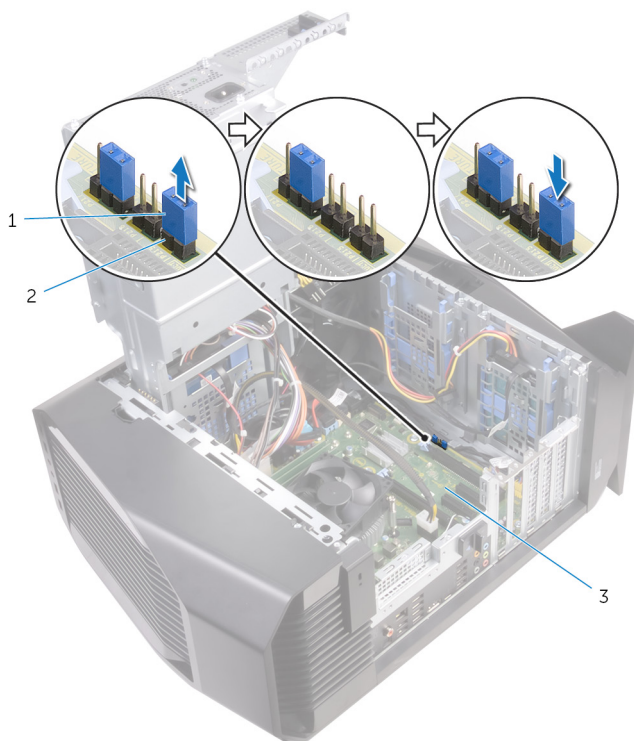
Figure 52. Effacement des mots de passe oubliés
