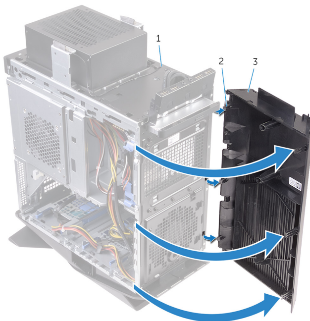
Figure 46. Retrait du cadre avant
