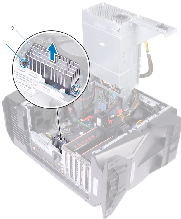
Figure 29. Retrait du dissipateur de chaleur du régulateur de tension
