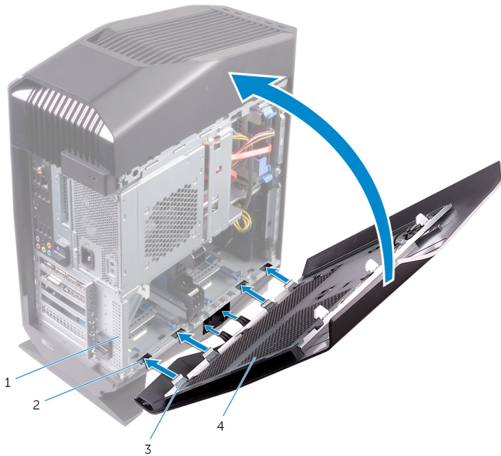
Figure 3. Remise en place du panneau latéral gauche
