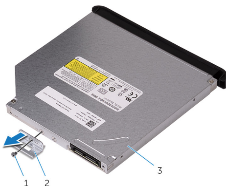
Figure 43. Retrait du lecteur optique
