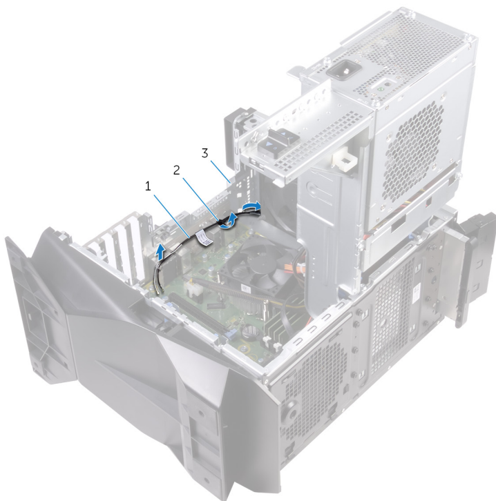
Figure 35. Retrait des câbles d'antenne
