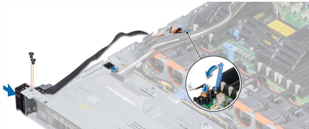
Figura 114. Instalación del panel de control izquierdo
