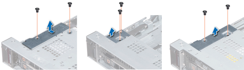
Figura 112. Extracción de la cubierta de cables
