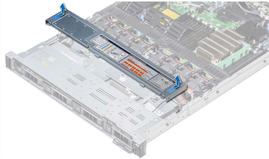
Figura 24. Extracción de la cubierta del plano posterior
