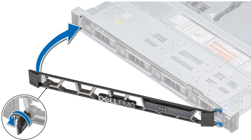
Figura 21. Instalación del bisel frontal opcional con panel LCD
