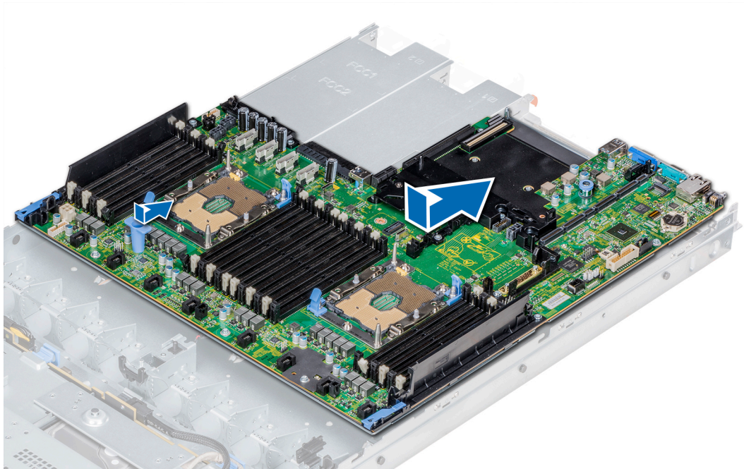
Figura 110. Instalación de la placa base
