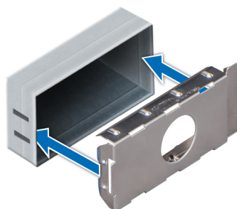
Figura 106. Instalación de una unidad de fuente de alimentación de relleno
