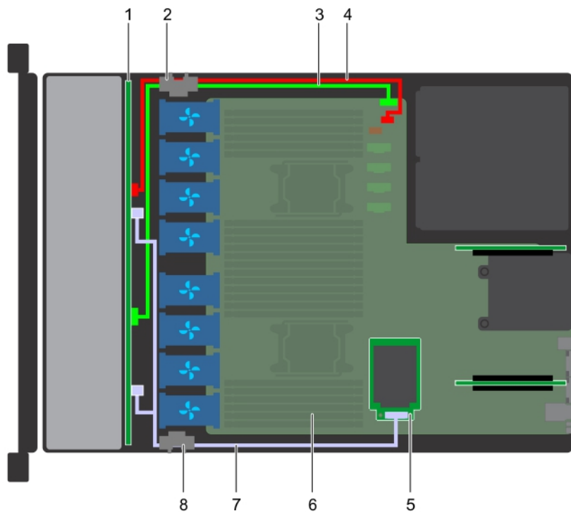
Figura 91. Colocación de los cables: backplane de unidad de 8 x 2.5 pulgadas con miniPERC
