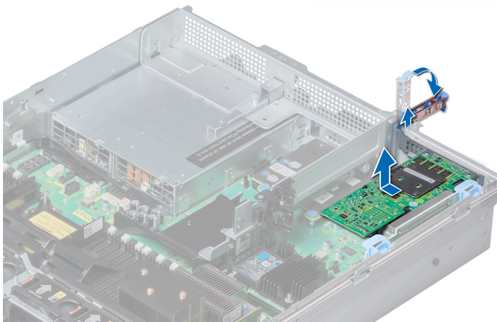
Figura 54. Extracción de una tarjeta de expansión del soporte vertical para tarjetas de expansión 1
