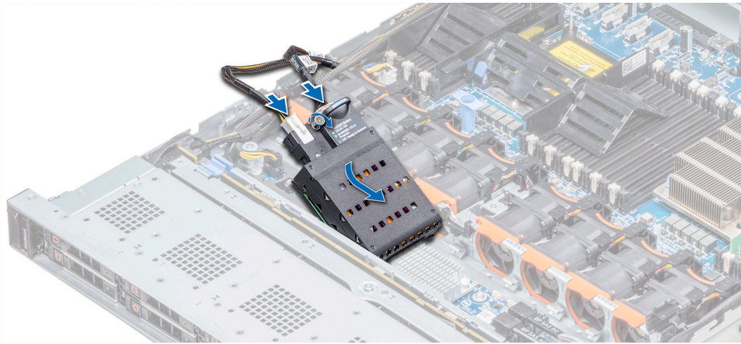
Figura 37. Instalación de la batería NVDIMM-N
