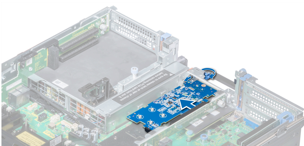
Figura 55. Extracción de la tarjeta de expansión del soporte vertical para tarjetas de expansión 2B
