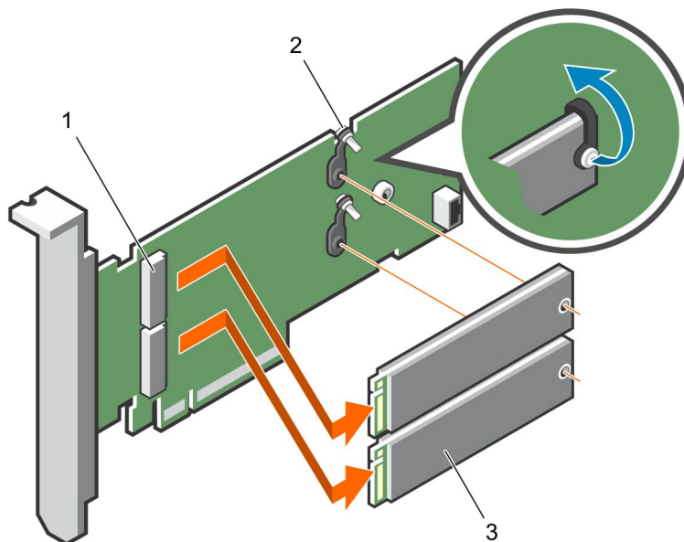
Figura 63. Extracción del módulo M.2 SSD
