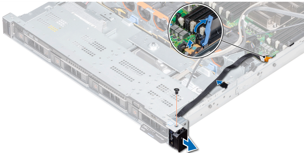
Figura 117. Desmontaje del panel de control derecho
