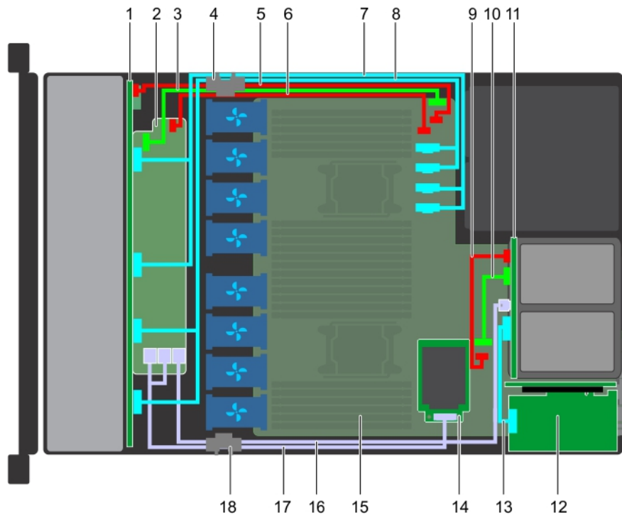
Figura 87. Colocación de cables: backplane de unidad de 10 x 2.5 pulgadas y backplane de unidad posterior de 2 x 2.5 pulgadas con miniPERC
