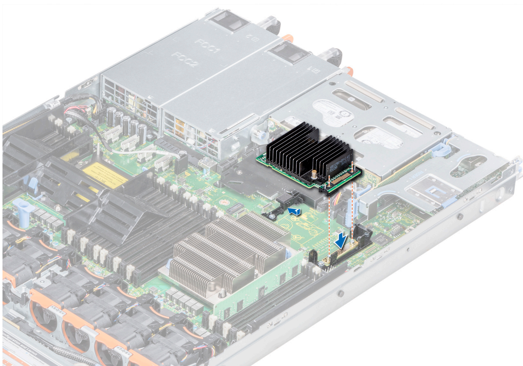
Figura 71. Instalación de la tarjeta controladora de almacenamiento integrada
