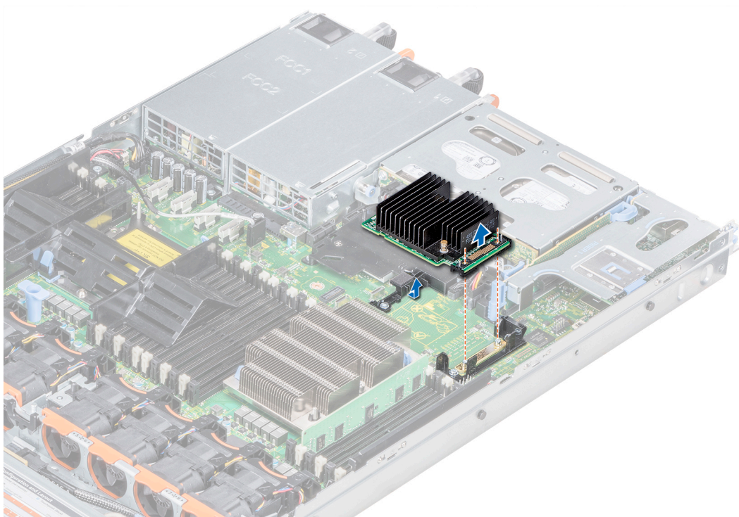
Figura 70. Extracción de la tarjeta controladora de almacenamiento integrada
