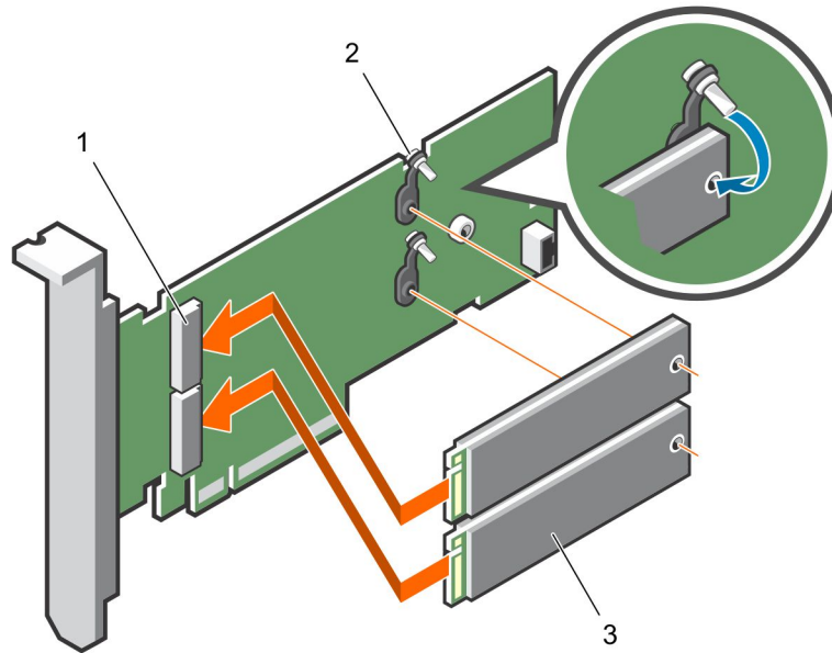
Figura 64. Instalación del módulo M.2 SSD
