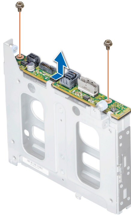
Figura 84. Extracción del plano posterior interno de la unidad de disco de 2.5 pulgadas
