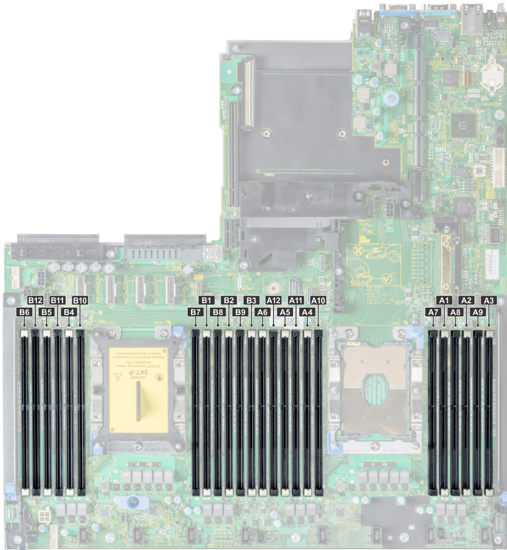
Figura 33. Vista de memoria del sistema
