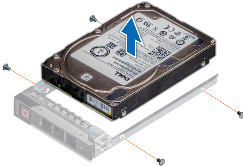
Figura 77. Extracción de la unidad del portaunidades
