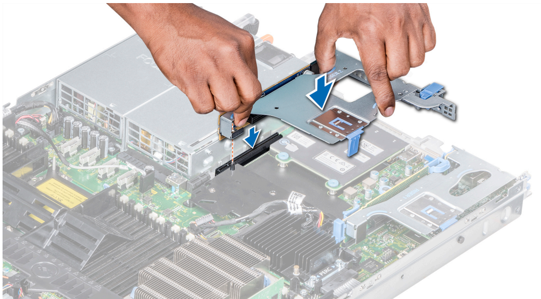
Figura 53. Instalación del soporte vertical de expansión 2B
