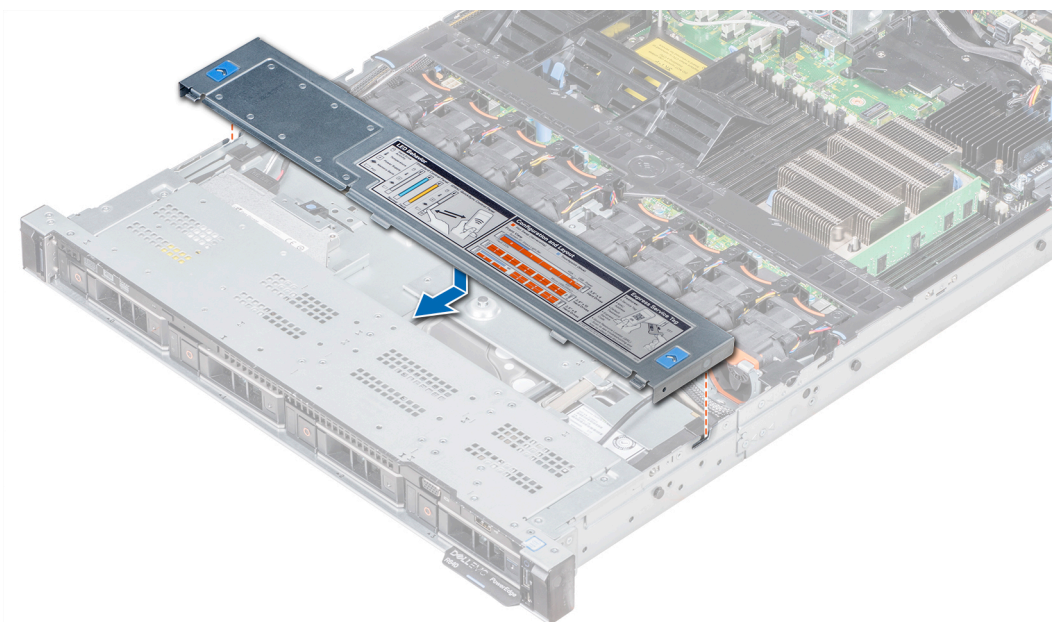
Figura 25. Instalación de la cubierta del plano posterior
