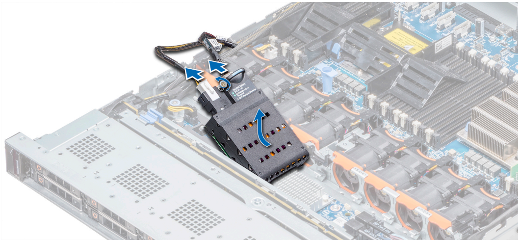
Figura 36. Extracción de la batería NVDIMM-N
