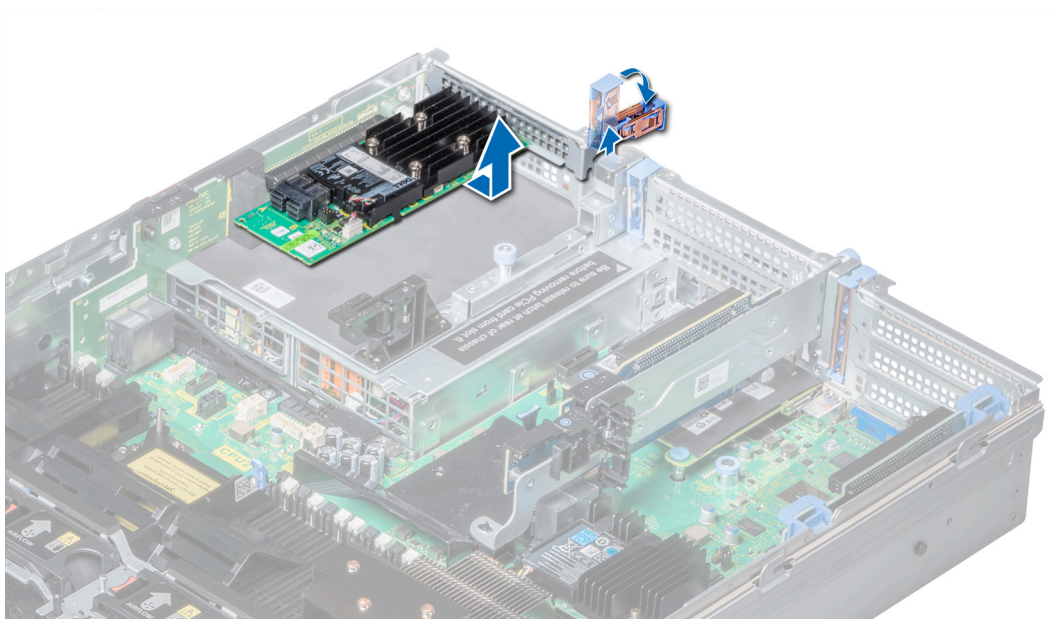
Figura 57. Extracción de una tarjeta de expansión del soporte vertical para tarjetas de expansión 3
