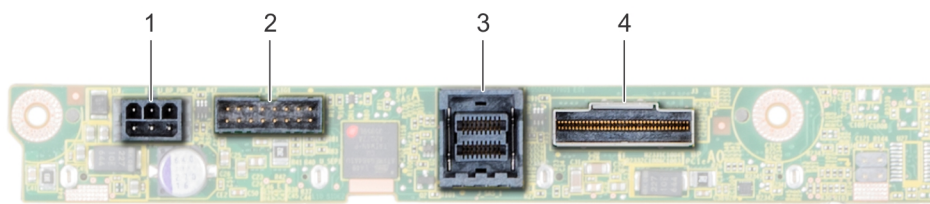
Figura 84. Extracción del plano posterior interno de la unidad de disco de 2.5 pulgadas
