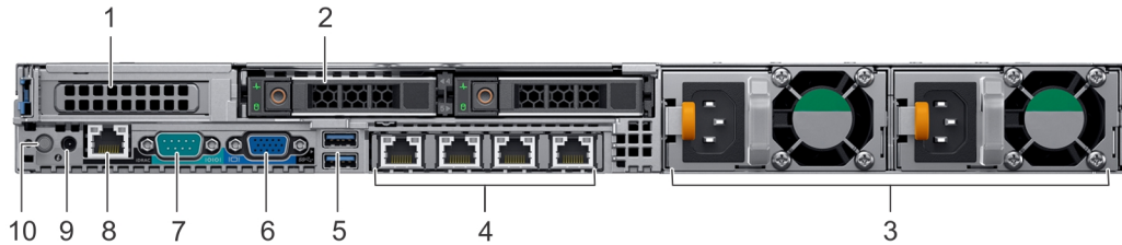
Figura 7. Vista posterior de las unidades de 2 x 2.5 pulgadas con 1 ranura de expansión PCIe
