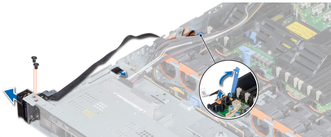
Figura 113. Extracción del panel de control izquierdo
