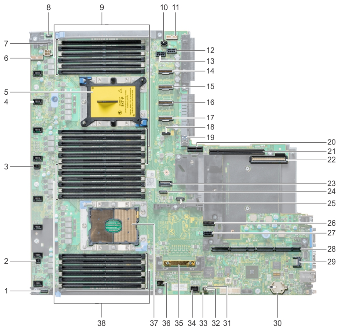
Figura 120. Puentes y conectores de la placa base
