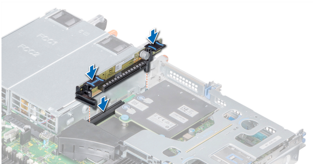
Figura 52. Instalación del soporte vertical de expansión 2A
