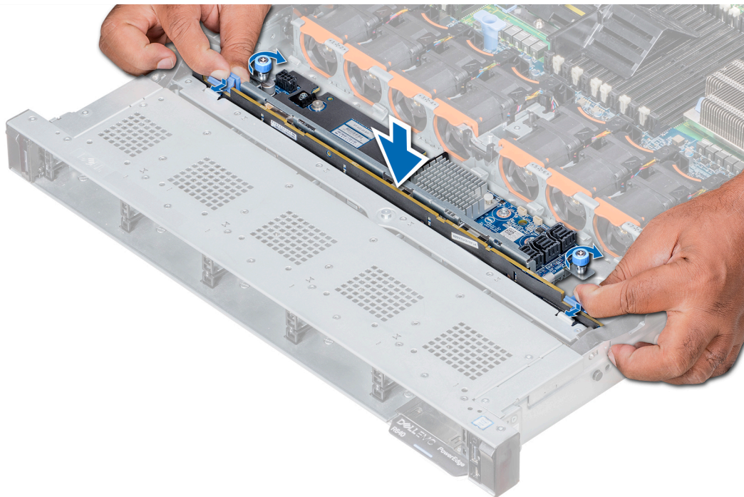
Figura 83. Instalación del plano posterior
