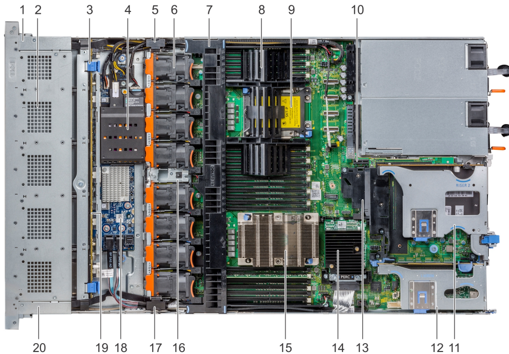
Figura 27. Interior del sistema: 2 soportes verticales para tarjetas de expansión PCIe
