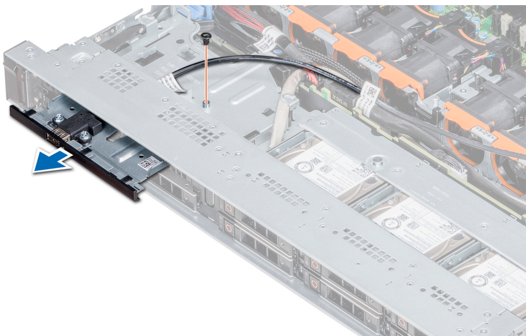
Figura 99. Extracción del módulo USB
