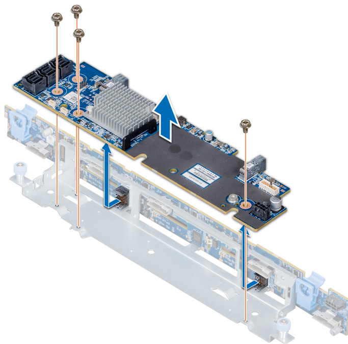
Figura 93. Extracción de la tarjeta expansora SAS
