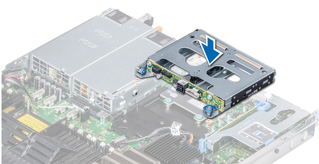
Figura 96. Instalación de la caja para unidades de disco internas
