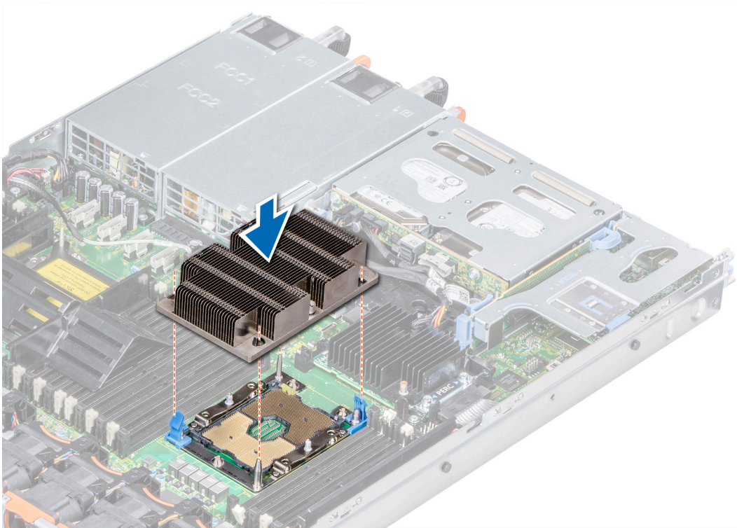
Figura 45. Instalación de un procesador y módulo del disipador de calor
