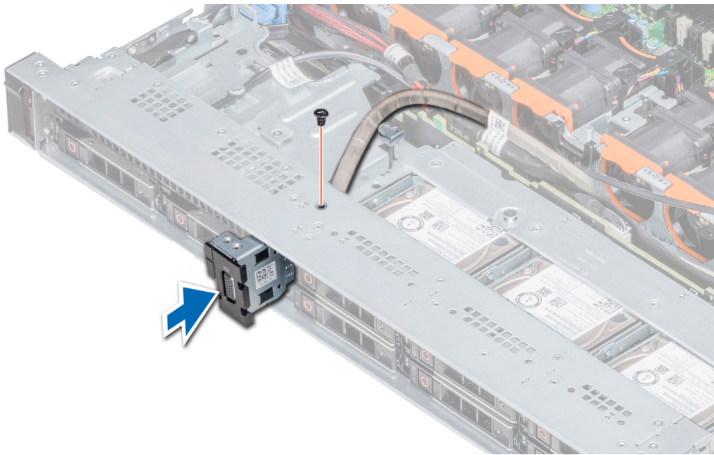
Figura 102. Instalación del módulo VGA
