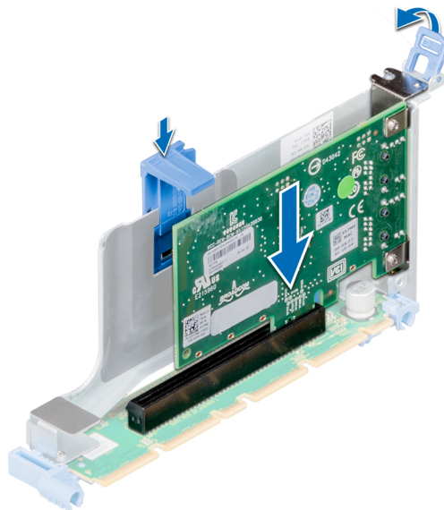
Figura 60. Instalación de una tarjeta de expansión en el soporte vertical para tarjetas de expansión 1B
