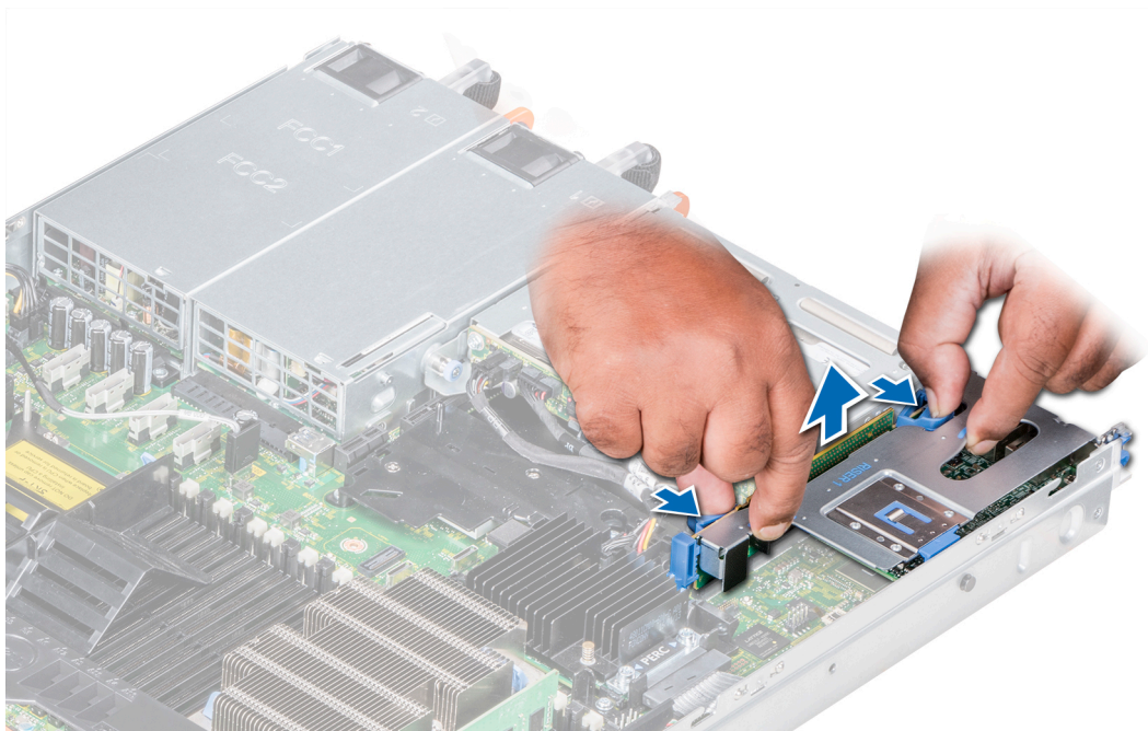
Figura 46. Extracción del soporte vertical para tarjetas de expansión 1B
