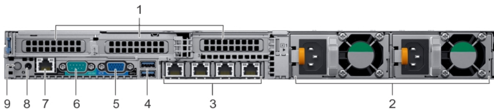
Figura 8. Vista posterior del sistema con 3 ranuras de expansión PCIe
