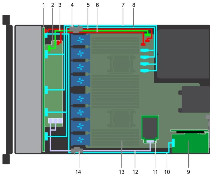
Figura 89. Colocación de los cables: backplane de unidad de 10 x 2.5 pulgadas con NVMe
