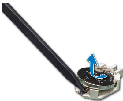
Figura 97. Extracción de la batería del sistema
