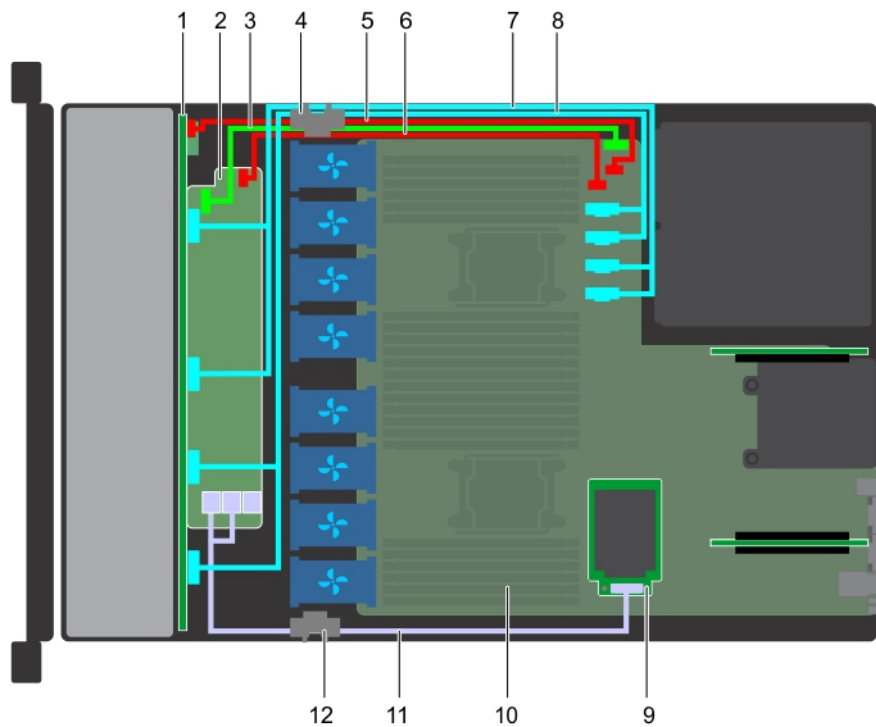
Figura 88. Colocación de los cables: backplane de unidad de 10 x 2.5 pulgadas con miniPERC
