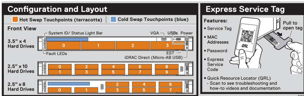
Figura 16. Etiqueta de servicio expreso, configuración y diseño
