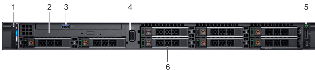
Figura 2. Vista frontal del sistema de la unidad de disco de 8 x 2.5 pulgadas
