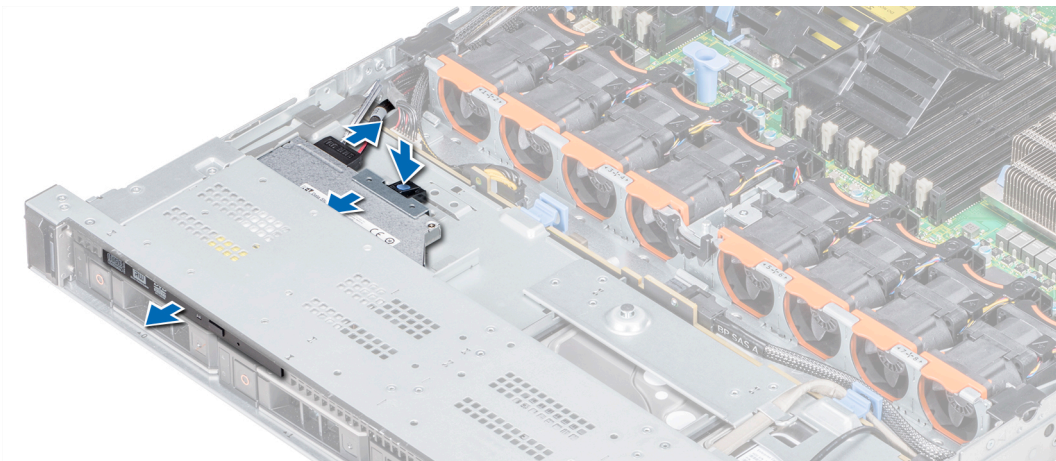
Figura 103. Extracción de la unidad óptica
