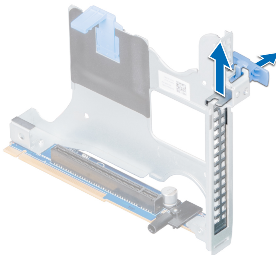
Figura 58. Extracción del soporte de relleno metálico del soporte vertical para tarjetas 2B
