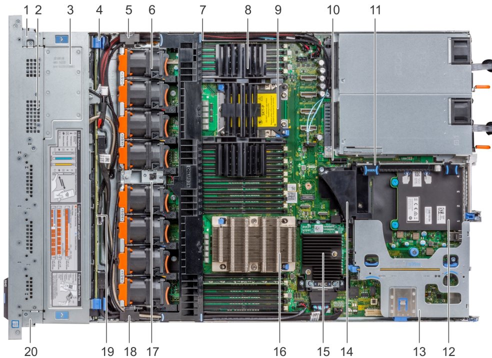
Figura 28. Interior del sistema: 3 soportes verticales para tarjetas de expansión PCIe
