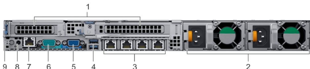
Figura 9. Vista posterior del sistema con 2 ranuras de expansión PCIe
