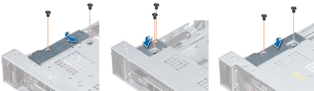
Figura 115. Instalación de la cubierta de cables
