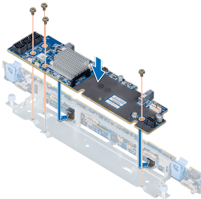
Figura 94. Instalación de la tarjeta expansora SAS
