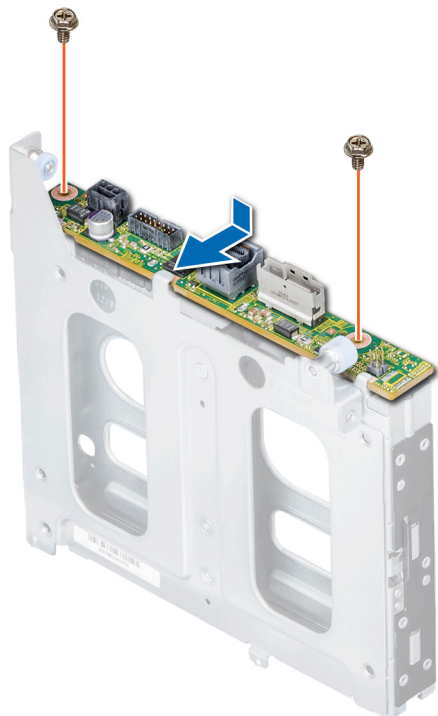
Figura 86. Instalación del backplane trasero de la unidad de 2,5 pulgadas
