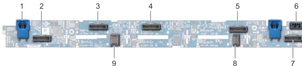
Figura 81. Backplane de la unidad de 10 x 2,5
