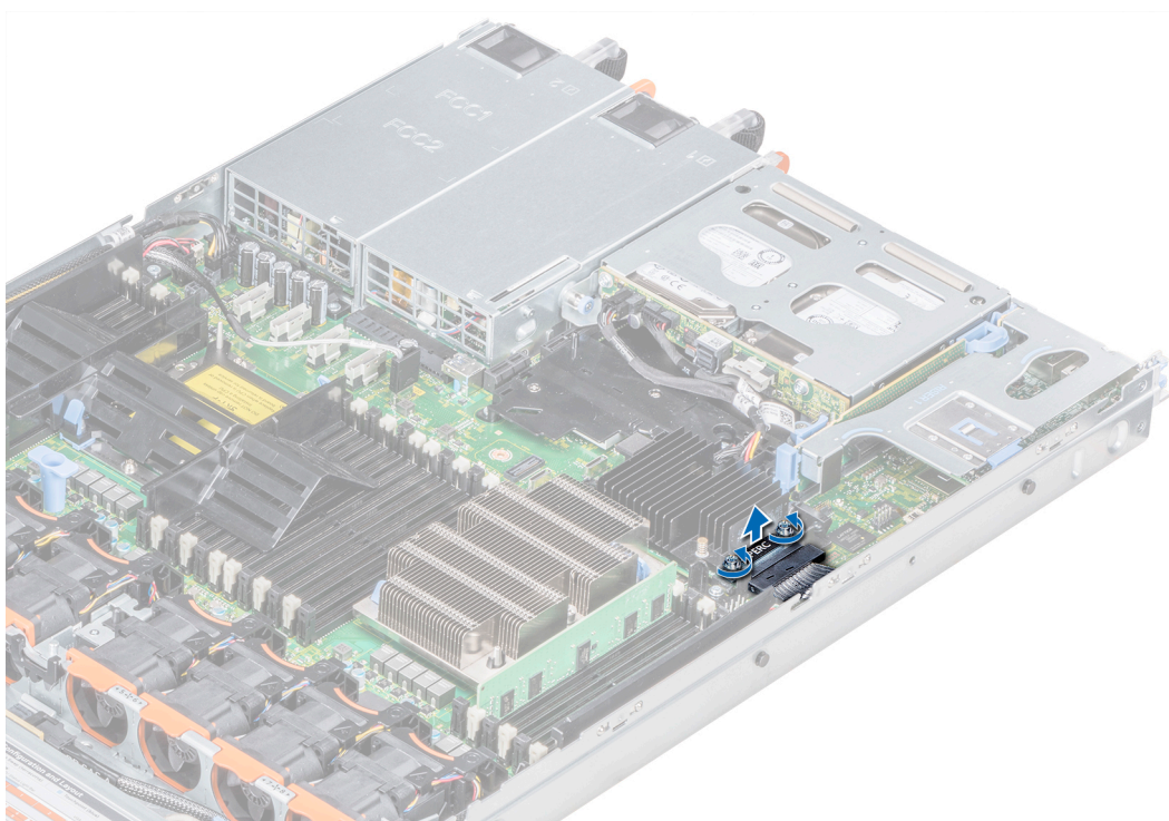
Figura 69. Extracción del cable de la controladora de almacenamiento integrada
