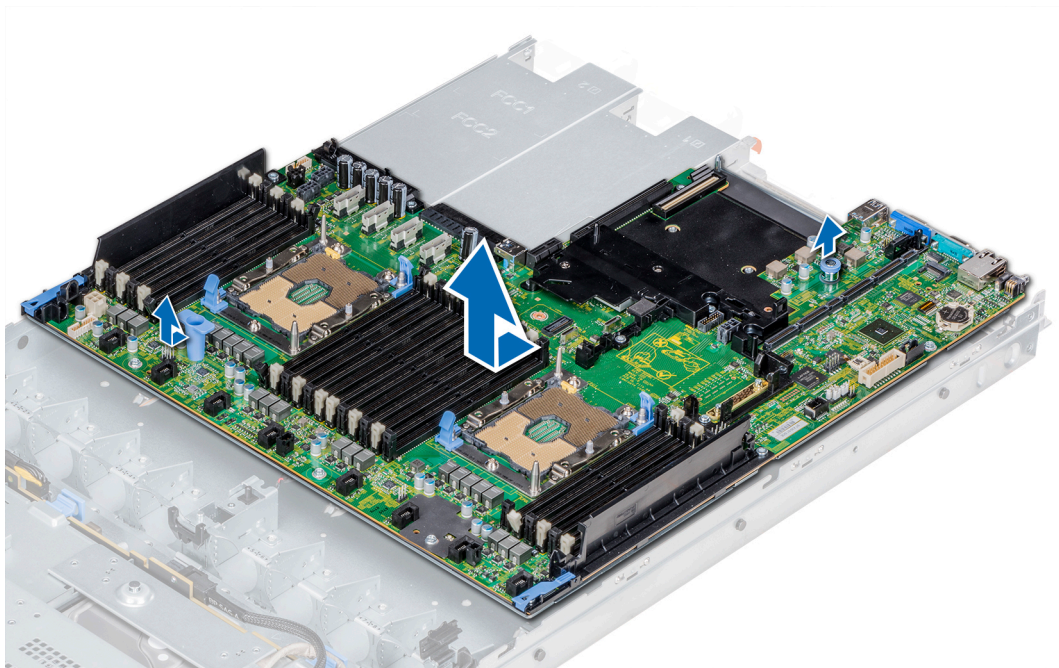
Figura 109. Extracción de la placa base
