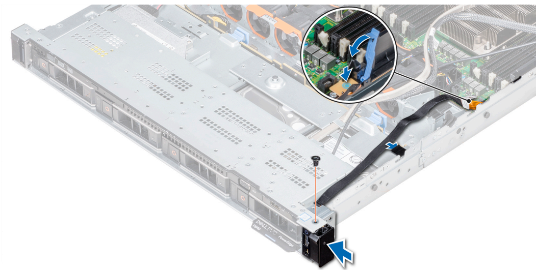
Figura 118. Instalación del panel de control derecho
