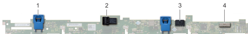
Figure 79. Backplane de 4 disques de 3,5 pouces
