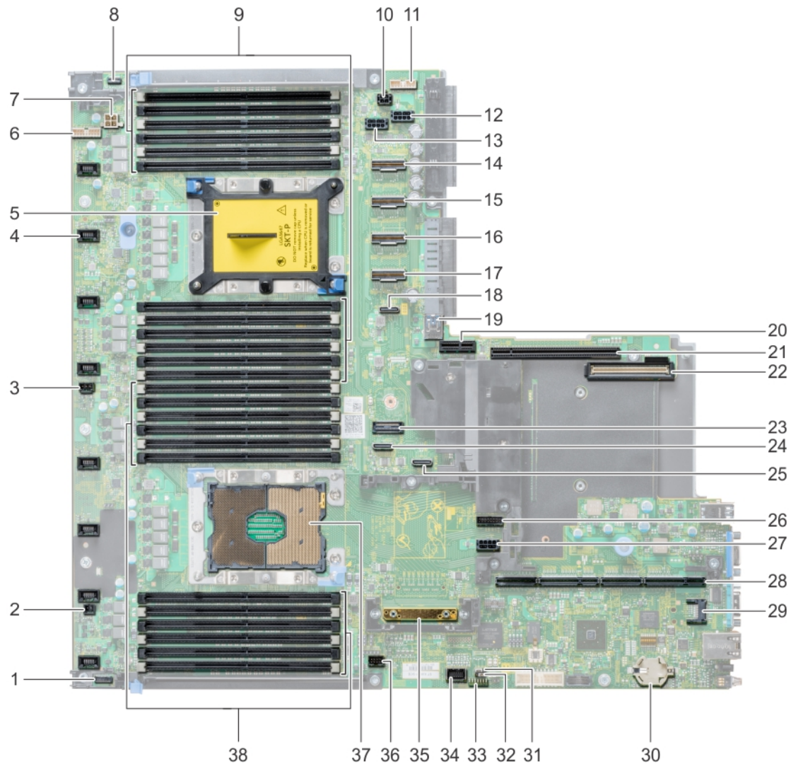
Figure 120. Connecteurs et cavaliers de la carte système
