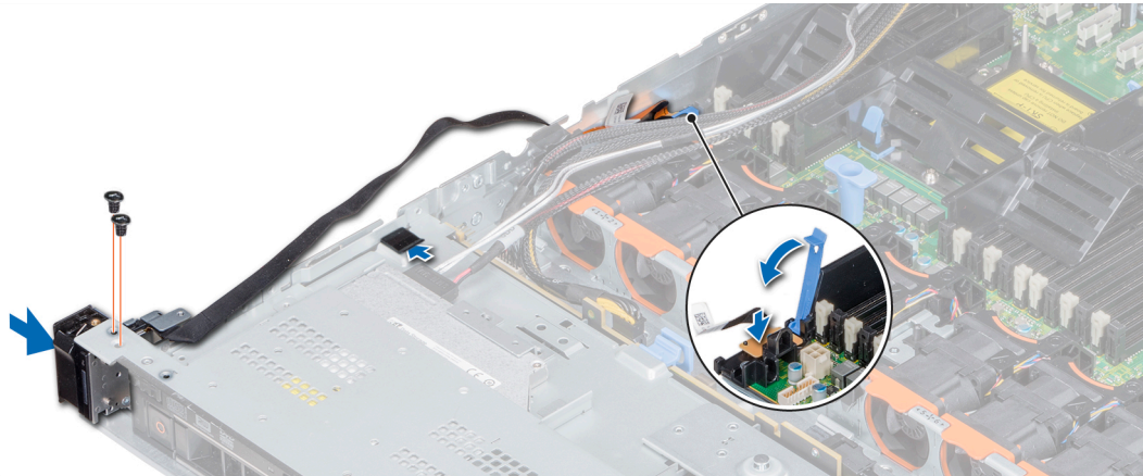
Figure 114. Installation du panneau de commande gauche
