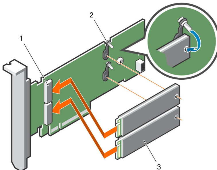
Figure 64. Installation du module SSD M.2
