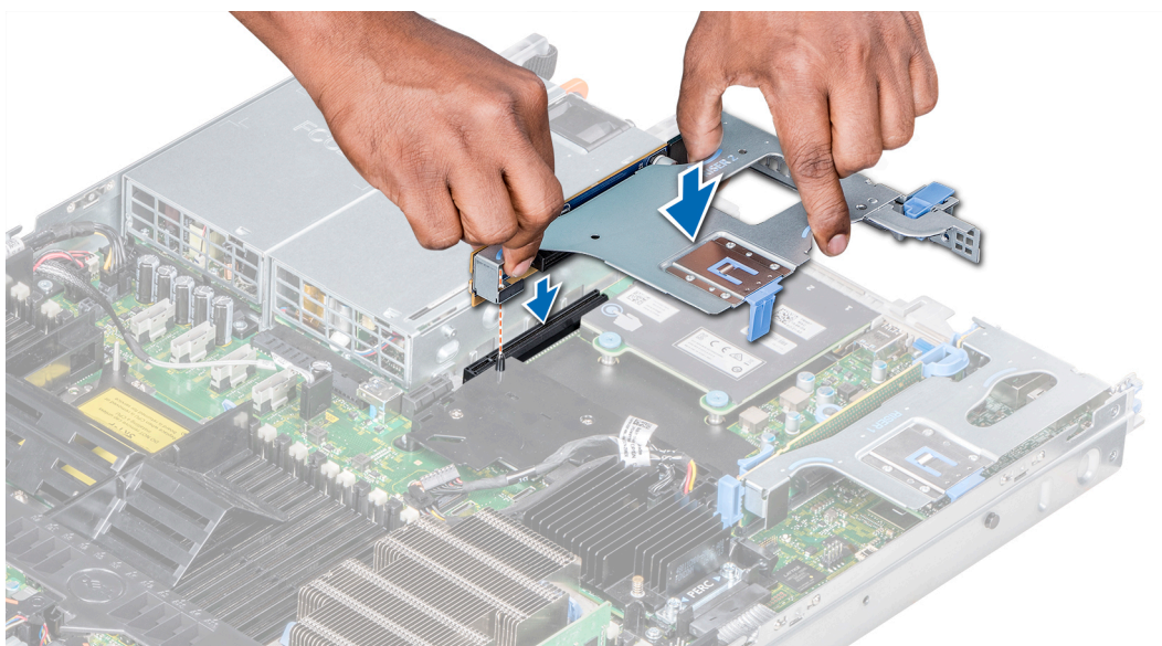
Figure 53. Installation de la carte de montage d'extension 2B
