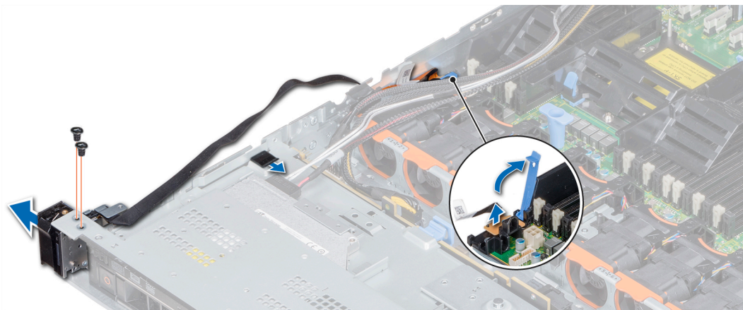
Figure 113. Retrait du panneau de commande de gauche
