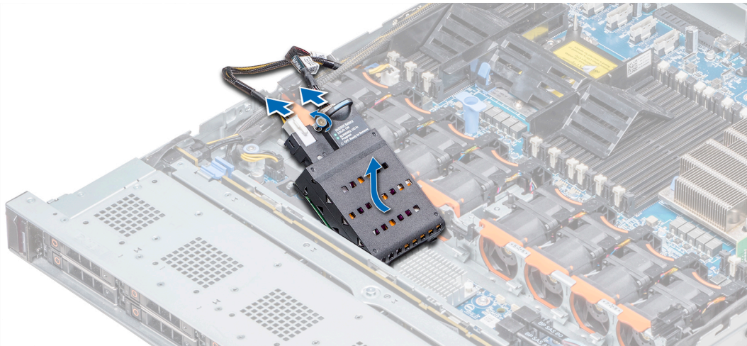
Figure 36. Retrait de la pile du module NVDIMM-N
