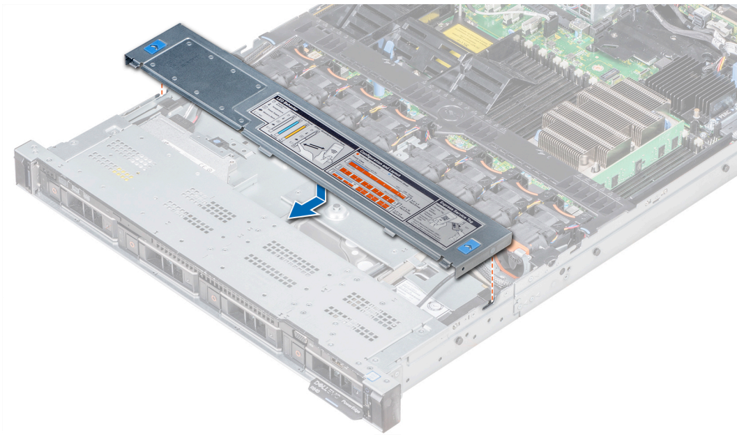
Figure 25. Installation du cache de fond de panier
