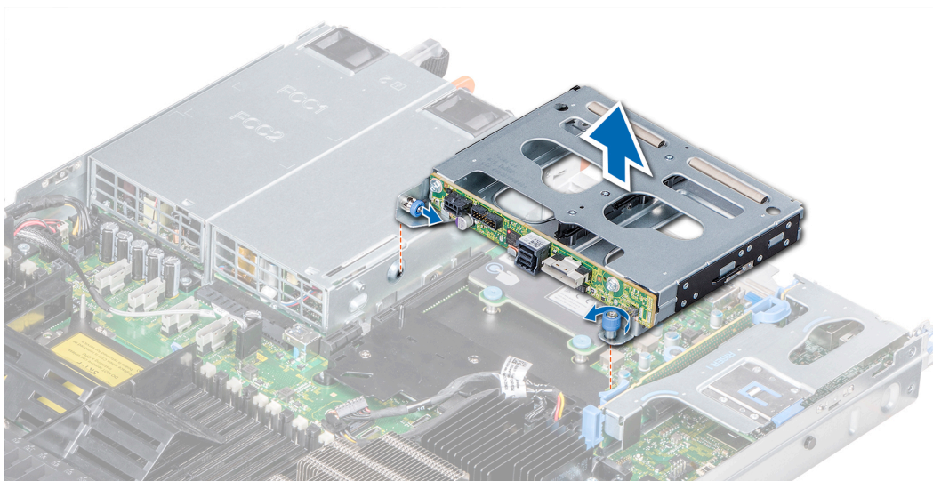
Figure 95. Retrait du bâti de disque arrière
