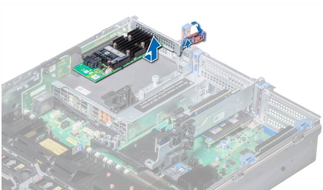
Figure 57. Retrait de la carte d'extension hors de la carte de montage pour cartes d'extension 3
