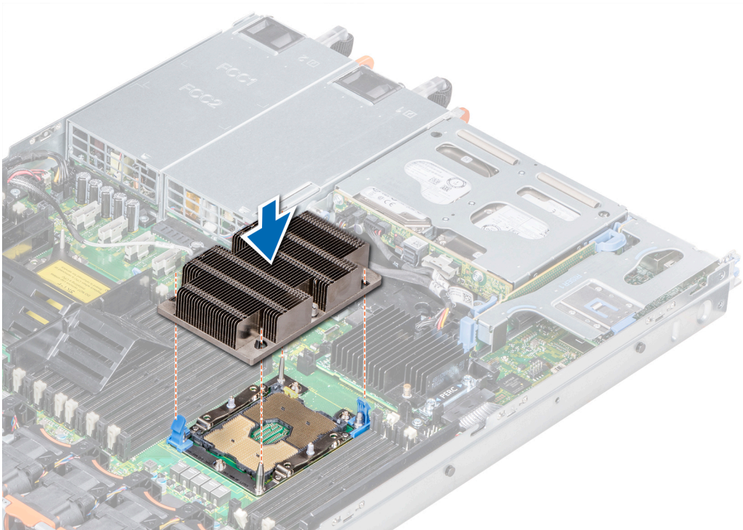
Figure 45. Installation du module processeur et dissipateur de chaleur
