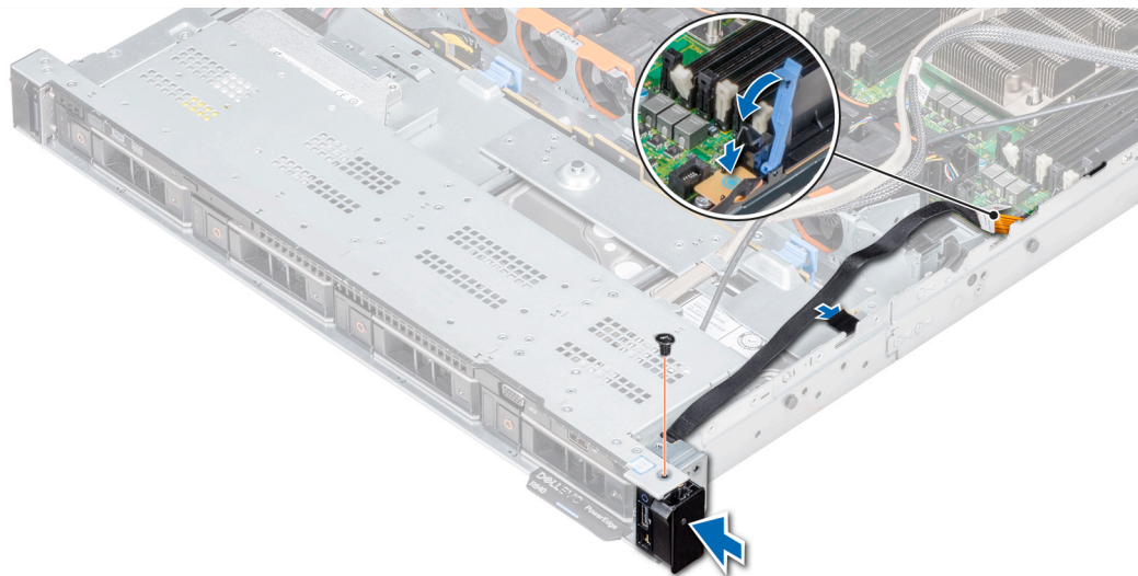
Figure 118. Installation du panneau de commande droit
