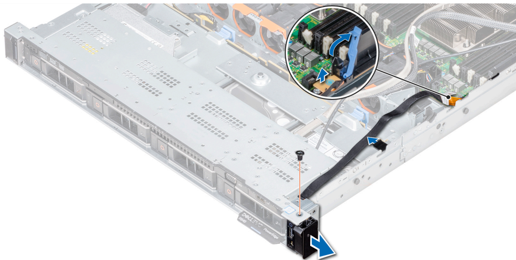
Figure 117. Retrait du panneau de commande droit
