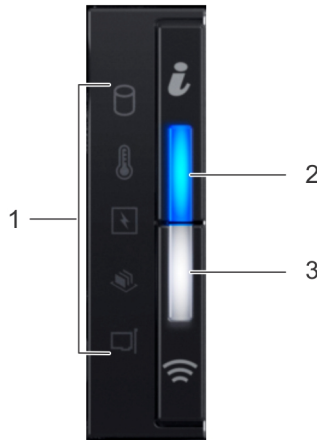
Figure 5. Panneau de commande de gauche avec voyant iDRAC Quick Sync 2.0 en option
