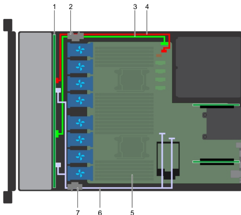
Figure 92. Acheminement des câbles : backplane de 8 disques de 2,5 pouces avec disque SATA intégré
