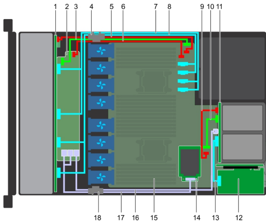
Figure 87. Acheminement des câbles : backplane doté de 10 disques de 2,5 pouces et backplane arrière doté de 2 disques de 2,5 pouces avec carte mini PERC
