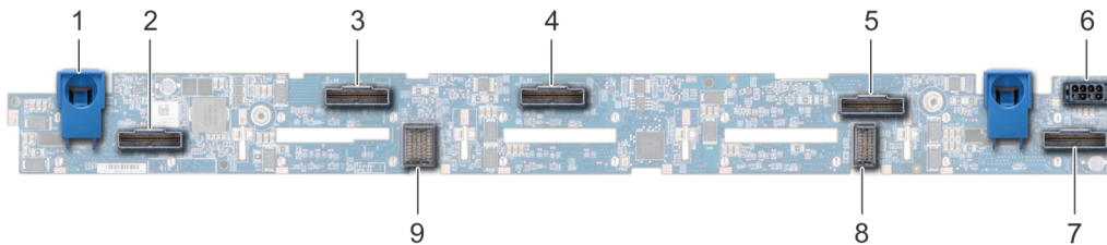
Figure 81. Backplane de 10 disques de 2,5 pouces
