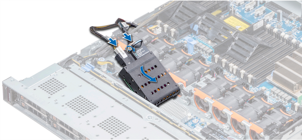
Figure 37. Installation de la batterie NVDIMM-N
