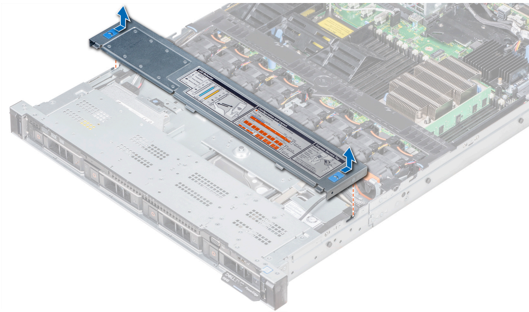
Figure 24. Retrait du cache de fond de panier
