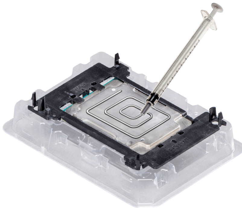
Figure 43. Application de graisse thermique sur la partie supérieure du processeur
