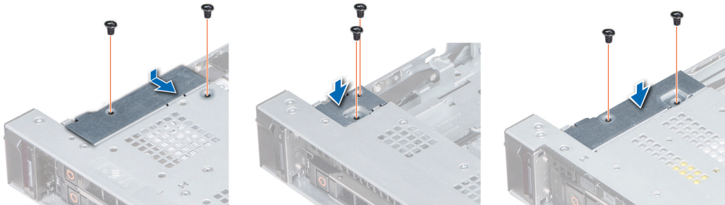
Figure 115. Installation du cache-câbles
