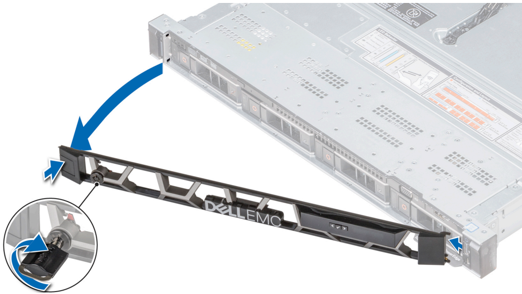
Figure 20. Retrait du cadre avant optionnel avec l'écran LCD
