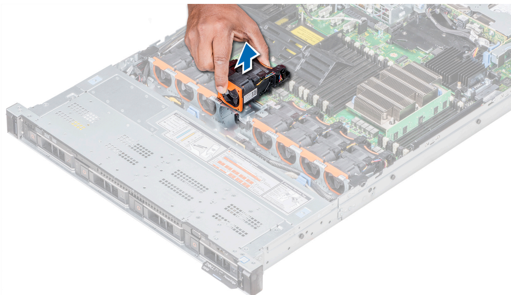
Figure 31. Retrait du ventilateur de refroidissement
