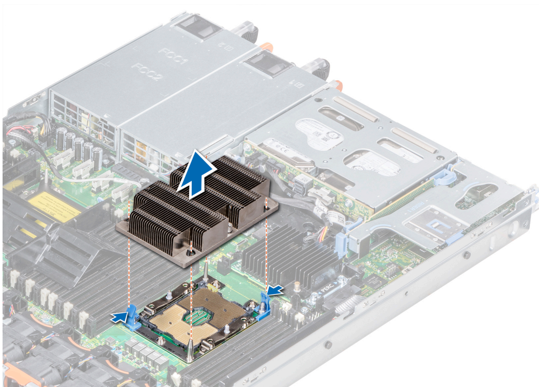
Figure 39. Retrait du module du processeur et du dissipateur de chaleur
