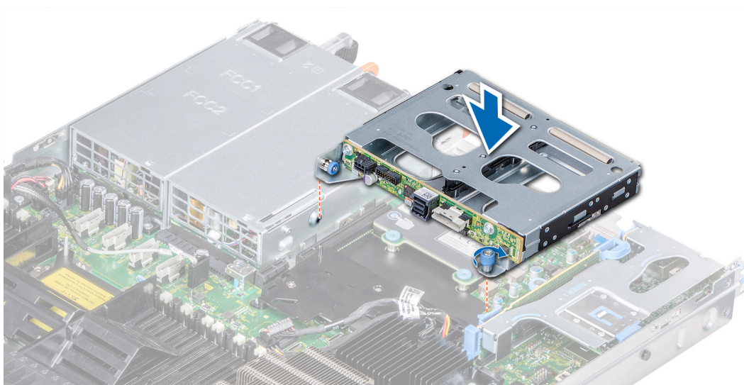
Figure 96. Installation du bâti des disques arrière
