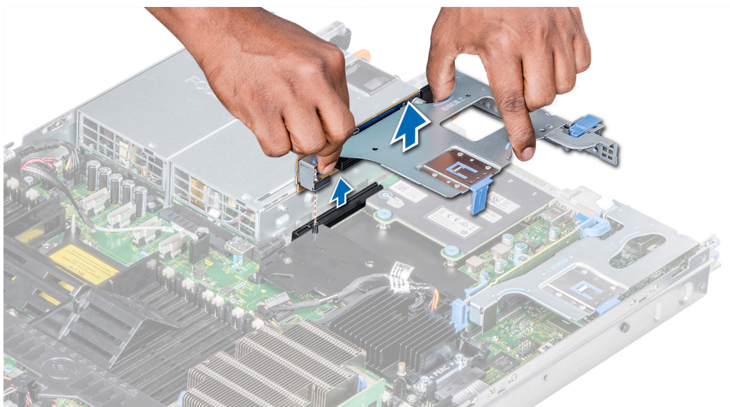
Figure 49. Retrait de la carte de montage d'extension 2B
