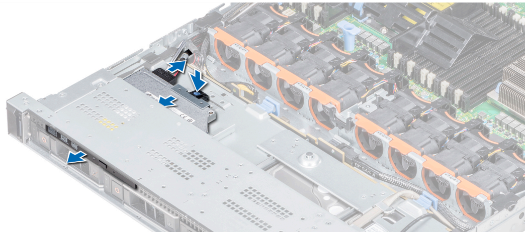
Figure 103. Retrait du lecteur optique
