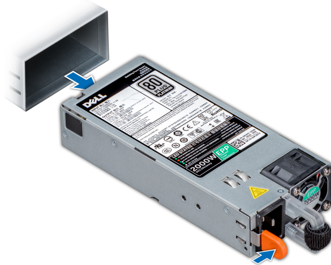
Figure 107. Retrait d'une unité d'alimentation
