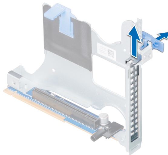
Figure 58. Retrait de la plaque de recouvrement métallique sur la carte de montage 2B
