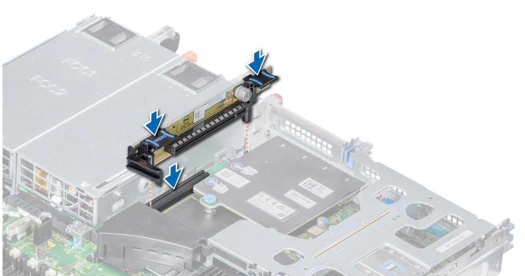
Figure 52. Installation de la carte de montage d'extension 2A
