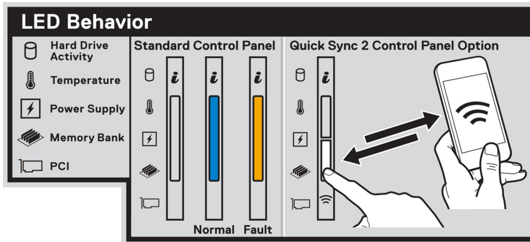
Figure 15. Comportement du voyant
