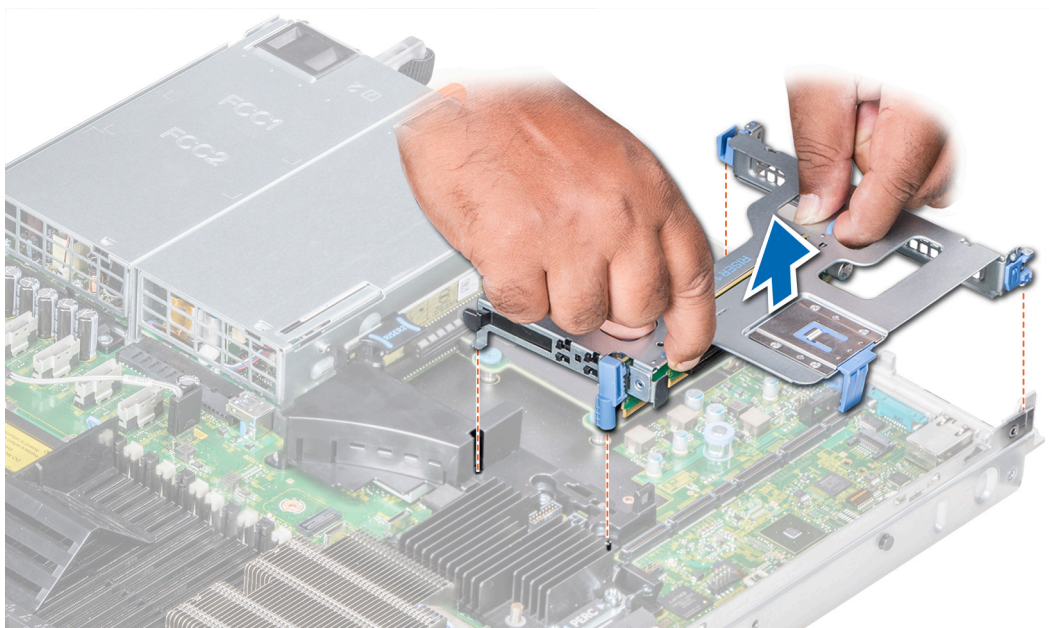
Figure 47. Retrait de la carte de montage d'extension 1A
