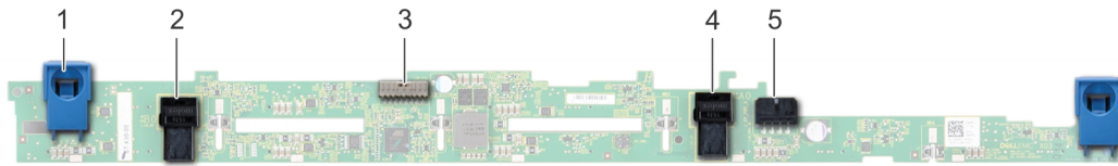
Figure 80. Backplane de 8 disques de 2,5 pouces
