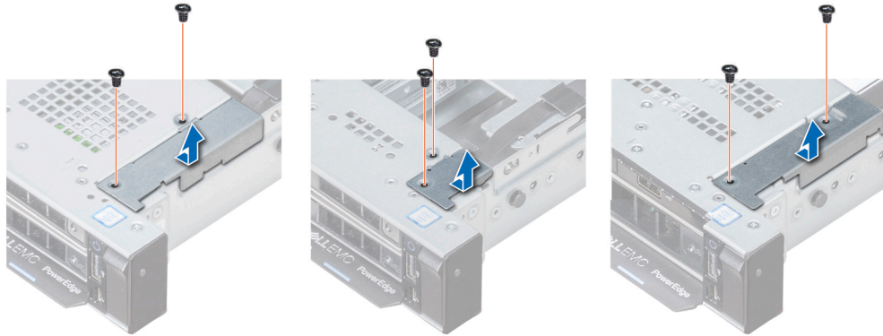
Figure 116. Retrait du cache-câbles
