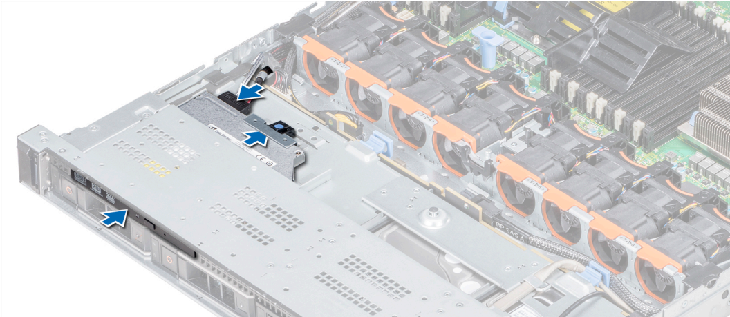
Figure 104. Installation du lecteur optique
