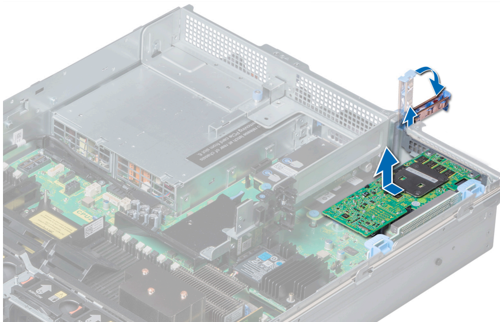
Figure 54. Retrait de la carte d'extension hors de la carte de montage pour cartes d'extension 1
