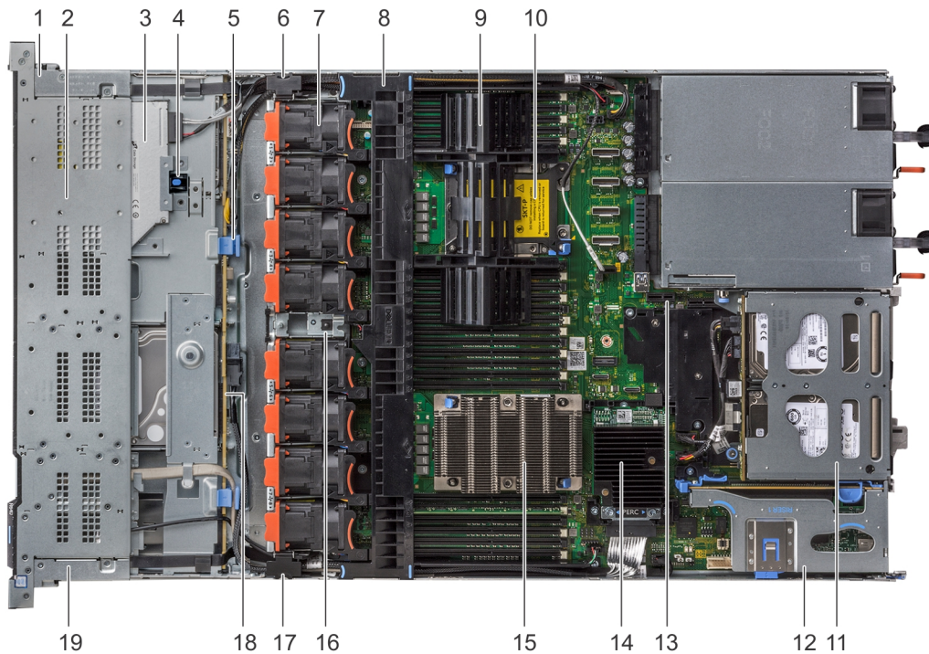
Figure 26. Intérieur du système : 1 carte de montage d'extension PCIe
