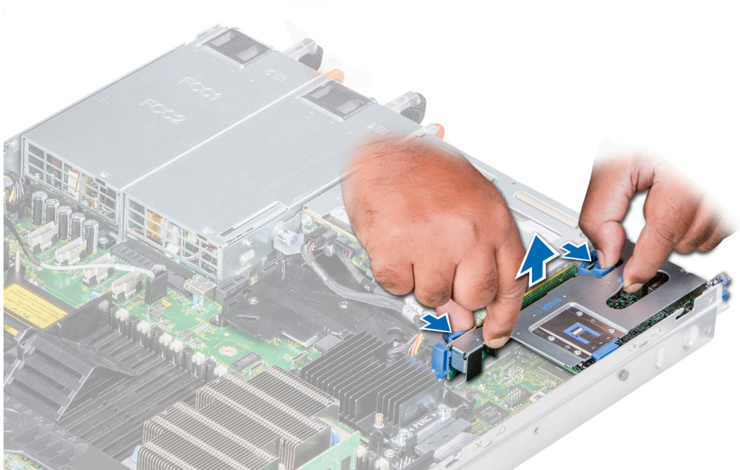
Figure 46. Retrait de la carte de montage d'extension 1B
