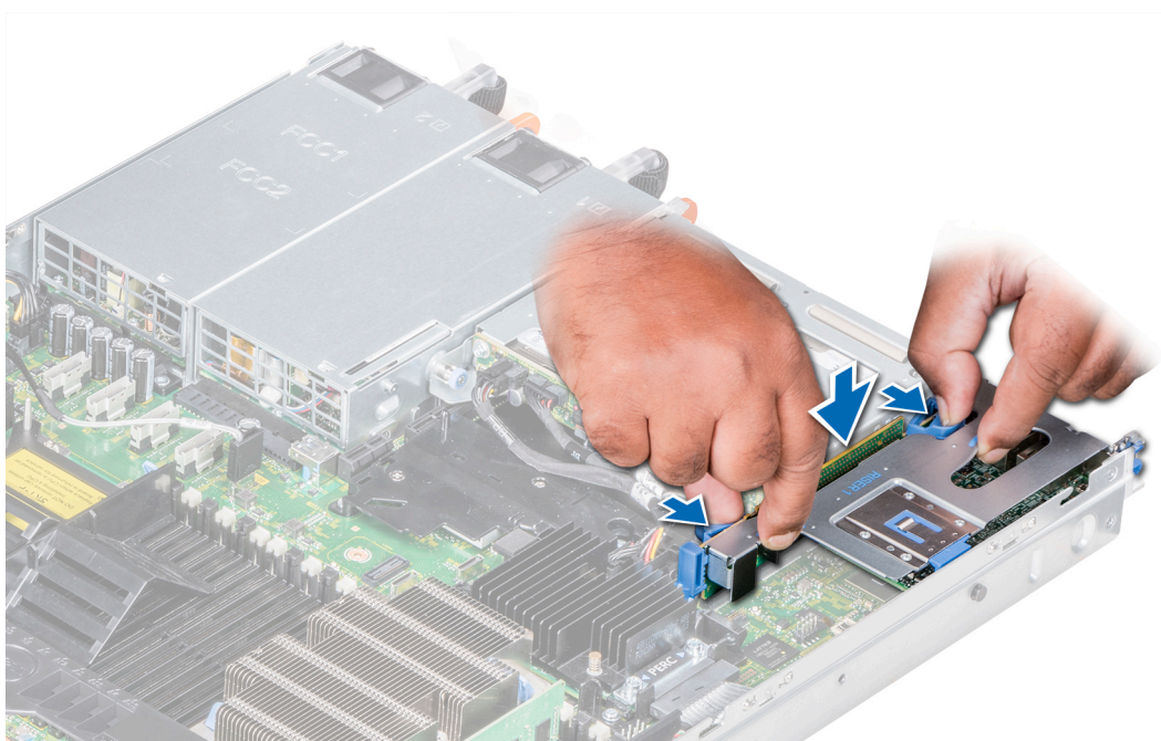
Figure 51. Installation de la carte de montage d'extension 1B
