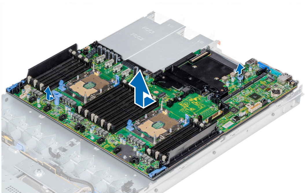
Figure 109. Retrait de la carte système
