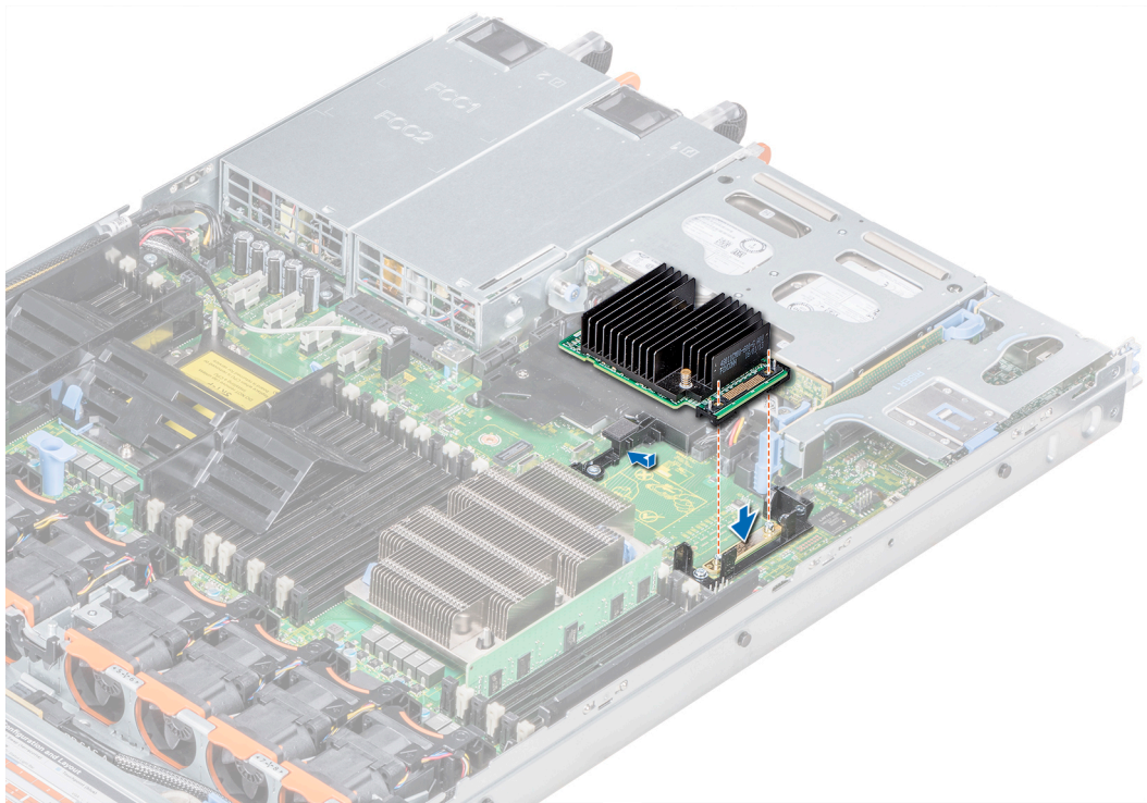
Figure 71. Installation de la carte contrôleur de stockage intégrée
