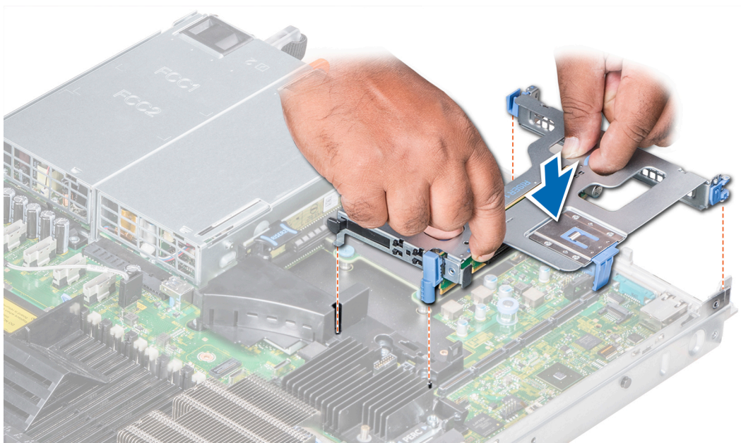
Figure 50. Installation de la carte de montage d'extension 1A
