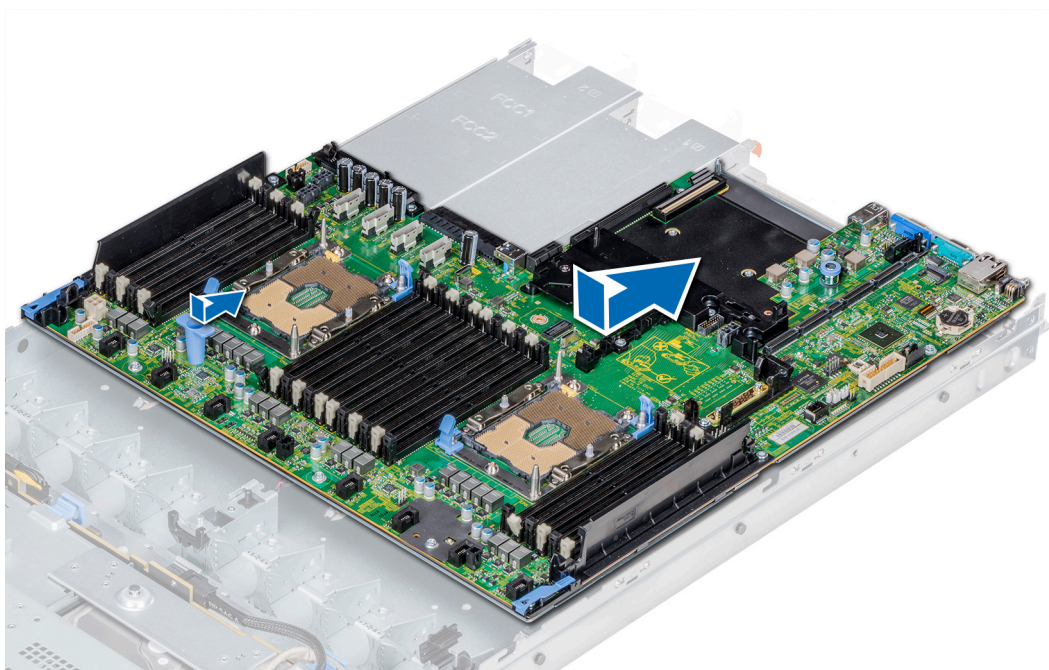
Figure 110. Installation de la carte système
