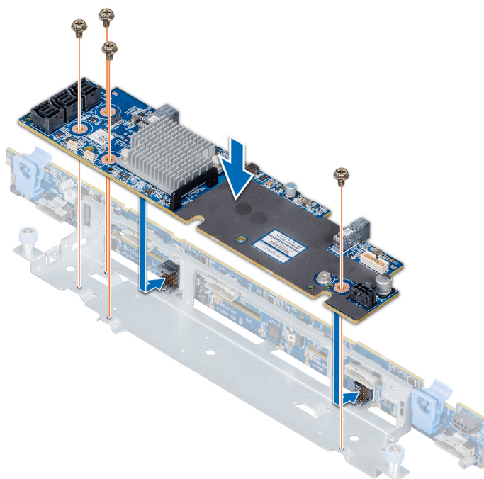
Figure 94. Installation de la carte du module d'extension SAS
