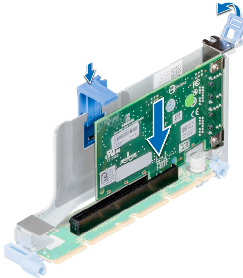
Figure 60. Installation d'une carte d'extension dans la carte de montage 1B
