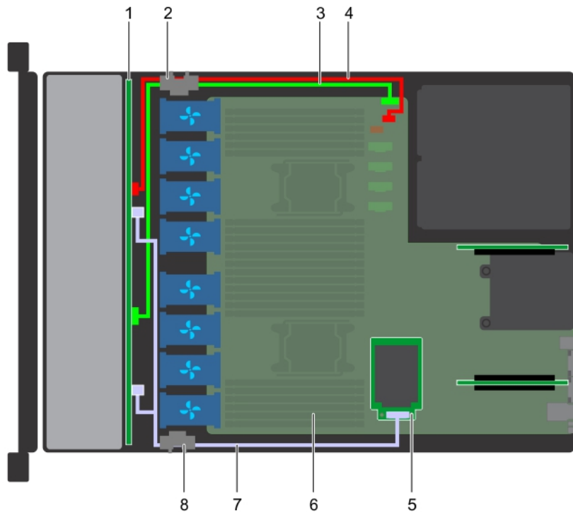
Figure 91. Acheminement des câbles : backplane de 8 disques de 2,5 pouces avec carte mini PERC
