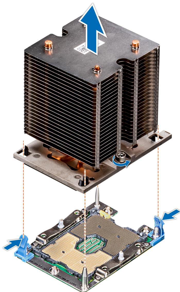
Figure 38. Retrait du module du processeur et du dissipateur de chaleur
