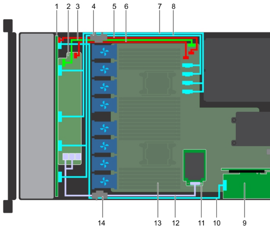
Figure 89. Acheminement des câbles : backplane de 10 disques de 2,5 pouces avec technologie NVMe
