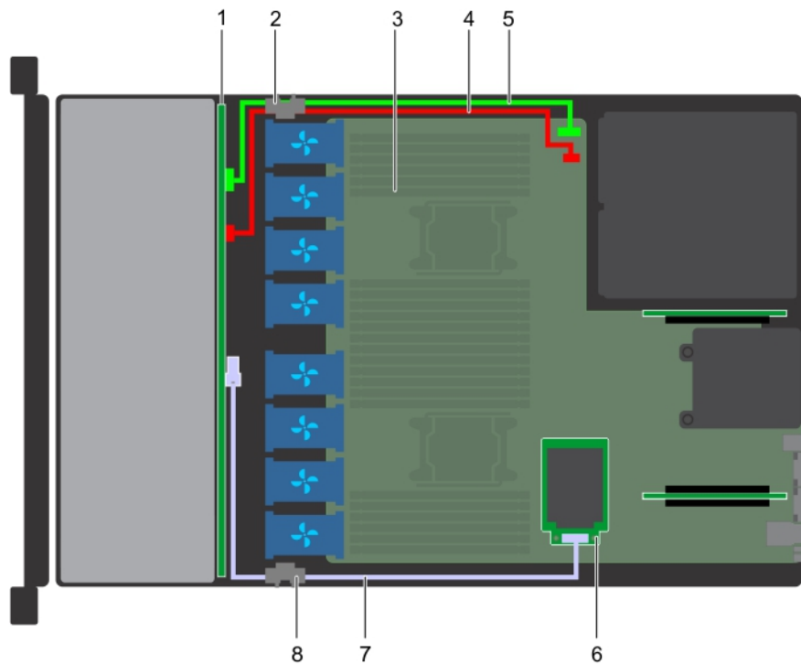
Figure 90. Acheminement des câbles : backplane de 4 disques de 3,5 pouces avec carte mini PERC
