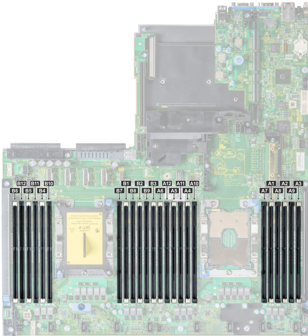
Figure 33. Vue du dessus du système
