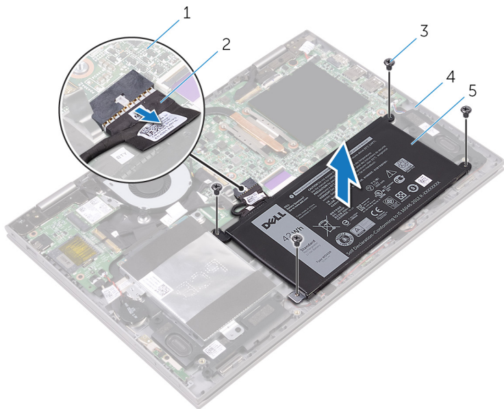
Figura 3. Batteria
