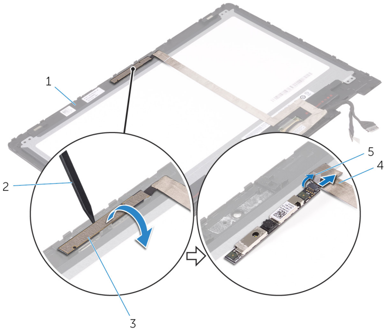
Figura 32. Fotocamera
