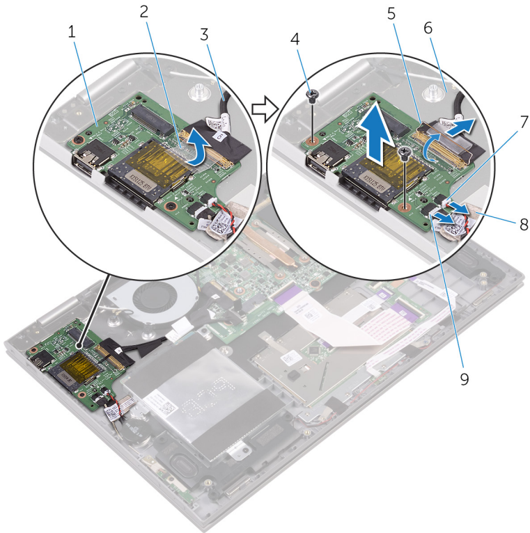
Figura 20. scheda I/O
