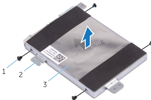
Figura 9. Disco rigido
