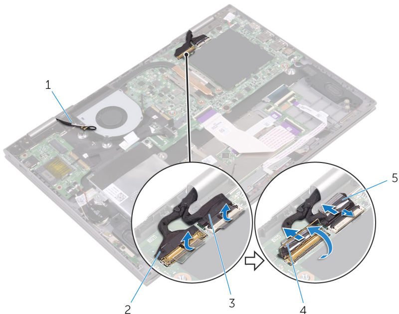
Figura 21. Gruppo schermo
