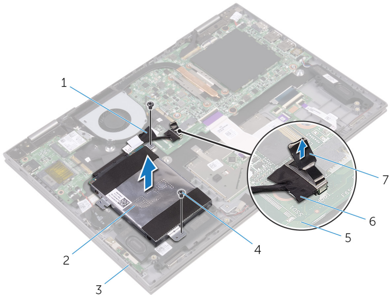
Figura 7. Disco rigido
