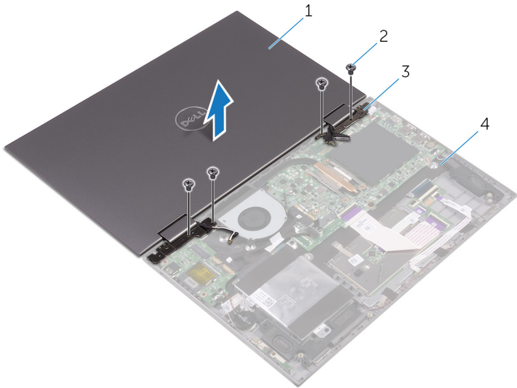
Figura 22. Gruppo schermo
