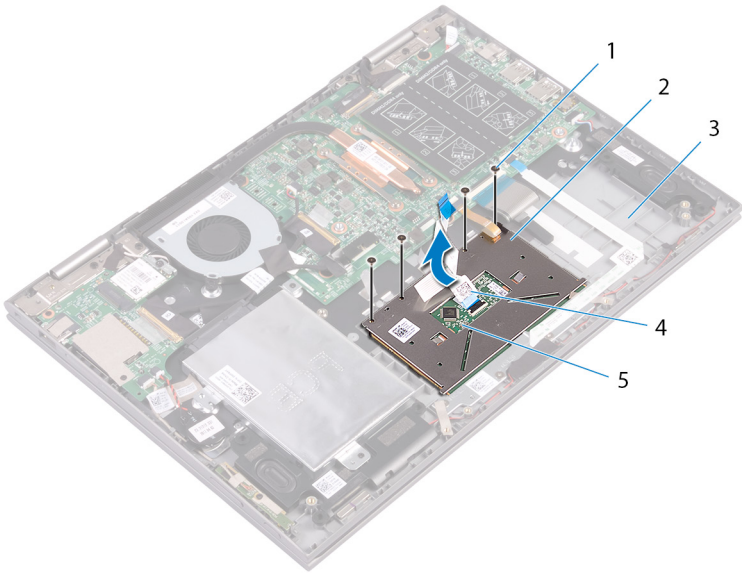
Figura 19. Touchpad
