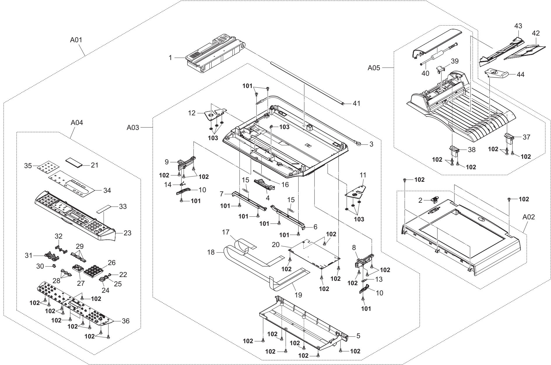
FIG. 9 MFP Unit
