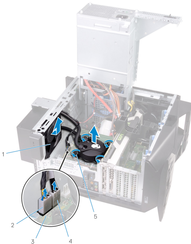
Abbildung 21. Entfernen der Prozessorkühlung-Baugruppe
