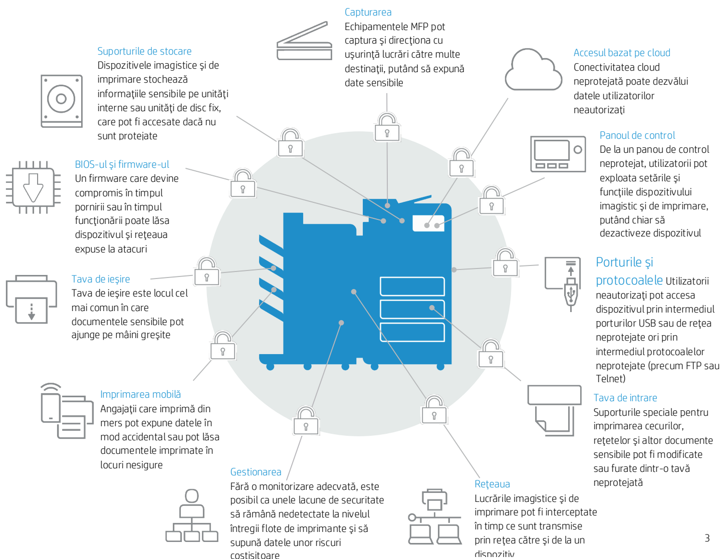
Figura 2. Punctele de vulnerabilitate din procesele imagistice și de imprimare
