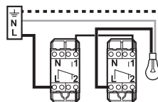
En va-et-vient lumineux
