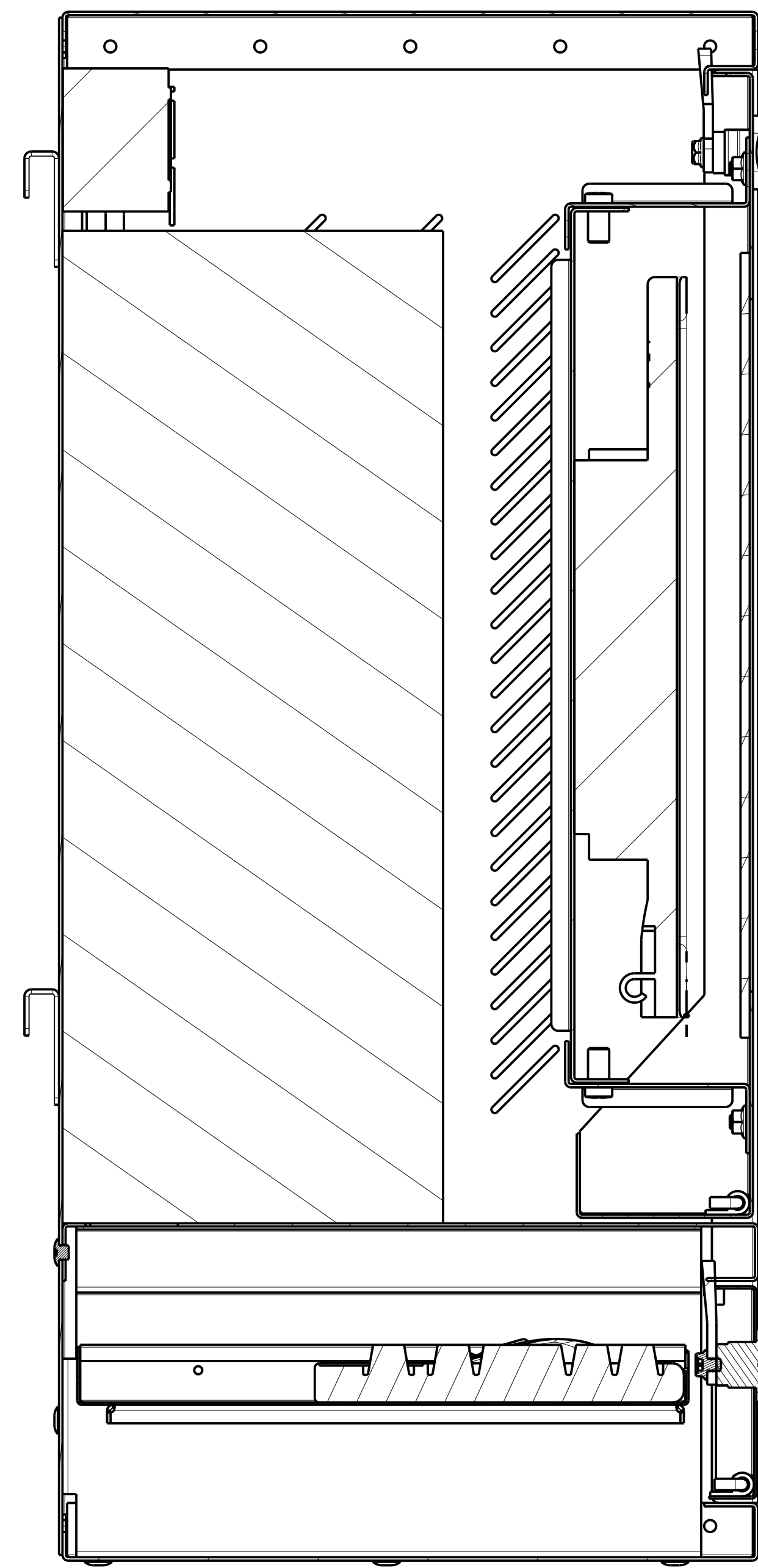
SEZIONE A-A
