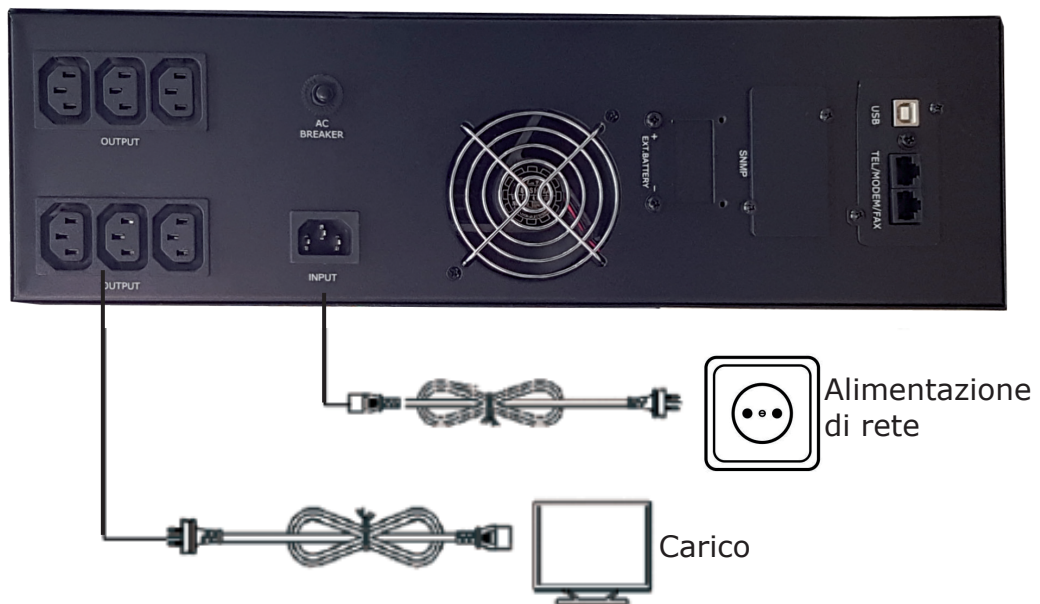
UPS Rack DC 48V Schema di collegamento ingresso/uscita
