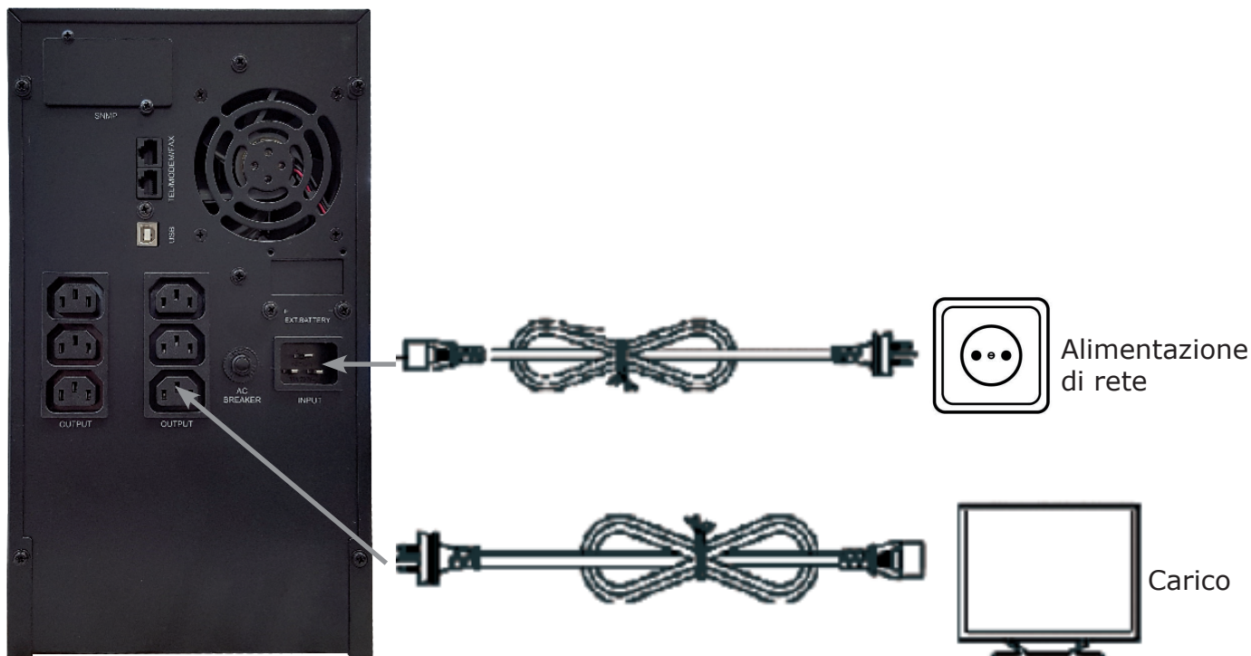
UPS Tower 3KVA Schema di collegamento ingresso/uscita
