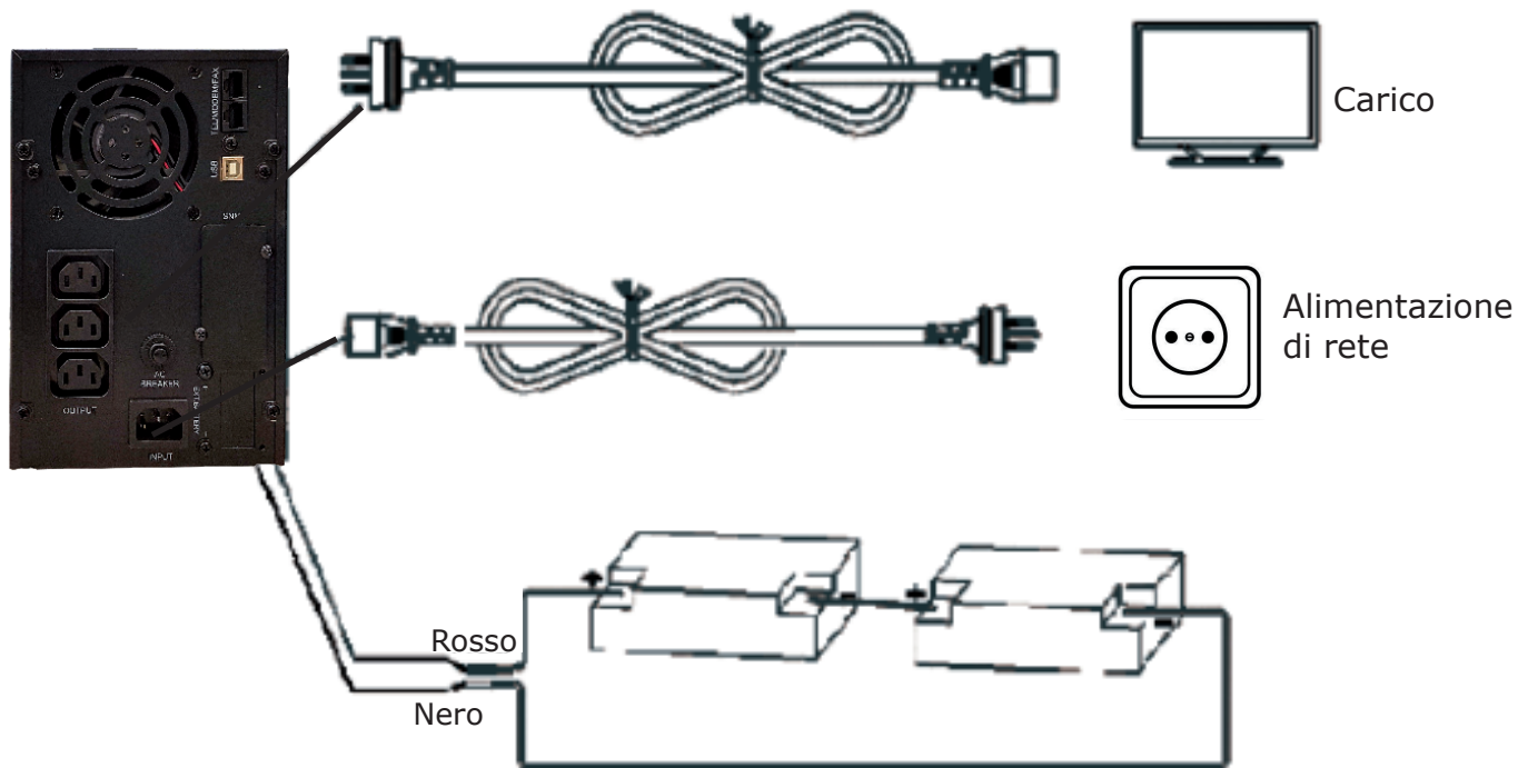
UPS Tower DC 24V Schema di collegamento ingresso/uscita
