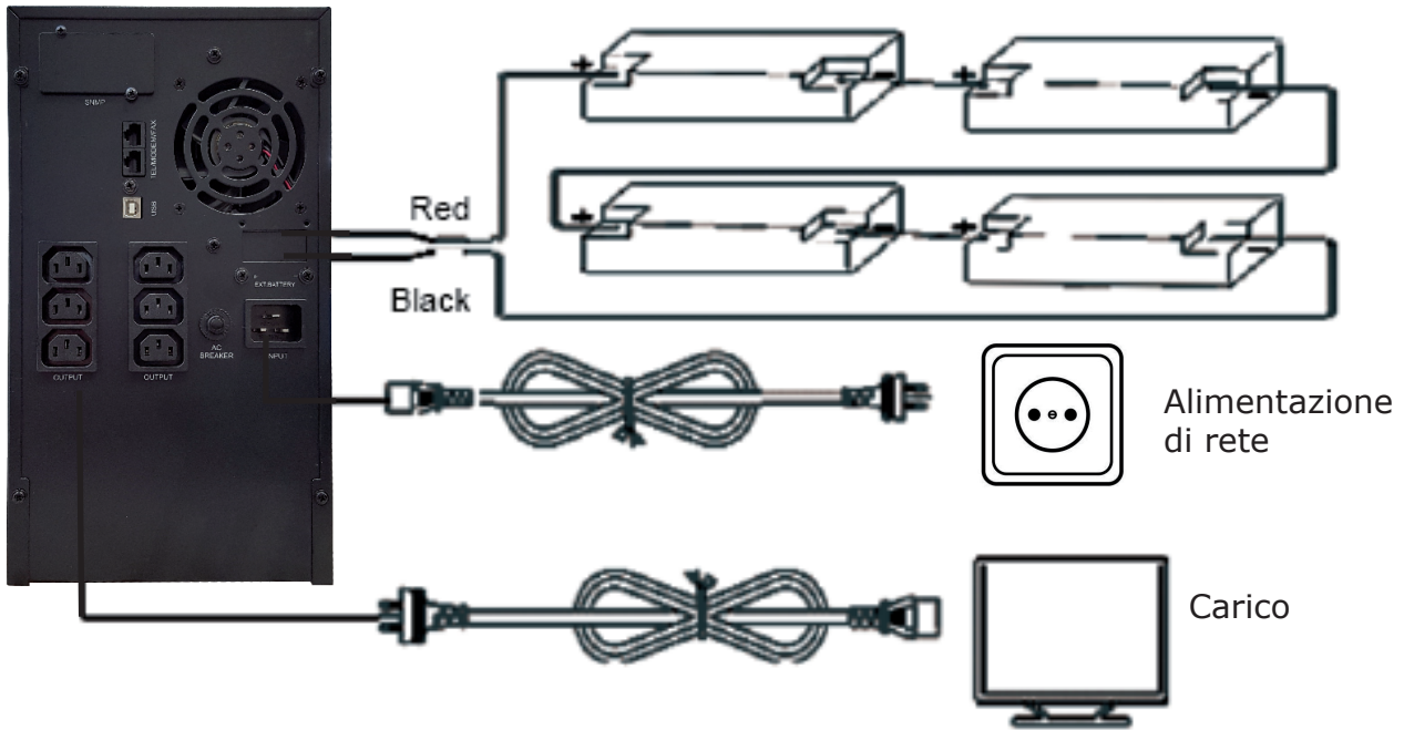
UPS Tower DC 48V Schema di collegamento ingresso/uscita
