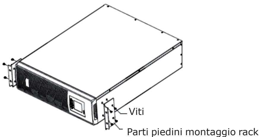
Schema di montaggio dei componenti per l'installazione UPS Rack
