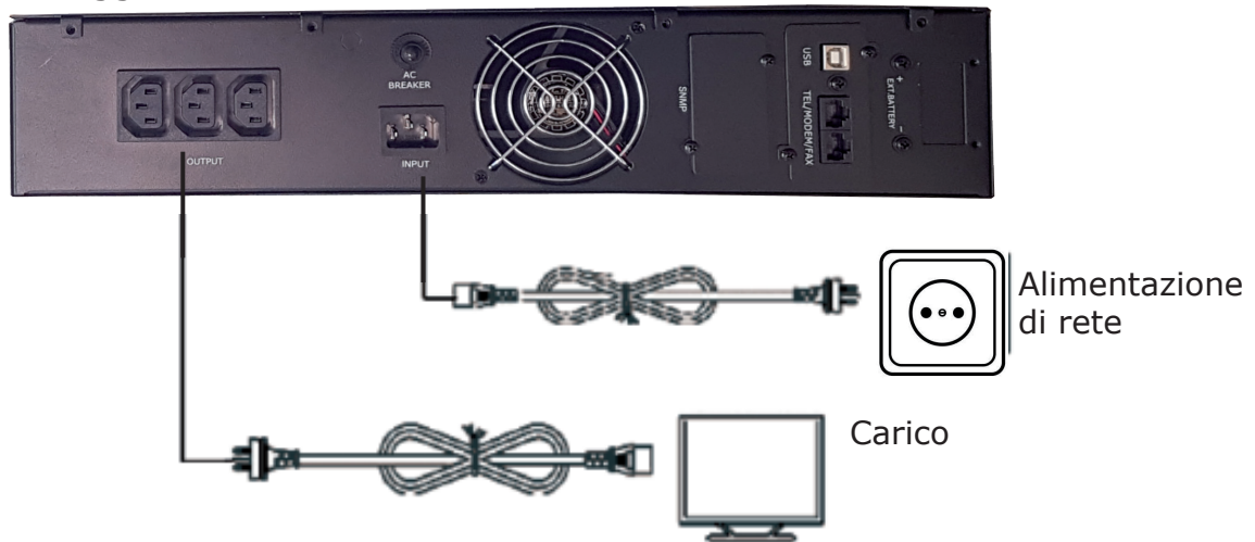
UPS Rack DC 24V Schema di collegamento ingresso/uscita
