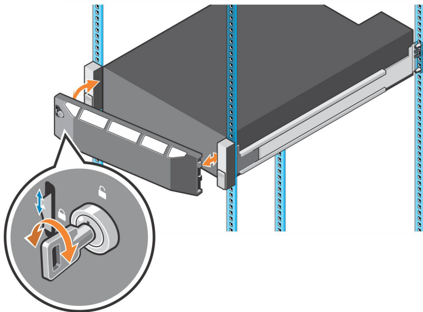
Rysunek 5. Osłona przednia
