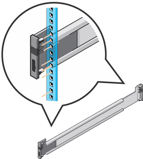
Rysunek 2. Mocowanie prowadnic w stelażu
