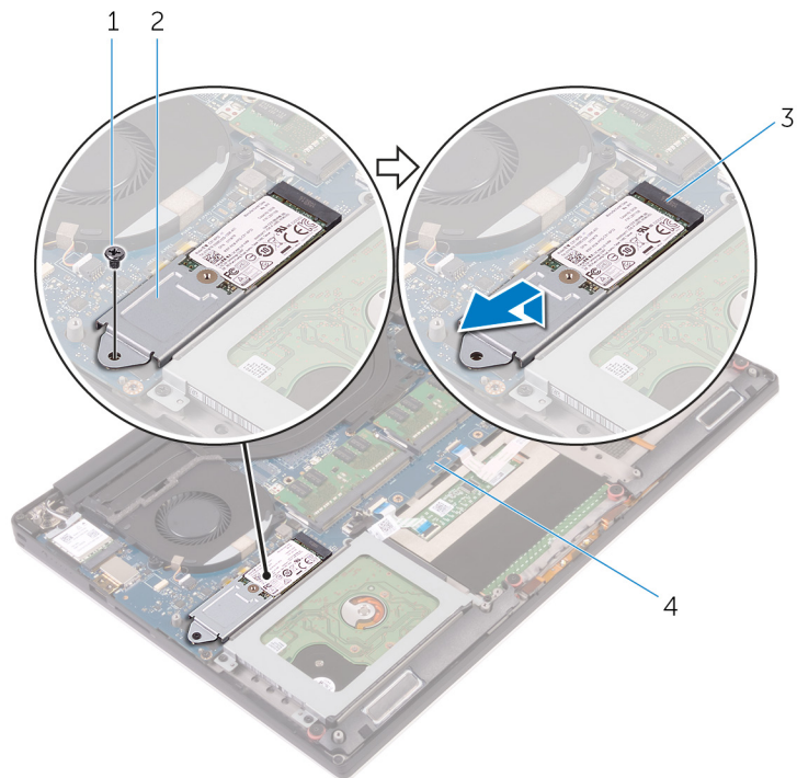
Figura 11. Rimozione del gruppo dell'unità a stato solido
