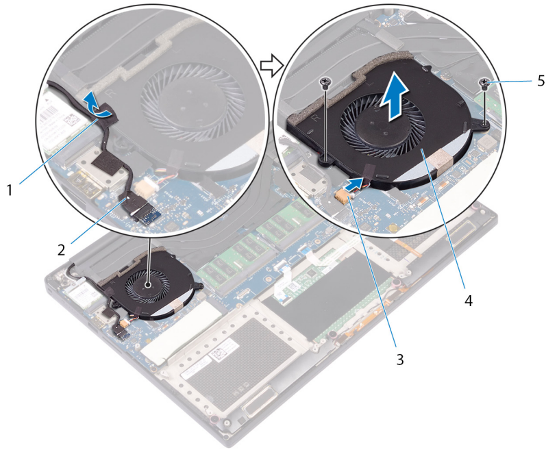
Figura 18. Rimozione della ventola destra
