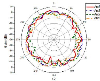
5GHz E-Plane
