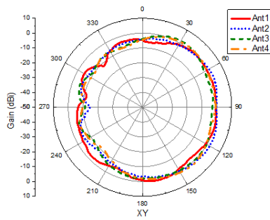
2.4GHz H-Plane
