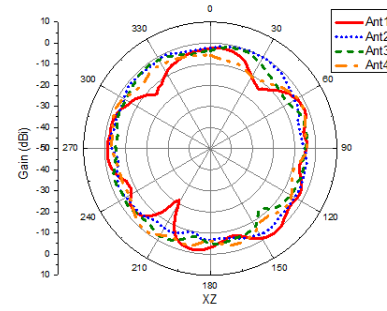
2.4GHz E-Plane
