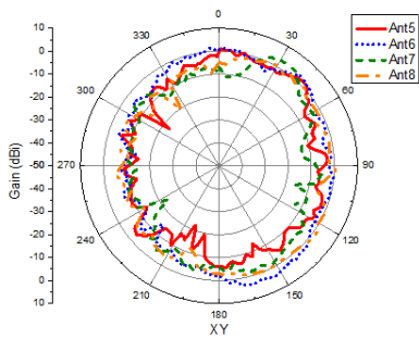
5GHz H-Plane
