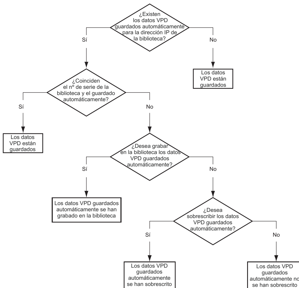
Figura 101. Guardar/Restaurar la configuración con cookies
