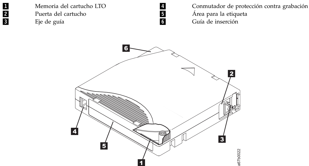
Figura 108. Cartucho de datos LTO Ultrium
