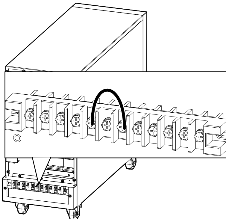
Vue arrière de l'ASI 10-15 kVA
