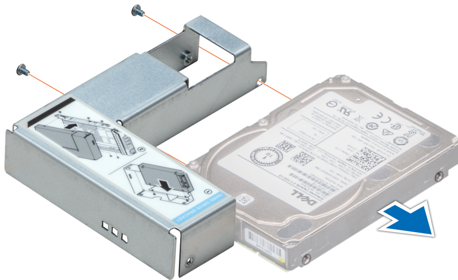
Figura 50. Extracción de una unidad de 2.5 pulgadas de un adaptador de unidad de 3.5 pulgadas
