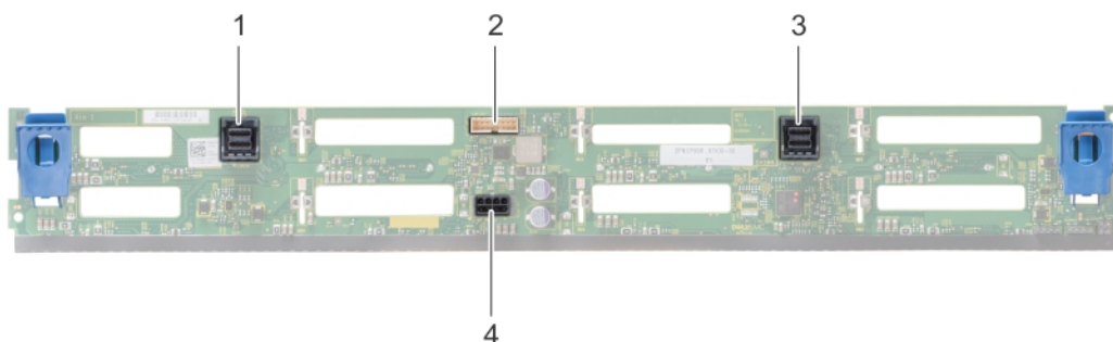
Figura 111. Vista posterior del plano posterior de una unidad de 8 x 3,5 pulgadas
