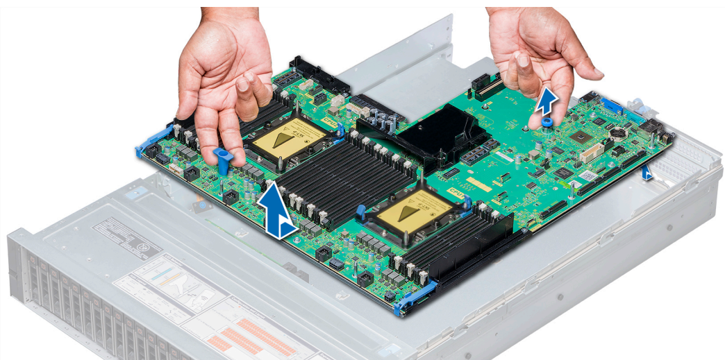
Figura 131. Extracción de la placa base
