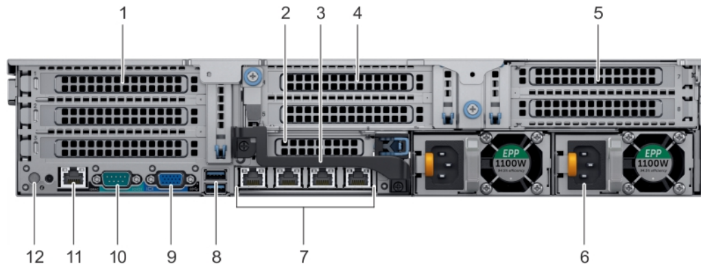
Figura 9. Vista posterior del sistema de tres soportes verticales
