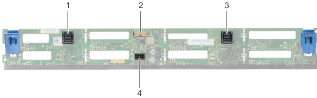
Figure 111. Vue arrière du fond de panier de 8 disques durs de 3,5 pouces
