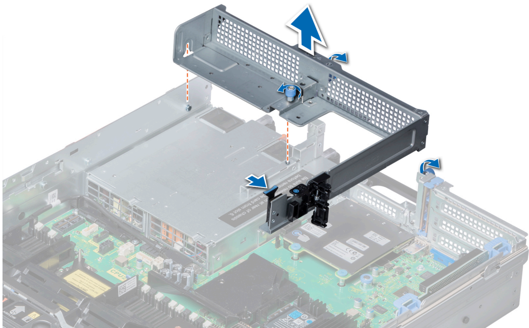
Figure 75. Retrait du cache des cartes de montage 2 et 3
