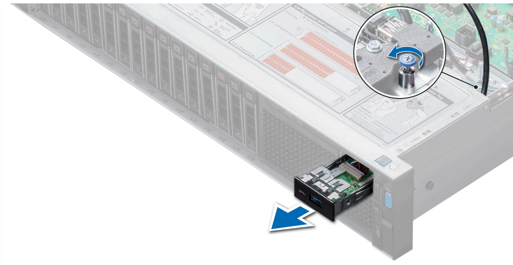
Figure 123. Retrait du module USB 3.0
