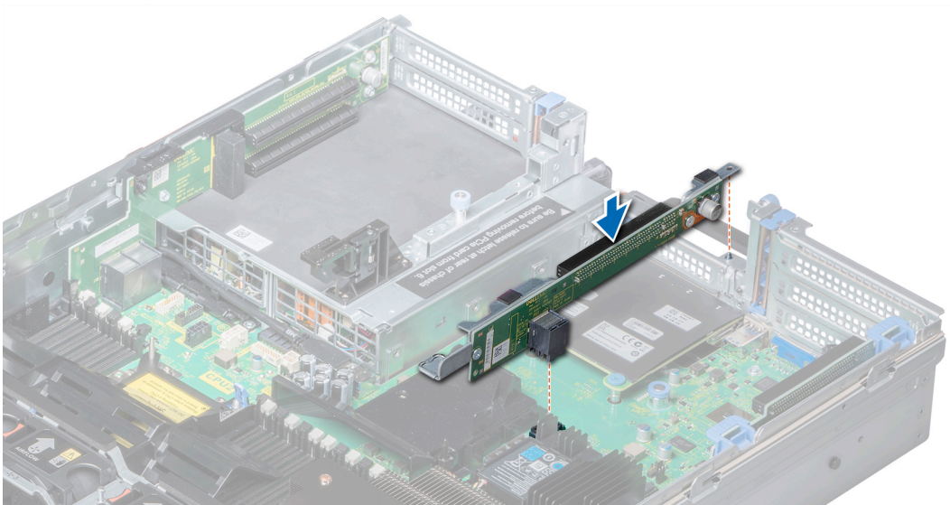
Figure 84. Installation de la carte de montage pour carte d'extension 2
