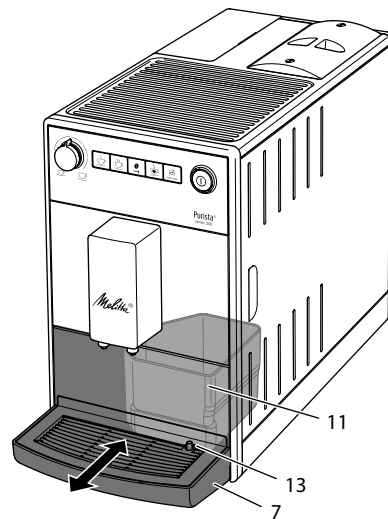
Joon. 8: Tilkumisaluse ja kohvipaksusah- kli tühjendamine
