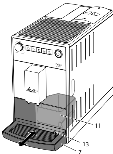
Afb. 8: Lekbakje en residubak legen
