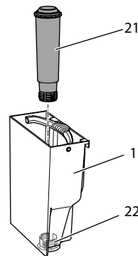
Fig. 15: Skru vannfilteret inn eller ut
