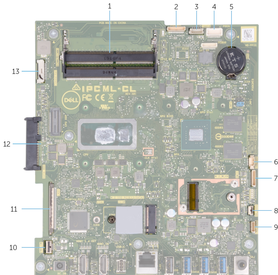
Figure 1. Connecteurs de la carte système
