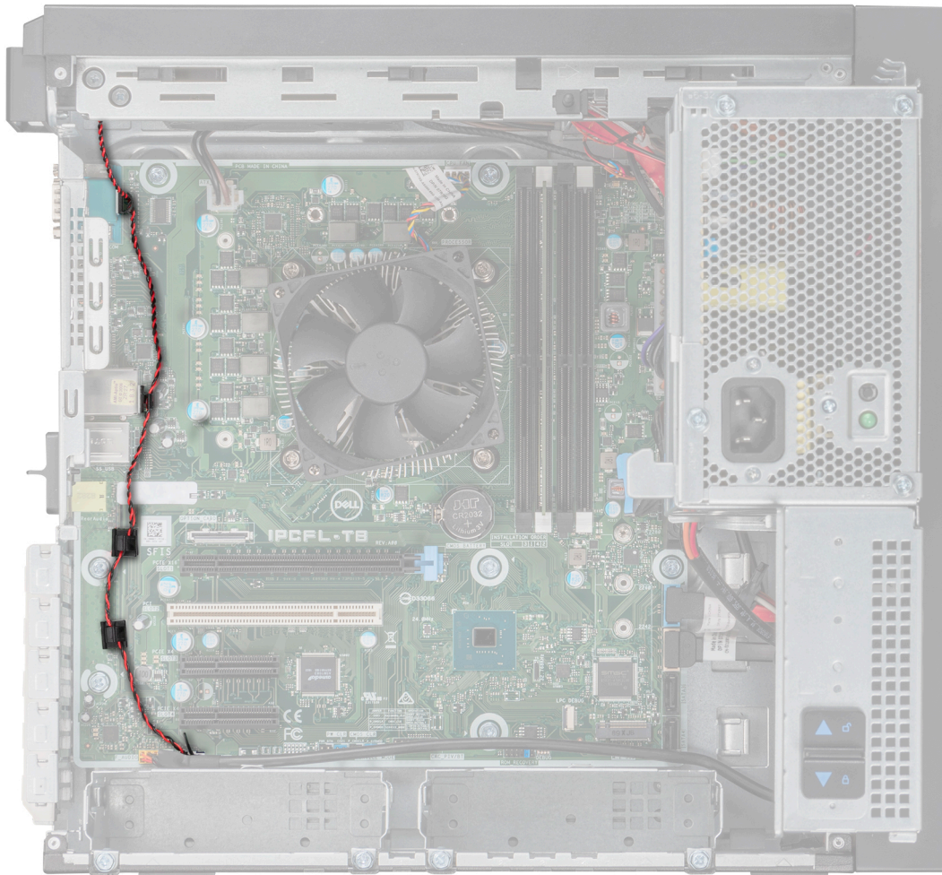
Abbildung 36. Lautsprecherkabelführung
