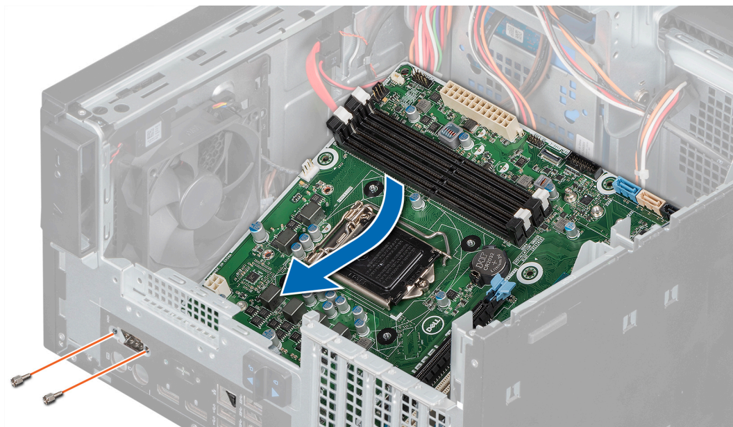
Figure 50. Installation de la carte système
