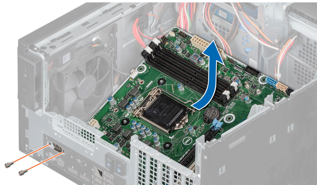
Figure 49. Retrait de la carte système
