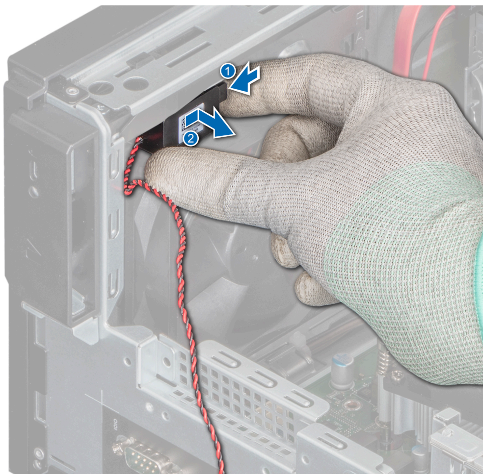
Figure 34. Retrait du haut-parleur
