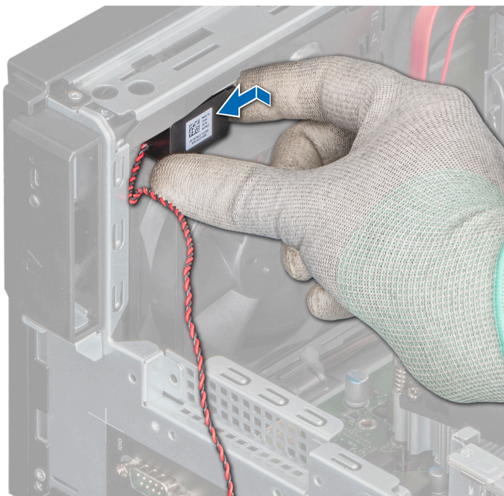
Figure 35. Installation du haut-parleur
