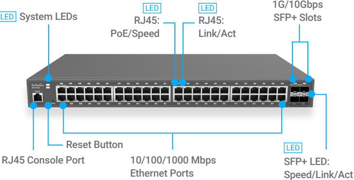
CloudSwitch L2Plus 48 (ECS1552)
