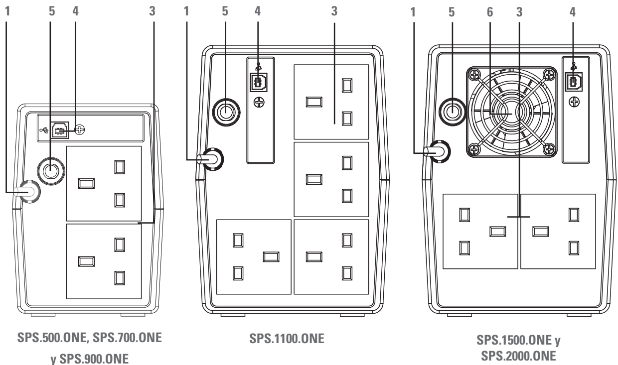
Fig. 3. Vistas posteriores con tomas de salida inglesa (UK).
