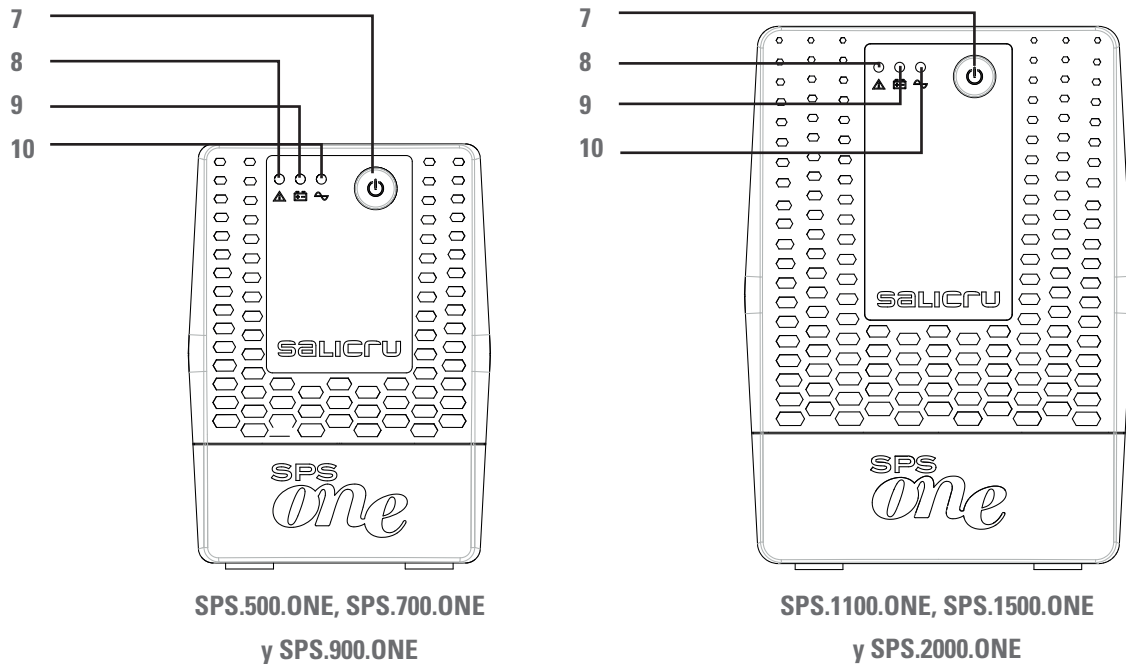
Fig. 1. Vistas frontales SPS.ONE.
