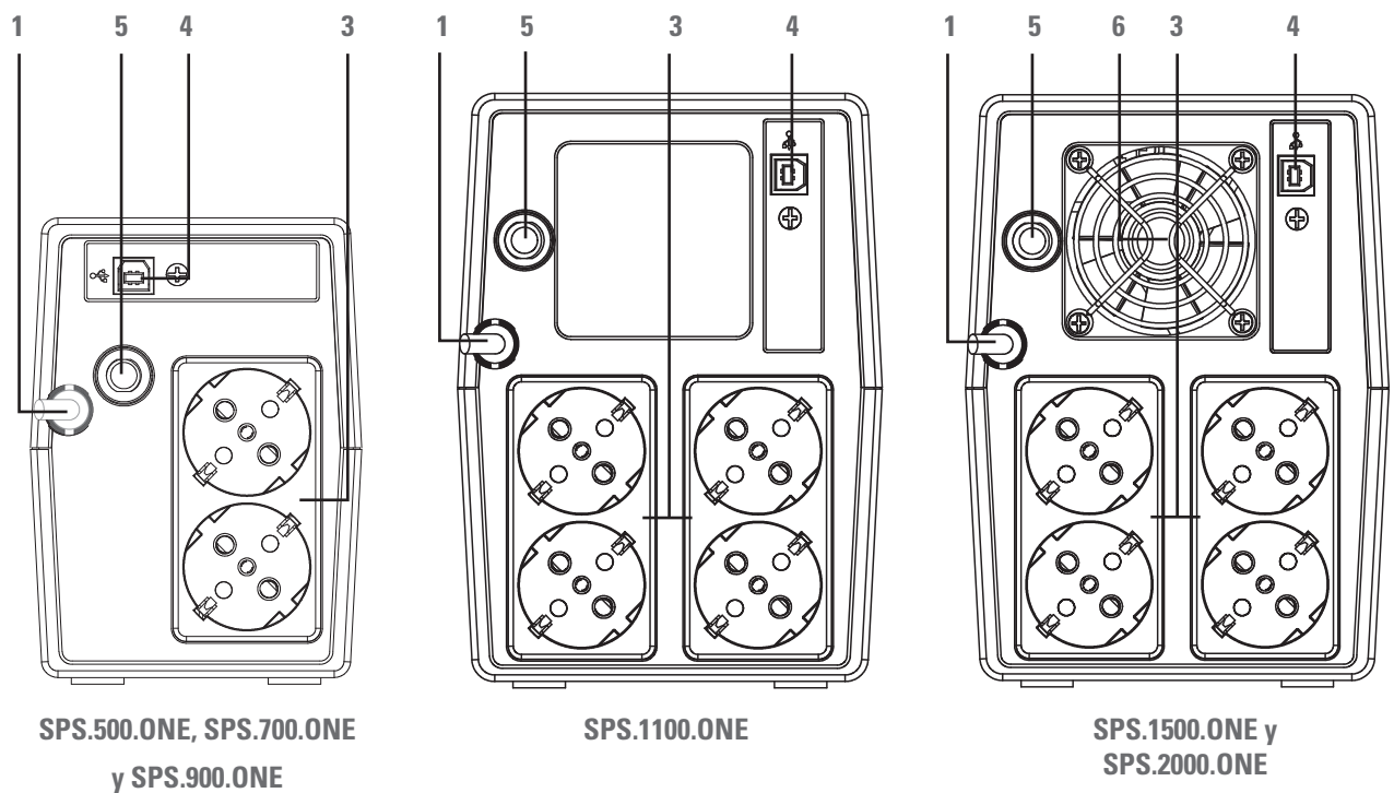
Fig. 2. Vistas posteriores con tomas de salida schuko.
