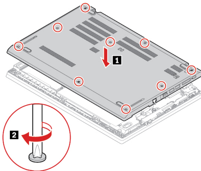
Figura 7. Installazione dell'assieme del coperchio della base per L590
