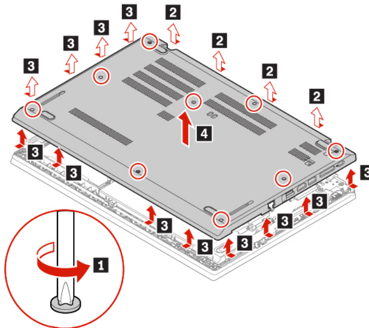
Figura 5. Rimozione dell'assieme del coperchio della base per L590
