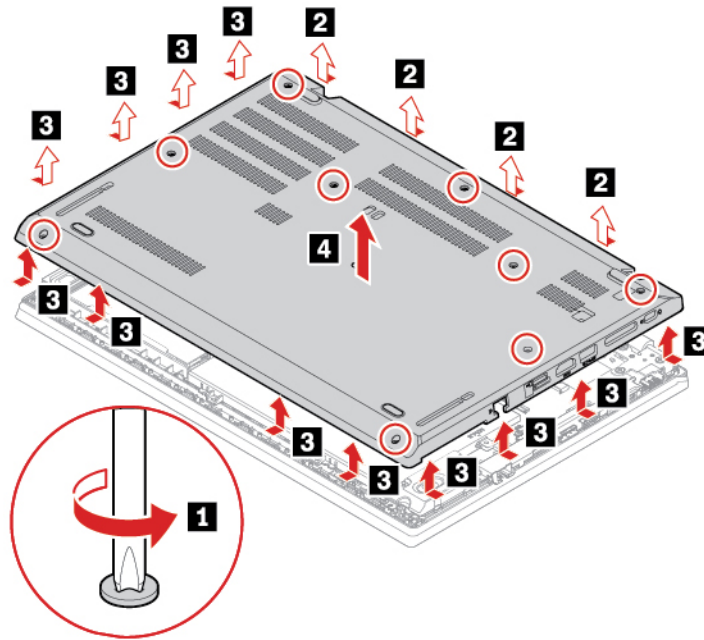
Figura 4. Rimozione dell'assieme del coperchio della base per L490
