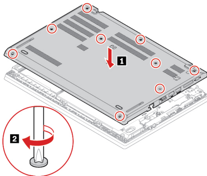
Figura 6. Installazione dell'assieme del coperchio della base per L490
