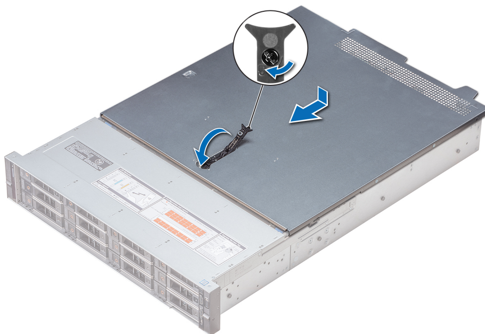
Figure 25. Installation du capot du système
