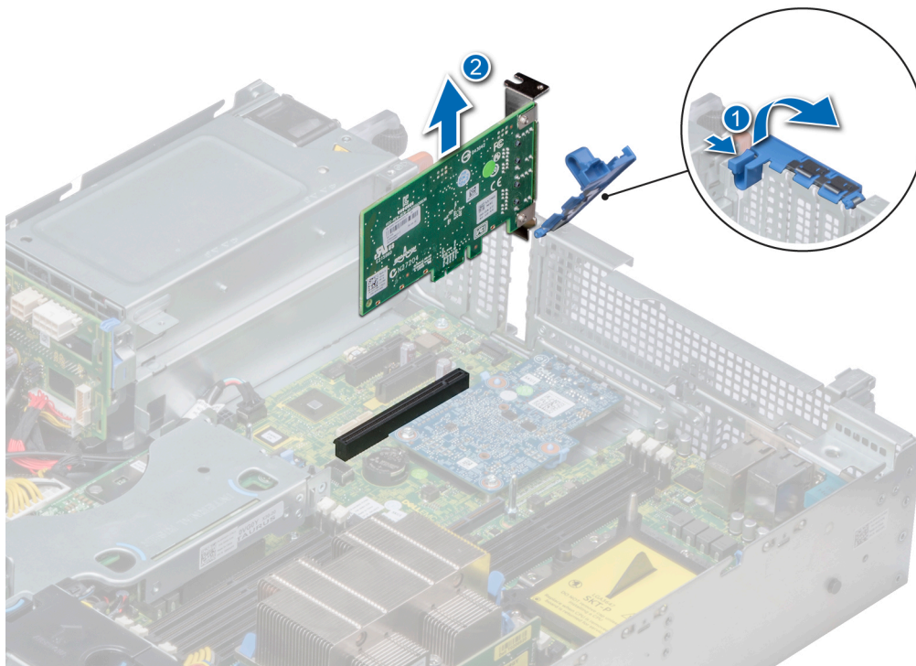
Figure 76. Retrait d'une carte d'extension de la carte système
