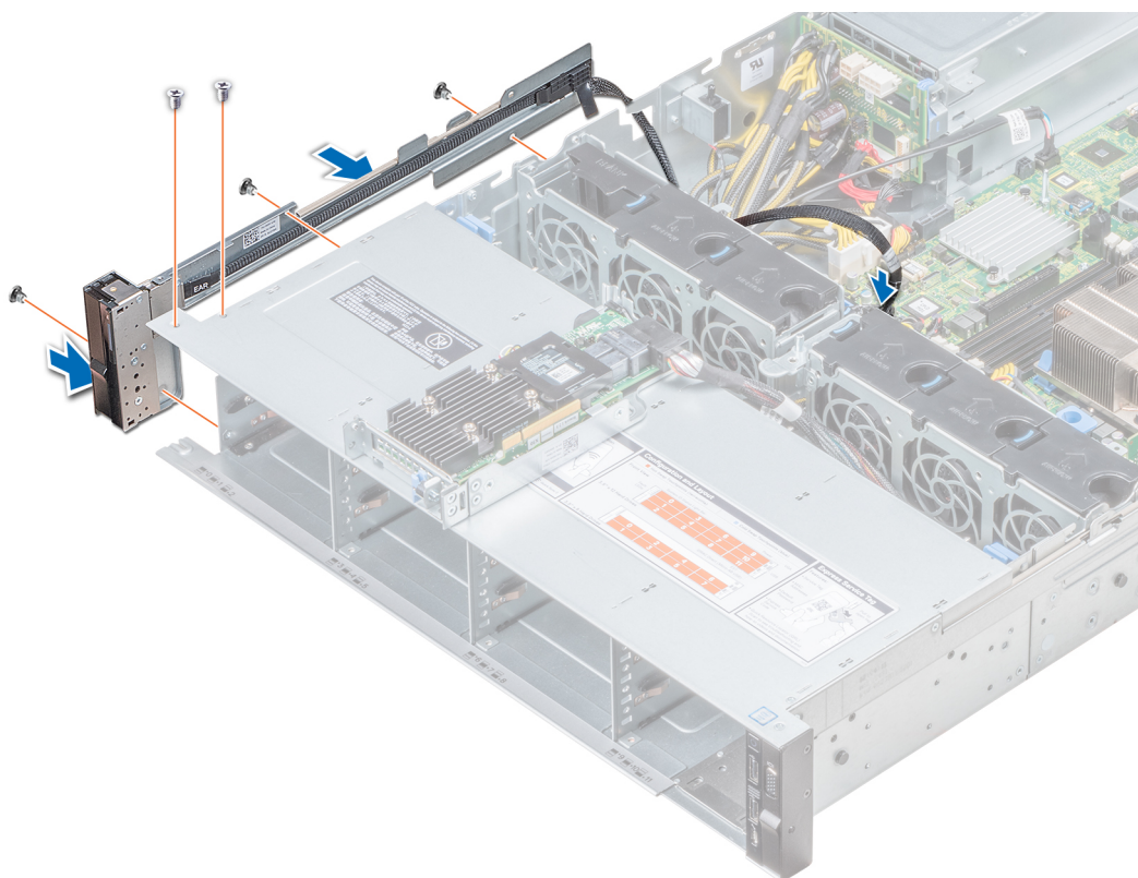
Figure 124. Installation du panneau de commande gauche
