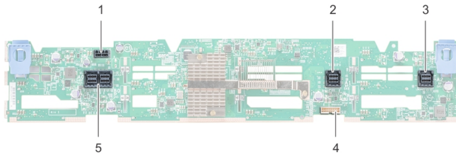
Figure 97. Backplane à 12 disques de 3,5 pouces
