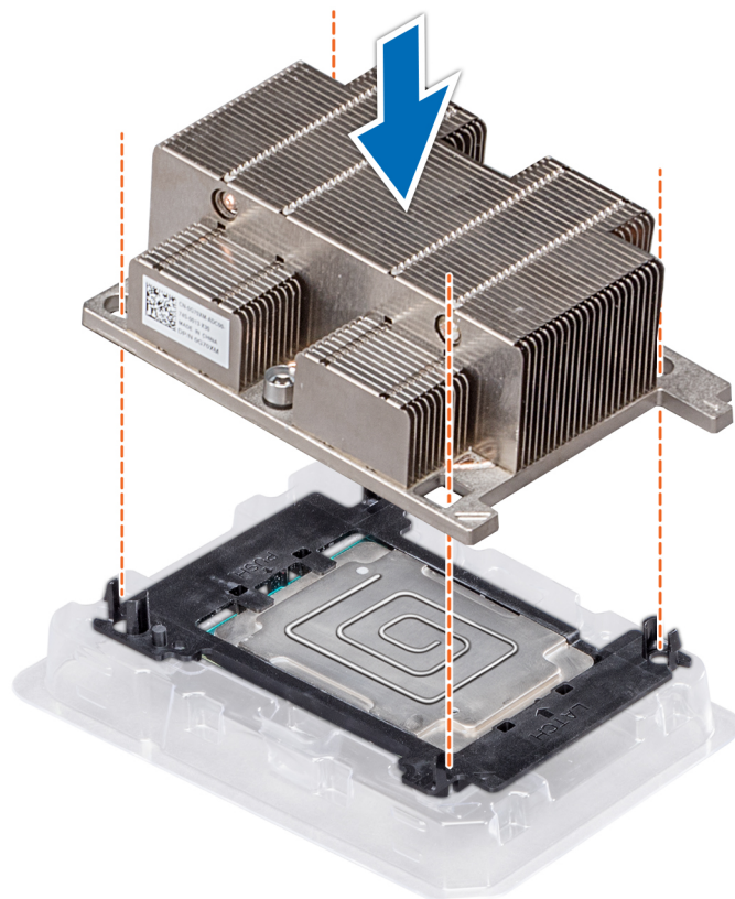
Figure 62. Installation du dissipateur de chaleur sur le processeur
