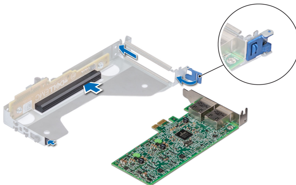
Figure 73. Installation d'une carte d'extension dans la carte de montage mi-hauteur
