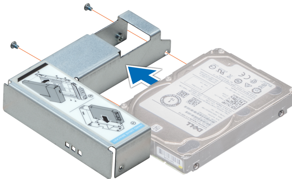
Figure 47. Installation d'un disque de 2,5 pouces dans un adaptateur de disque de 3,5 pouces
