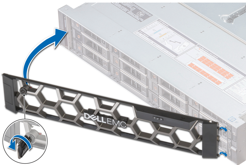
Figure 23. Installation du cadre avant avec le panneau LCD
