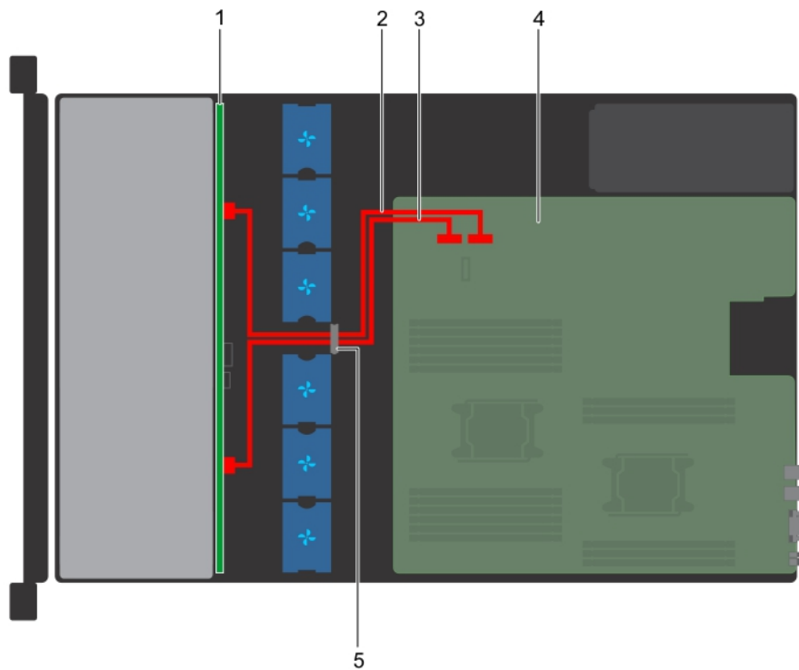
Figure 107. Acheminement des câbles : backplane de 8 disques de 3,5 pouces
