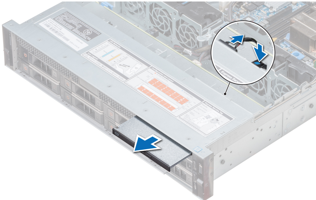
Figure 113. Retrait du lecteur optique
