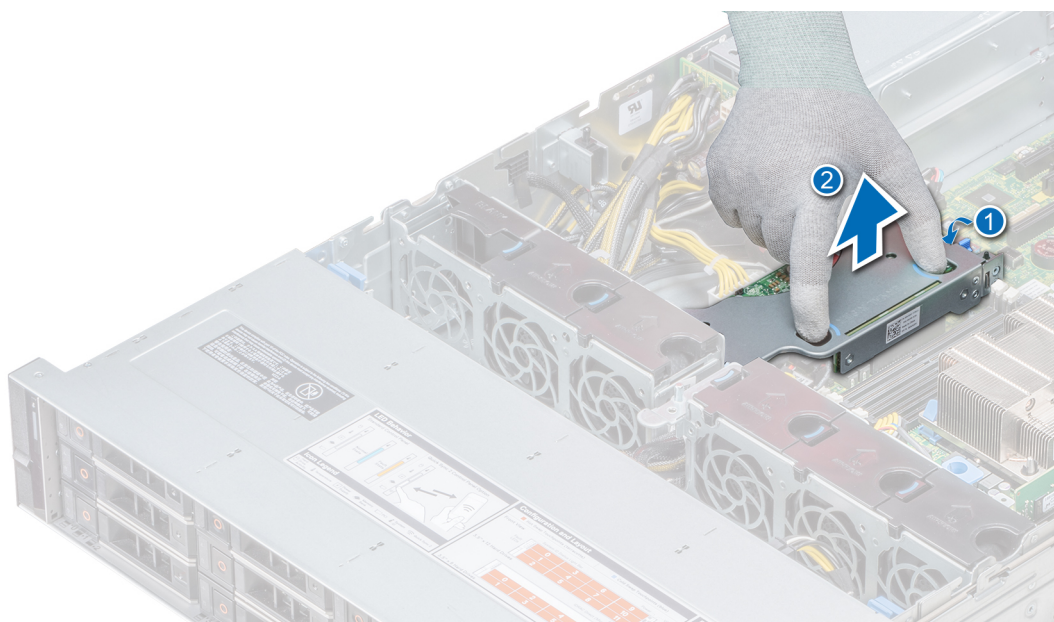
Figure 36. Retrait de la carte de montage PERC interne
