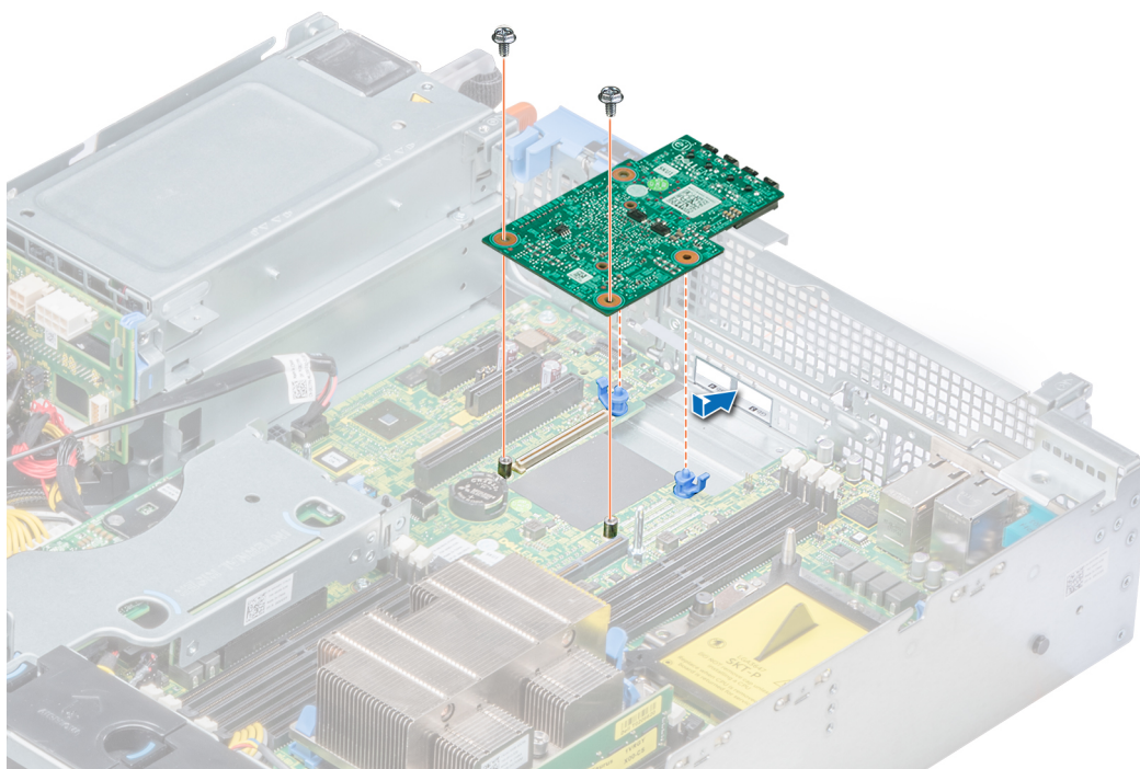
Figure 95. Installation de la carte de montage LOM
