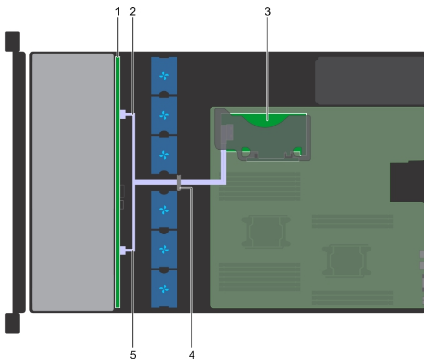
Figure 105. Acheminement des câbles : backplane de 8 disques de 3,5 pouces avec carte de montage PERC interne
