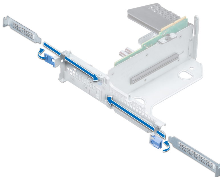
Figure 69. Installation d'une plaque de recouvrement pour la carte de montage papillon
