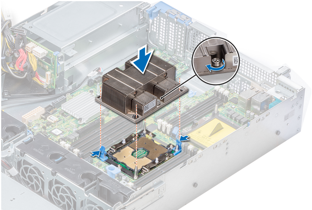
Figure 63. Installation du module du processeur et du dissipateur de chaleur
