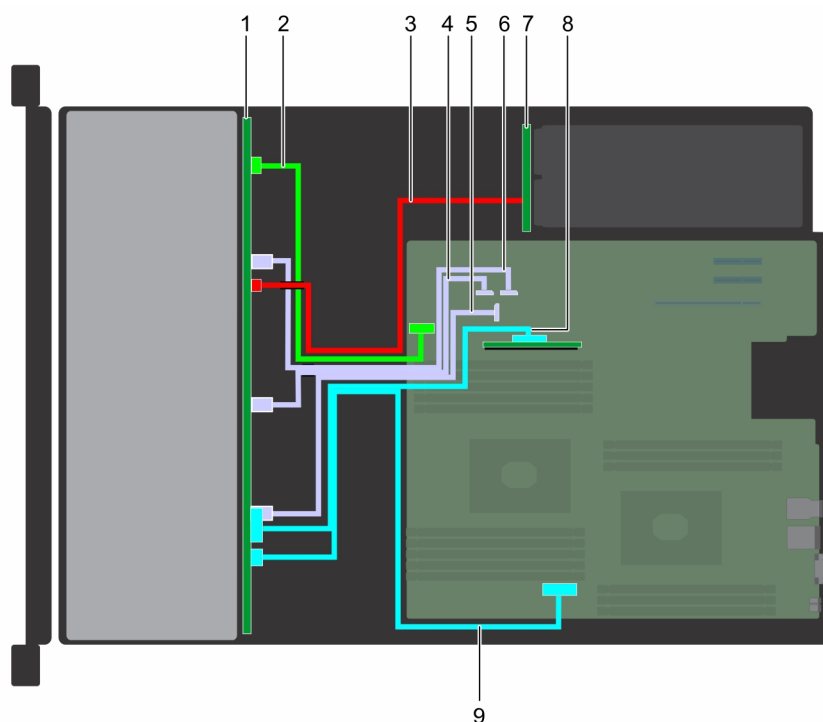
Figure 108. Acheminement des câbles : backplane de 2 disques hybrides de 3,5 pouces avec SSD NVMe U.2
