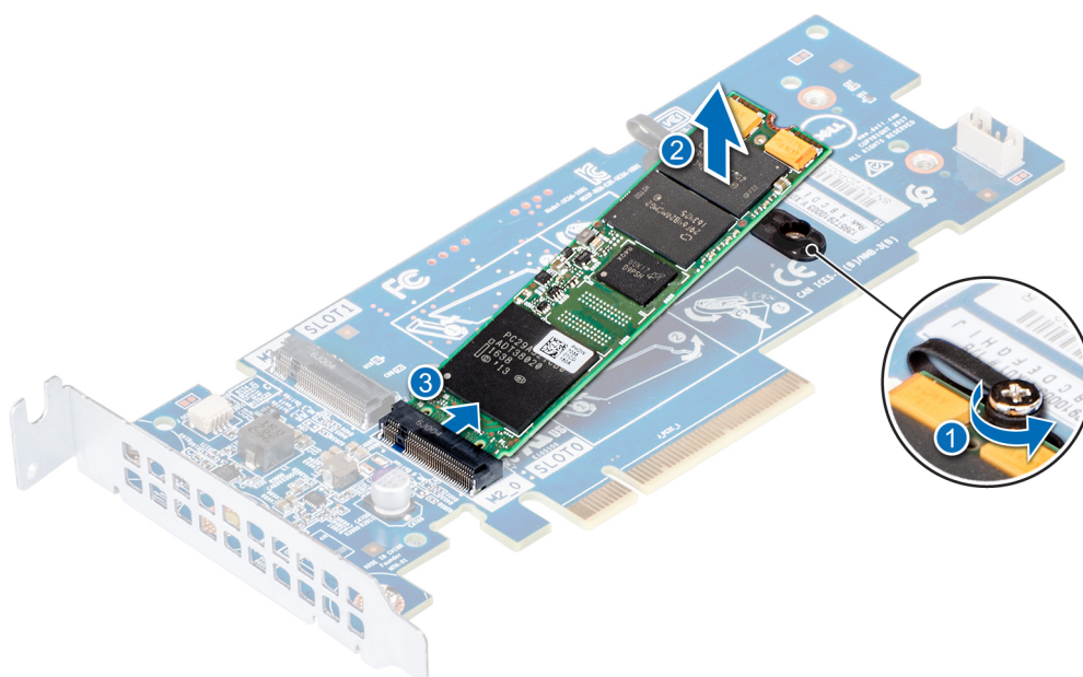
Figure 88. Retrait du module SSD M.2
