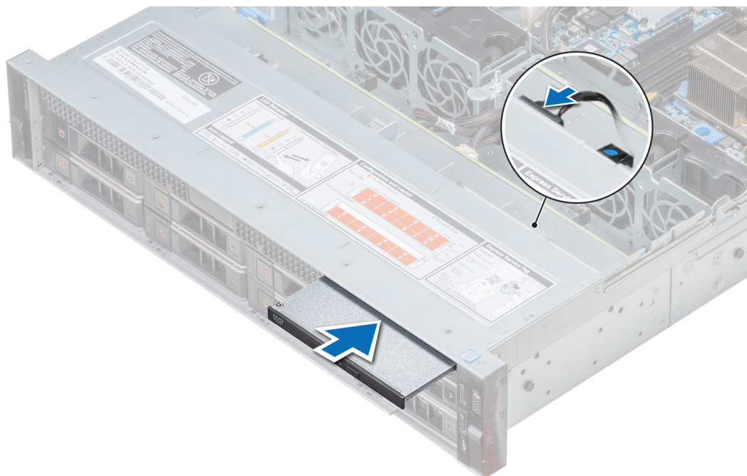
Figure 114. Installation du lecteur optique
