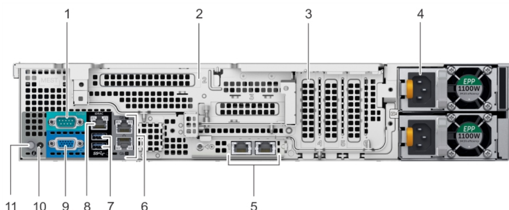
Figure 11. Caractéristiques du panneau arrière d'un système équipé de 12 disques (arrière) de 3,5 pouces avec une carte de montage Butterfly
