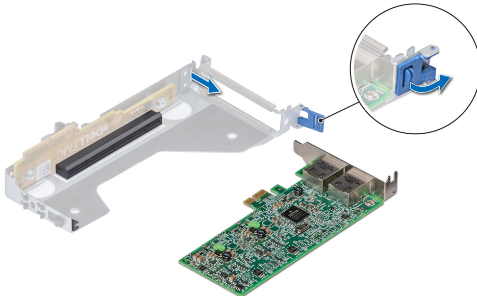
Figure 64. Retrait d'une carte d'extension de la carte de montage mi-hauteur
