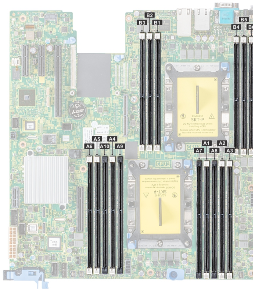
Figure 54. Emplacement des sockets de mémoire
