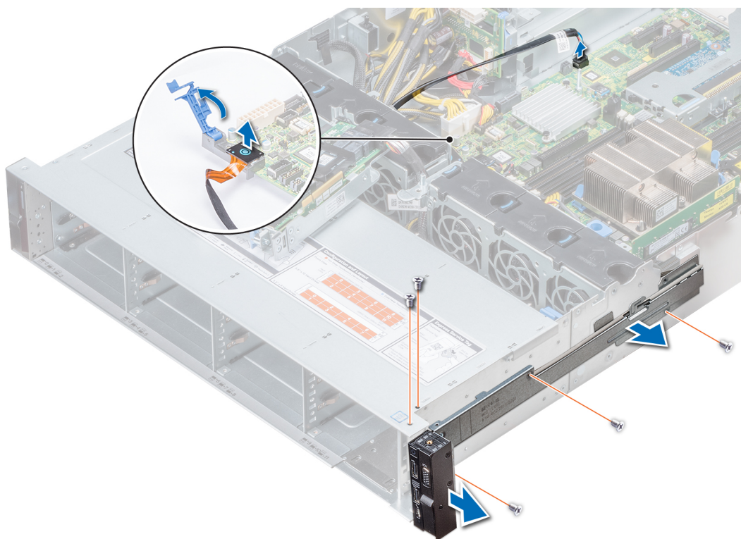
Figure 125. Retrait du panneau de commande droit
