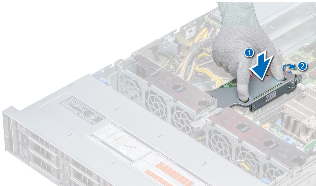
Figure 39. Installation de la carte de montage PERC interne
