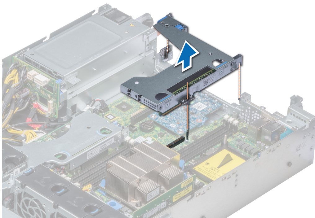
Figure 82. Retrait de la carte de montage pleine hauteur X1
