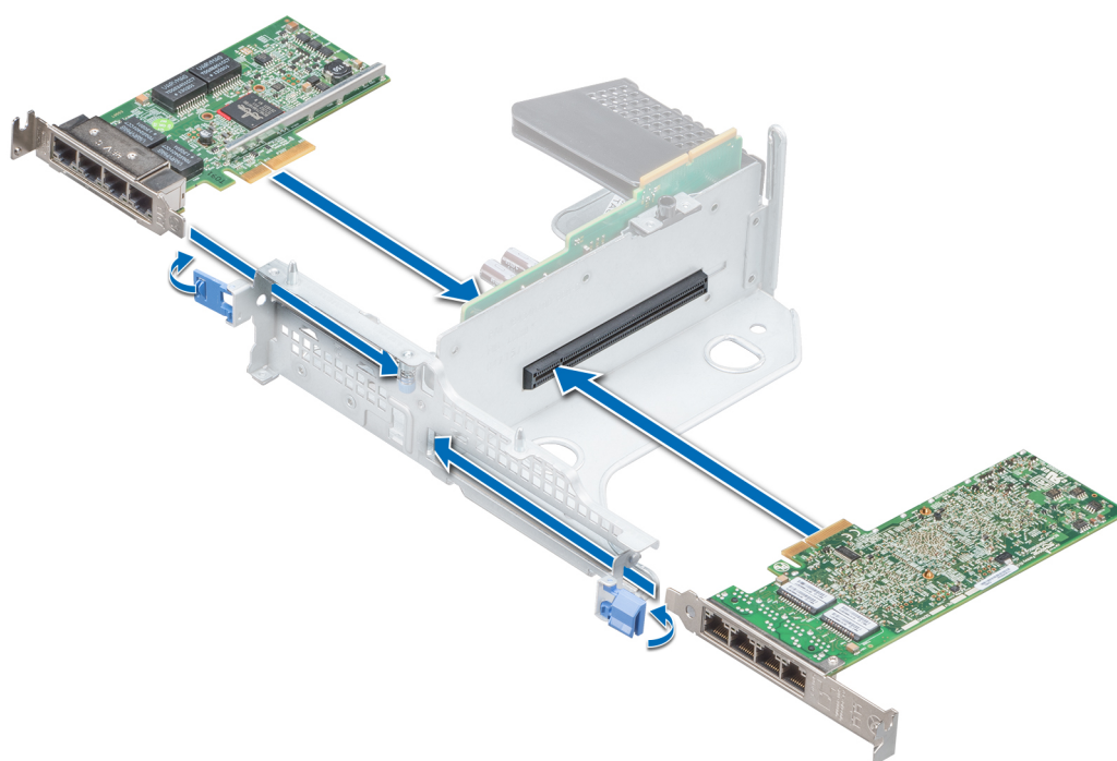
Figure 75. Installation d'une carte d'extension dans la carte de montage papillon
