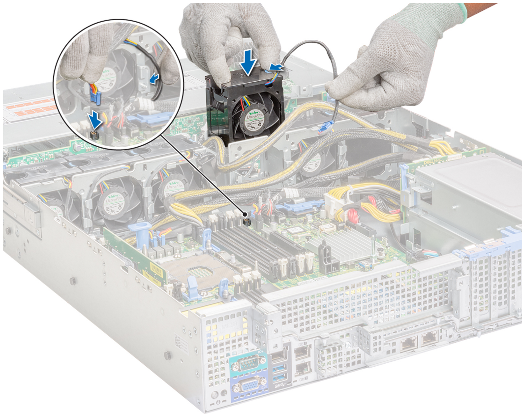
Figure 34. Installation du ventilateur de refroidissement
