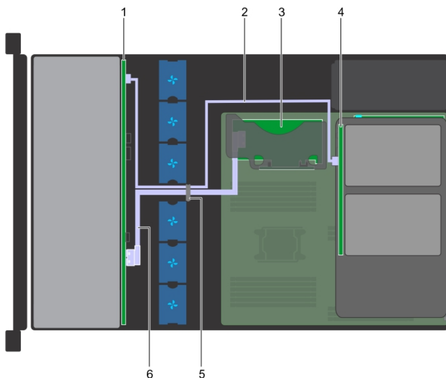
Figure 104. Acheminement des câbles : backplane de 12 disques de 3,5 pouces et backplane de 2 disques arrière de 3,5 pouces avec carte de montage PERC interne
