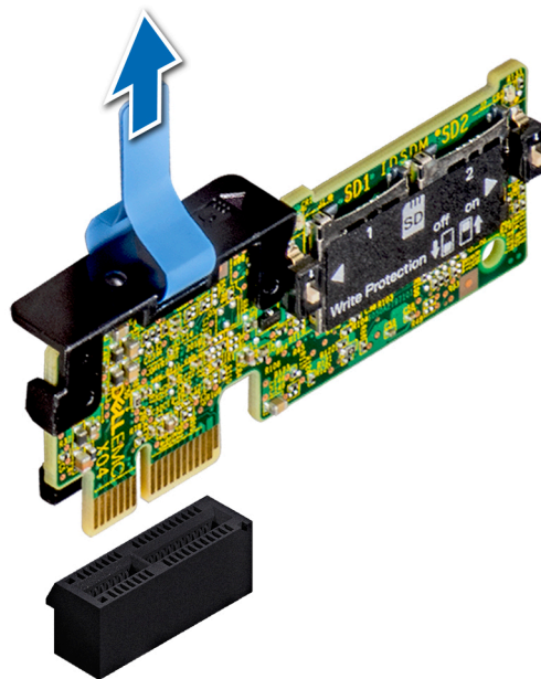
Figure 92. Retrait de la carte IDSDM/vFlash en option
