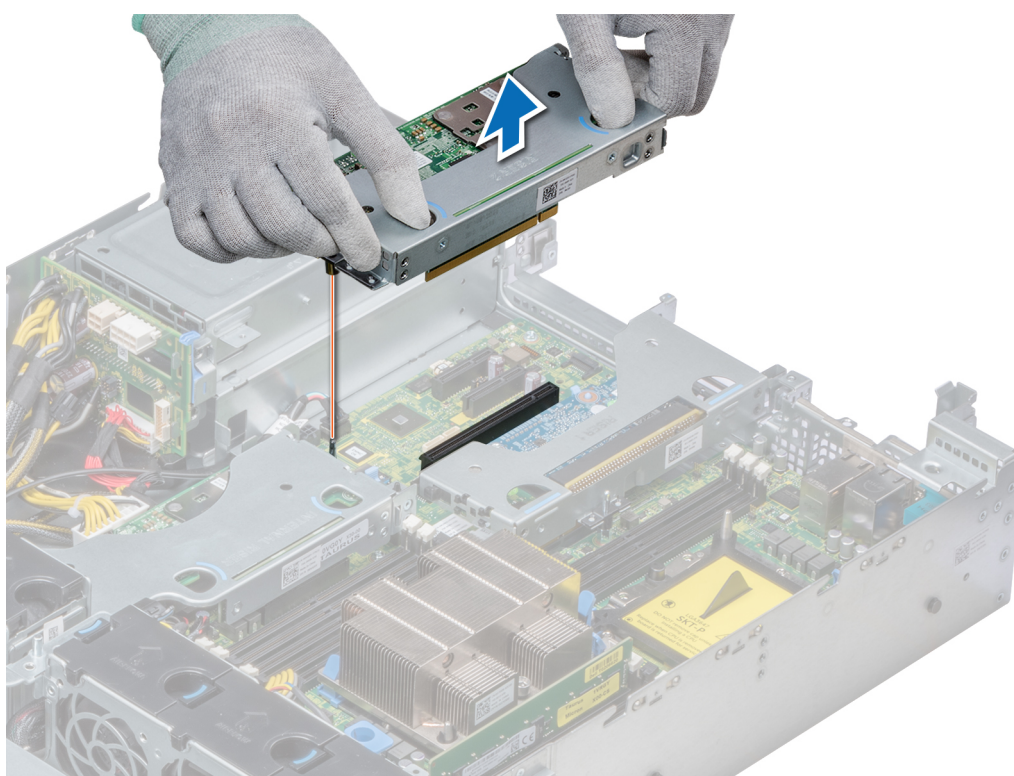
Figure 81. Retrait de la carte de montage mi-hauteur gauche
