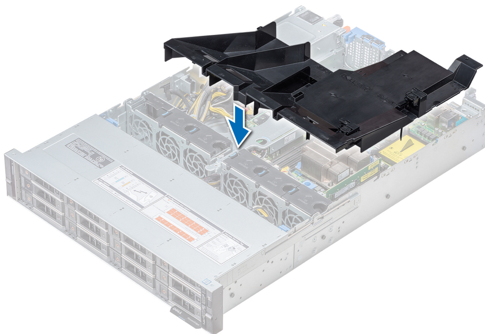
Figure 31. Installation du carénage d'aération
