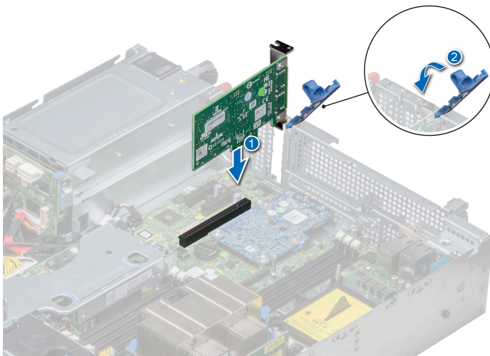
Figure 79. Installation d'une carte d'extension sur la carte système
