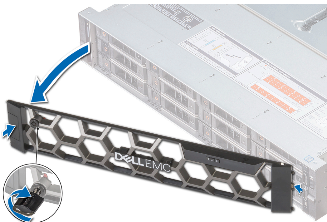
Figure 22. Retrait du cadre avant avec le panneau LCD
