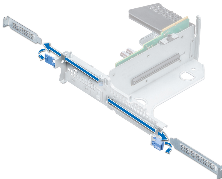
Figure 72. Retrait d'une plaque de recouvrement pour la carte de montage papillon
