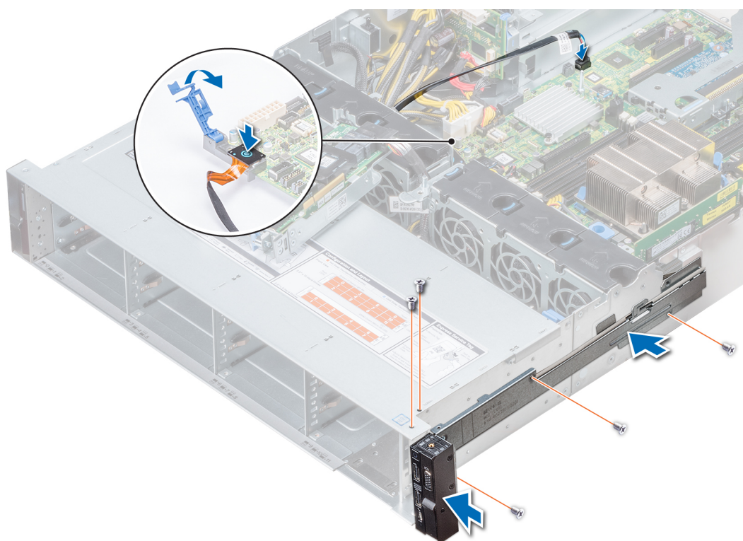
Figure 126. Installation du panneau de commande droit
