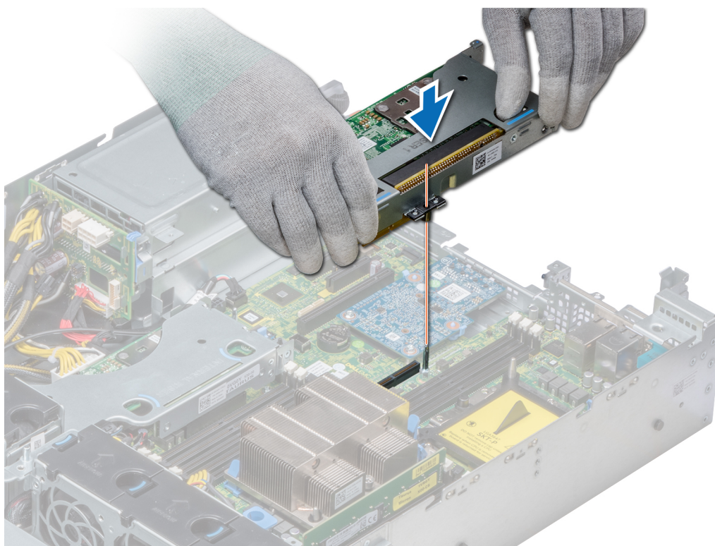
Figure 80. Retrait de la carte de montage mi-hauteur droite
