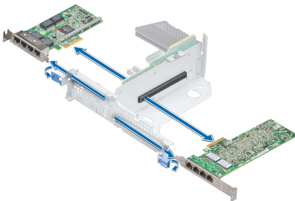
Figure 66. Retrait d'une carte d'extension de la carte de montage papillon
