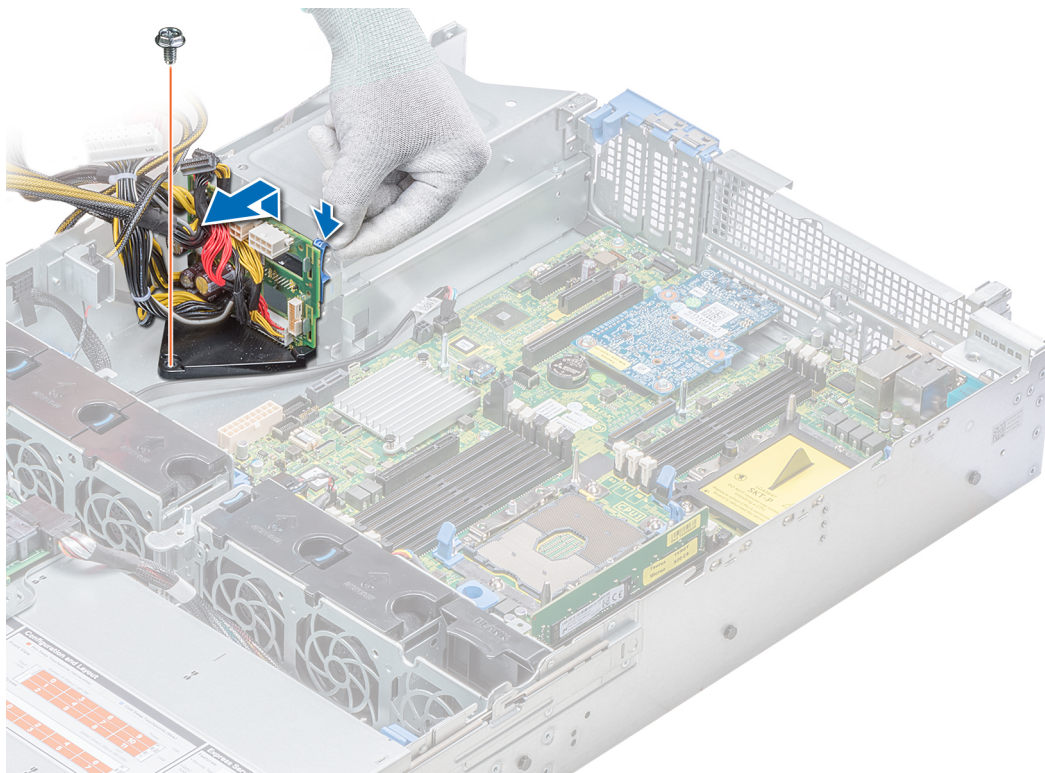
Figure 121. Retrait de la carte intercalaire d'alimentation
