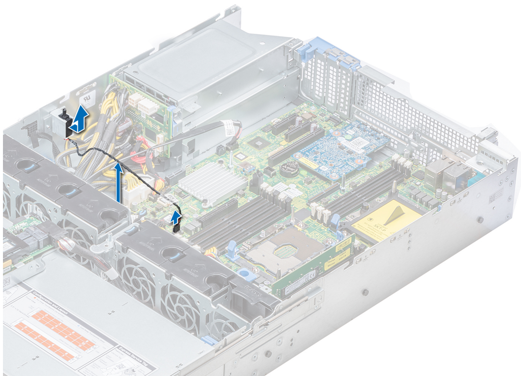
Figure 42. Retrait d'un commutateur d'intrusion
