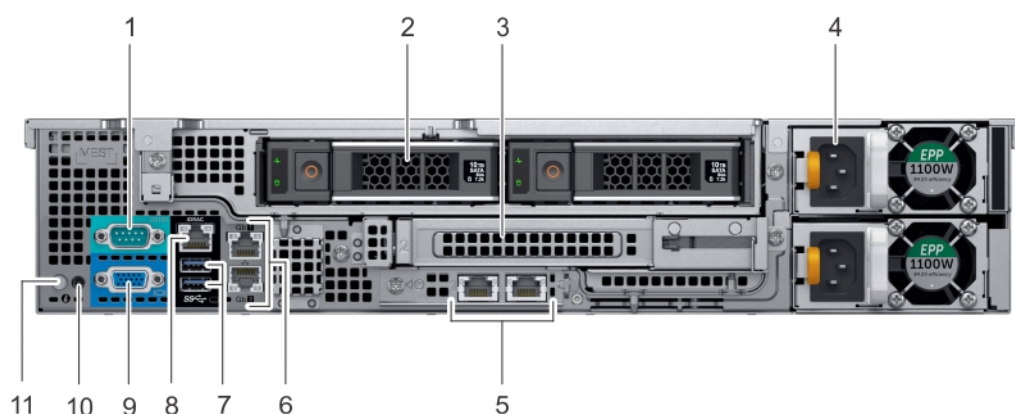
Figure 10. Caractéristiques du panneau arrière d'un système équipé de 12 disques (arrière) de 3,5 pouces et de 2 disques (arrière) de 2,5 pouces
