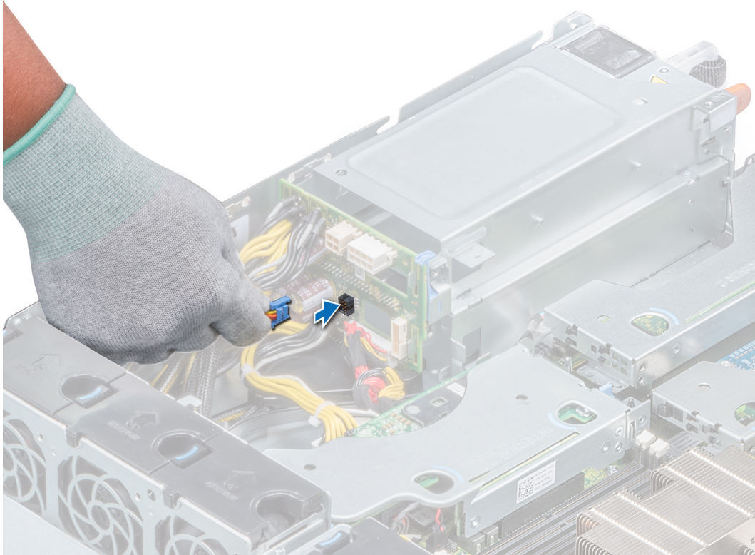
Figure 35. Connexion du câble du ventilateur au connecteur PIB
