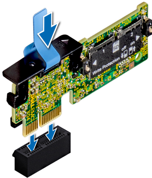
Figure 93. Installation d'une carte IDSDM/vFlash (en option)
