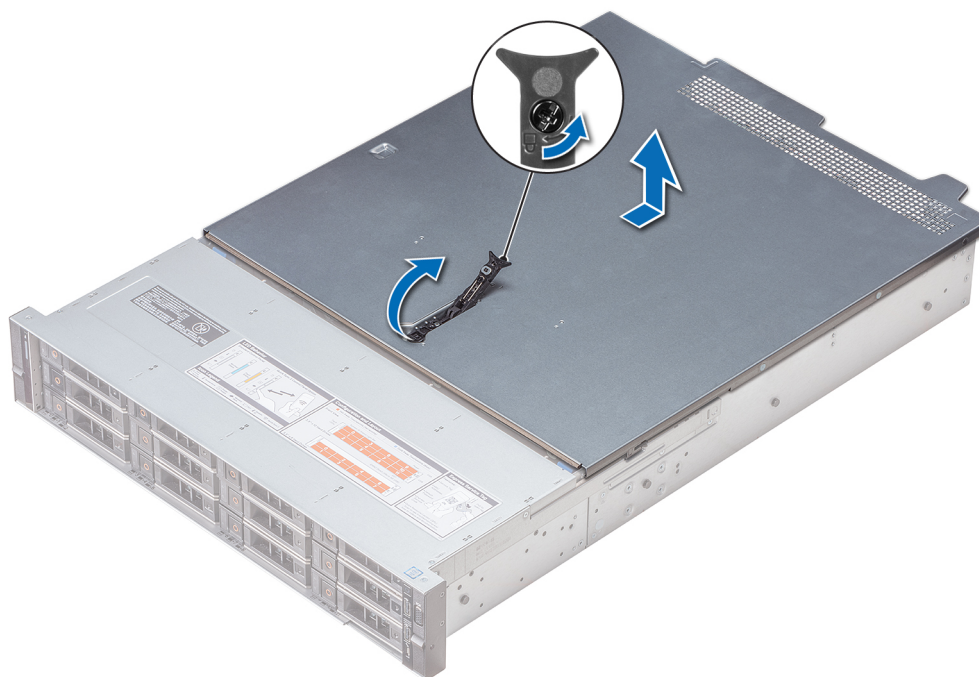
Figure 24. Retrait du capot du système
