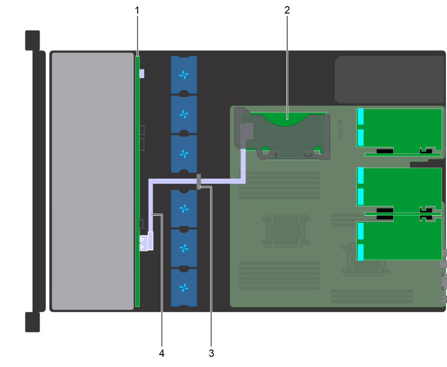
Figure 106. Acheminement des câbles : fond de panier de 12 disques de 3,5 pouces avec carte de montage PERC interne
