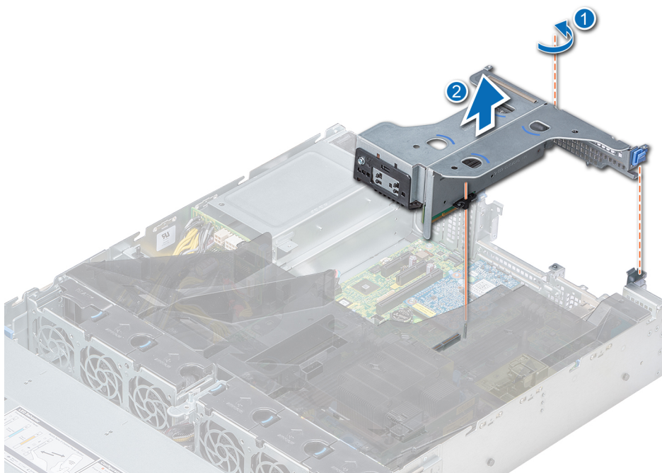
Figure 83. Retrait de la carte de montage papillon
