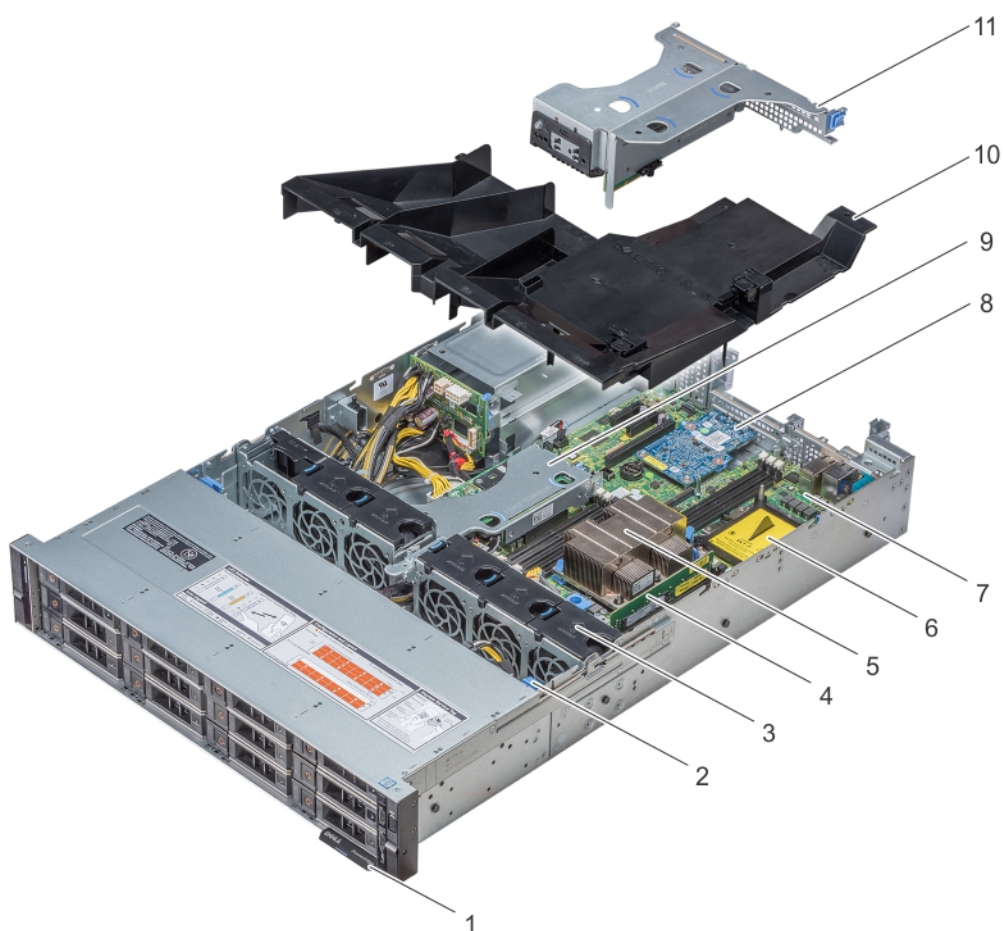
Figure 28. Intérieur du système sans bâti des lecteurs arrière
