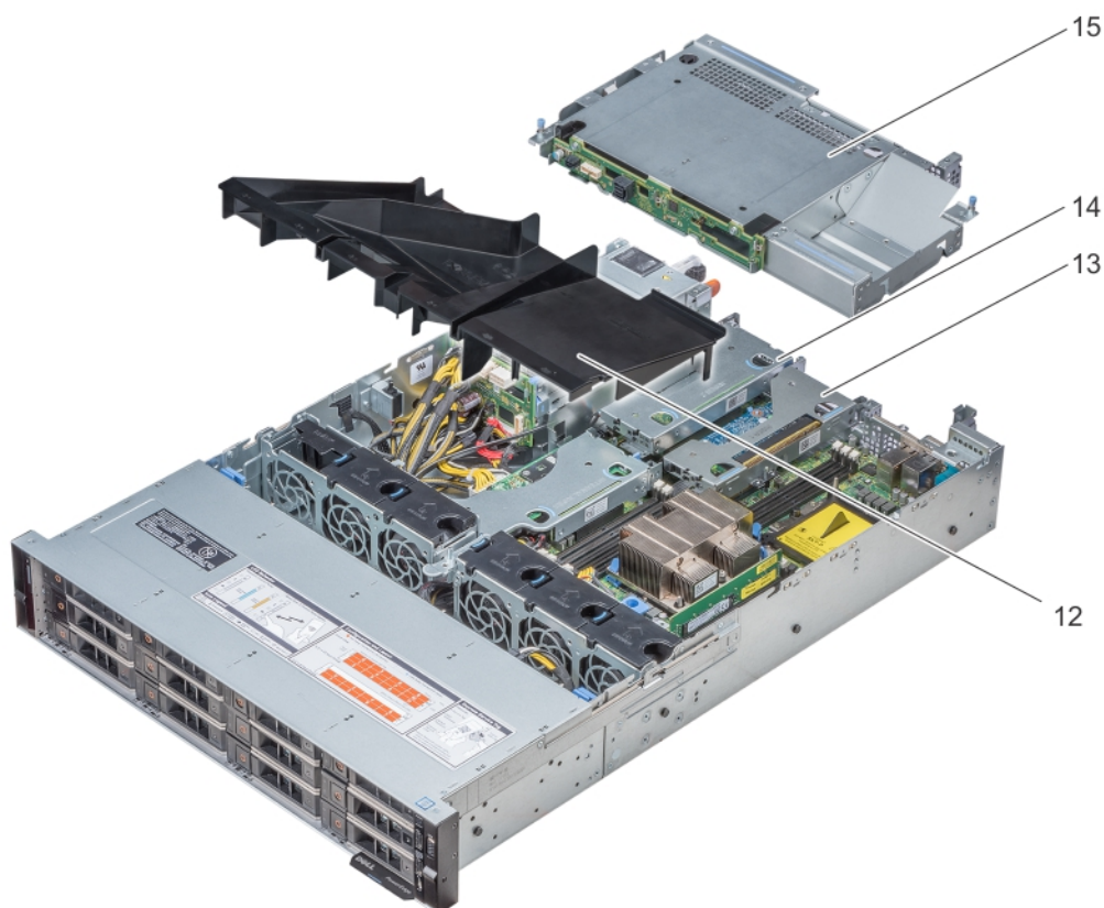
Figure 29. Intérieur du système avec bâti des lecteurs arrière
