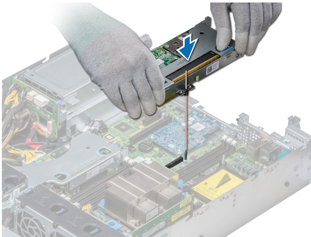
Figure 84. Installation de la carte de montage mi-hauteur droite
