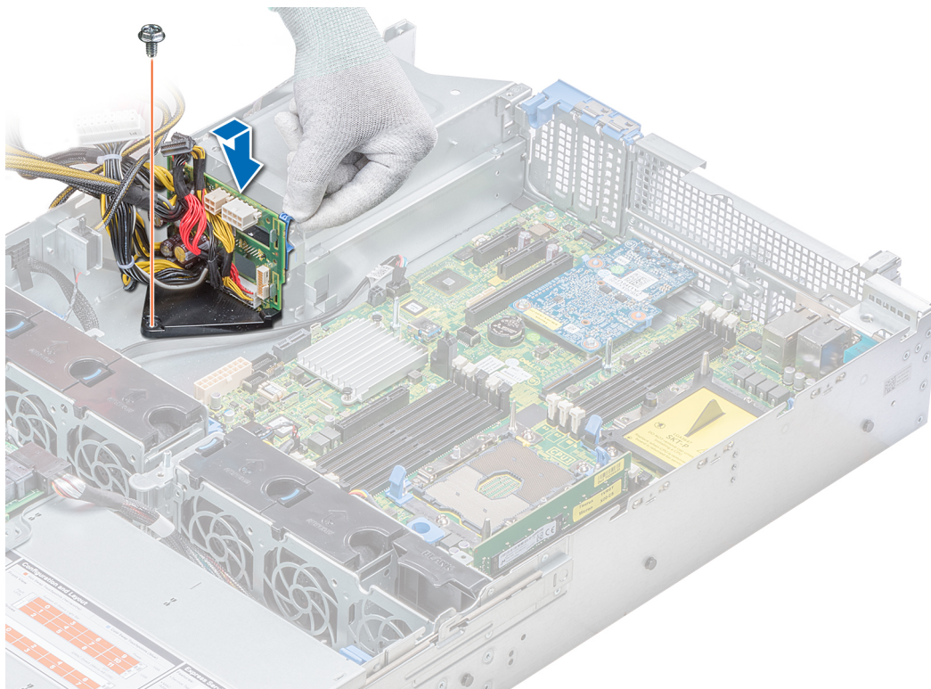
Figure 122. Installation de la carte intercalaire d'alimentation
