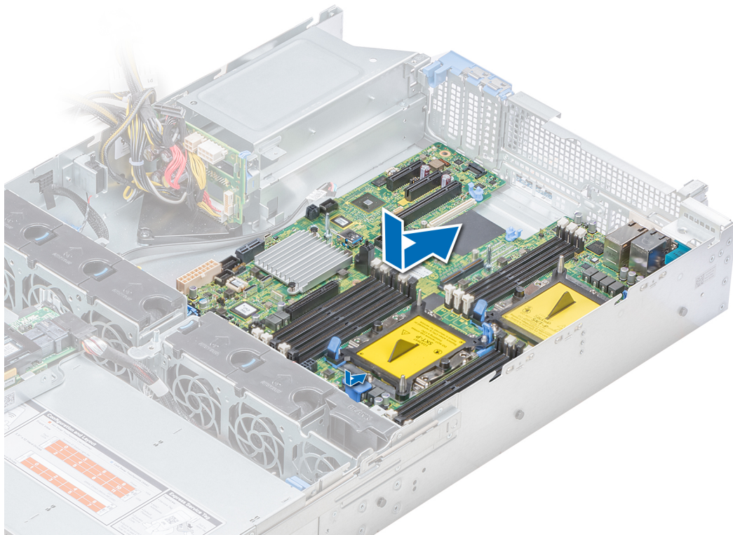
Figure 129. Installation de la carte système
