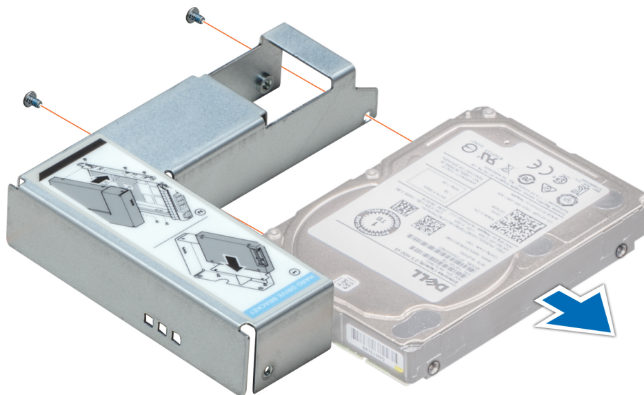
Figure 46. Retrait d'un disque de 2,5 pouces d'un adaptateur de disque de 3,5 pouces
