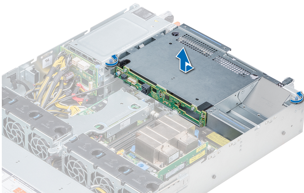
Figure 109. Retrait du bâti des disques arrière
