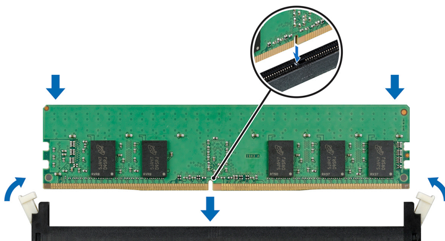
Figure 56. Installation d'une barrette de mémoire
