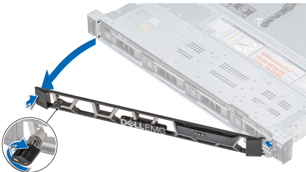
Ilustración 20. Extracción del bisel frontal opcional con el panel LCD
