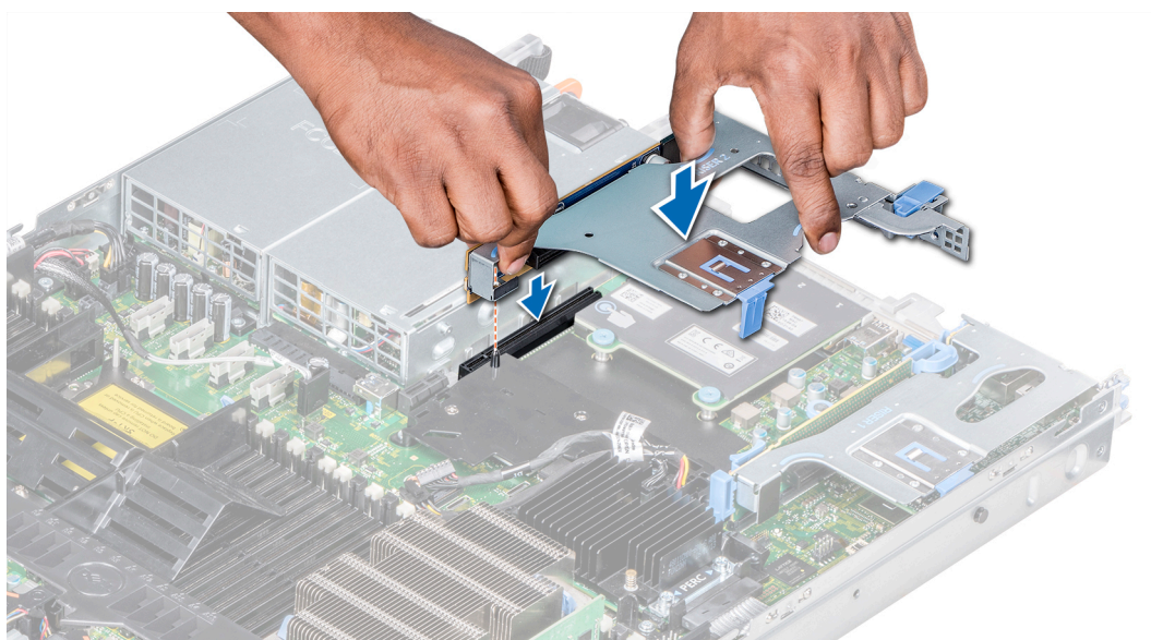
Ilustración 58. Instalación del soporte vertical de expansión 2B
