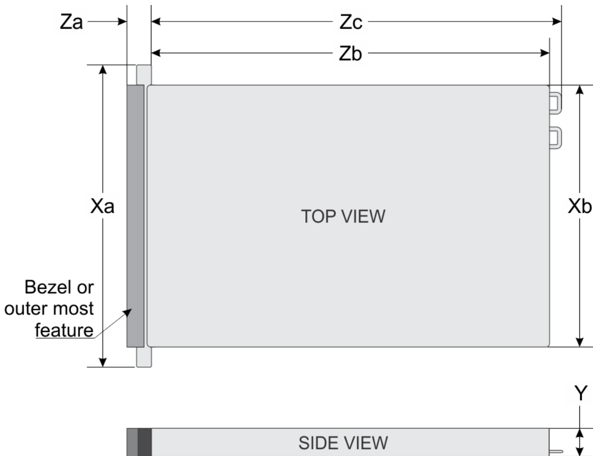
Ilustración 19. Dimensiones del sistema
