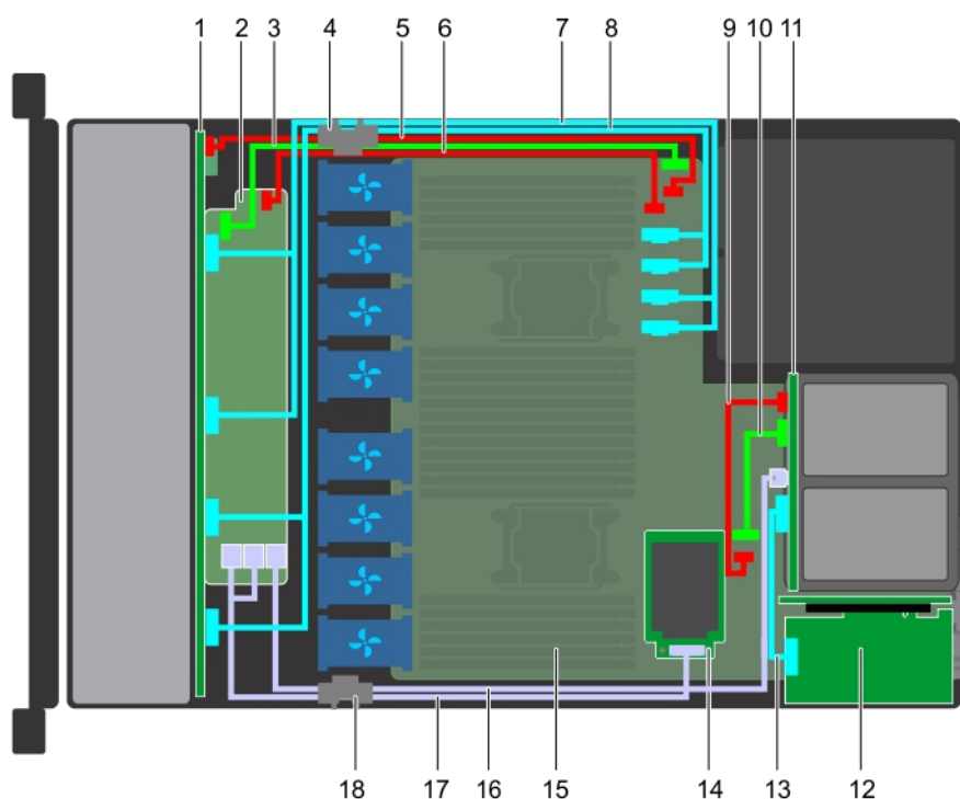
Ilustración 88. Colocación de cables: backplane de unidad de 10 x 2.5 pulgadas y backplane de unidad posterior de 2 x 2.5 pulgadas con miniPERC
