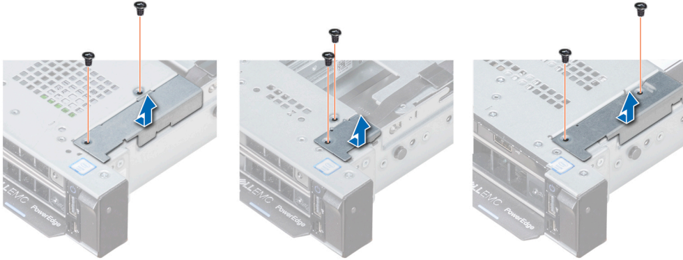
Ilustración 117. Extracción de la cubierta de cables
