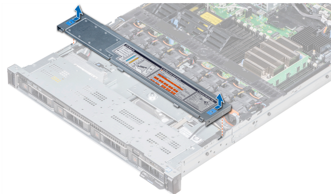
Ilustración 30. Extracción de la cubierta del plano posterior
