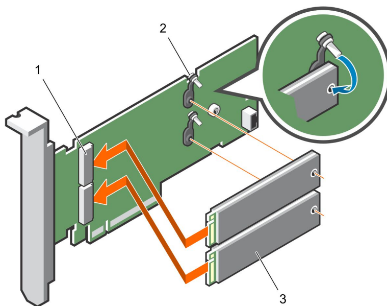
Ilustración 69. Instalación del módulo M.2 SSD
