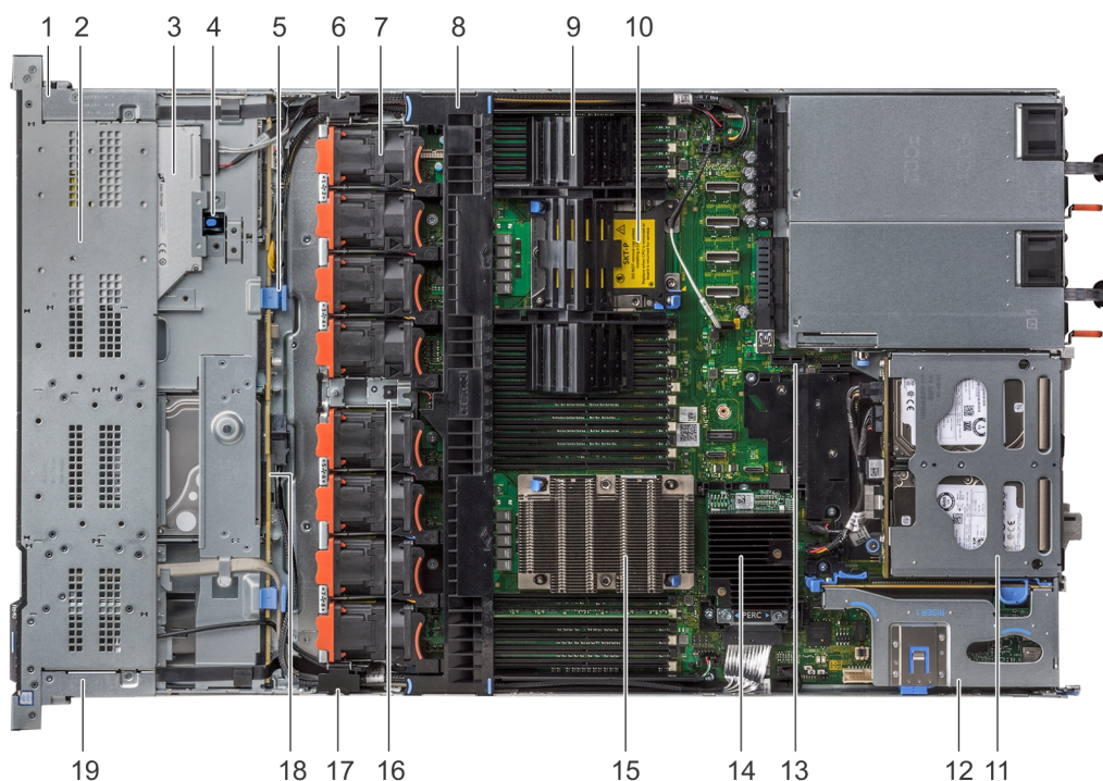
Ilustración 32. Interior del sistema: 1 soporte vertical para tarjetas de expansión PCIe
