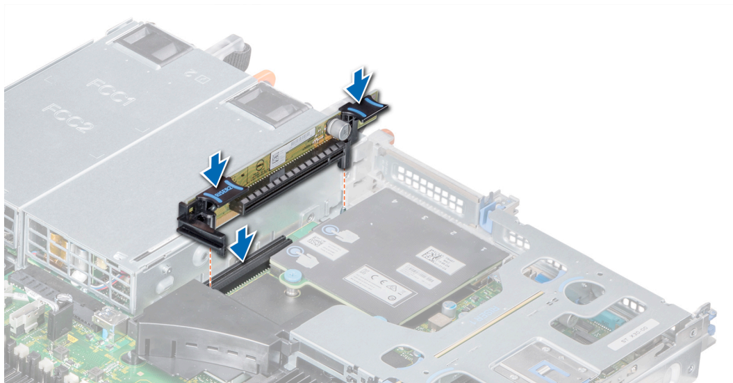
Ilustración 57. Instalación del soporte vertical de expansión 2A
