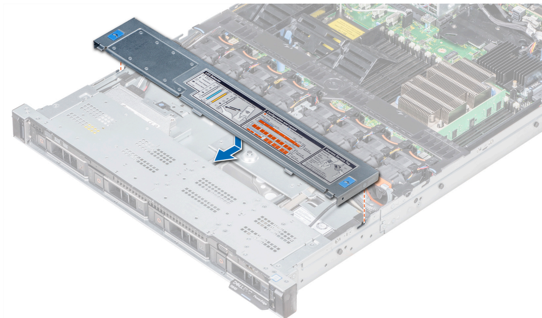
Ilustración 31. Instalación de la cubierta del plano posterior
