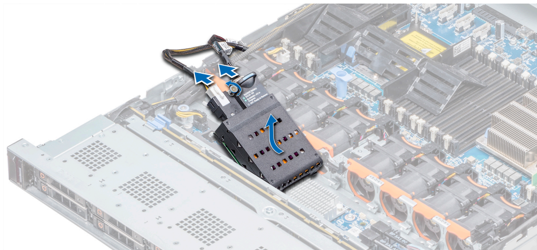
Ilustración 42. Extracción de la batería NVDIMM-N
