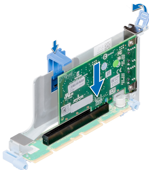
Ilustración 65. Instalación de una tarjeta de expansión en el soporte vertical para tarjetas de expansión 1B
