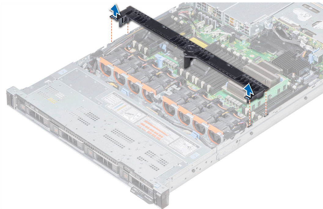
Ilustración 35. Extracción de la cubierta para flujo de aire
