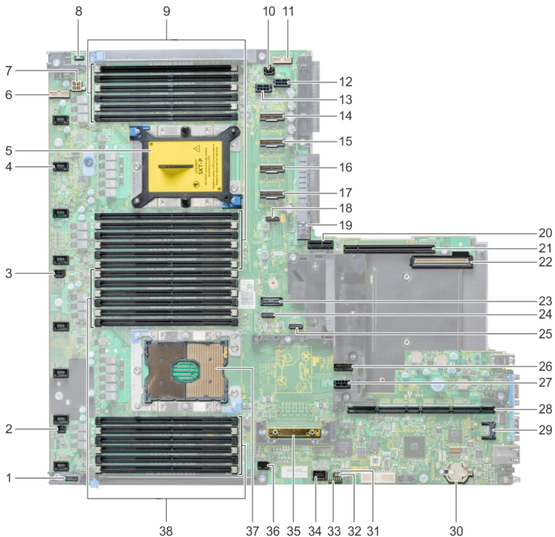
Ilustración 121. Puentes y conectores de la placa base
