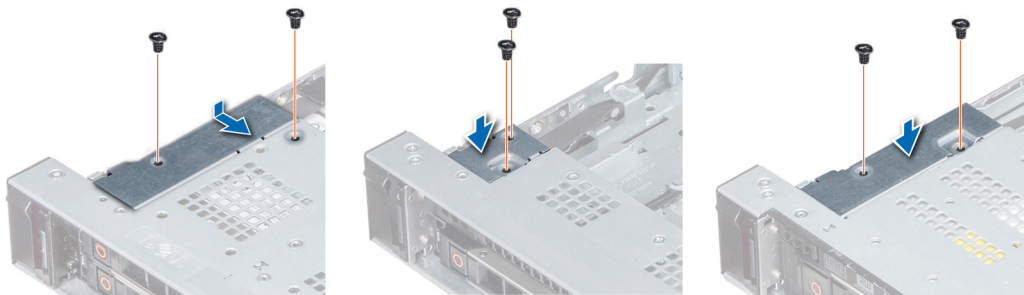
Ilustración 116. Instalación de la cubierta de cables
