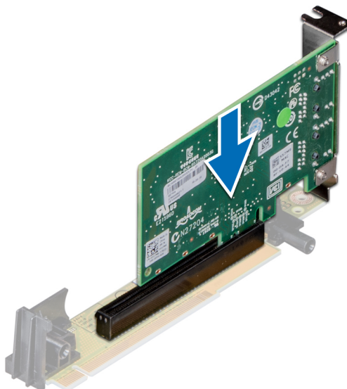
Ilustración 67. Instalación de una tarjeta de expansión en el soporte vertical para tarjetas de expansión 2A
