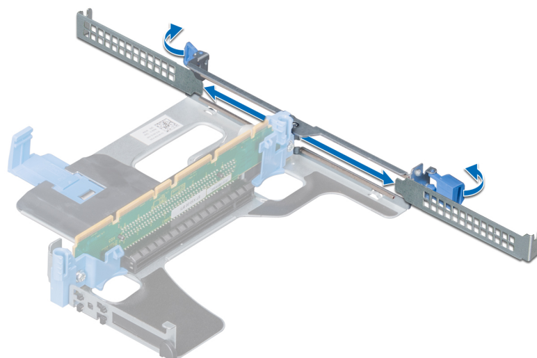
Ilustración 64. Extracción del soporte de relleno metálico del soporte vertical para tarjetas 1A
