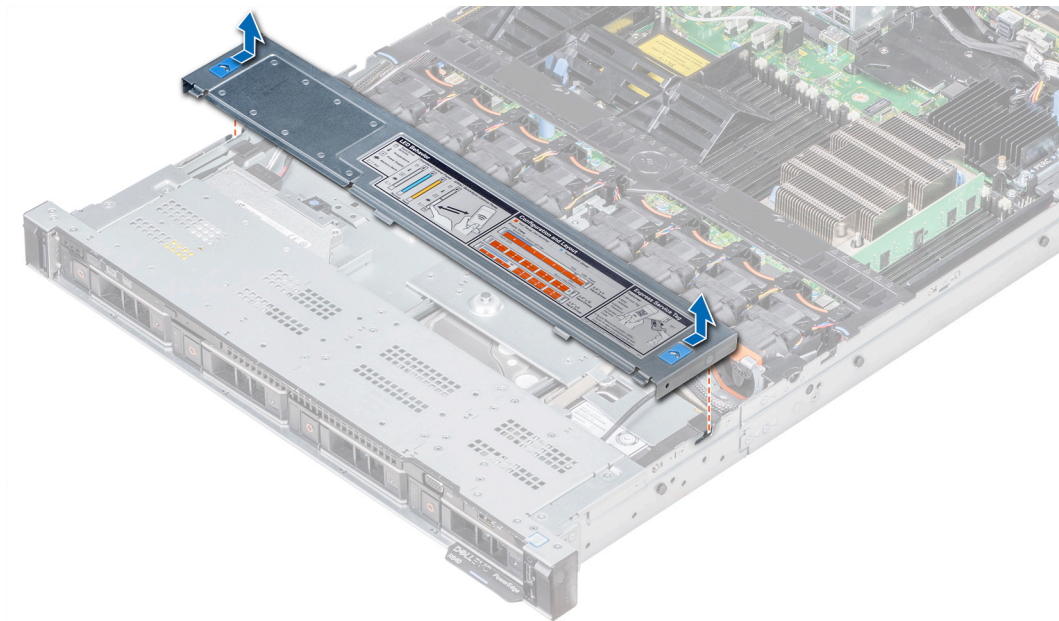
Ilustración 83. Extracción de la cubierta del plano posterior
