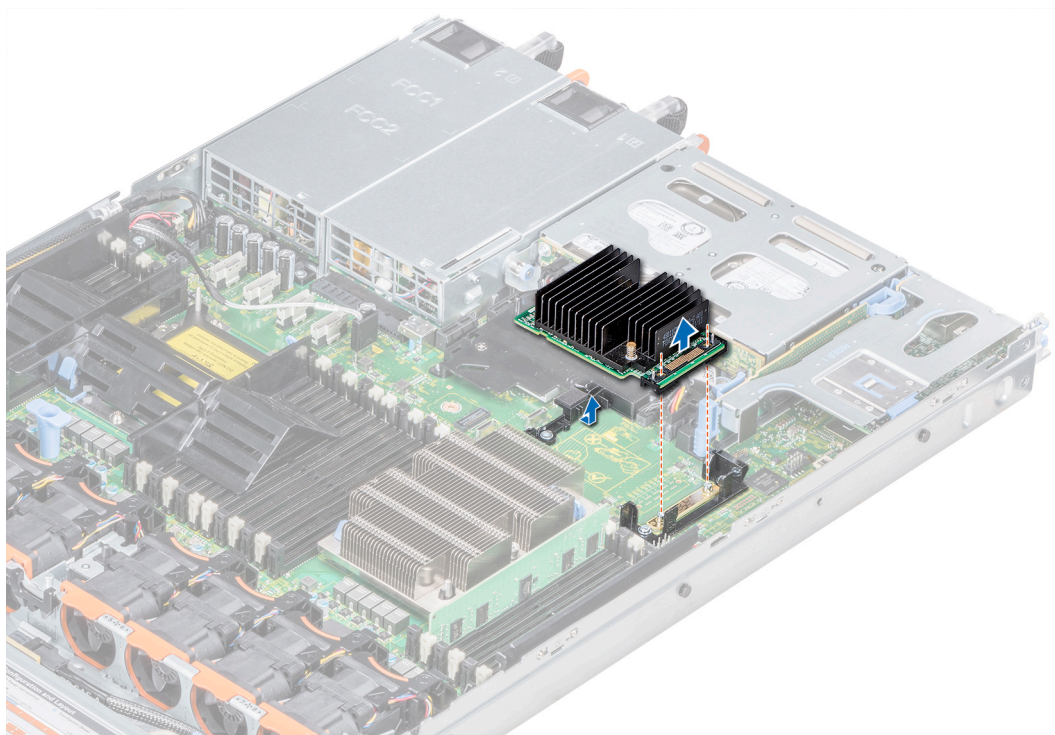
Ilustración 77. Extracción de la tarjeta controladora de almacenamiento integrada
