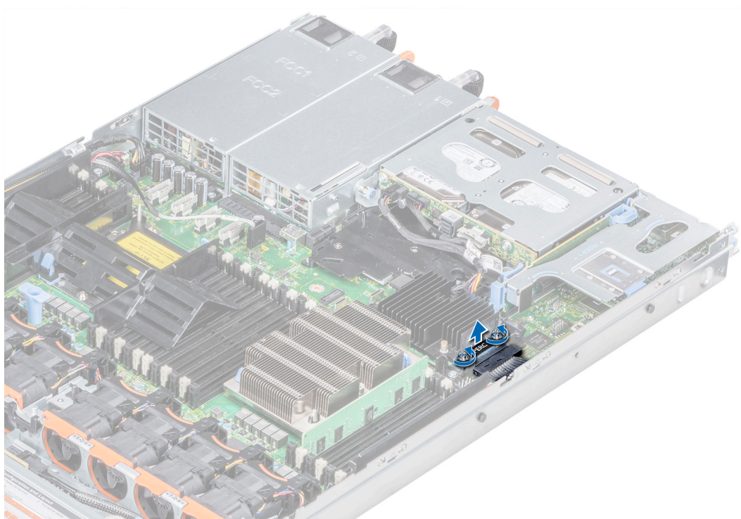
Ilustración 76. Extracción del cable de la controladora de almacenamiento integrada
