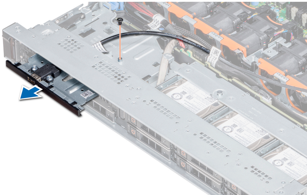
Ilustración 100. Extracción del módulo USB
