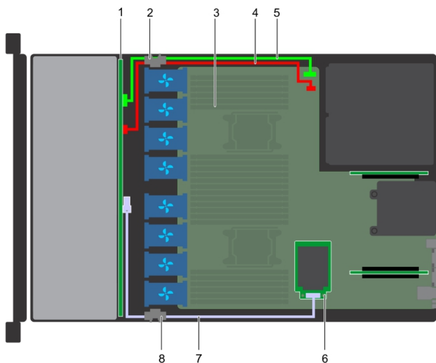
Ilustración 91. Colocación de los cables: backplane de unidad de 4 x 3.5 pulgadas con miniPERC
