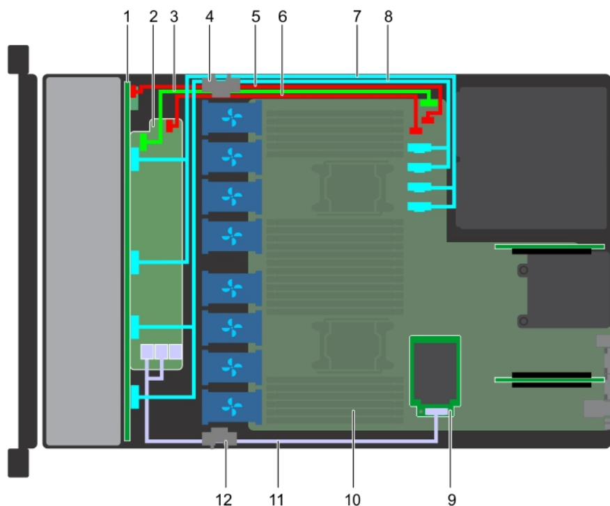
Ilustración 89. Colocación de los cables: backplane de unidad de 10 x 2.5 pulgadas con miniPERC
