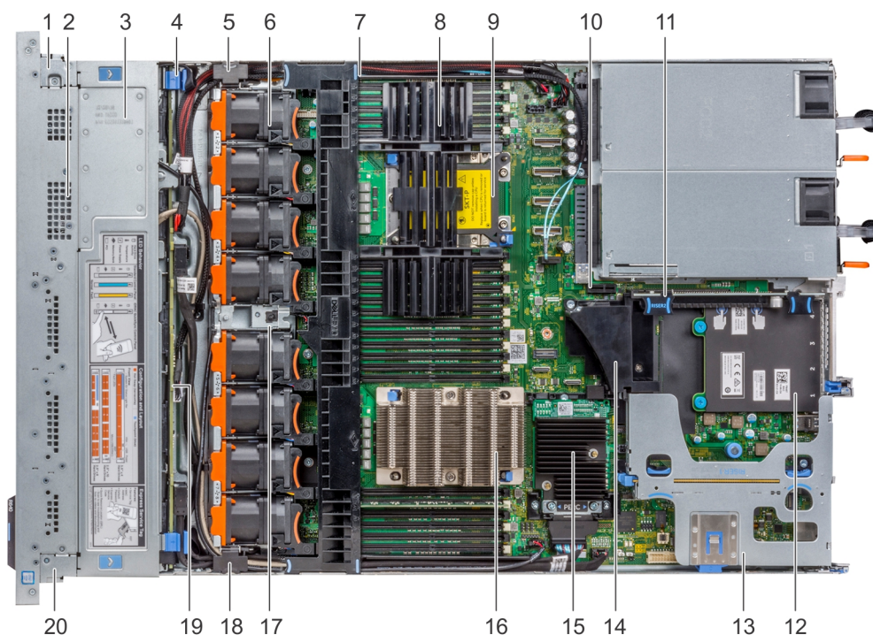
Ilustración 34. Interior del sistema: 3 soportes verticales para tarjetas de expansión PCIe
