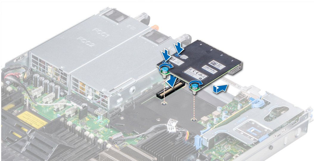
Ilustración 75. Instalación de la tarjeta secundaria de red
