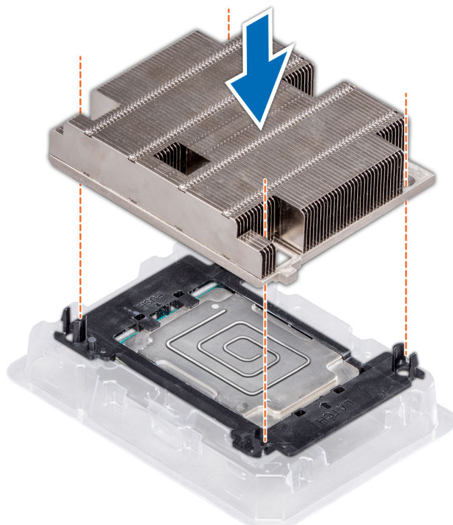
Ilustración 49. Instalación del disipador de calor en el procesador.
