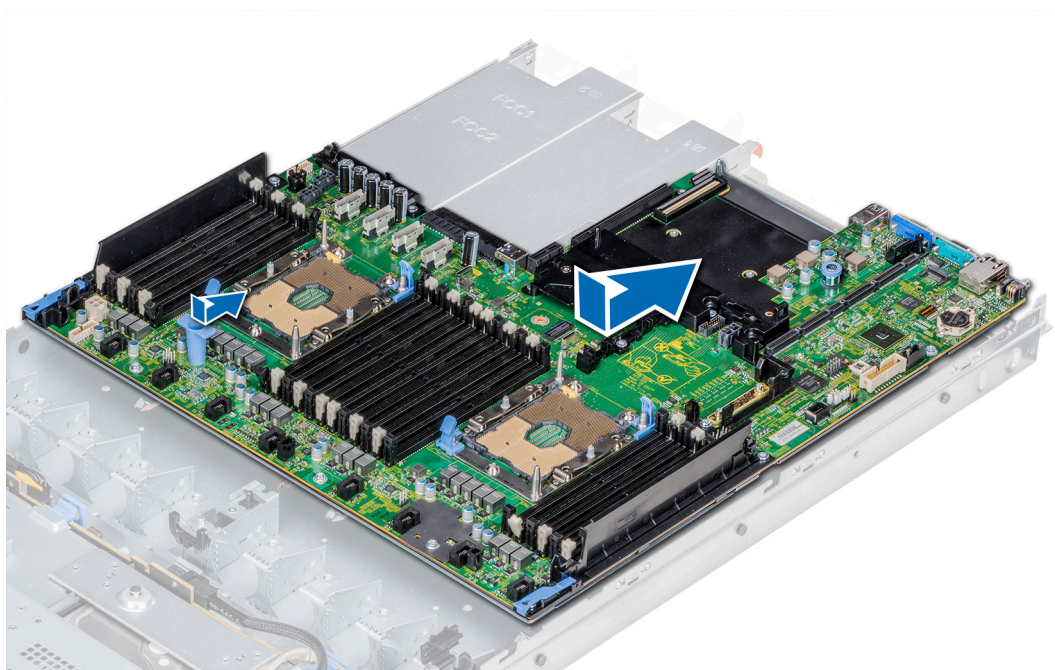
Ilustración 111. Instalación de la placa base
