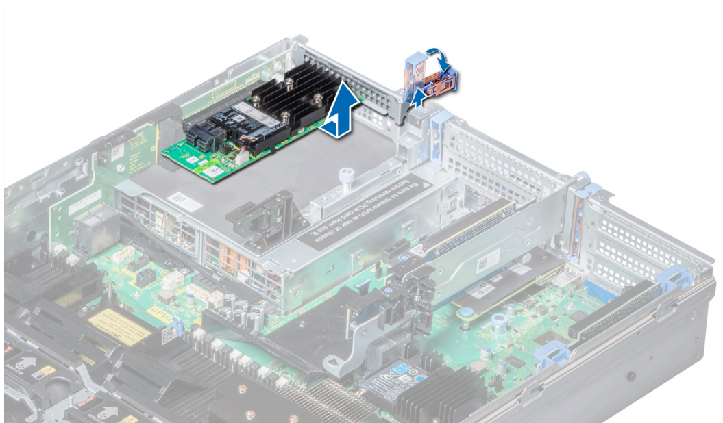
Ilustración 62. Extracción de una tarjeta de expansión del soporte vertical para tarjetas de expansión 3
