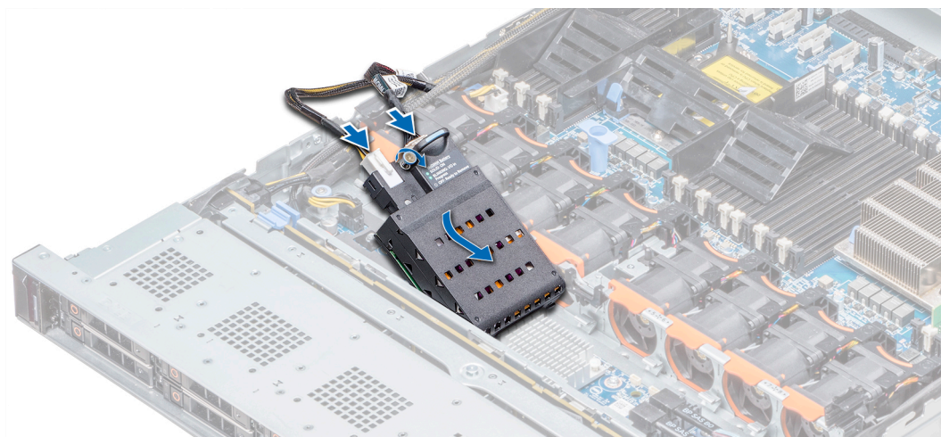
Ilustración 43. Instalación de la batería NVDIMM-N
