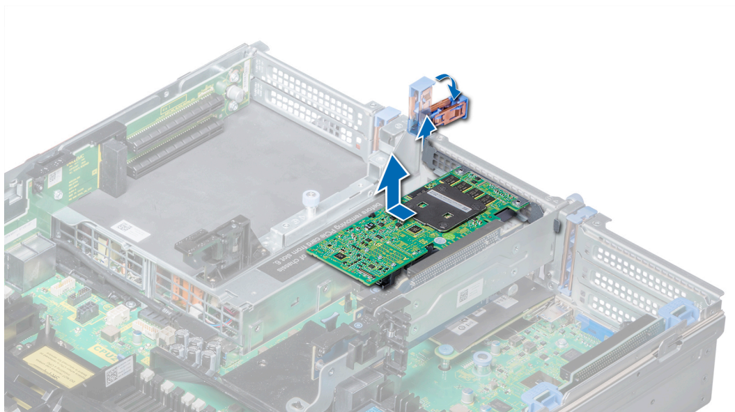
Ilustración 61. Extracción de una tarjeta de expansión del soporte vertical para tarjetas de expansión 2
