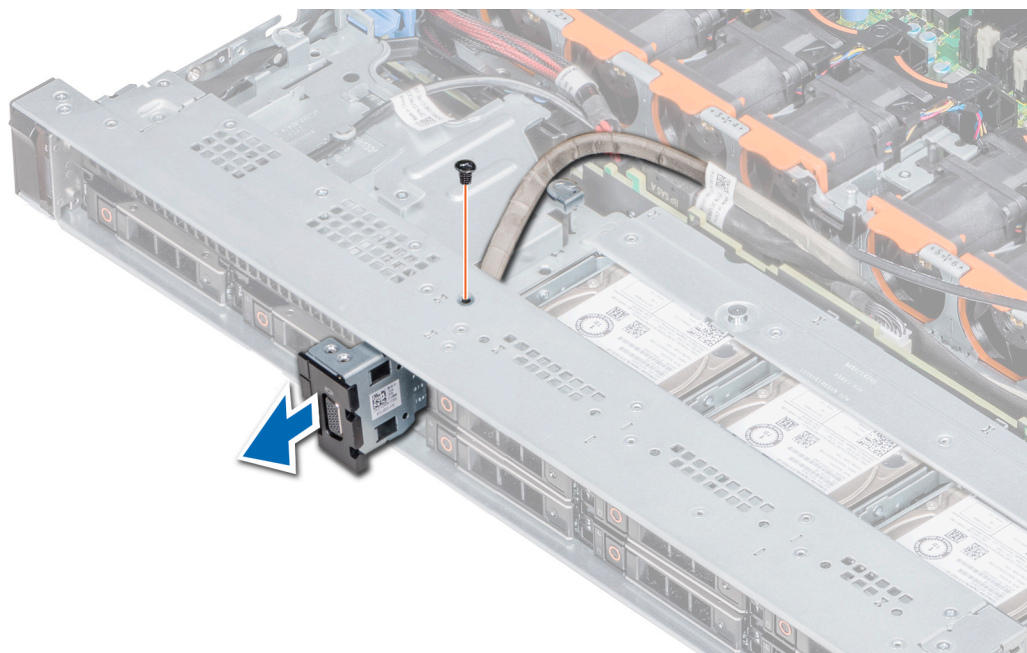
Ilustración 102. Extracción del módulo VGA
