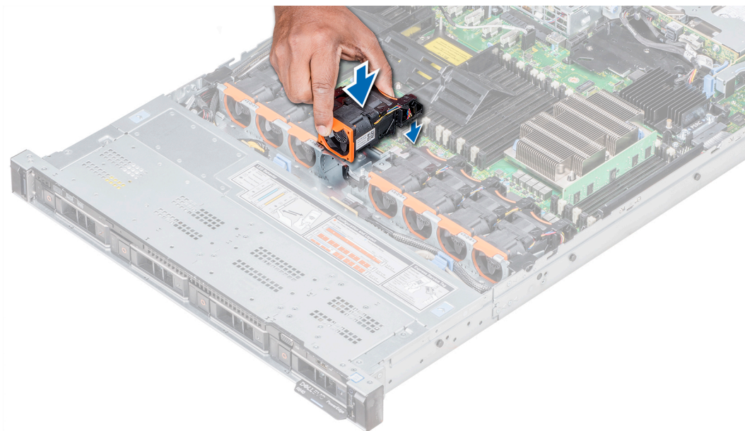
Ilustración 38. Instalación del ventilador de refrigeración
