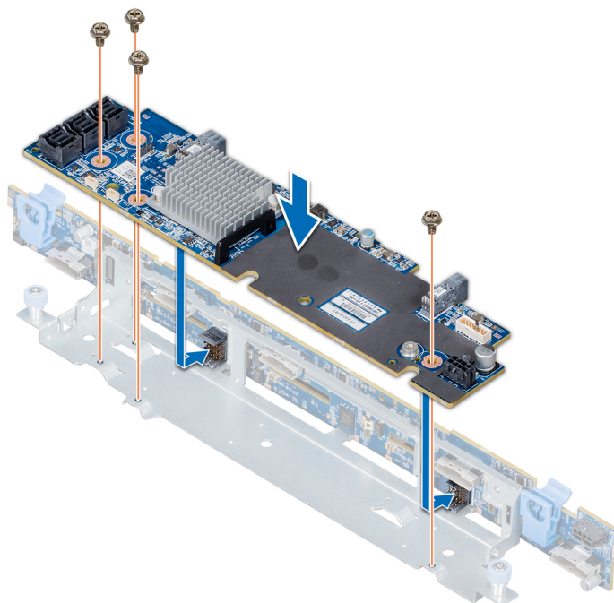
Ilustración 95. Instalación de la tarjeta expansora SAS
