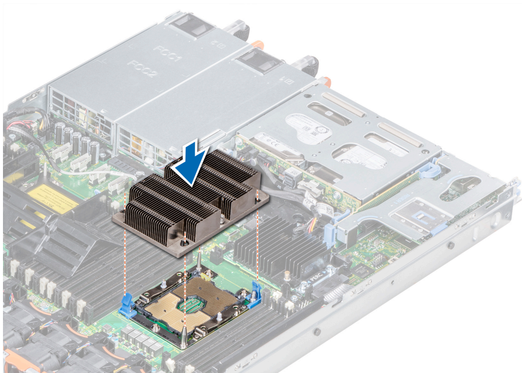
Ilustración 50. Instalación del módulo del disipador de calor y el procesador
