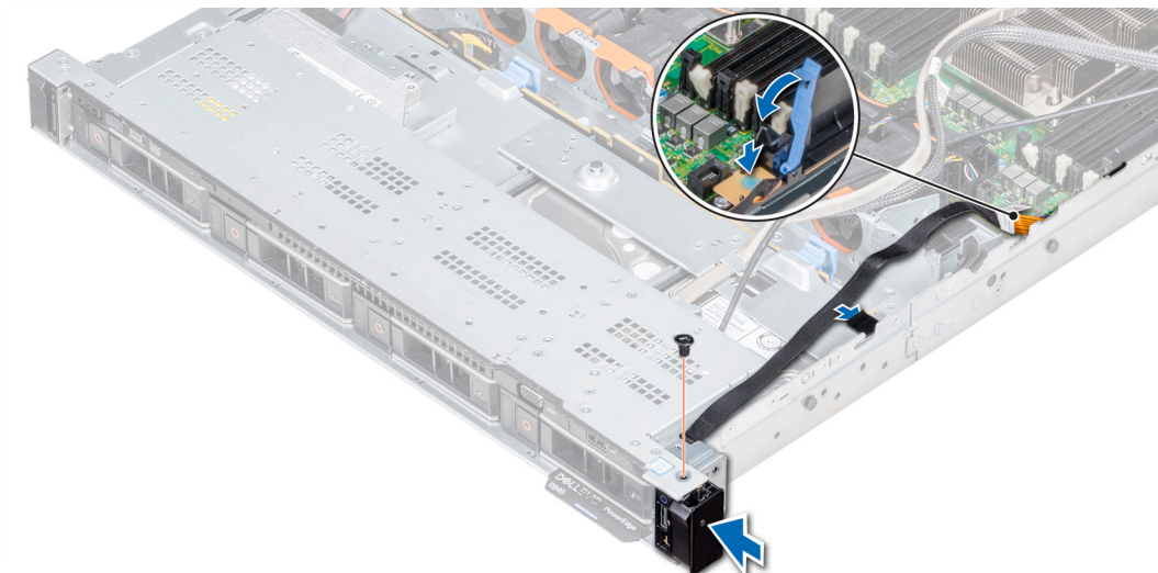
Ilustración 119. Instalación del panel de control derecho
