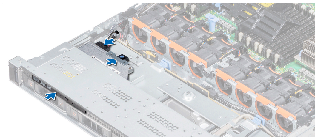
Ilustración 105. Instalación de la unidad óptica
