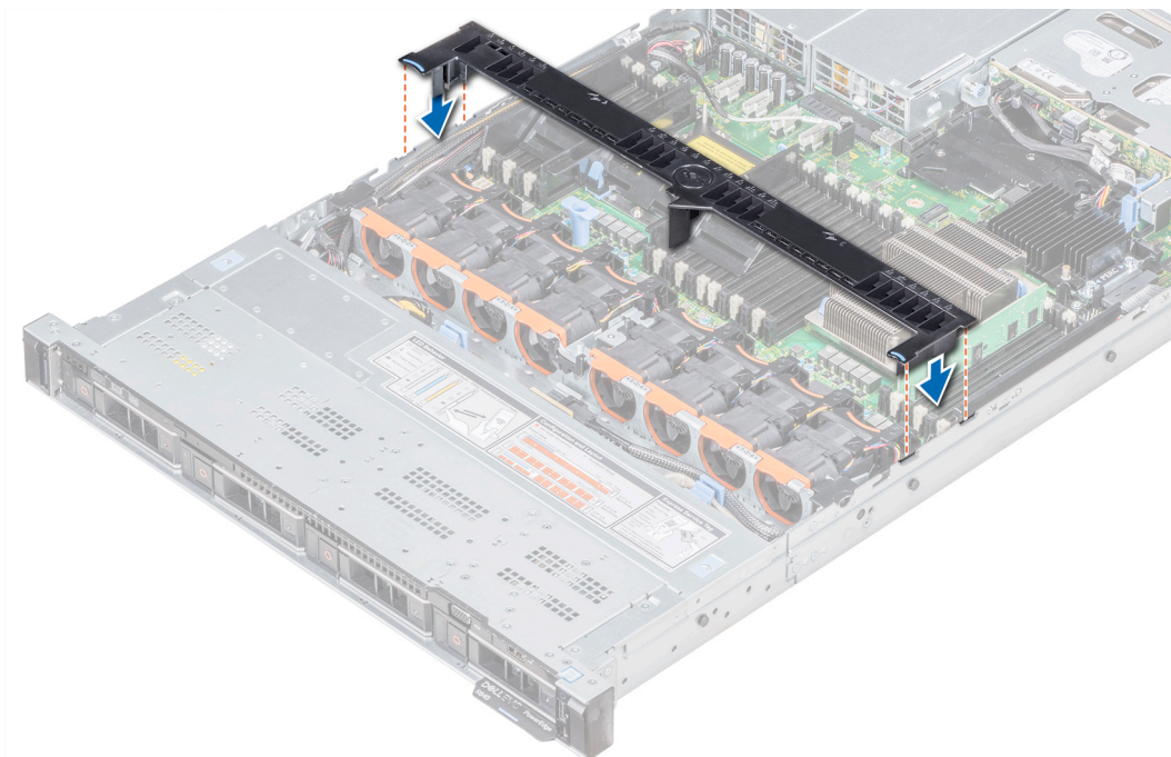
Ilustración 36. Instalación de la cubierta para flujo de aire
