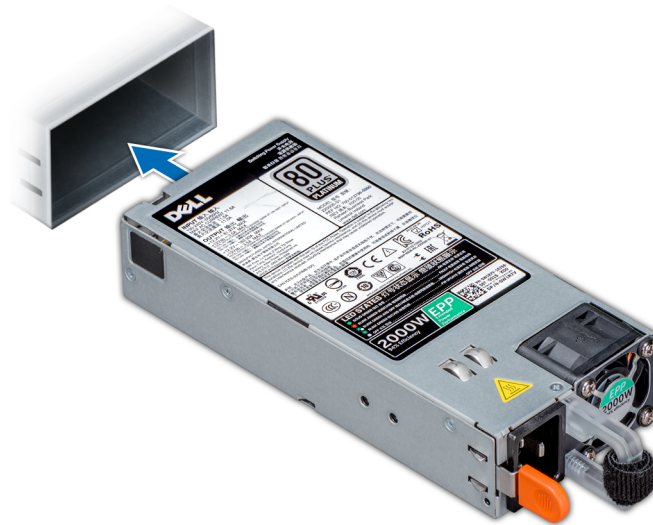
Ilustración 109. Instalación de una unidad de fuente de alimentación
