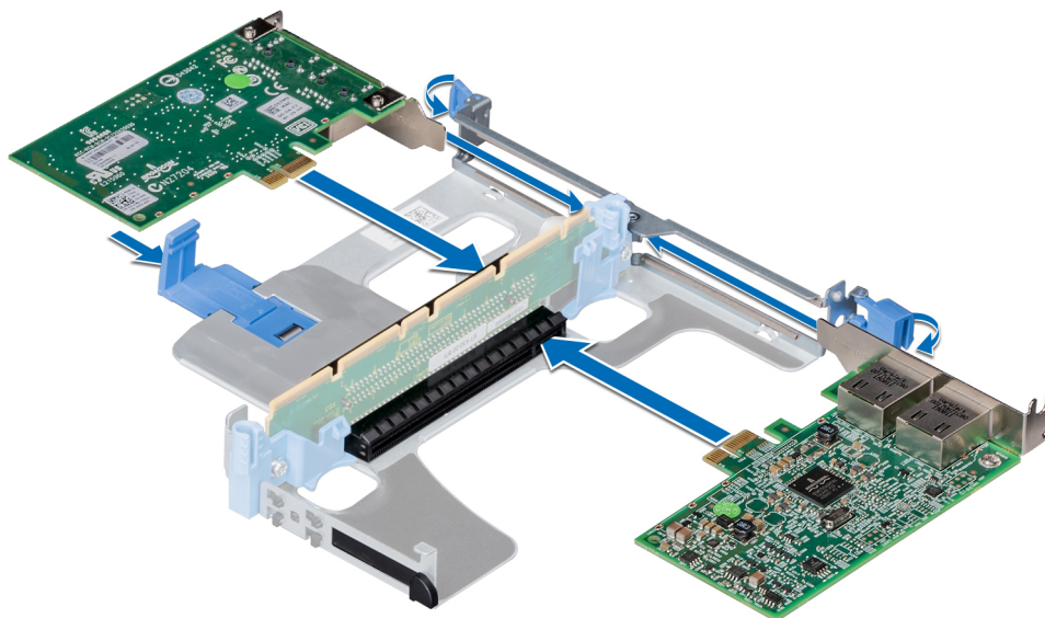
Ilustración 66. Instalación de tarjetas de expansión en el soporte vertical para tarjetas de expansión 1A
