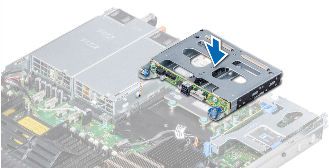
Ilustración 97. Instalación de la caja para unidades de disco internas
