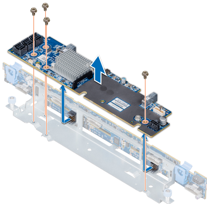
Ilustración 94. Extracción de la tarjeta de expansión SAS
