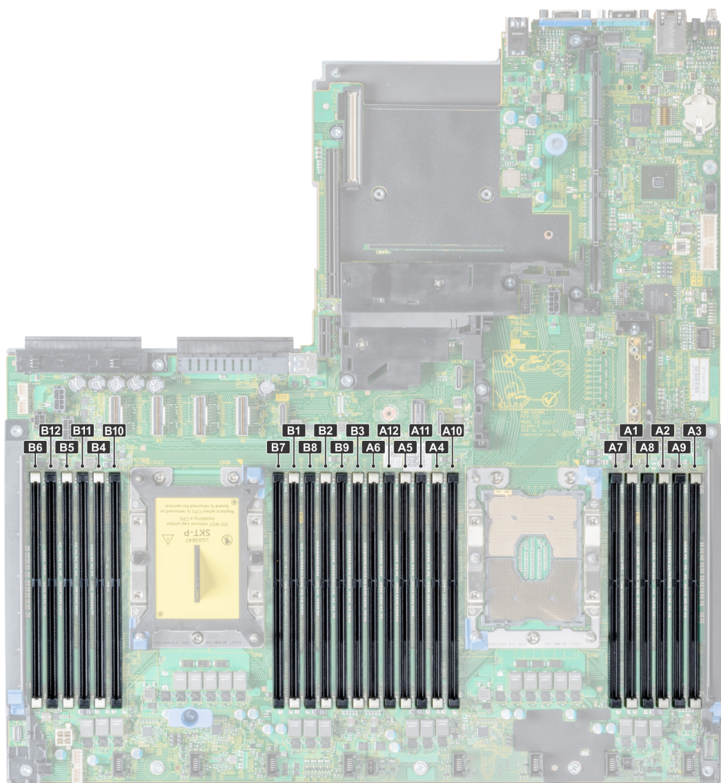
Ilustración 39. Vista de la memoria del sistema
