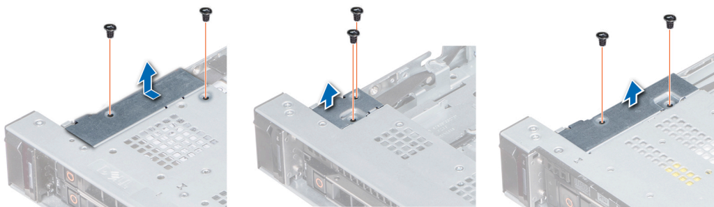
Ilustración 113. Extracción de la cubierta de cables
