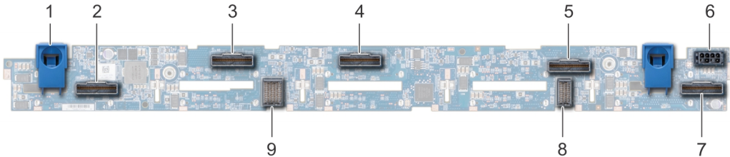
Ilustración 82. Backplane de unidad de 10 x 2,5 pulgadas
