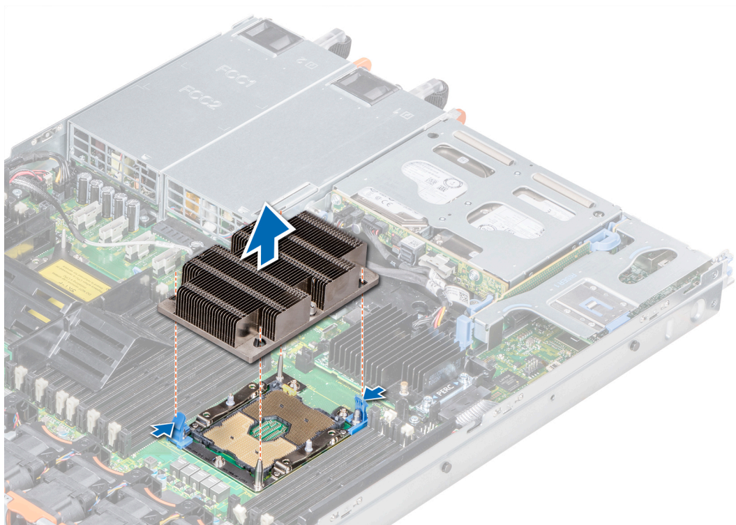
Ilustración 44. Extracción del módulo del procesador y el dissipador de calor
