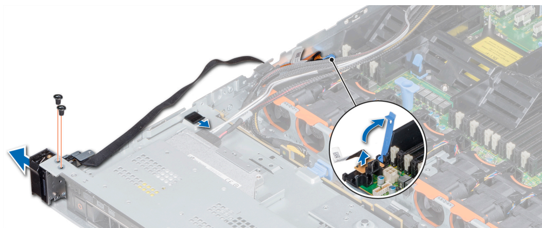
Ilustración 114. Extracción del panel de control izquierdo
