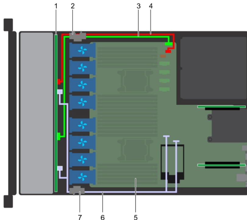
Ilustración 93. Colocación de los cables: backplane de unidad de 8 x 2.5 pulgadas con SATA integrada
