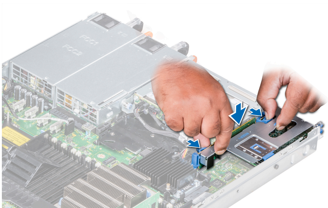
Ilustración 56. Instalación del soporte vertical de expansión 1B
