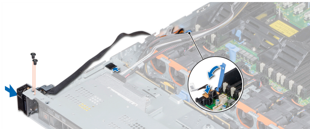
Ilustración 115. Instalación del panel de control izquierdo
