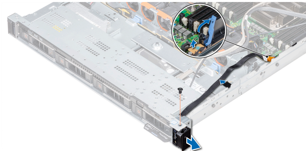
Ilustración 118. Desmontaje del panel de control derecho
