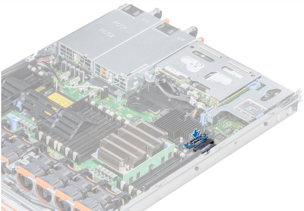
Ilustración 79. Instalación del cable de la tarjeta controladora de almacenamiento integrada
