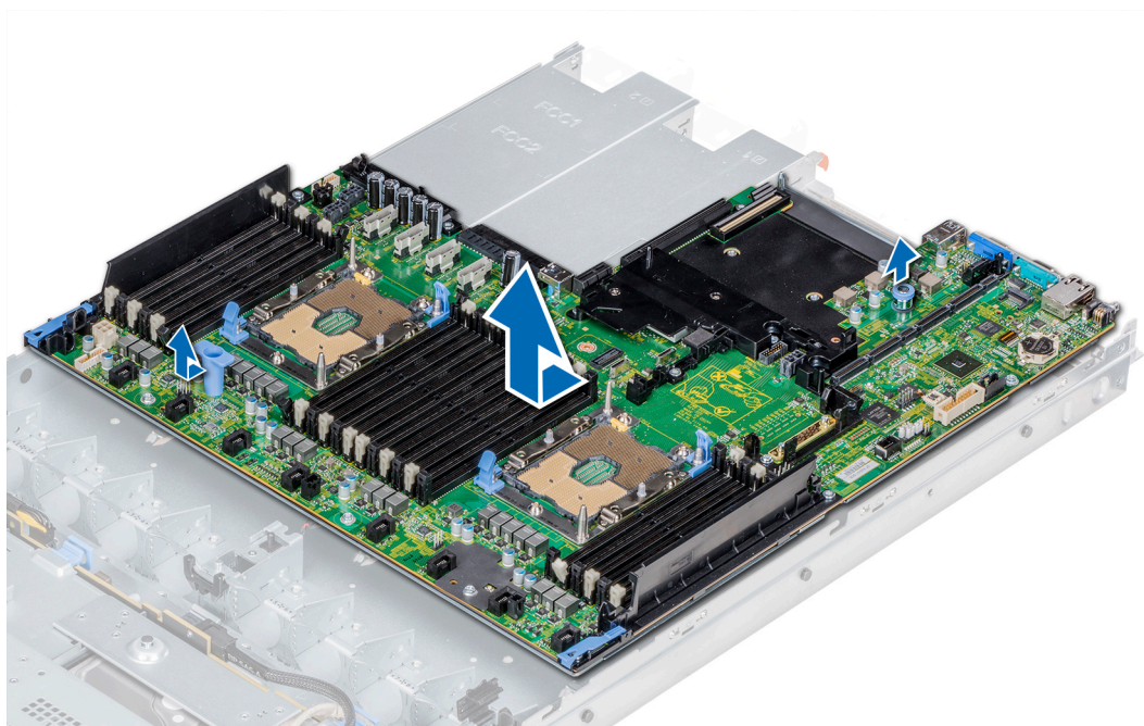
Ilustración 110. Extracción de la placa base
