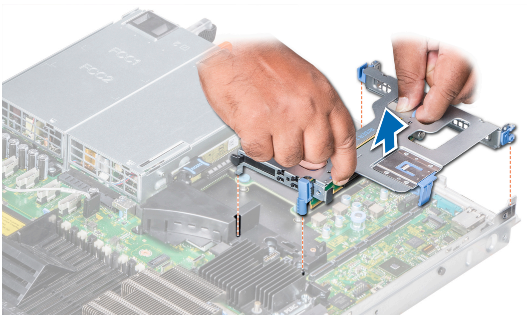
Ilustración 52. Extracción del soporte vertical para tarjetas de expansión 1A
