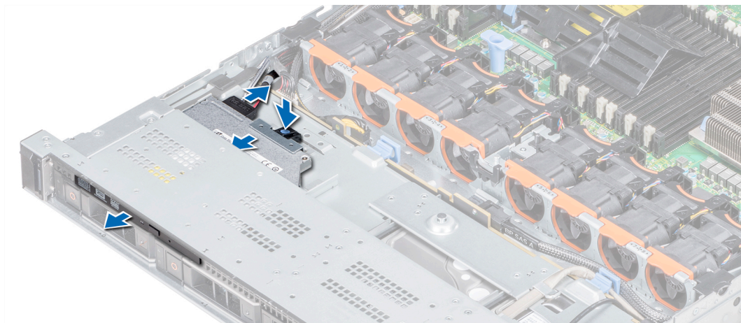
Ilustración 104. Extracción de la unidad óptica
