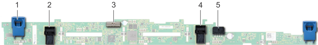
Ilustración 81. Backplane de unidad de 8 x 2,5 pulgadas
