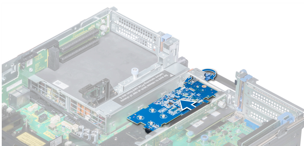
Ilustración 60. Extracción de la tarjeta de expansión del soporte vertical para tarjetas de expansión 2B
