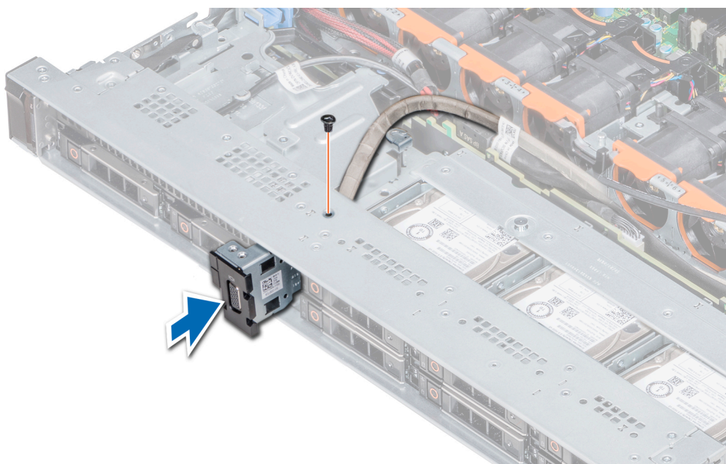
Ilustración 103. Instalación del módulo VGA
