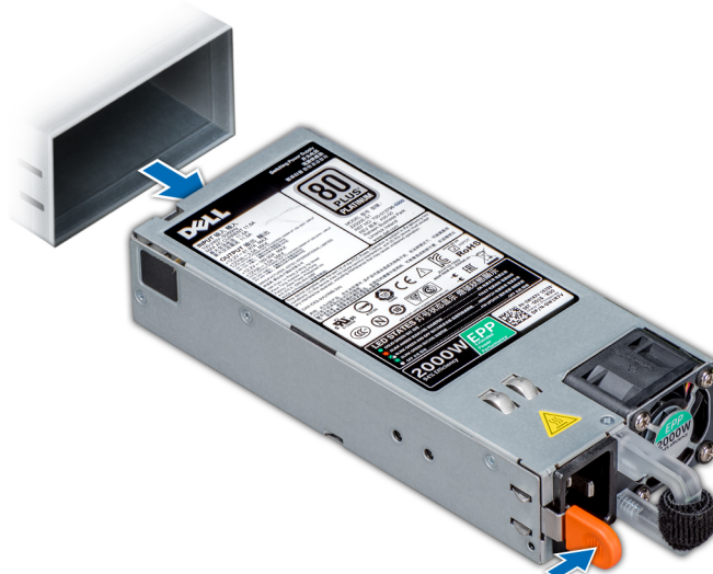
Ilustración 108. Extracción de una unidad de fuente de alimentación
