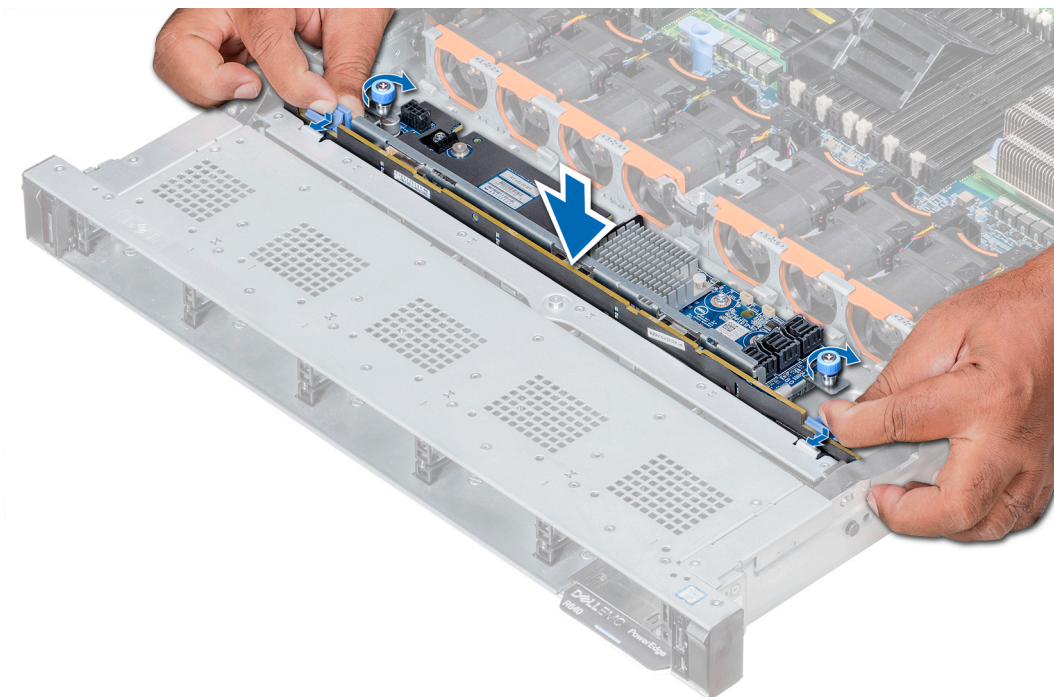
Ilustración 84. Instalación del plano posterior
