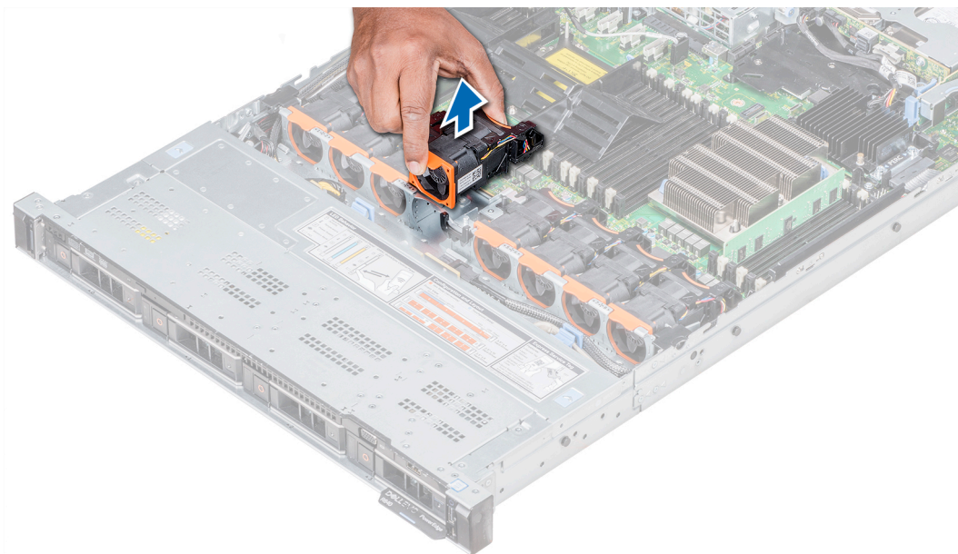
Ilustración 37. Extracción del ventilador de refrigeración
