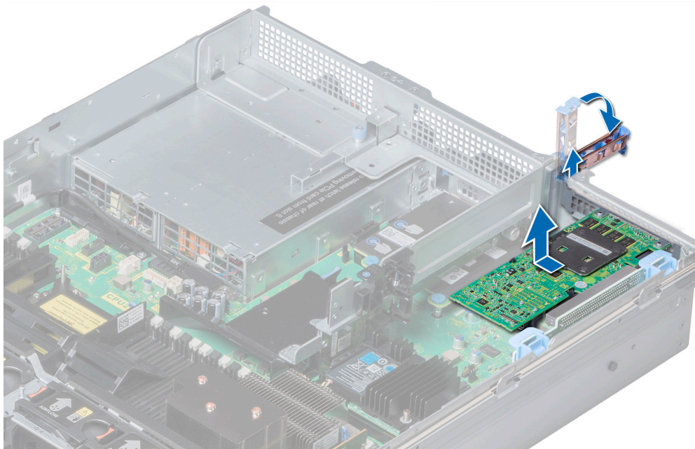
Ilustración 59. Extracción de una tarjeta de expansión del soporte vertical para tarjetas de expansión 1
