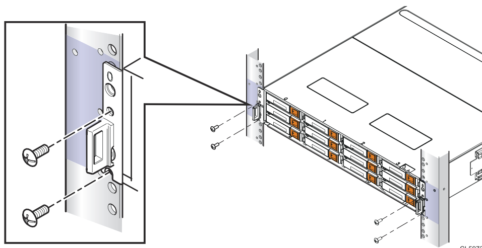
Figure 7. Fixation du boîtier à l'avant de l'armoire
