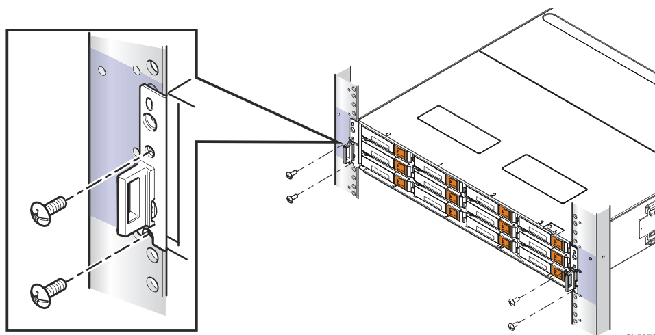
Abbildung 7. Befestigen des Gehäuses an der Schrankvorderseite
