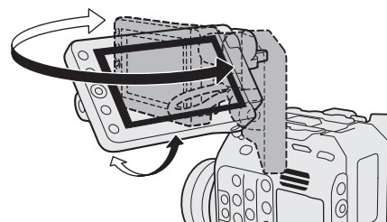
LCD-Monitor an der Kamera angebracht
