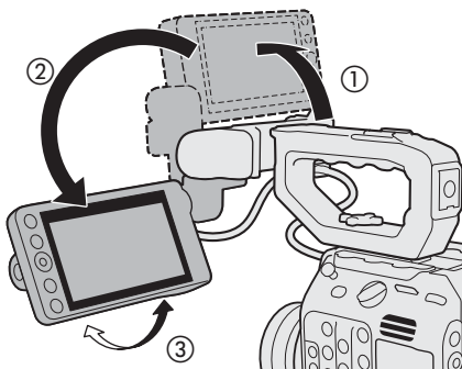
LCD-Monitor am Tragegriff angebracht
