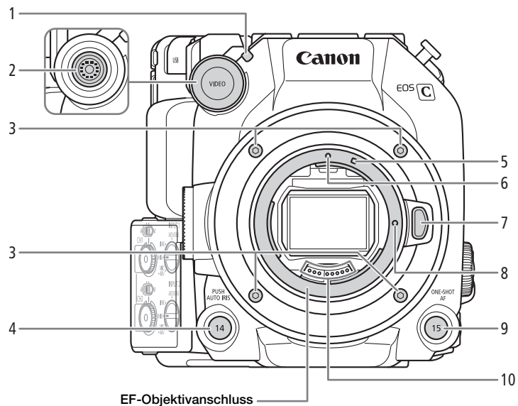
EF-Objektivanschluss
