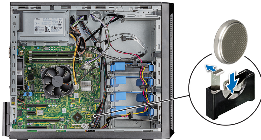
Ilustración 47. Instalación de la batería del sistema
