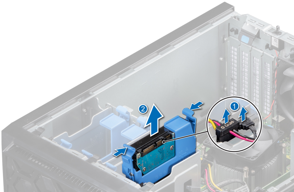
Ilustración 13. Extracción del portaunidades del compartimiento para unidad
