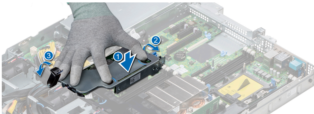
Ilustración 71. Instalación del soporte vertical para PERC interno
