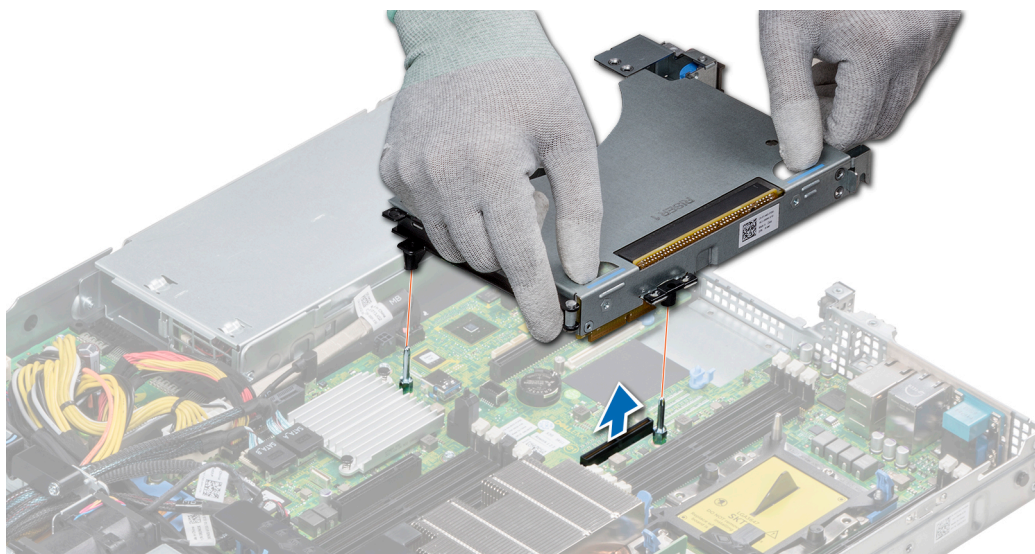
Ilustración 57. Extracción de un soporte vertical para tarjetas de expansión 1A
