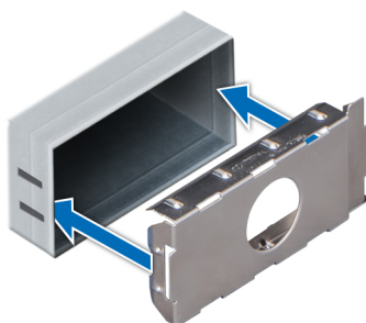
Ilustración 99. Instalación de una unidad de fuente de alimentación de relleno
