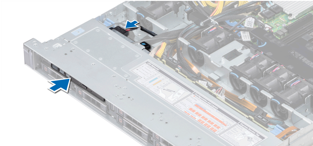
Ilustración 97. Instalación de la unidad óptica
