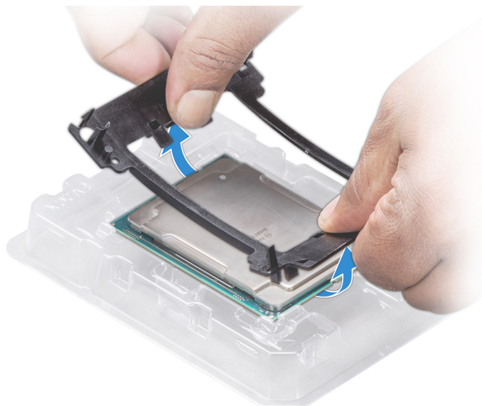
Ilustración 44. Extracción del soporte del procesador
