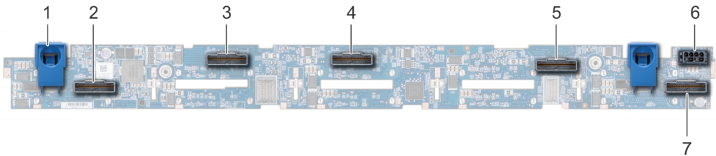
Ilustración 84. 10 backplanes de 2,5 pulgadas
