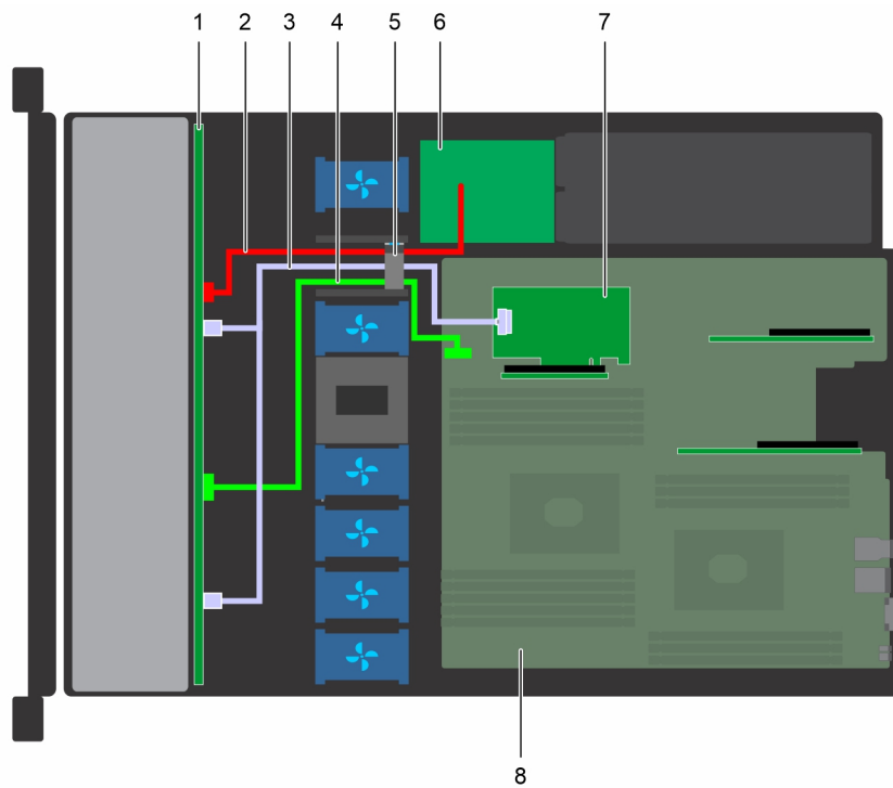
Ilustración 90. Enrutamiento de cables: backplane para 8 discos duros de 2,5 pulgadas con soporte vertical de PERC
