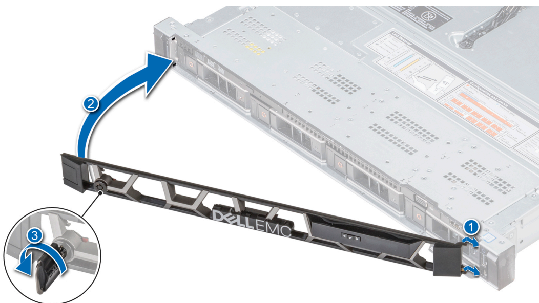
Ilustración 17. Instalación del bisel frontal con el panel LCD
