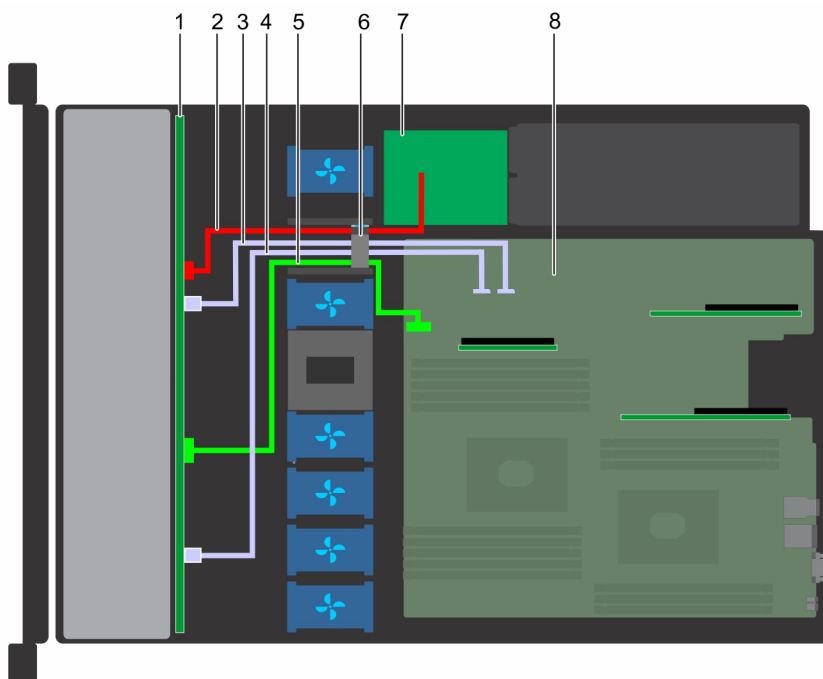
Ilustración 91. Enrutamiento de cables: backplane para 8 discos duros de 2,5 pulgadas con SATA a bordo
