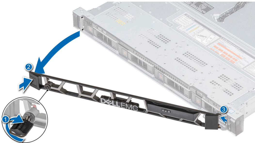
Ilustración 16. Extracción del bisel frontal con el panel LCD
