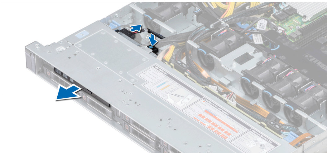
Ilustración 96. Extracción de la unidad óptica
