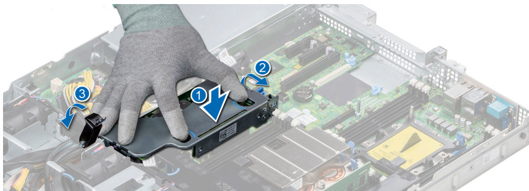
Ilustración 51. Instalación del soporte vertical para PERC interno
