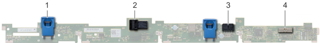
Ilustración 82. 4 backplanes de 3,5 pulgadas
