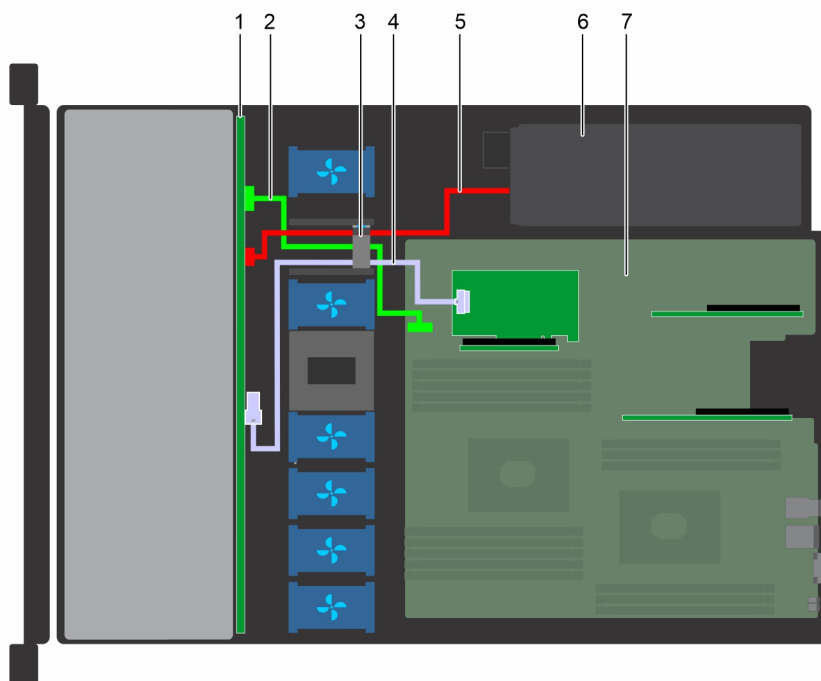
Ilustración 92. Enrutamiento de cables: backplane para 4 discos duros de 3,5 pulgadas con soporte vertical de PERC
