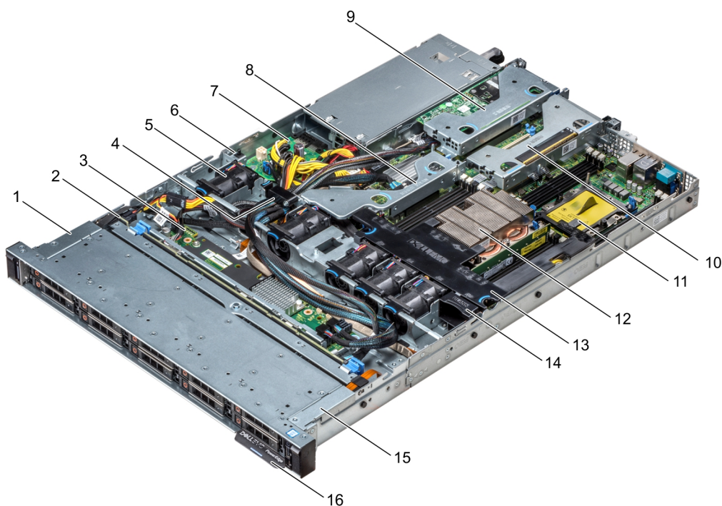
Figure 20. À l'intérieur du système
