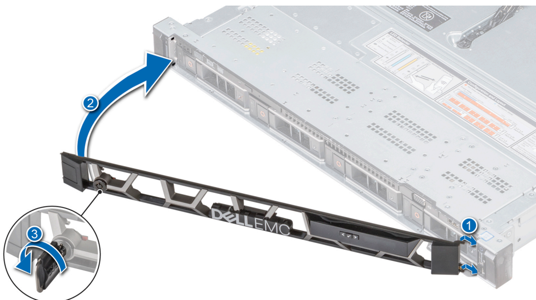
Figure 17. Installation du cadre avant avec le panneau LCD
