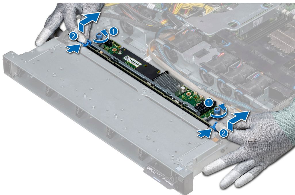
Figure 87. Retrait du fond de panier de disque dur
