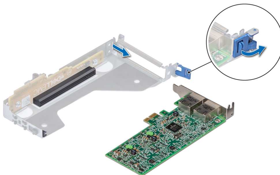
Figure 60. Retrait d'une carte d'extension sur la carte de montage 2
