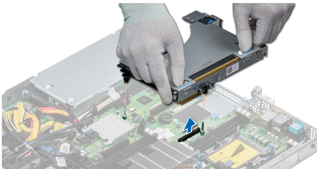
Figure 57. Retrait d'une carte de montage pour carte d'extension 1A
