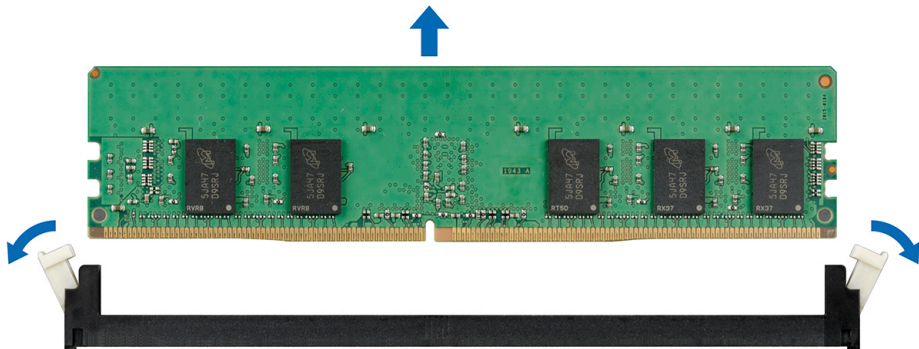
Figure 40. Retrait d’une barrette de mémoire
