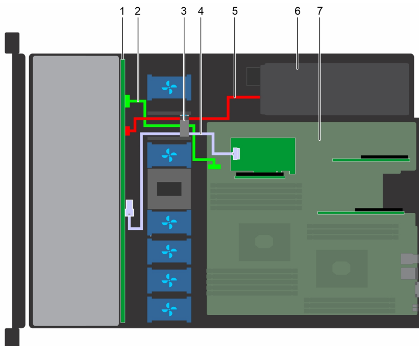
Figure 92. Acheminement des câbles : fond de panier de 4 disques durs de 3,5 pouces avec carte de montage PERC
