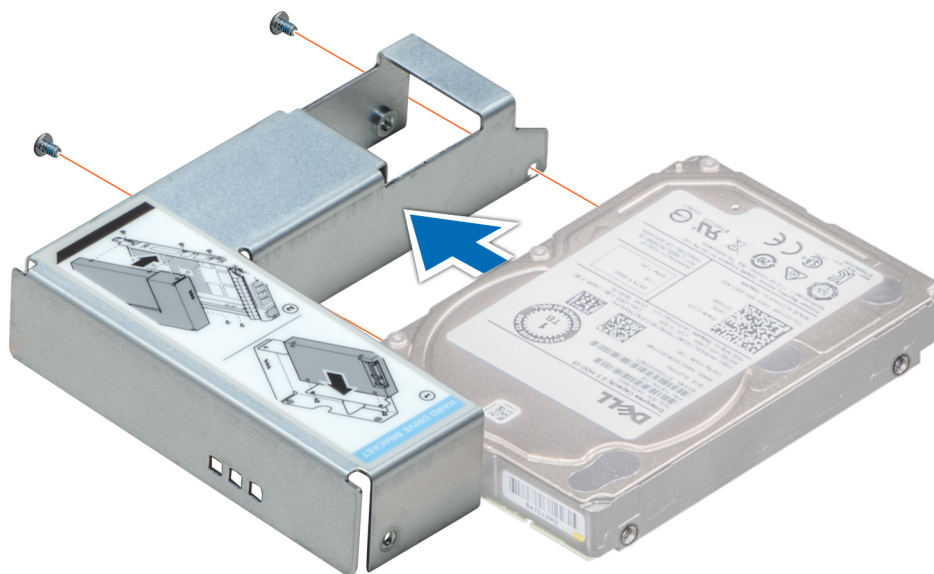
Figure 32. Installation d'un disque de 2,5 pouces dans un adaptateur de disque de 3,5 pouces
