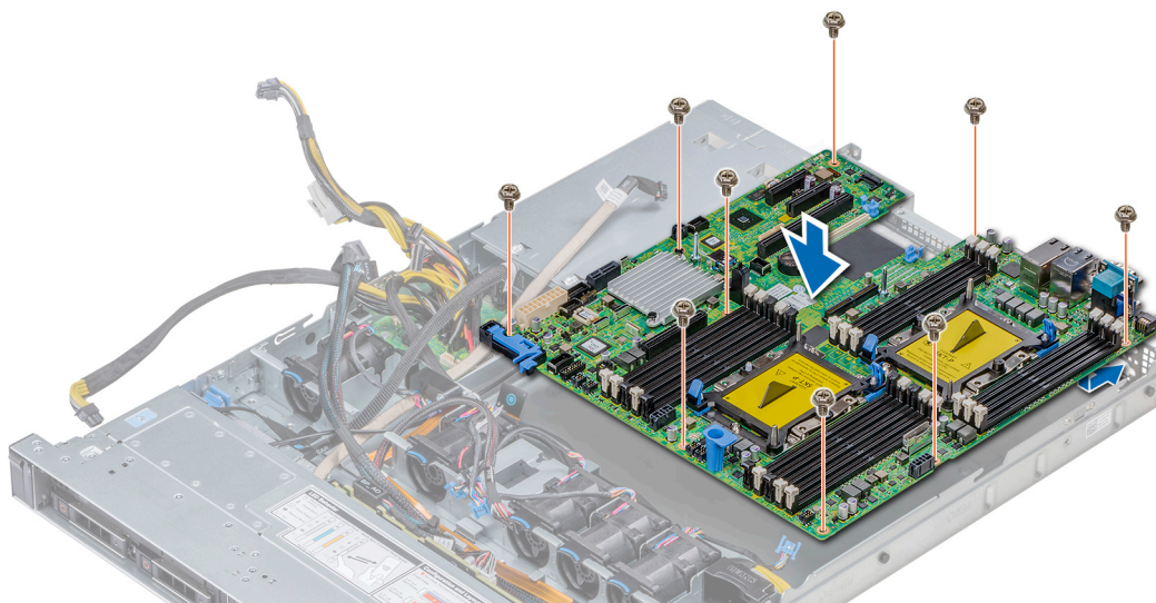
Figure 113. Installation de la carte système
