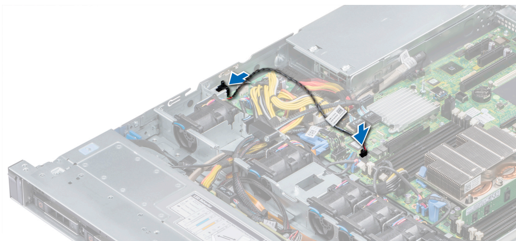
Figure 28. Installation d'un commutateur d'intrusion
