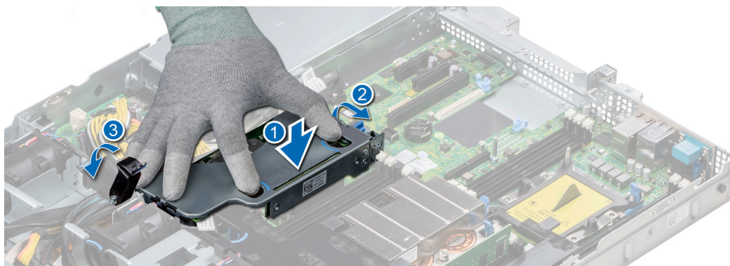
Figure 71. Installation de la carte de montage PERC interne
