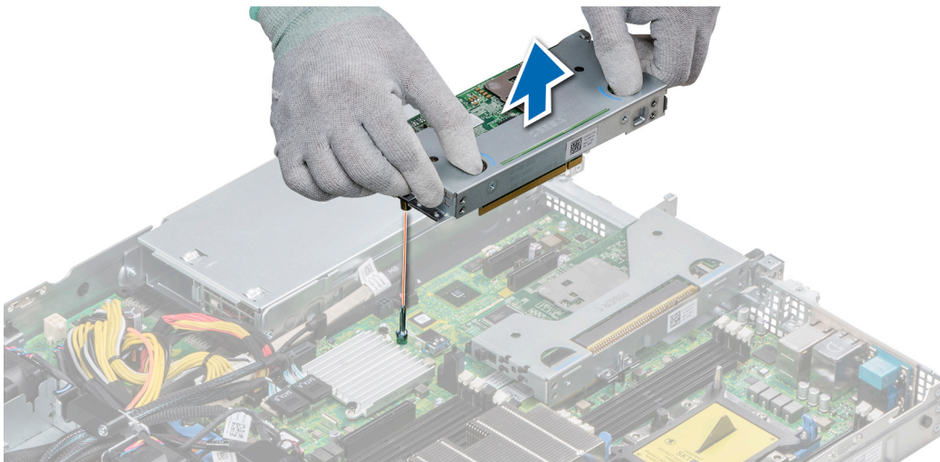
Figure 59. Retrait d'une carte de montage pour carte d'extension 2
