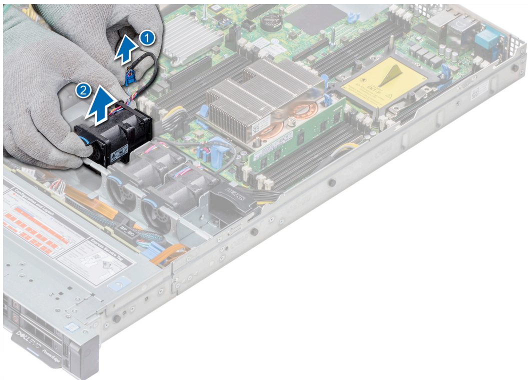
Figure 25. Retrait du ventilateur de refroidissement
