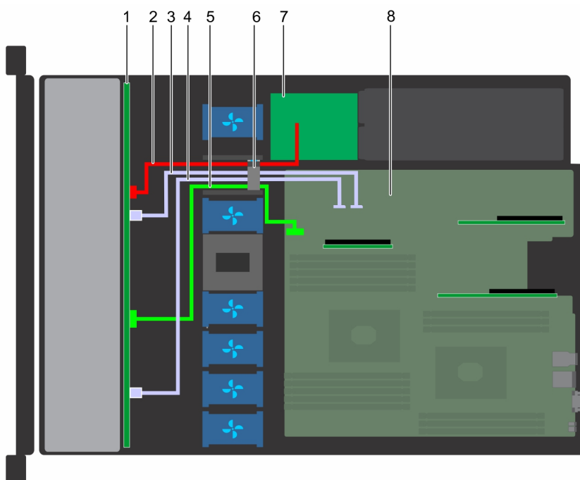
Figure 91. Acheminement des câbles : fond de panier de 8 disques durs de 2,5 pouces avec SATA intégré
