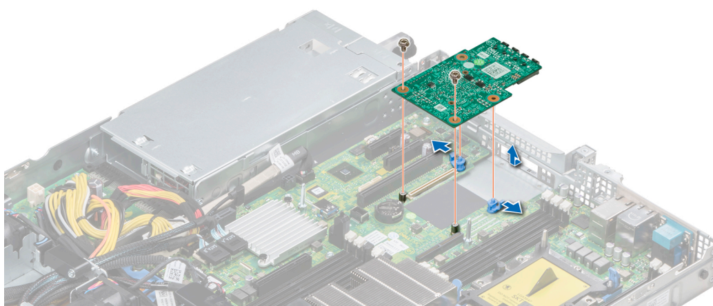
Figure 80. Retrait de la carte de montage LOM
