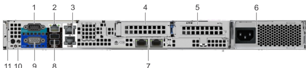
Figure 10. Vue arrière du système avec 2 cartes de montage
