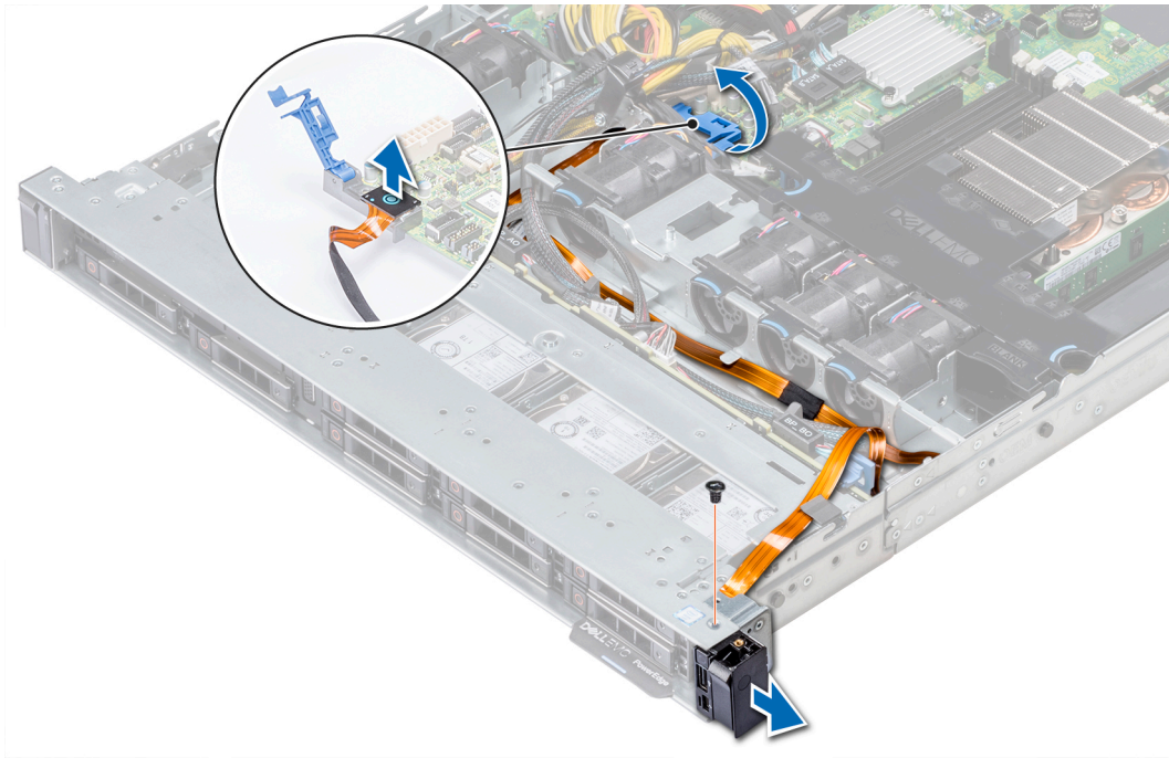
Figure 110. Retrait du panneau de commande droit
