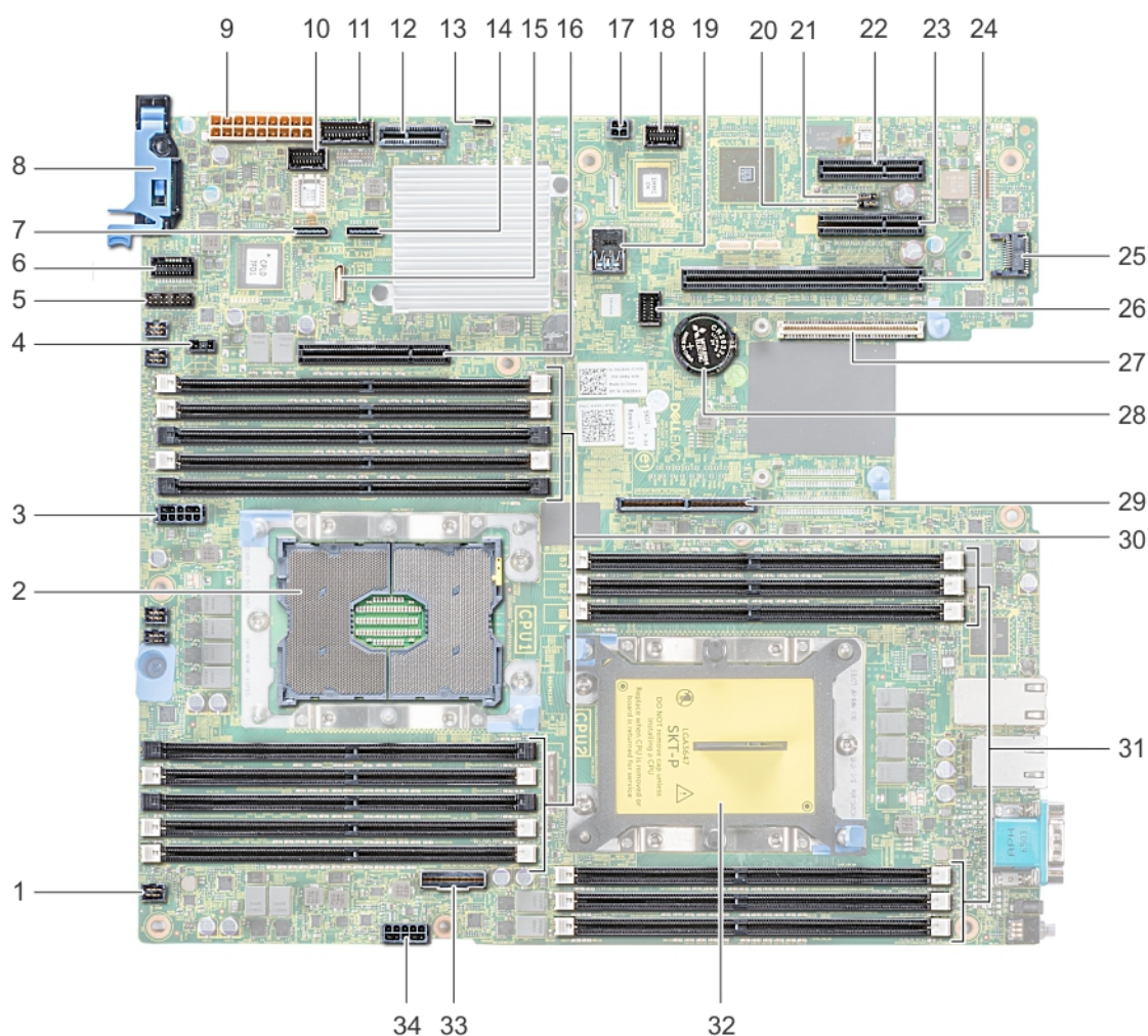
Figure 115. Connecteurs et cavaliers de la carte système
