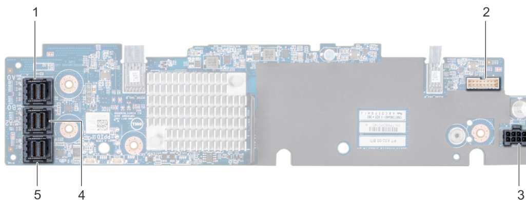
Figure 85. Backplane 10 x 2,5 avec carte d'extension
