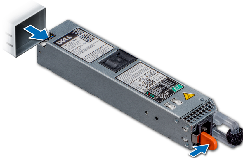
Figure 100. Retrait d'une unité d'alimentation
