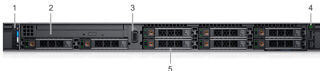
Figure 1. Vue avant d'un système à 8 disques de 2,5 pouces
