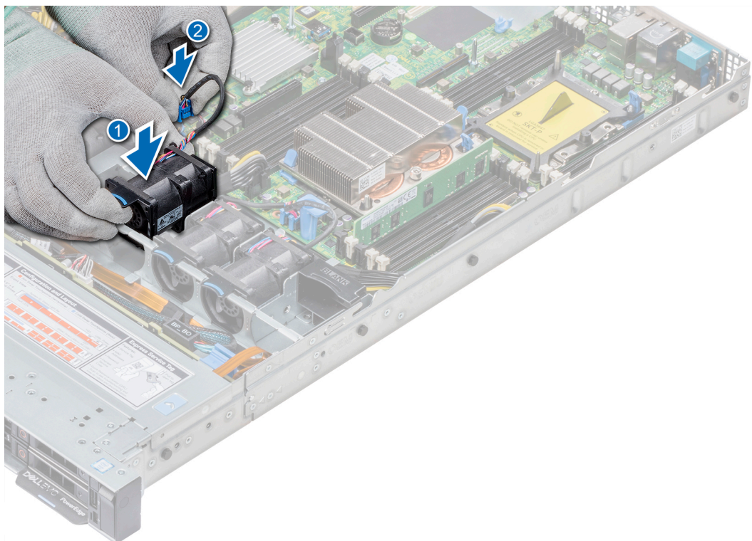
Figure 26. Installation du ventilateur de refroidissement
