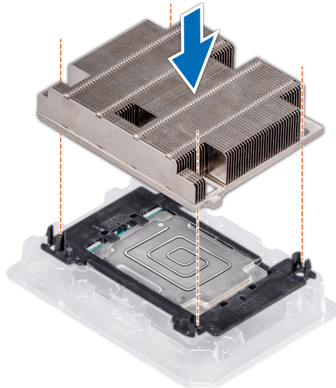
Figure 47. Installation du dissipateur de chaleur sur le processeur
