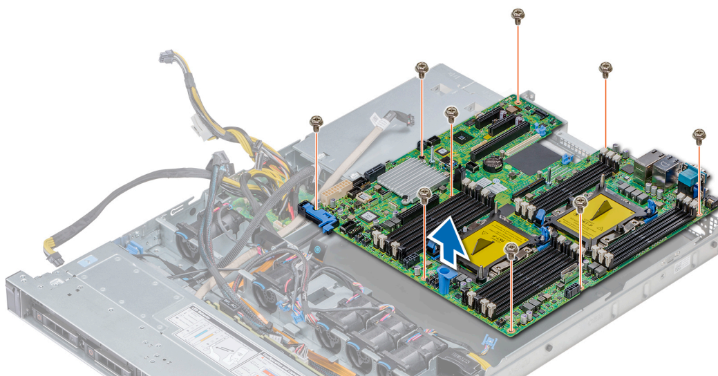
Figure 112. Retrait de la carte système
