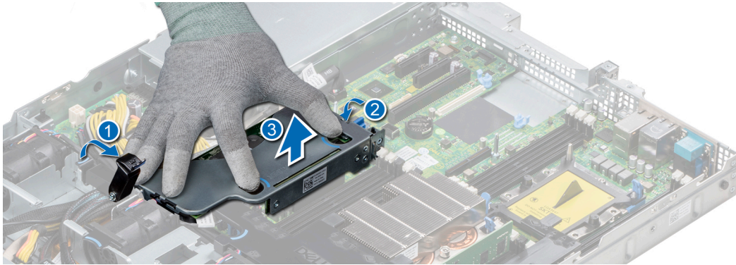
Figure 48. Retrait de la carte de montage PERC interne
