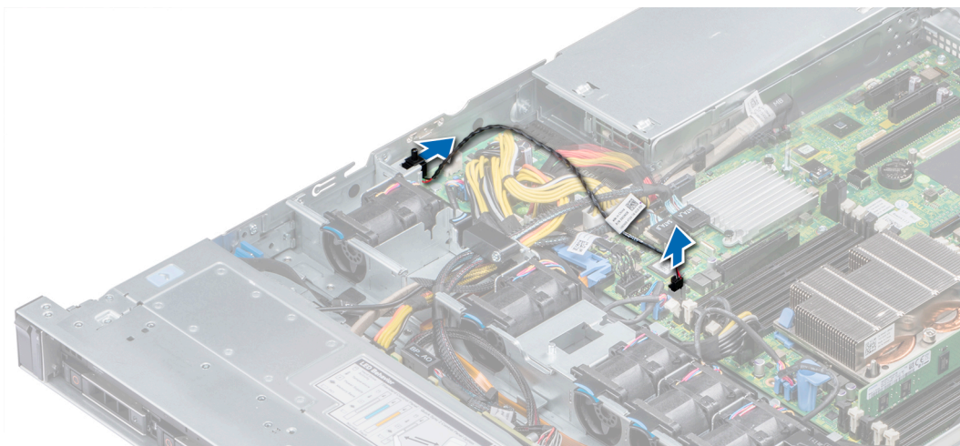
Figure 27. Retrait d'un commutateur d'intrusion
