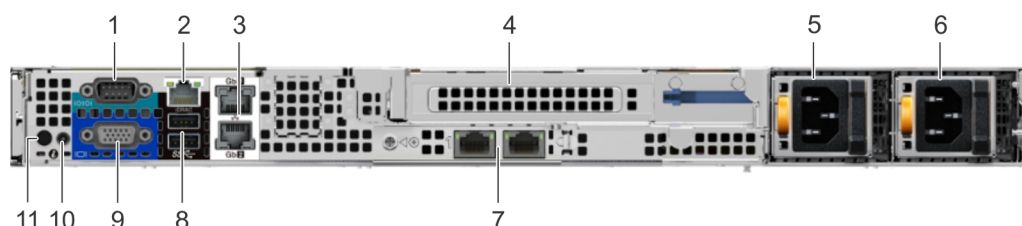
Figure 9. Vue arrière du système avec carte de montage hauteur standard
