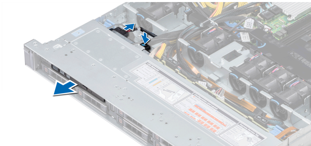
Figure 96. Retrait du lecteur optique
