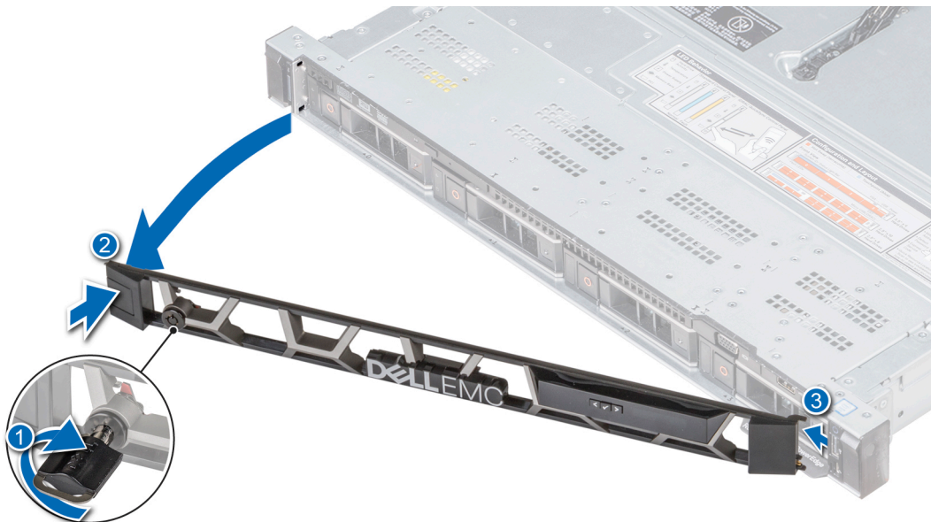
Figure 16. Retrait du cadre avant avec le panneau LCD
