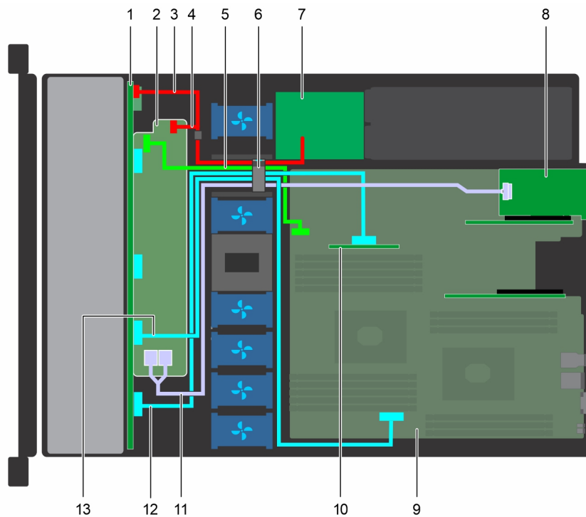
Figure 89. Acheminement des câbles : fond de panier de 10 disques de 2,5 pouces avec technologie NVMe
