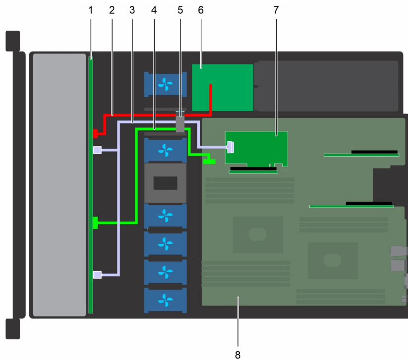
Figure 90. Acheminement des câbles : fond de panier de 8 disques durs de 2,5 pouces avec carte de montage PERC
