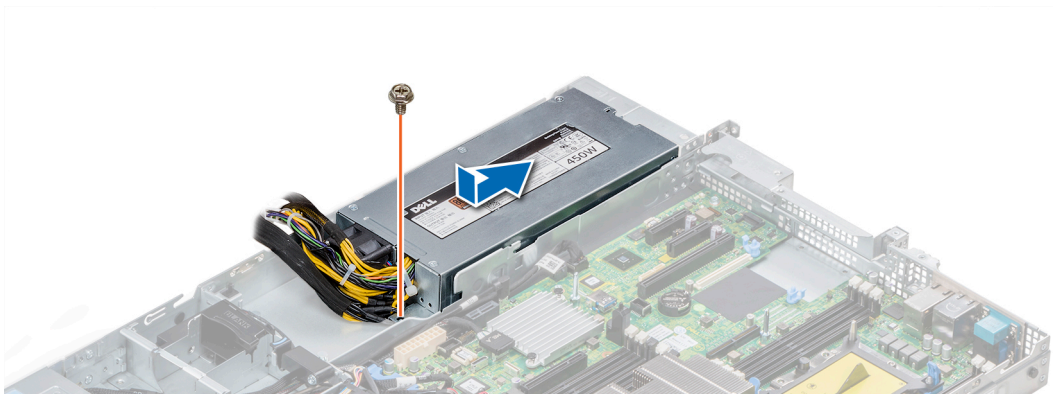
Figure 103. Installation d'un PSU secteur connecté non redondant
