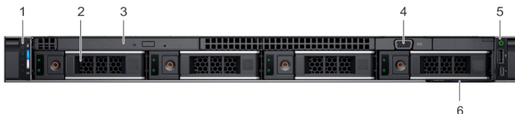
Figure 2. Vue avant d'un système à 4 disques de 3,5 pouces
