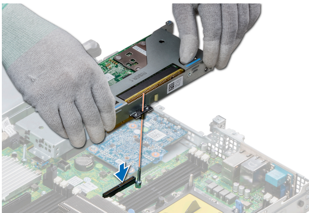
Figure 55. Installation d'une carte de montage pour carte d'extension 1
