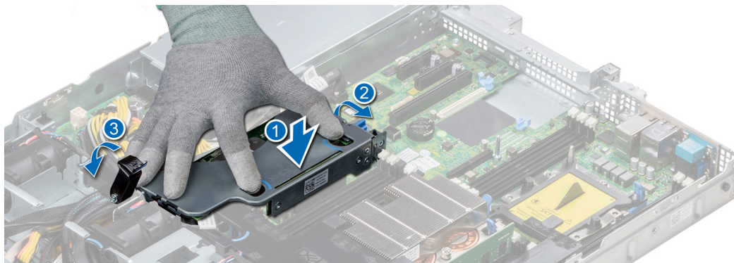
Figure 51. Installation de la carte de montage PERC interne
