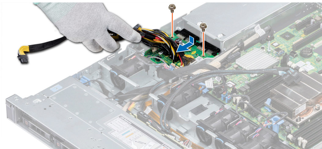
Figure 105. Installation de la carte interposeur d'alimentation
