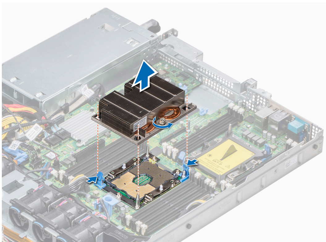
Figure 42. Retrait du module du processeur et du dissipateur de chaleur
