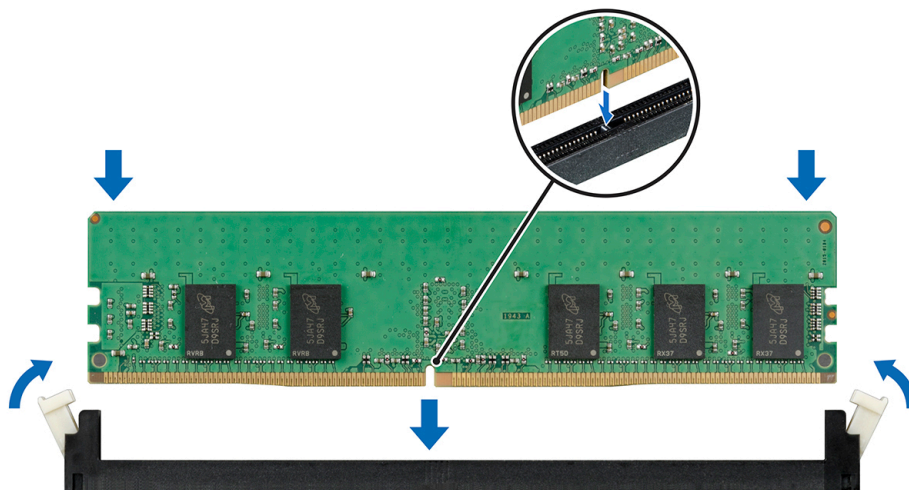
Figure 41. Installation d'une barrette de mémoire
