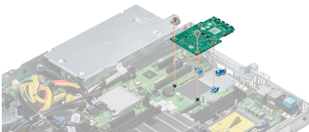
Figure 81. Installation de la carte de montage LOM
