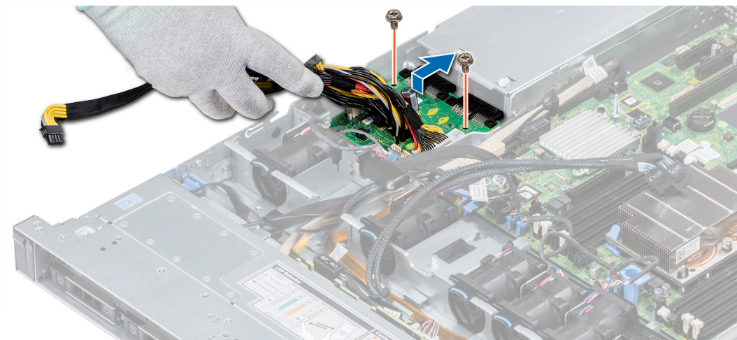
Figure 104. Retrait de la carte interposeur d'alimentation
