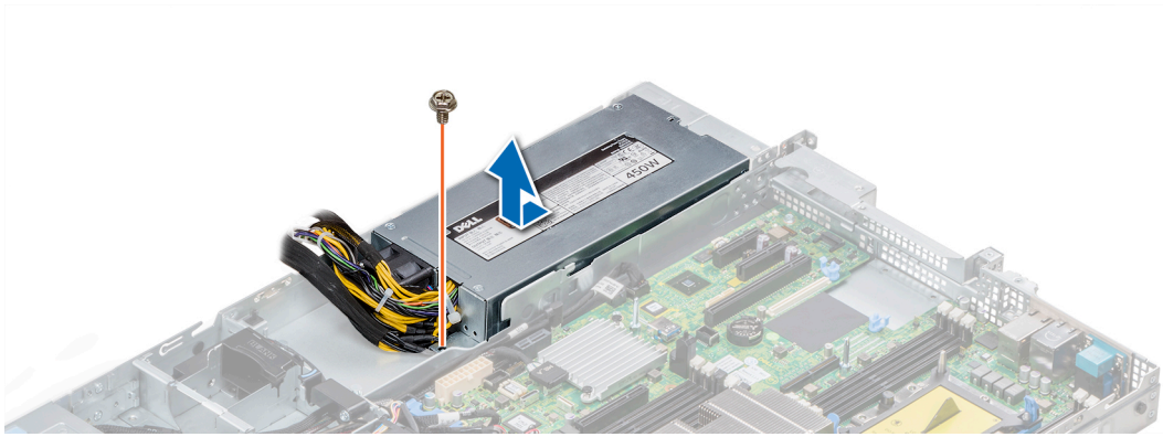
Figure 102. Retrait d'un PSU secteur connecté non redondant
