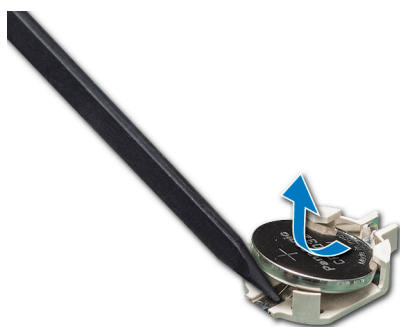
Figure 94. Retrait de la pile du système
