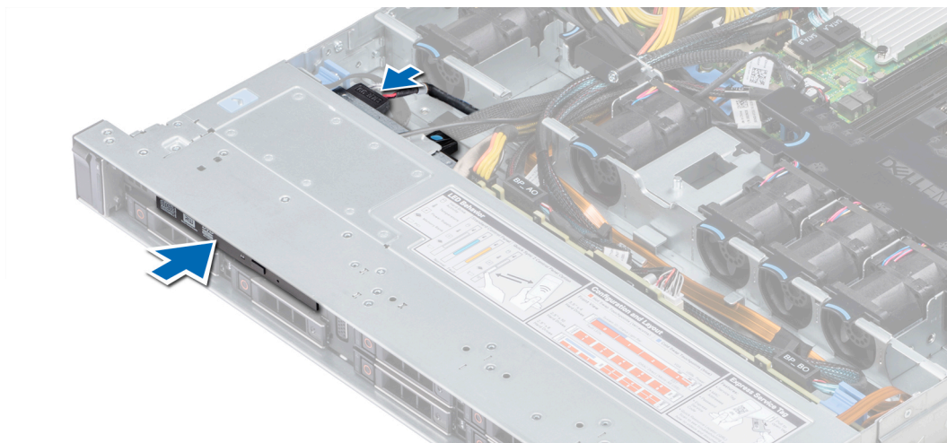
Figure 97. Installation du lecteur optique
