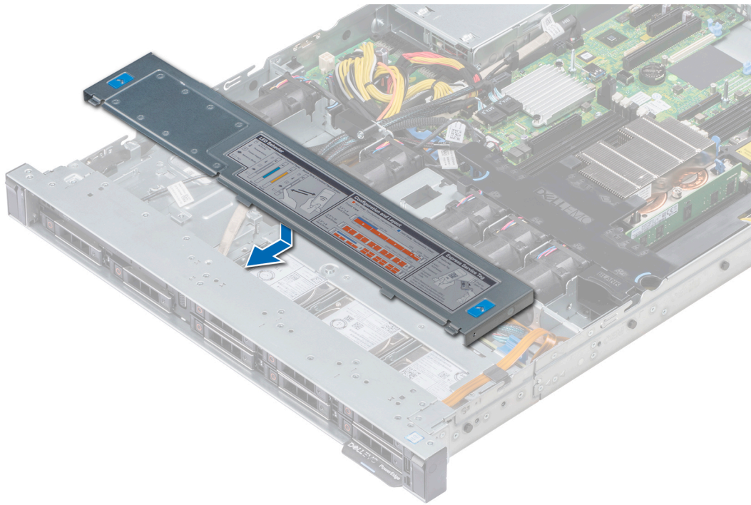
Figure 22. Installation du cache de fond de panier
