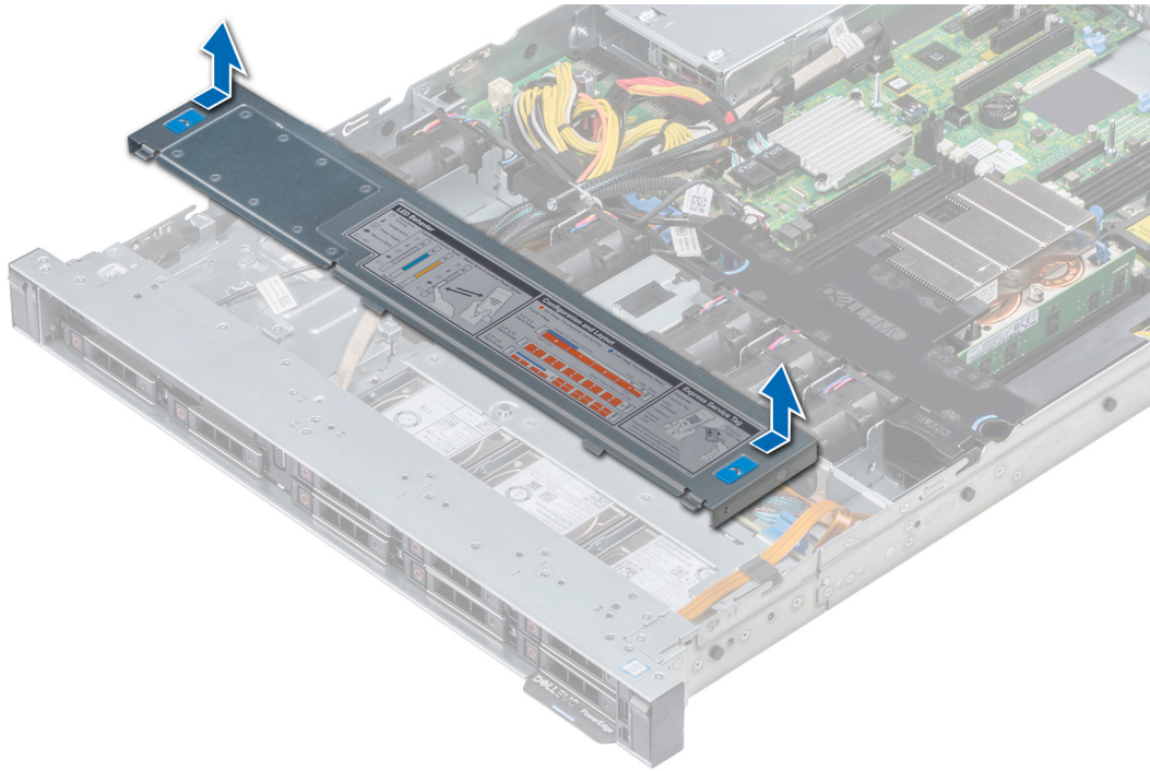
Figure 21. Retrait du cache de fond de panier
