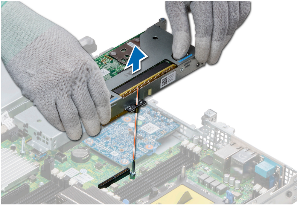
Figure 58. Retrait d'une carte de montage pour carte d'extension 1
