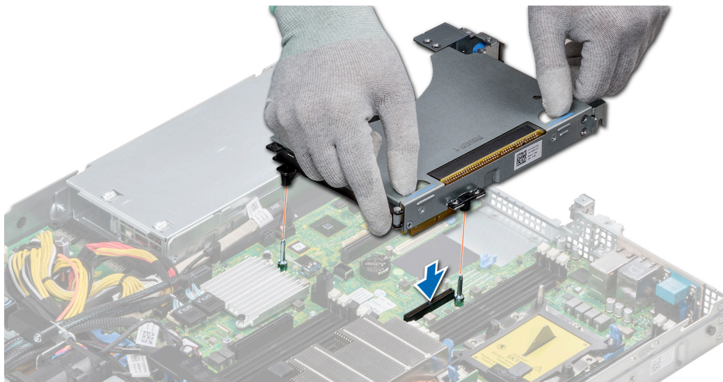
Figure 54. Installation d'une carte de montage pour carte d'extension 1A
