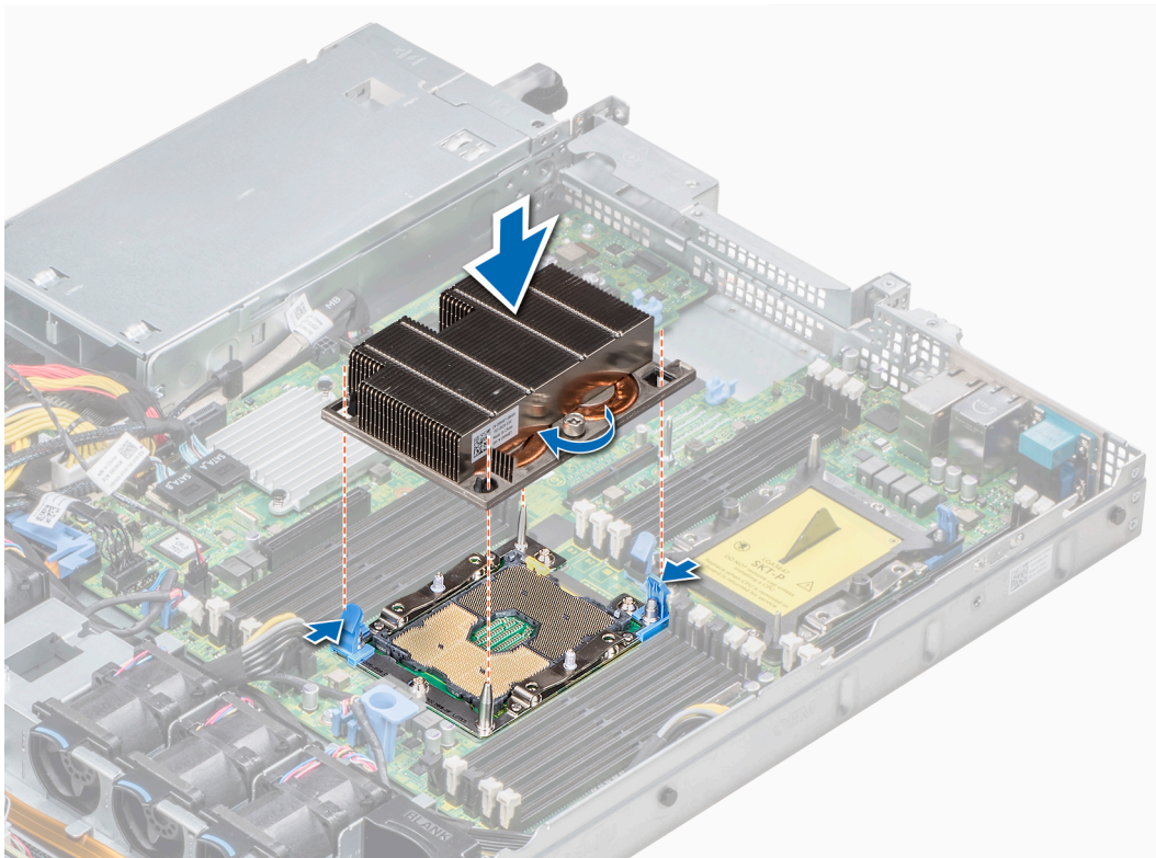
Figure 43. Installation du module du processeur et du dissipateur de chaleur
