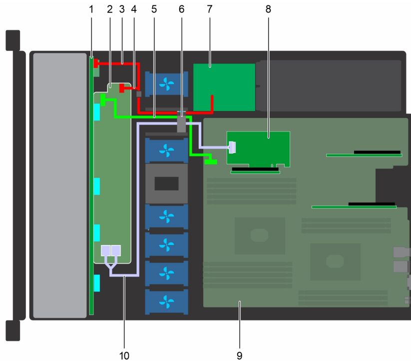
Figure 88. Acheminement des câbles : fond de panier de 10 disques durs de 2,5 pouces avec carte de montage PERC
