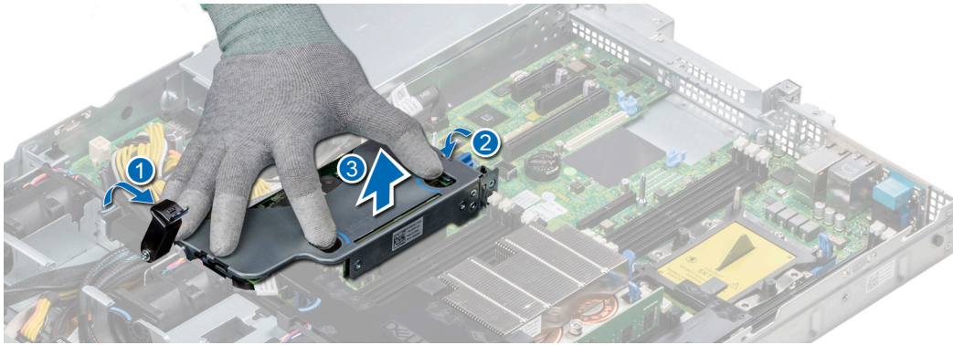
Figure 68. Retrait de la carte de montage PERC interne
