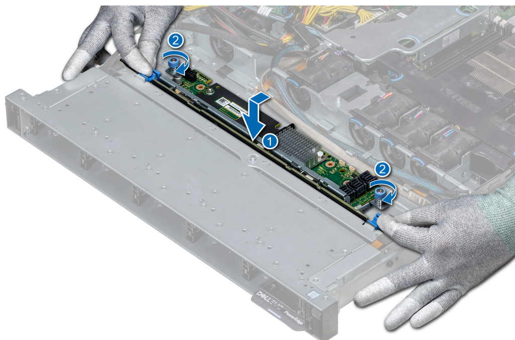
Figure 86. Installation du fond de panier de disque dur
