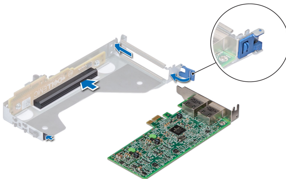
Figure 66. Installation d'une carte d'extension sur la carte de montage 2
