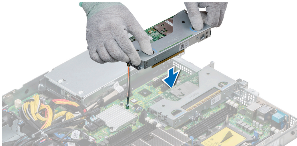
Figure 56. Installation d'une carte de montage pour carte d'extension 2
