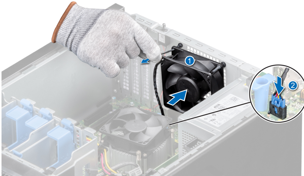
Figura 27. Instalación de un ventilador de refrigeración
