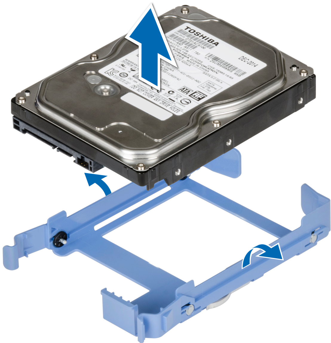
Figura 15. Extracción de la unidad del portaunidades
