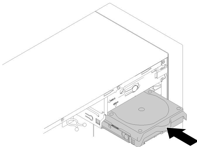
Figura 39. Installazione di un assieme dell'unità nel vano 3
