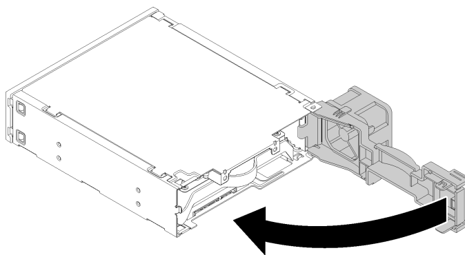
Figura 48. Chiusura del fermo dell'adattatore dell'unità
