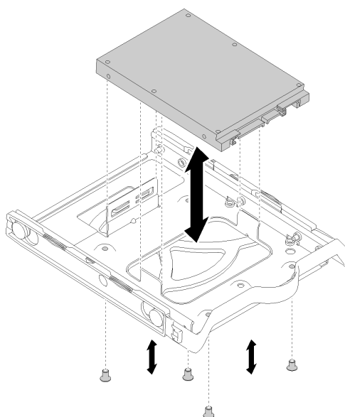
Figura 37. Installazione di un'unità da 2,5" nel supporto
