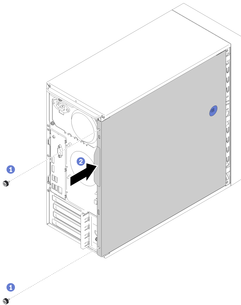
Figura 55. Installazione del coperchio del server
