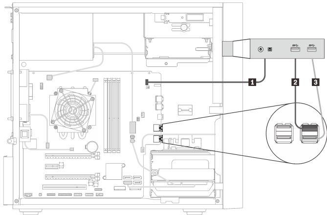
Figura 28. Instradamento dei cavi per il vano dell'unità 1
