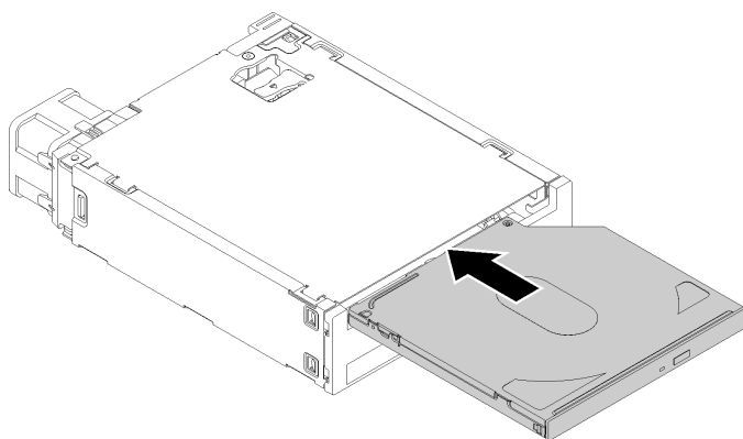
Figura 44. Installazione dell'unità ottica Slim nell'adattatore del vano dell'unità
