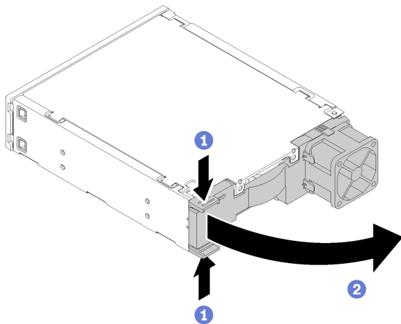
Figura 45. Aprire il fermo dell'assieme adattatore
