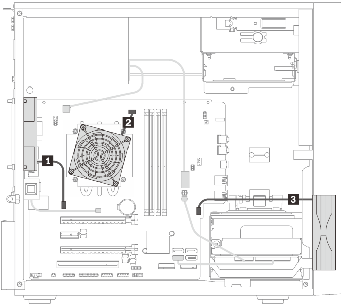
Figura 27. Instradamento dei cavi per le ventole
