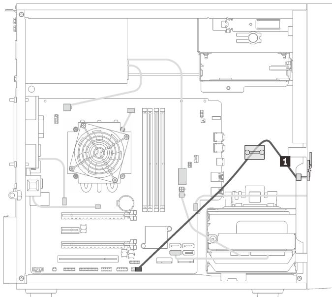
Figura 29. Instradamento dei cavi per il sensore termico
