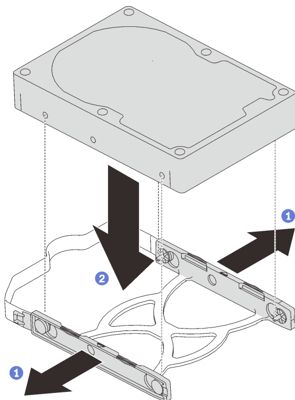
Figura 36. Installazione di un'unità da 3,5" nel supporto
