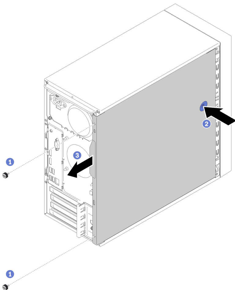
Figura 31. Rimozione del coperchio del server
