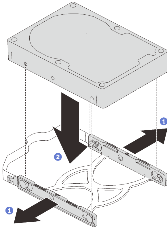
Figura 46. Installazione di un'unità da 3,5" nel supporto
