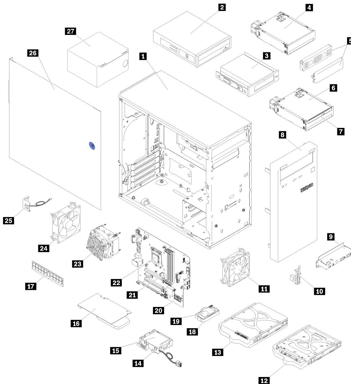
Figura 30. Componenti del server
