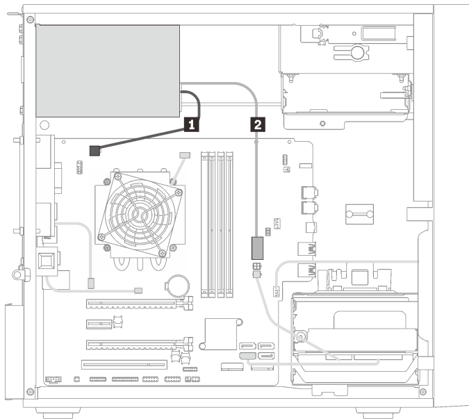
Figura 26. Instradamento dei cavi per l'unità di alimentazione
