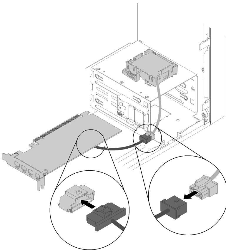
Figura 53. Collegamento del cavo del modulo di alimentazione flash
