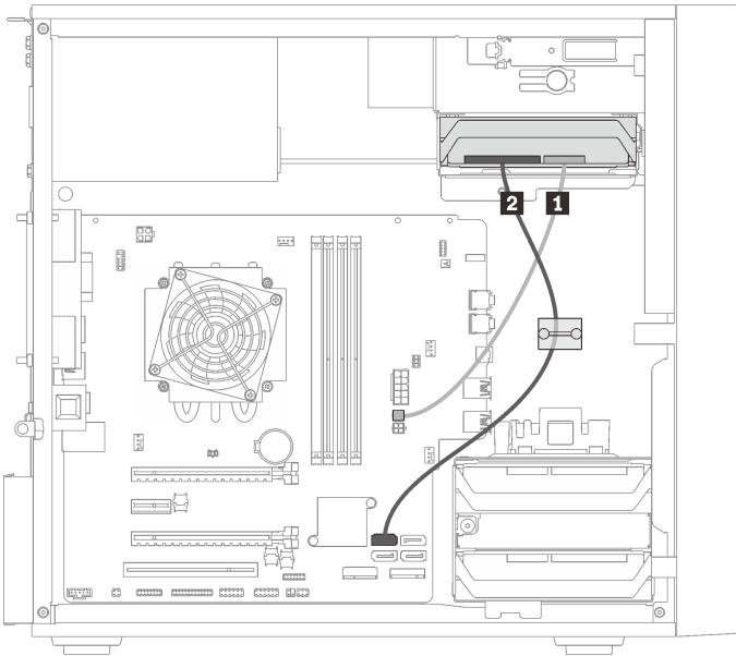
Figura 18. Instradamento dei cavi per il vano dell'unità 3
