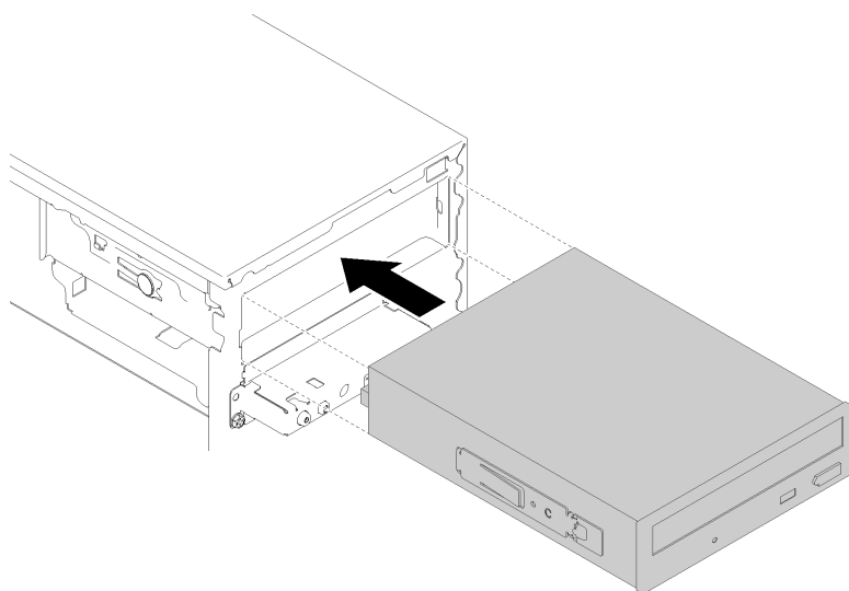
Figura 42. Installazione dell'insieme dell'unità ottica
