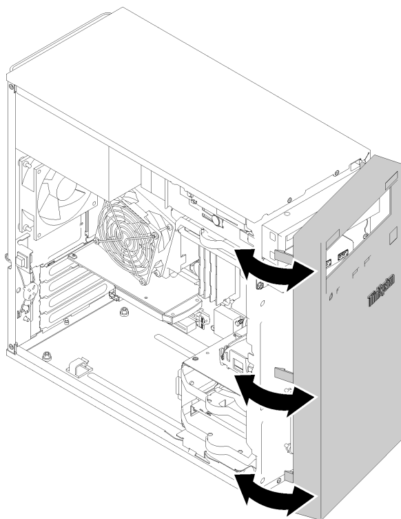
Figura 32. Rimozione della mascherina anteriore
