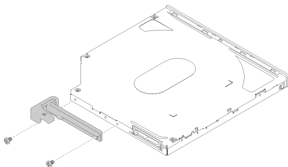
Figura 43. Installazione del supporto all'unità ottica Slim
