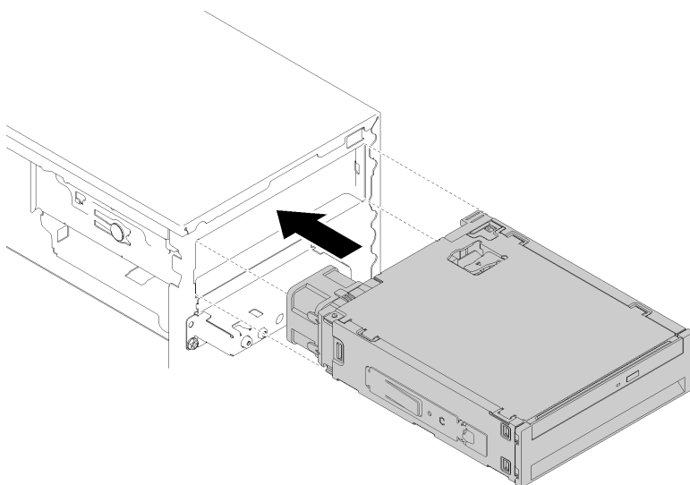
Figura 49. Installazione dell'assieme adattatore del vano dell'unità
