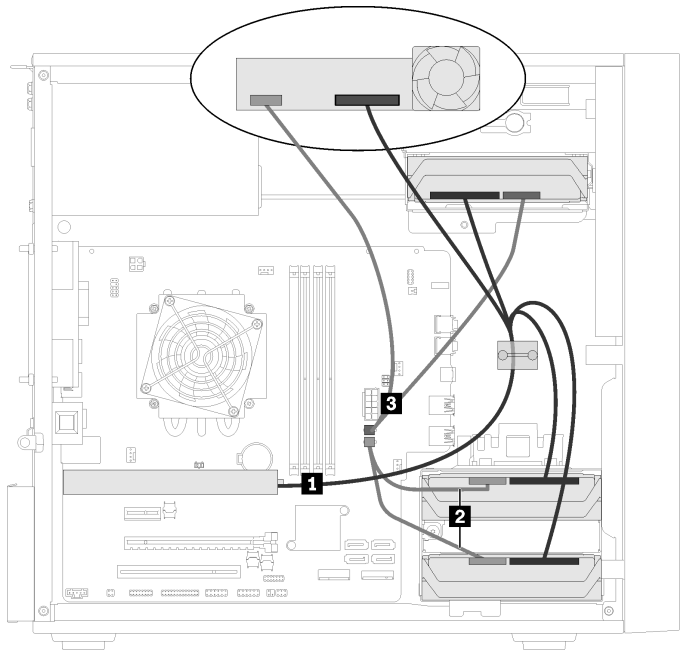
Figura 25. Instradamento dei cavi per quattro unità con l'adattatore RAID
