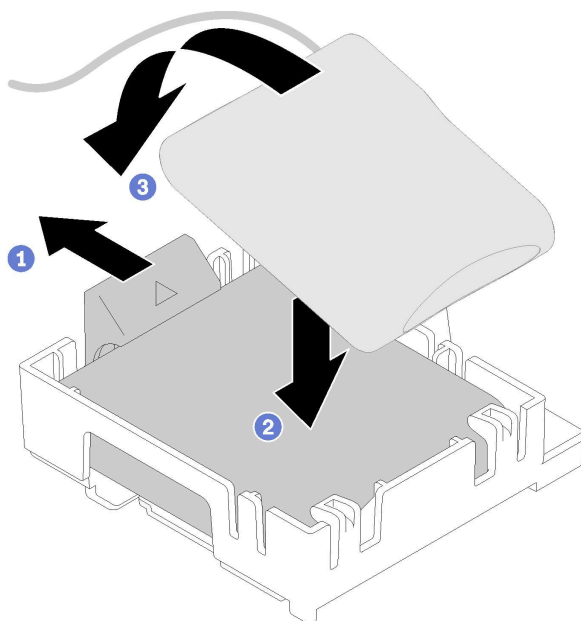
Figura 51. Installazione del modulo di alimentazione flash nel fermo
