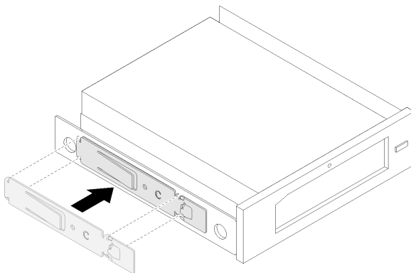
Figura 41. Installazione del fermo dell'unità su un'unità nastro
