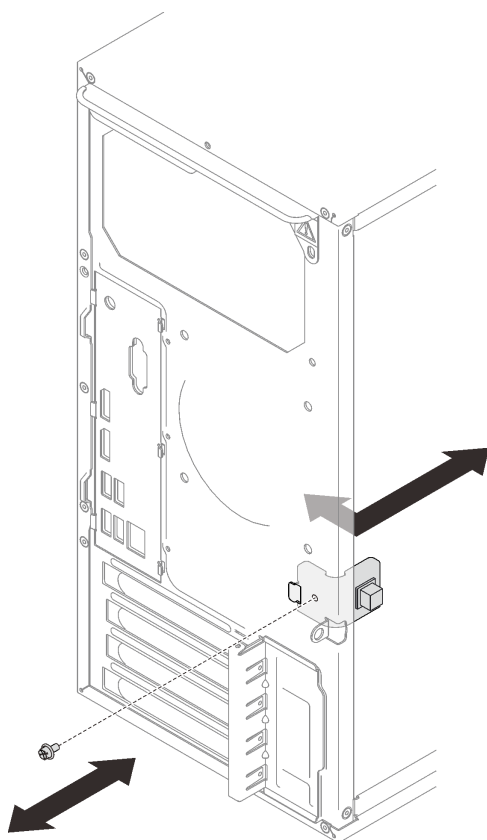
Figura 54. Installazione dello switch di intrusione
