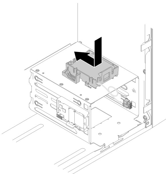
Figura 52. Installazione dell'assieme del modulo di alimentazione flash
