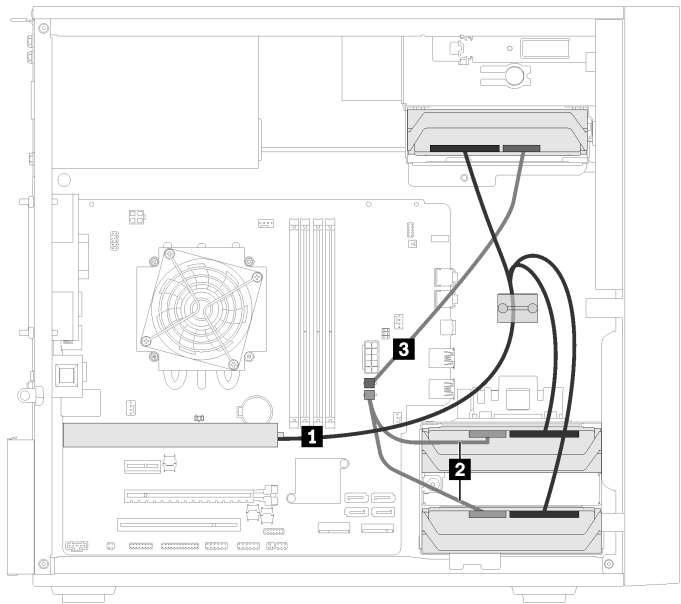
Figura 24. Instradamento dei cavi per tre unità con l'adattatore RAID
