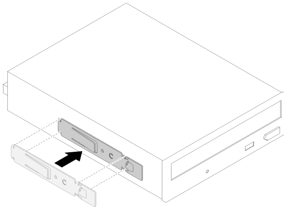
Figura 40. Installazione del fermo dell'unità su un'unità ottica
