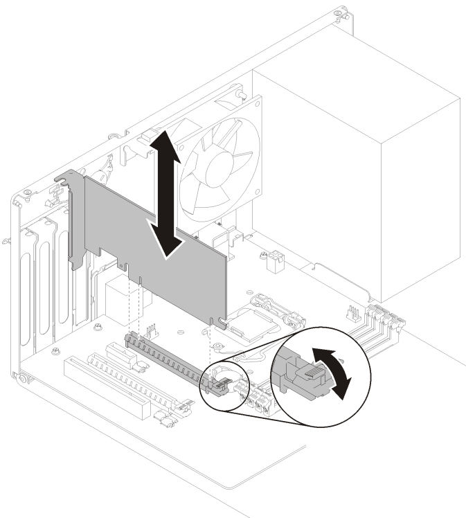
Figura 50. Installazione dell'adattatore PCIe
