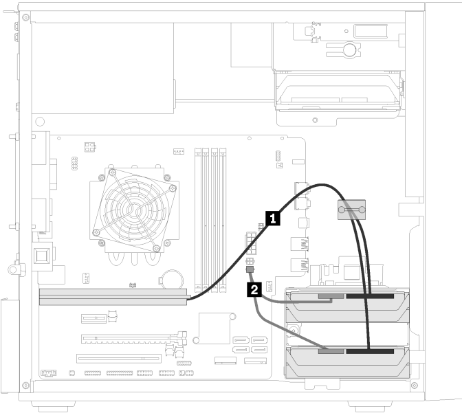
Figura 23. Instradamento dei cavi per due unità con l'adattatore RAID
