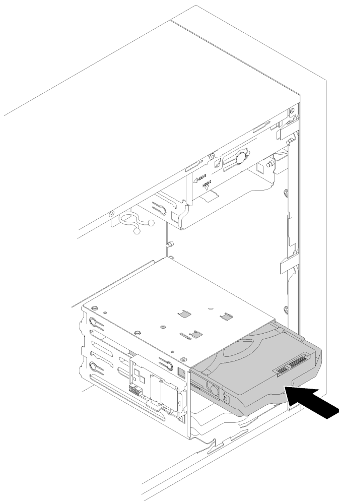
Figura 38. Installazione di un assieme dell'unità nel vano 2
