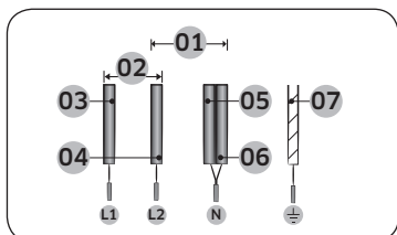
2N~ (16A): Separare i cavi a 2 fasi (L1 e L2) prima di eseguire il collegamento.
