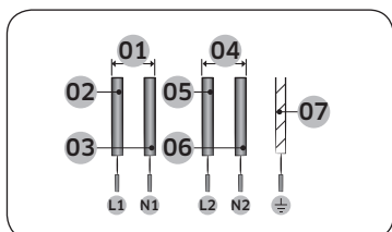
2 x 1N~ (16A): Prima di effettuare il collegamento separare i fili.
