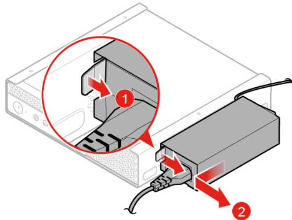
Figura 13. Rimozione della staffa dell'adattatore di alimentazione
