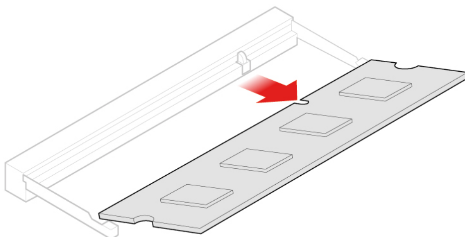
Figura 43. Apertura del fermo del modulo di memoria
