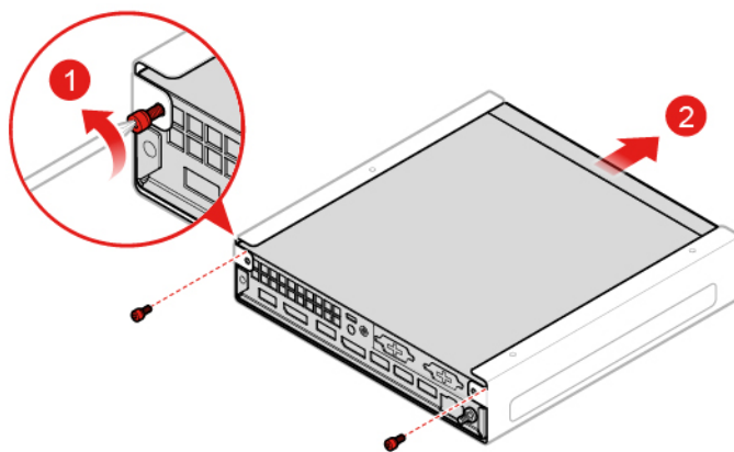
Figura 7. Rimozione della staffa di montaggio VESA
