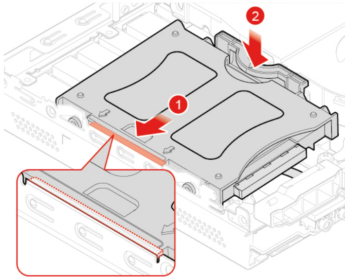
Figura 20. Installazione della staffa dell'unità di memorizzazione
