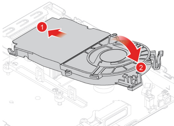
Figura 24. Installazione della ventola di sistema
