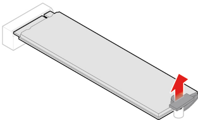
Figura 47. Sblocco del fermo dell'unità SSD M.2
