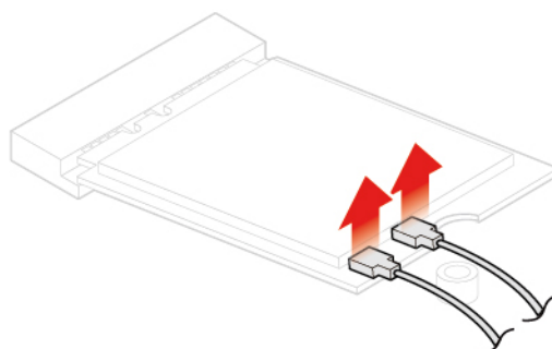
Figura 30. Scollegamento delle antenne Wi-Fi
