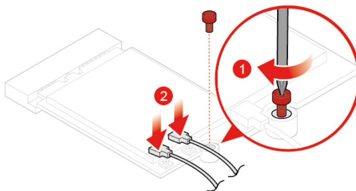
Figura 33. Collegamento delle antenne Wi-Fi
