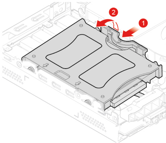
Figura 17. Rimozione della staffa dell'unità di memorizzazione
