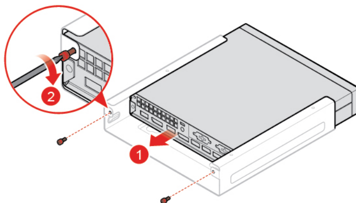
Figura 8. Installazione della staffa di montaggio VESA
