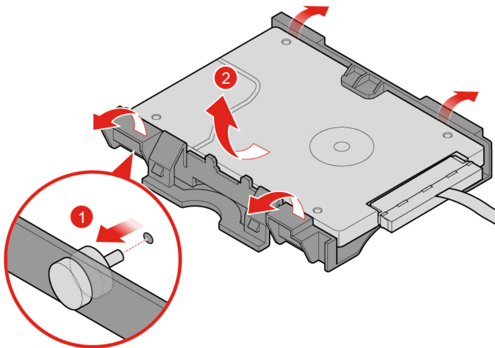
Figura 18. Rimozione dell'unità di memorizzazione
