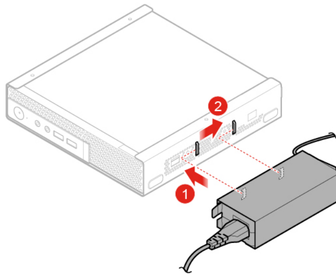
Figura 14. Installazione della staffa dell'adattatore di alimentazione
