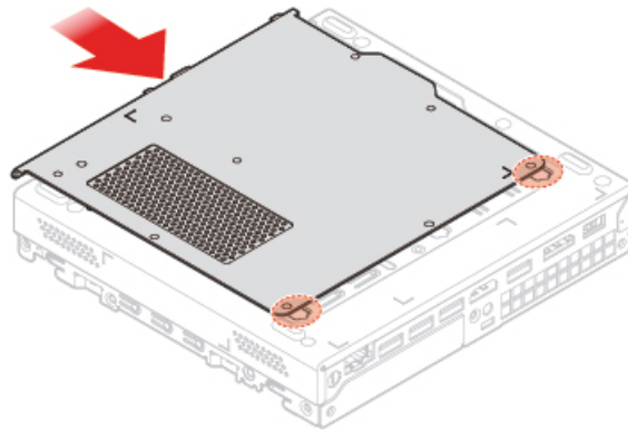
Figura 42. Installazione del coperchio inferiore
