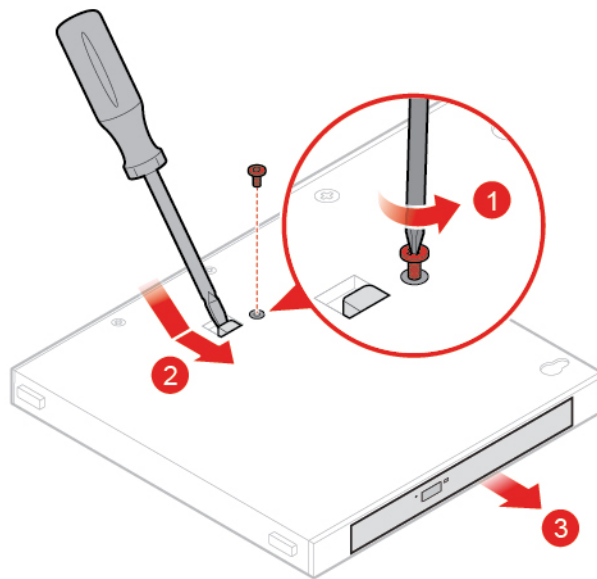
Figura 10. Rimozione dell'unità ottica esterna
