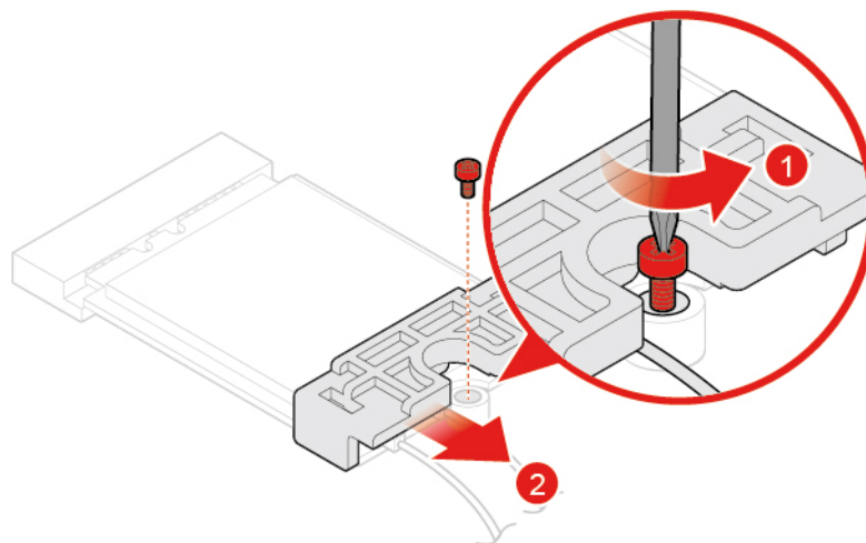
Figura 29. Rimozione dello schermo della scheda Wi-Fi
