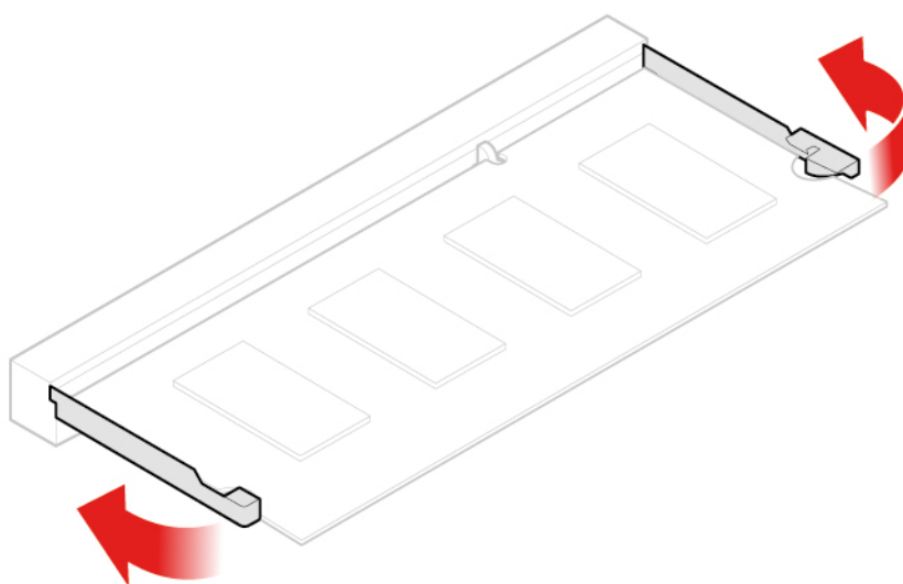
Figura 43. Apertura del fermo del modulo di memoria
