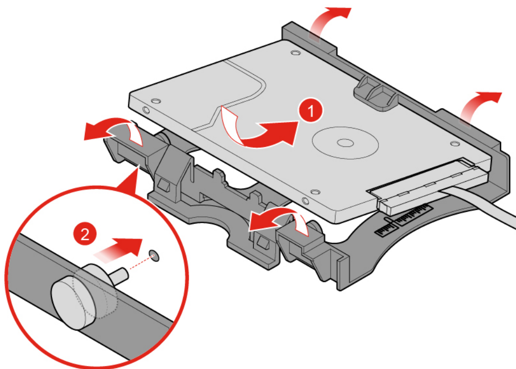
Figura 19. Installazione dell'unità di memorizzazione
