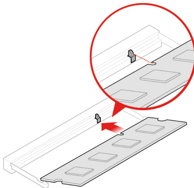
Figura 45. Installazione del modulo di memoria
