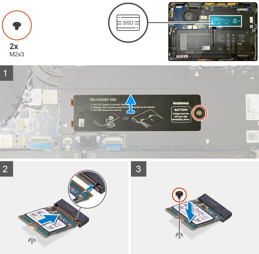
Abbildung 1. 2230-SSD
