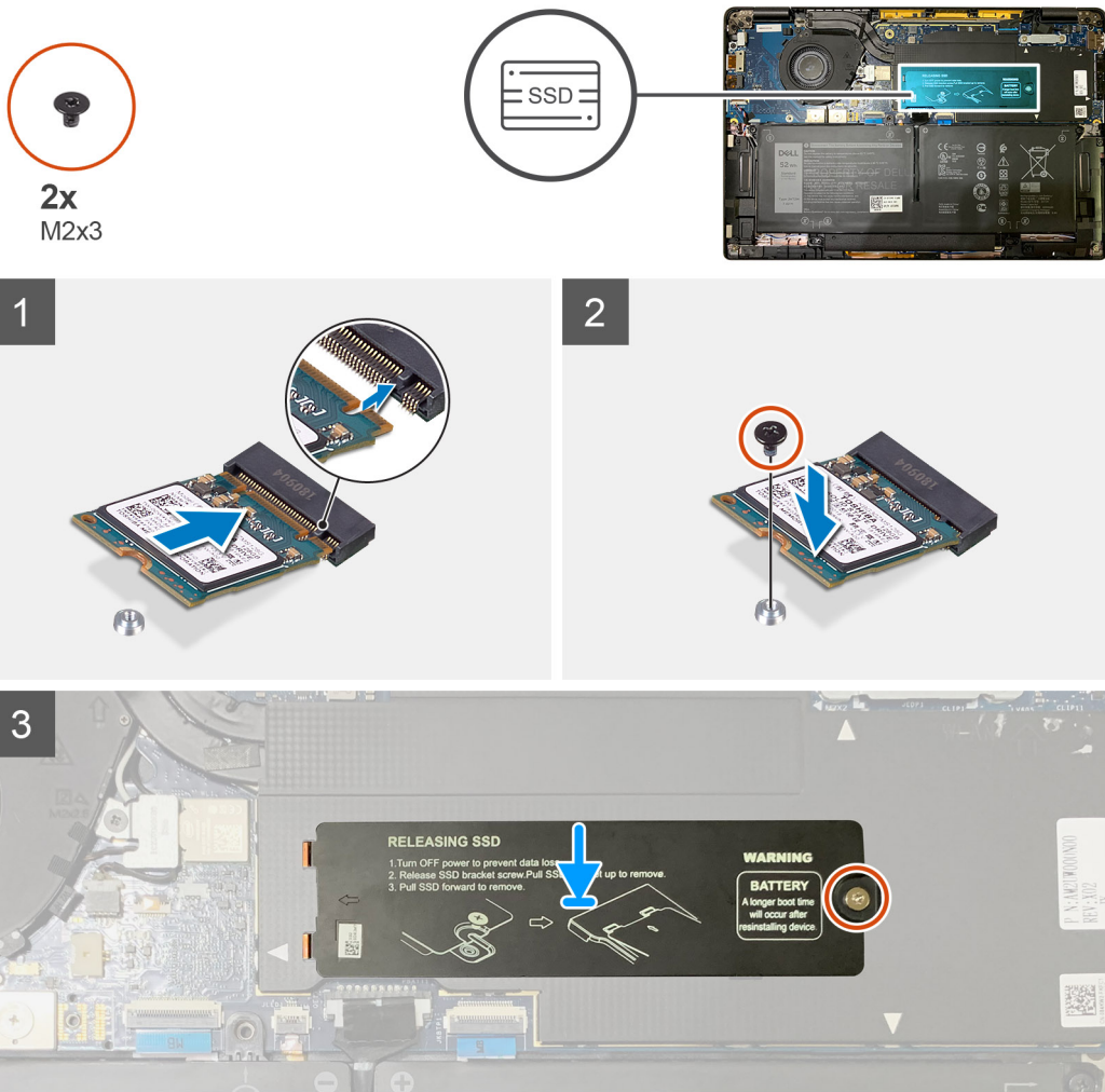
Abbildung 3. 2230-SSD
