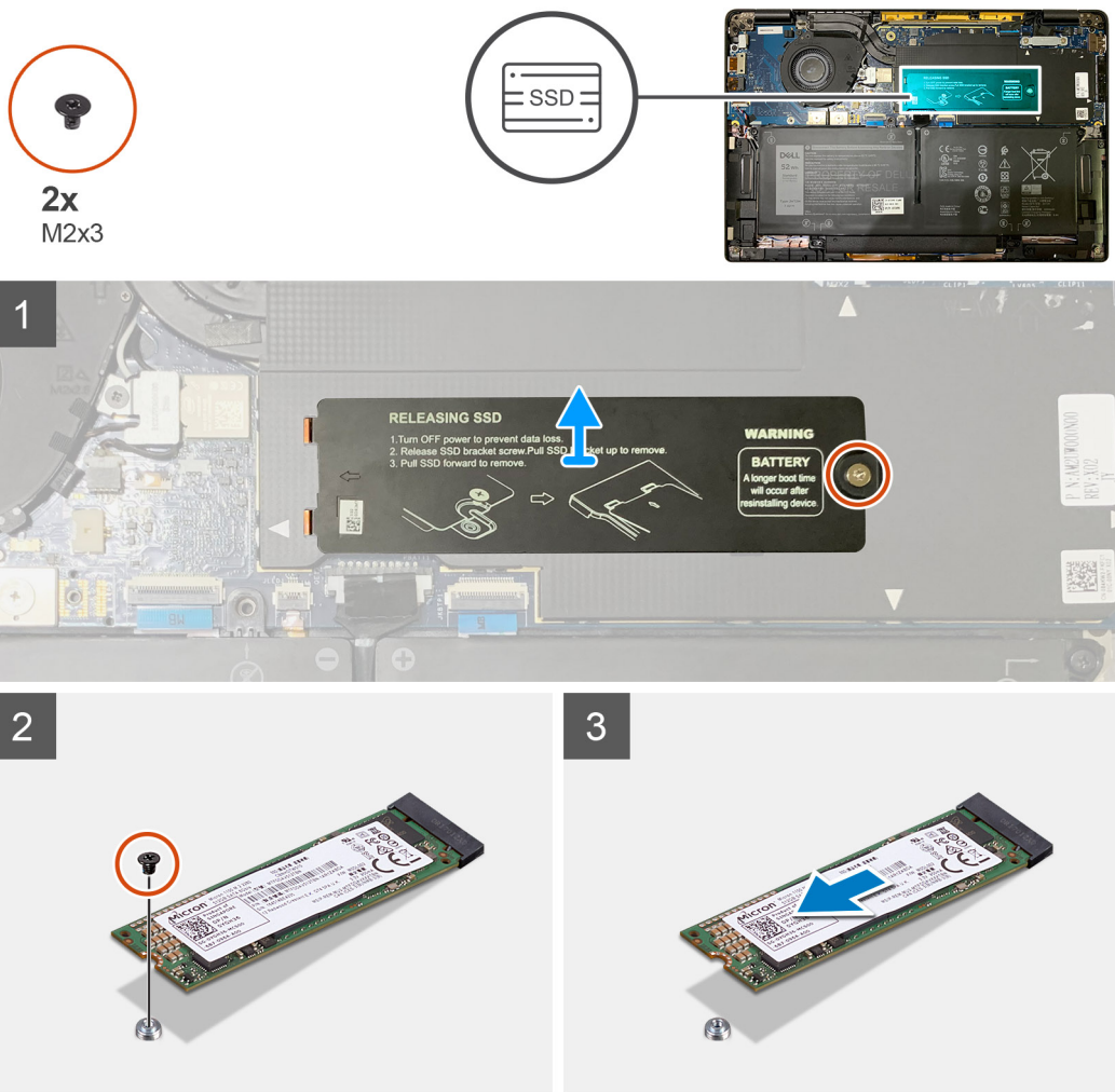
Abbildung 2. 2280-SSD
