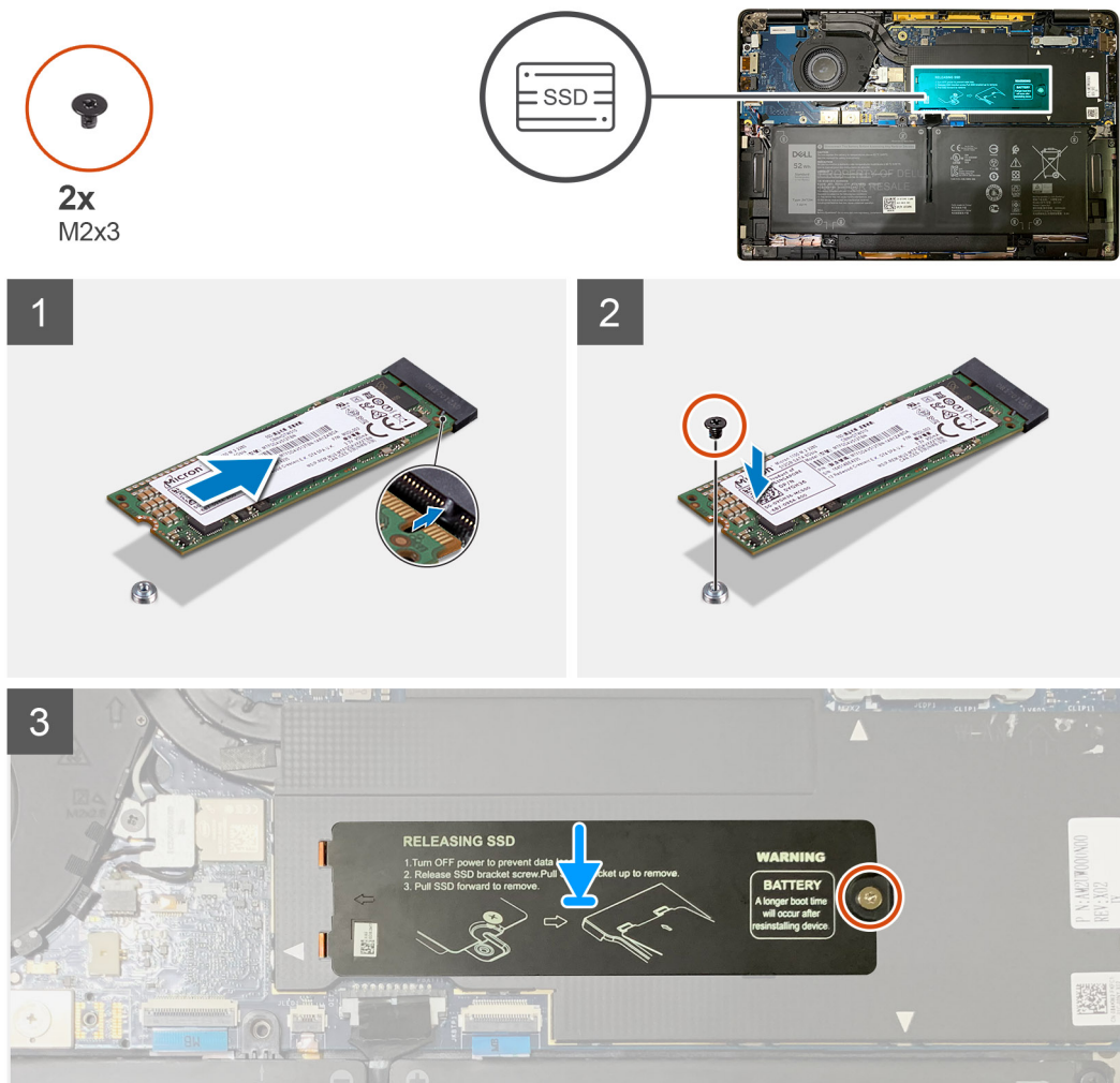
Abbildung 4. 2280-SSD
