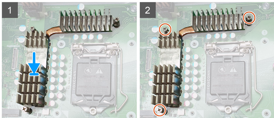
Figura 15. Gruppo dissipatore di calore VR per sistemi spediti con CPU da 125 W
