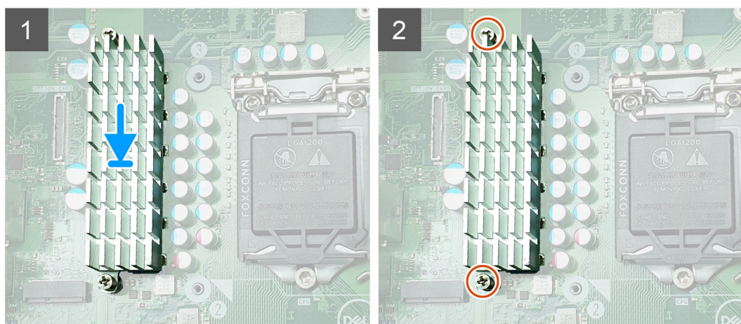
Figura 14. Gruppo dissipatore di calore VR per sistemi spediti con CPU da 65 W o 80 W
