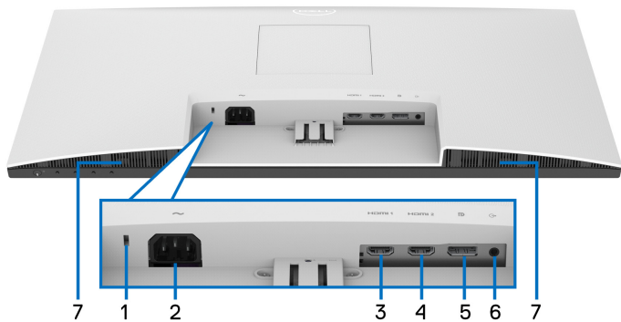
Widok od dołu bez podstawy monitora
