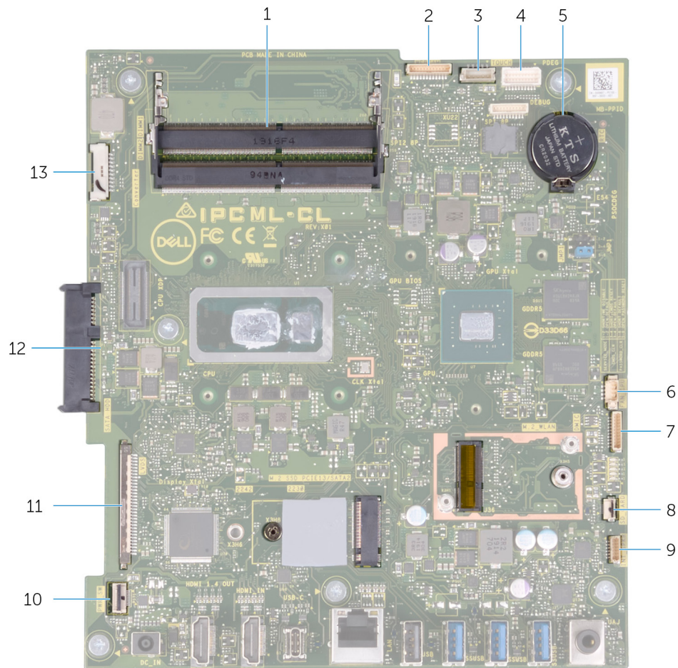
Abbildung 2. Systemplatinenanschlüsse
