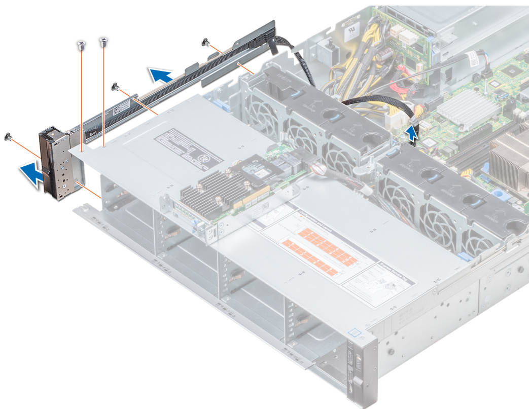
Ilustración 123. Extracción del panel de control izquierdo
