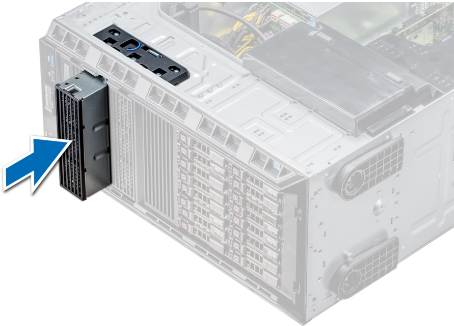
Ilustración 38. Instalación de la unidad óptica o de cinta de relleno
