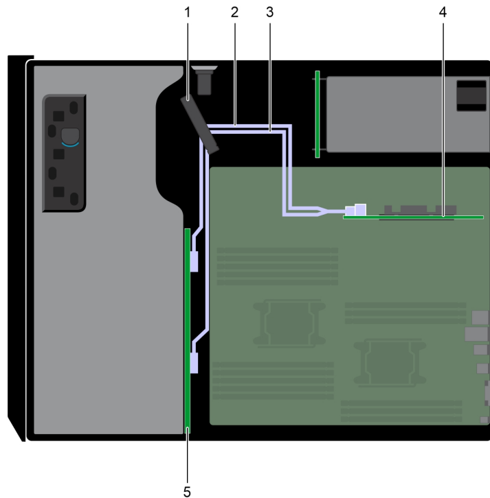
Ilustración 47. Enrutamiento de cables: backplane para 8 unidades de 3,5 pulgadas con soporte vertical de PERC interno
