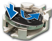
Ilustración 87. Instalación de la batería del sistema
