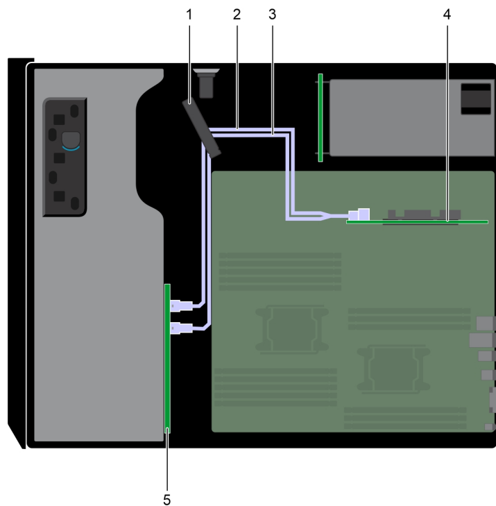
Ilustración 48. Enrutamiento de cables: backplane para 16 unidades de 2,5 pulgadas con soporte vertical de PERC interno
