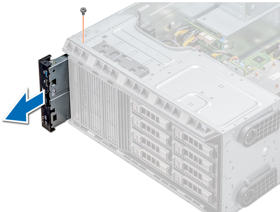
Ilustración 88. Extracción del ensamblaje del panel de control
