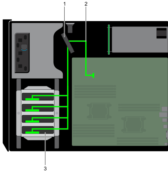
Ilustración 49. Enrutamiento de cables: backplane para 4 HDD de 3,5 pulgadas cableados
