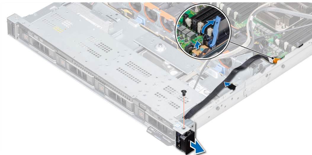
Ilustración 118. Desmontaje del panel de control derecho
