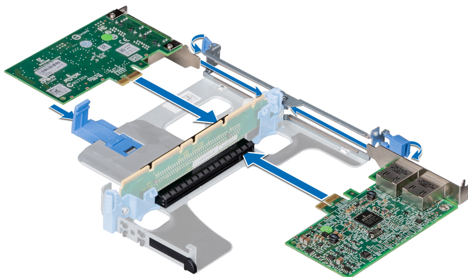
Ilustración 66. Instalación de tarjetas de expansión en el soporte vertical para tarjetas de expansión 1A
