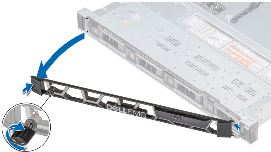
Ilustración 20. Extracción del bisel frontal opcional con el panel LCD
