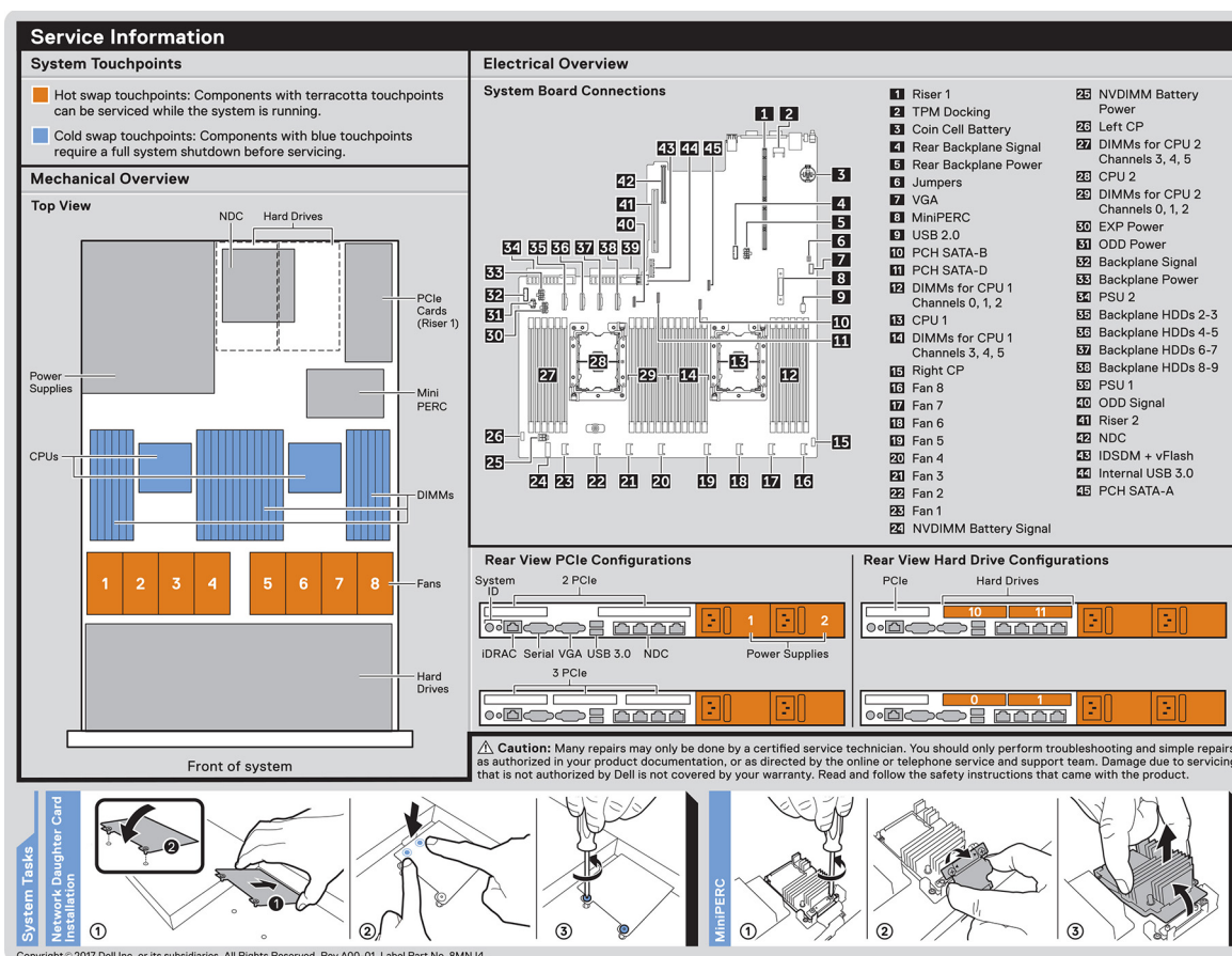
Ilustración 17. Información del servicio, información general sobre electricidad, tarjeta secundaria de red e instalación de miniPERC
