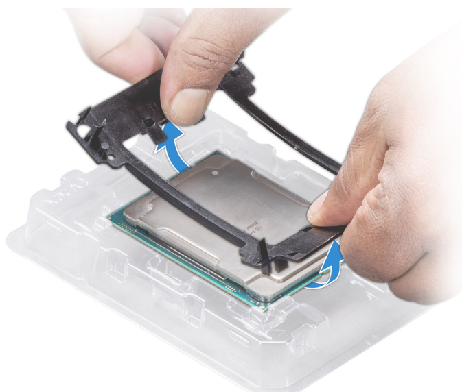
Ilustración 46. Extracción del soporte del procesador
