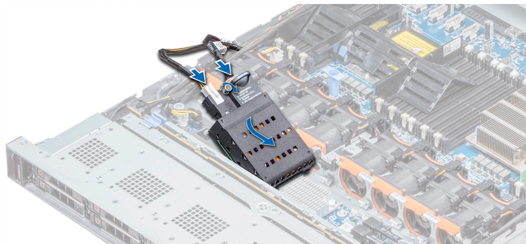
Ilustración 43. Instalación de la batería de NVDIMM-N
