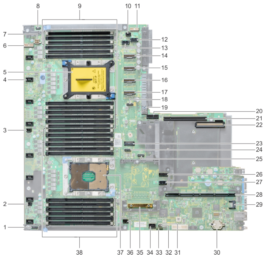
Ilustración 121. Puentes y conectores de la tarjeta madre del sistema
