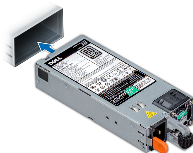
Ilustración 109. Instalación de una unidad de fuente de alimentación
