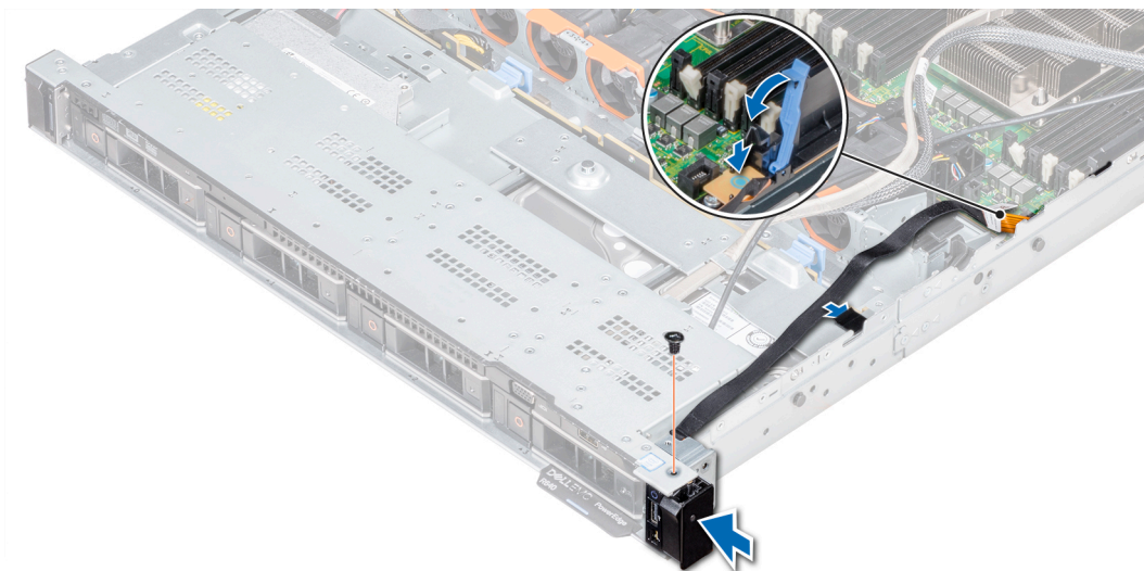
Ilustración 119. Instalación del panel de control derecho
