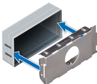
Ilustración 107. Instalación de una unidad de fuente de alimentación de relleno
