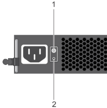
Figura 8. Indicador de estado de la fuente de alimentación de CA cableada no redundante y botón de autodiagnóstico
