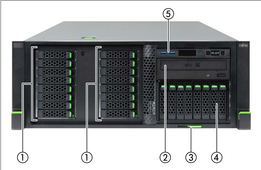
Immagine 2: Lato frontale del server modello HDD/SSD da 2,5 pollici - esempio TX1330 M4 modello rack
