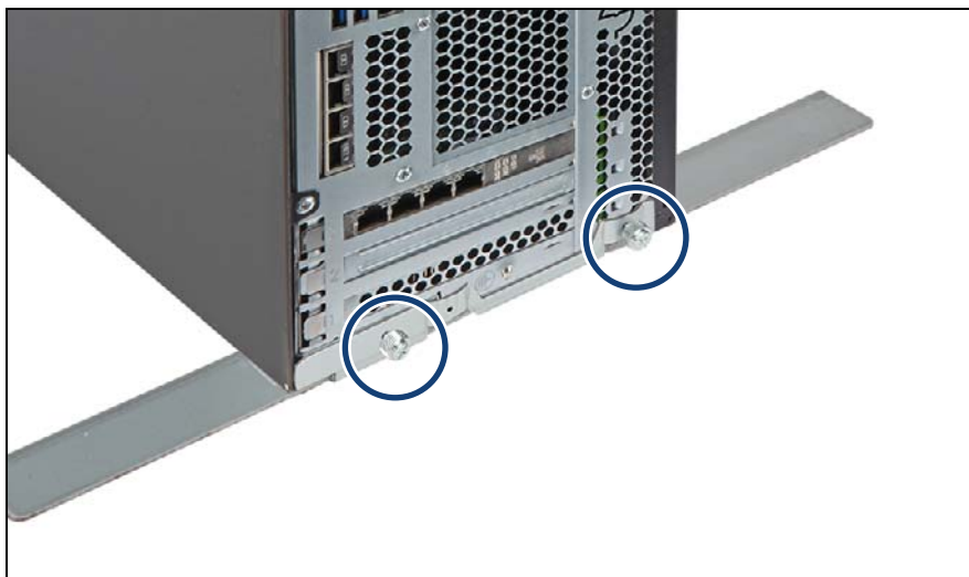
Immagine 17: Installazione della protezione antiribaltamento (B)
