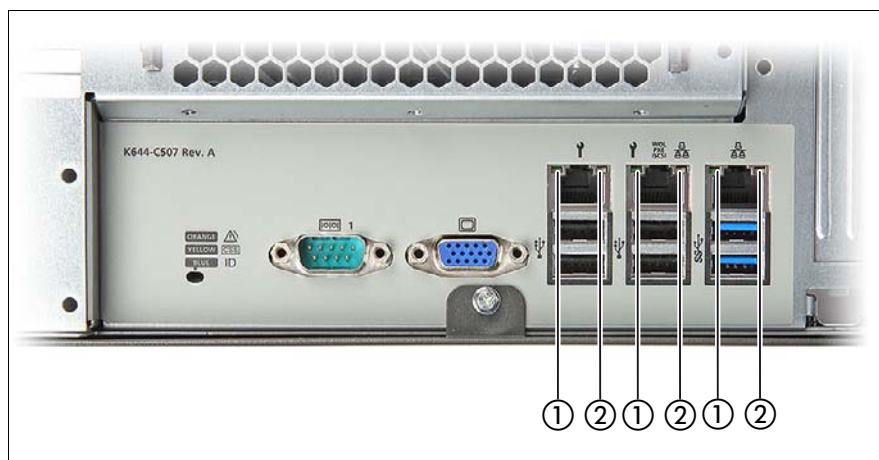
Immagine 12: Spie LAN
