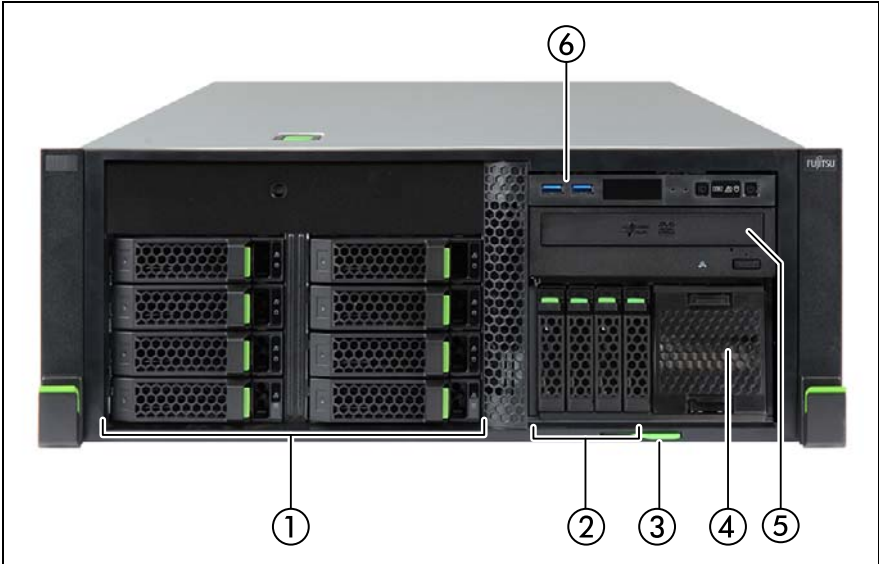
Immagine 4: Lato frontale del server modello HDD da 3,5 pollici con unità SSD PCIe - esempio TX1330 M4 modello rack
