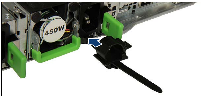
Immagine 33: Installazione del morsetto antitrazione
