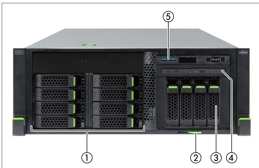
Immagine 3: Lato frontale del server modello HDD da 3,5 pollici - esempio TX1330 M4 modello rack
