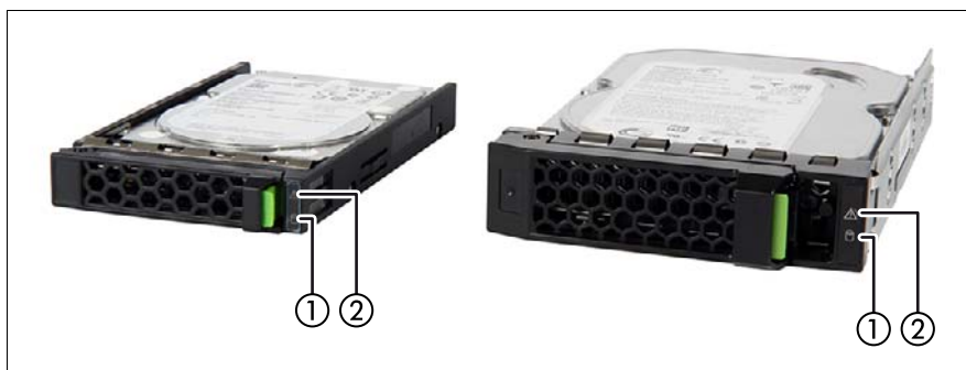
Immagine 10: Spie sul modulo HDD/SSD hot-plug
