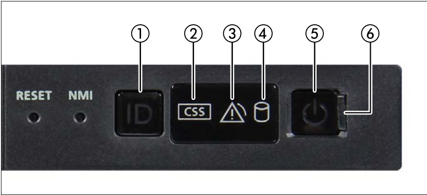
Immagine 8: Spie sul modulo del pannello frontale
