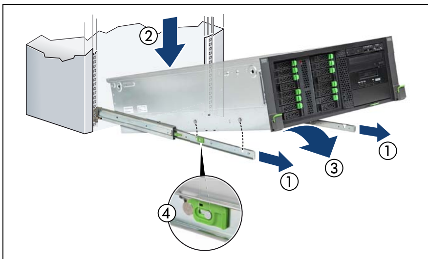
Immagine 18: Installazione del server sulle guide del rack
