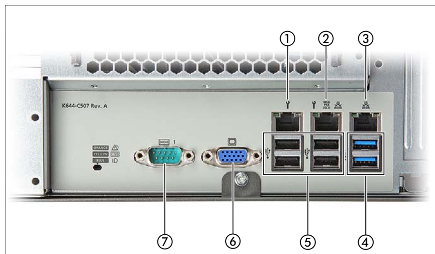
Immagine 6: Connettori sul pannello I/O
