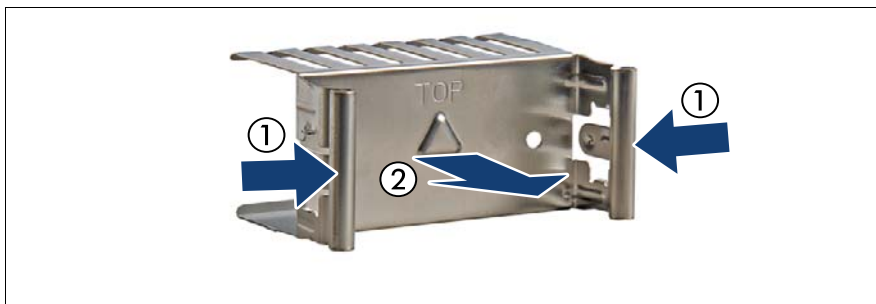
Immagine 30: Rimozione del pannello vuoto di copertura
