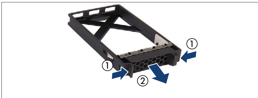
Immagine 24: Rimozione di un modulo vuoto HDD/SSD da 2,5 pollici
