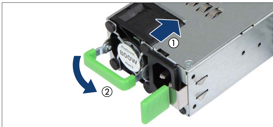
Immagine 32: Installazione dell'unità PSU
