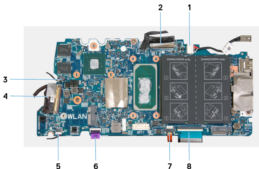
Figure 1. Connecteurs de la carte système
