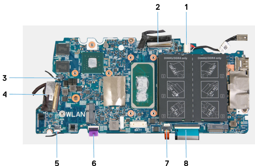
Figure 2. Connecteurs de la carte système
